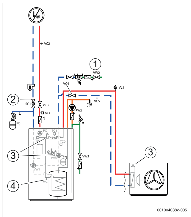
Afb. 24 Binnenunit, warmtepomp en cv-installatie
