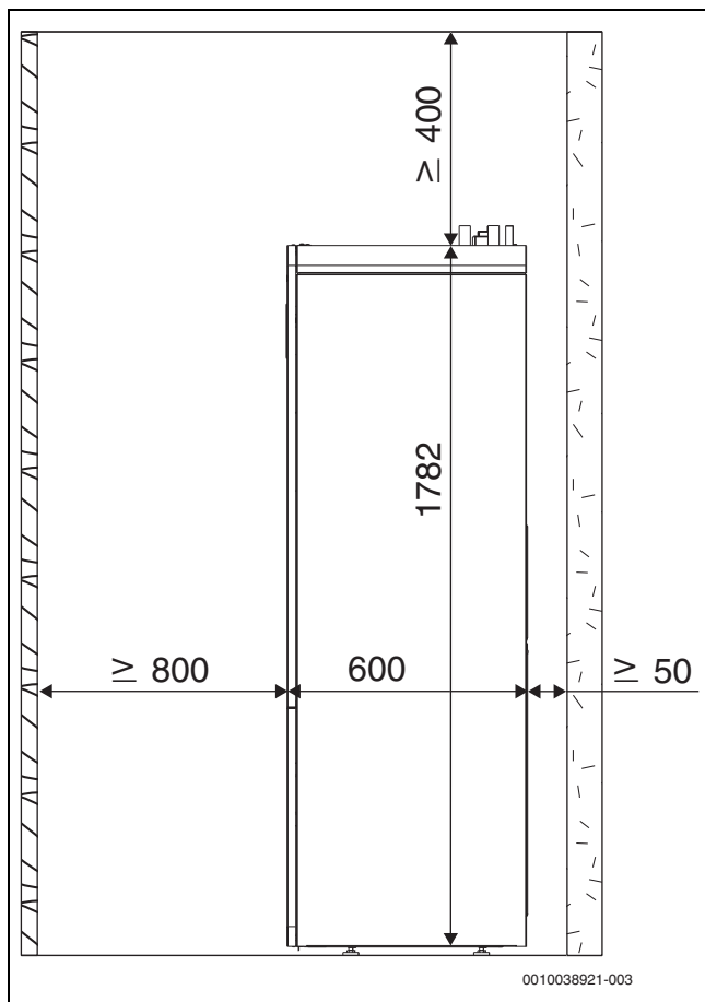
Afb. 2 Minimiavstånd (mm)
