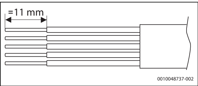
Afb. 30 Aders strippen aansluiting voedingsspanning
