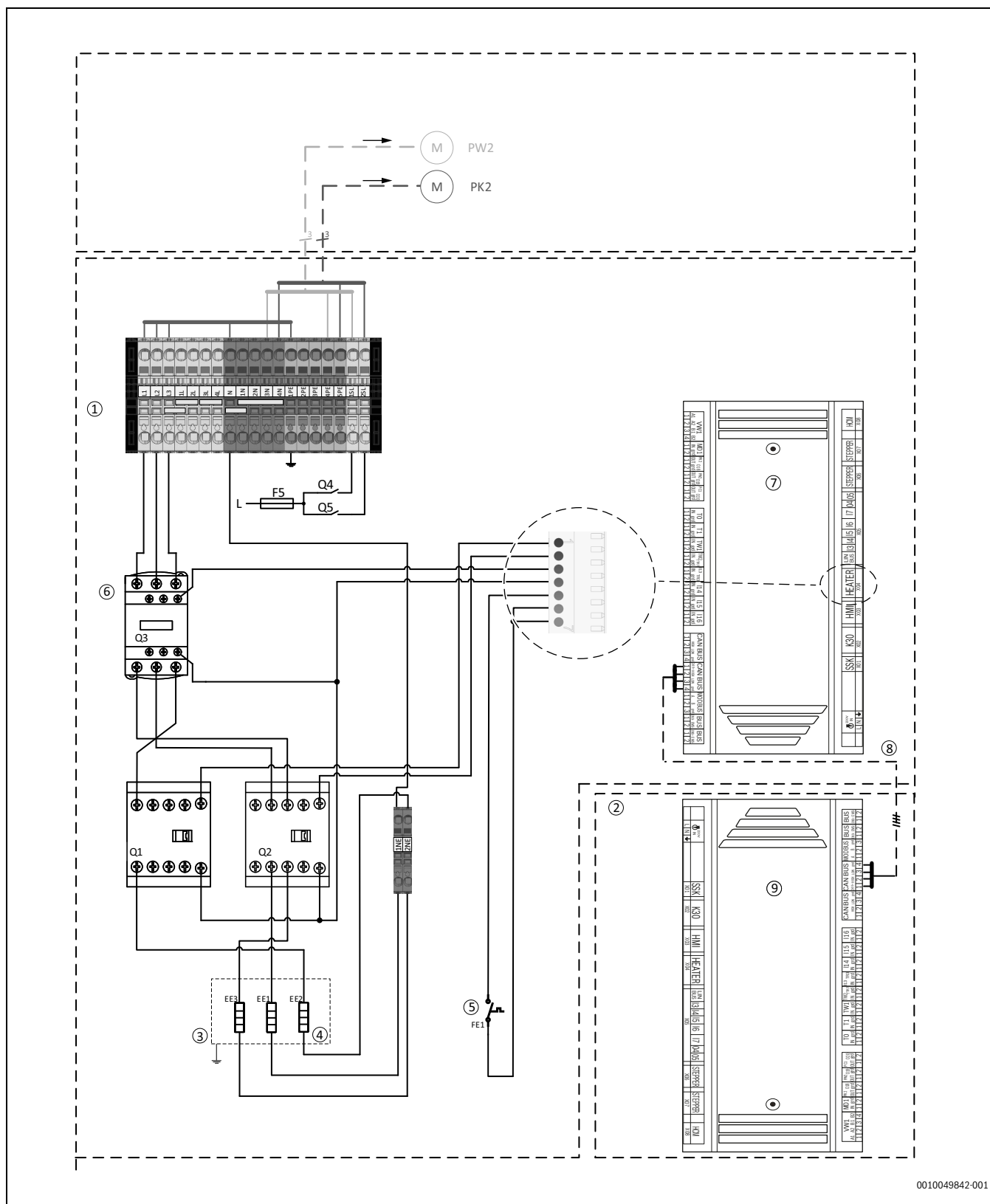
Afb. 46 Voedingsspanning binnenunit
