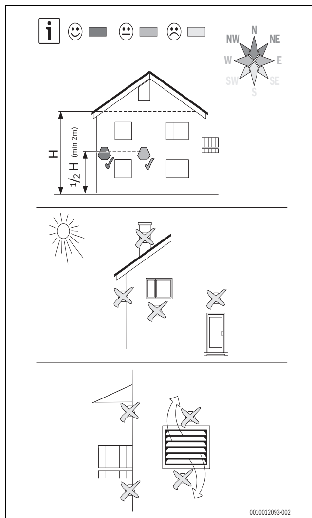
Afb. 29 Positie van de buitentemperatuursensor
