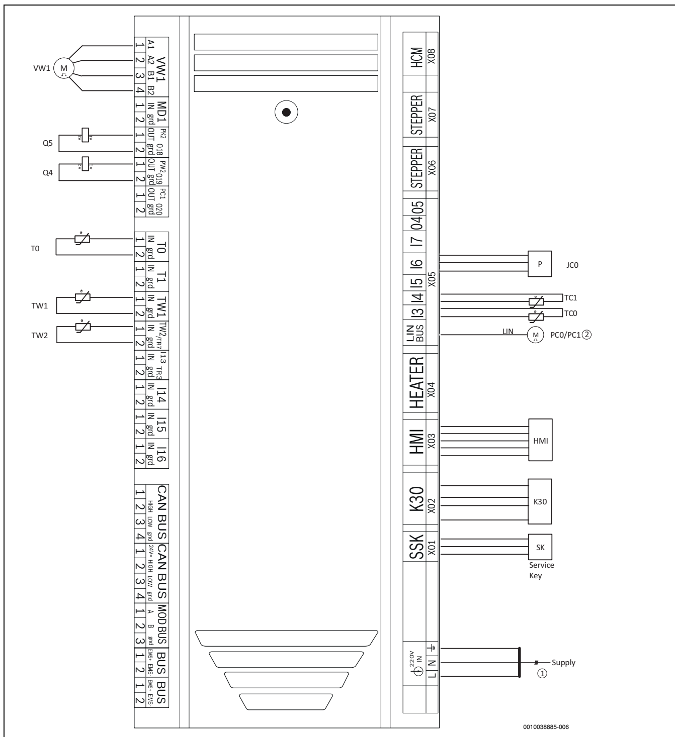
Afb. 45 Elektrisch schema XCU-THH (XCU HY)-module
