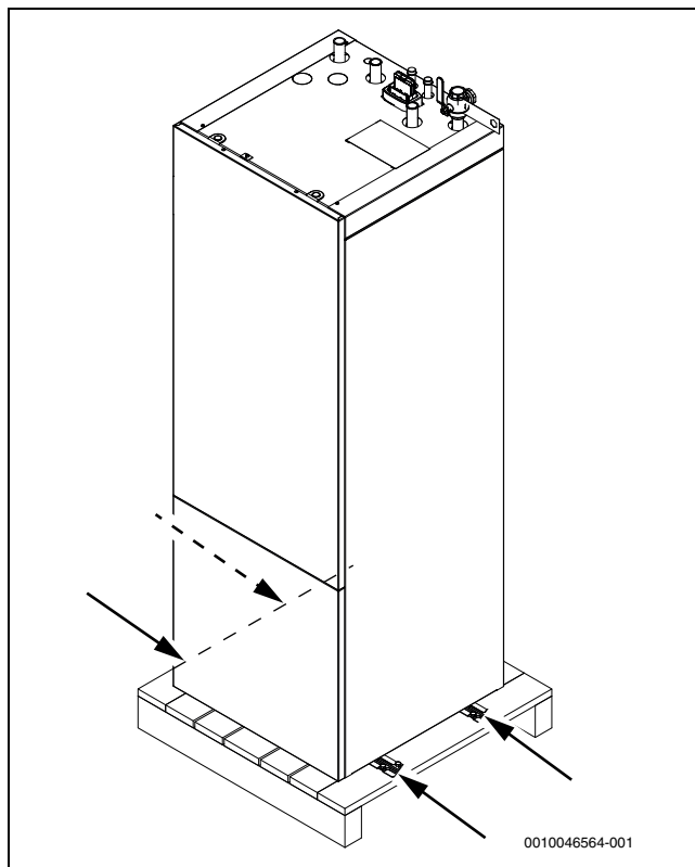
Afb. 9 Verwijder de bouten en de beugels
