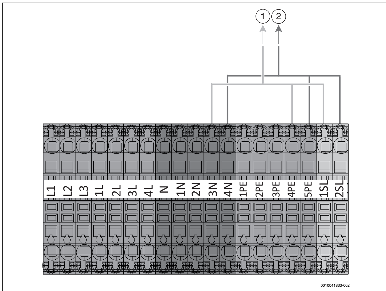
Afb. 36 Elektrische aansluitingen voor accessoires
