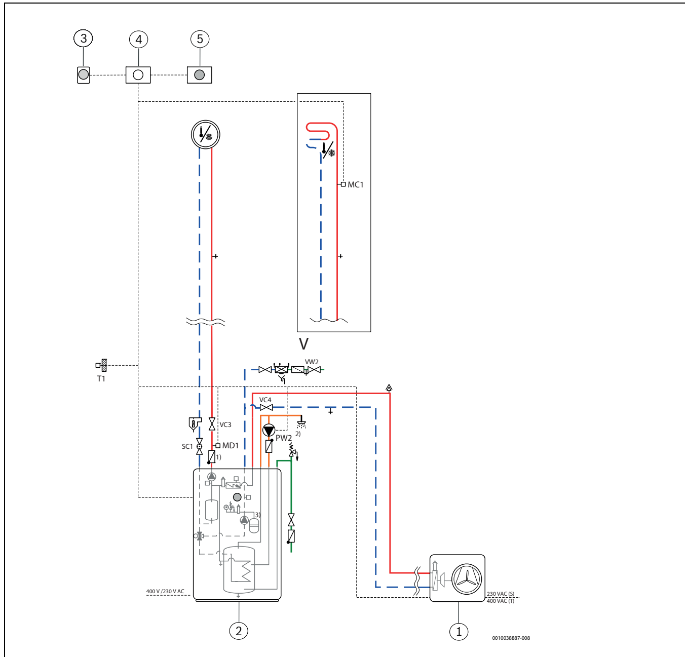
Afb. 43 Binnenunit Tower, warmtepomp (ODU) zonder ongemengde groep
