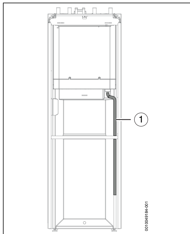
Afb. 22 Achterkant binnenunit
