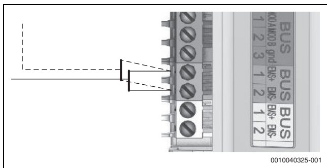
Afb. 28 EMS-verbinding
