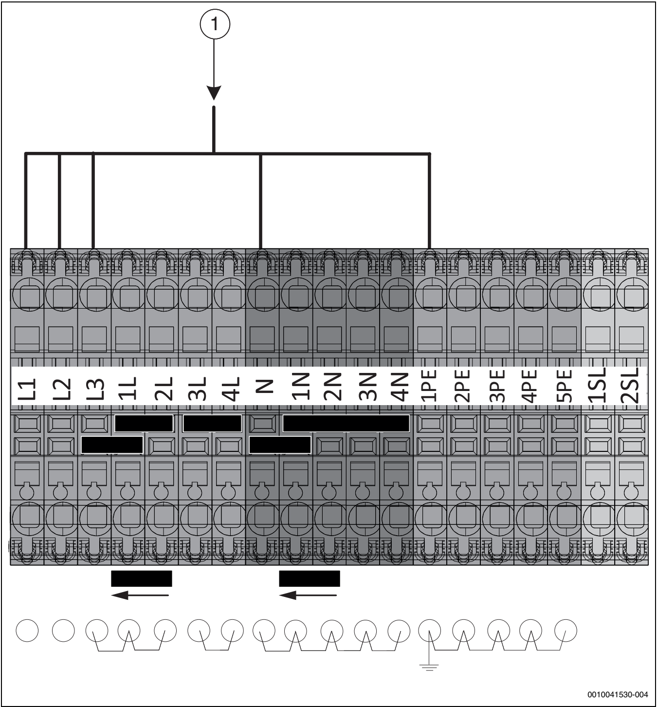
Afb. 34 Elektrische aansluitingen
