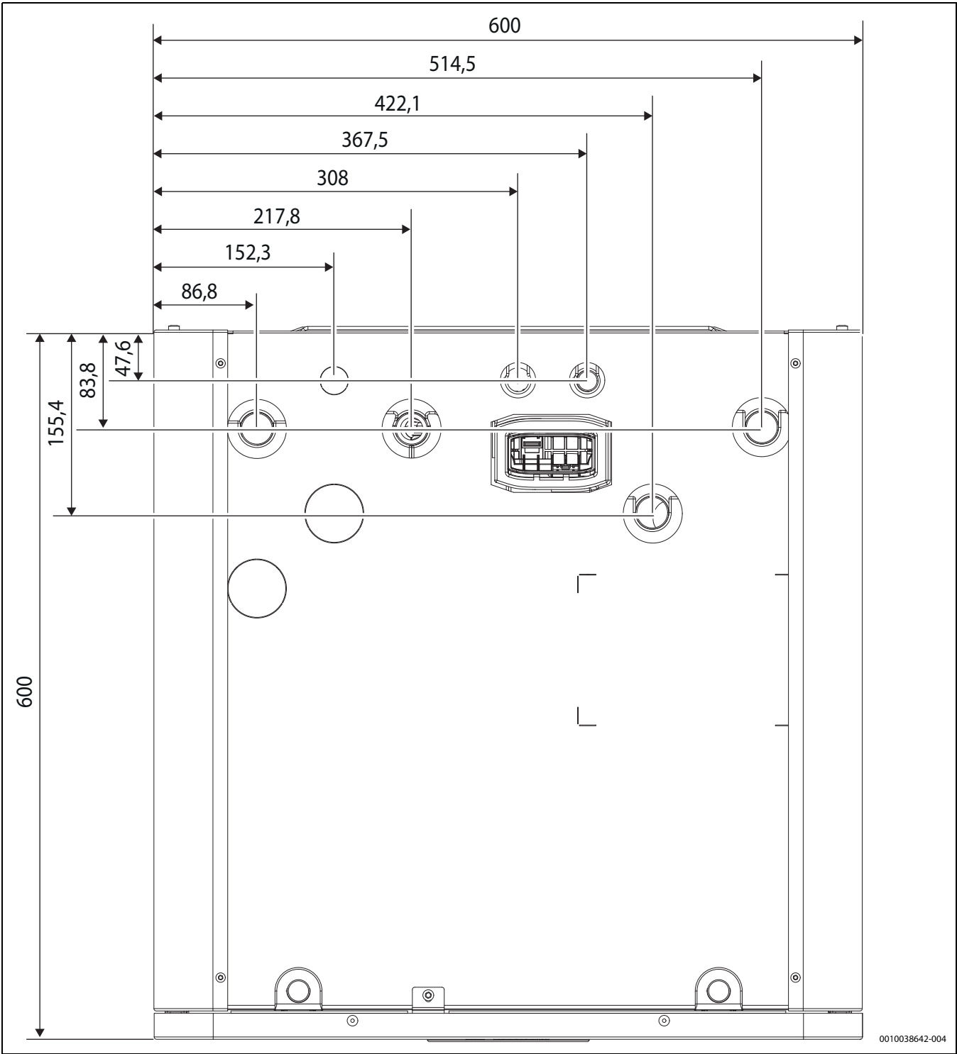
Afb. 4 Mått anslutningar, takvy
