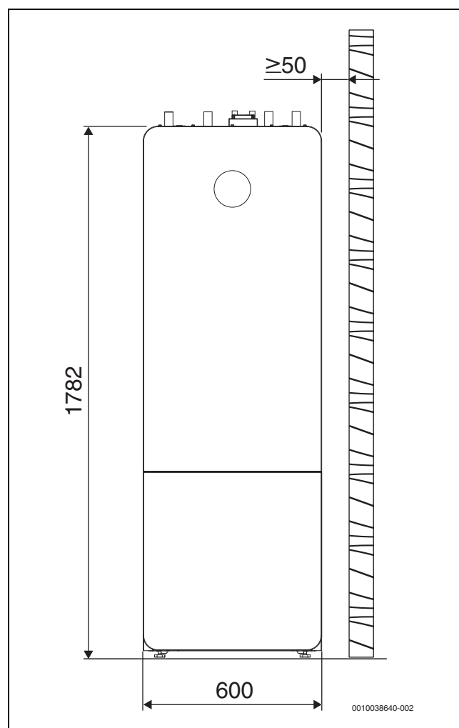
Afb. 3 Mått (mm)
