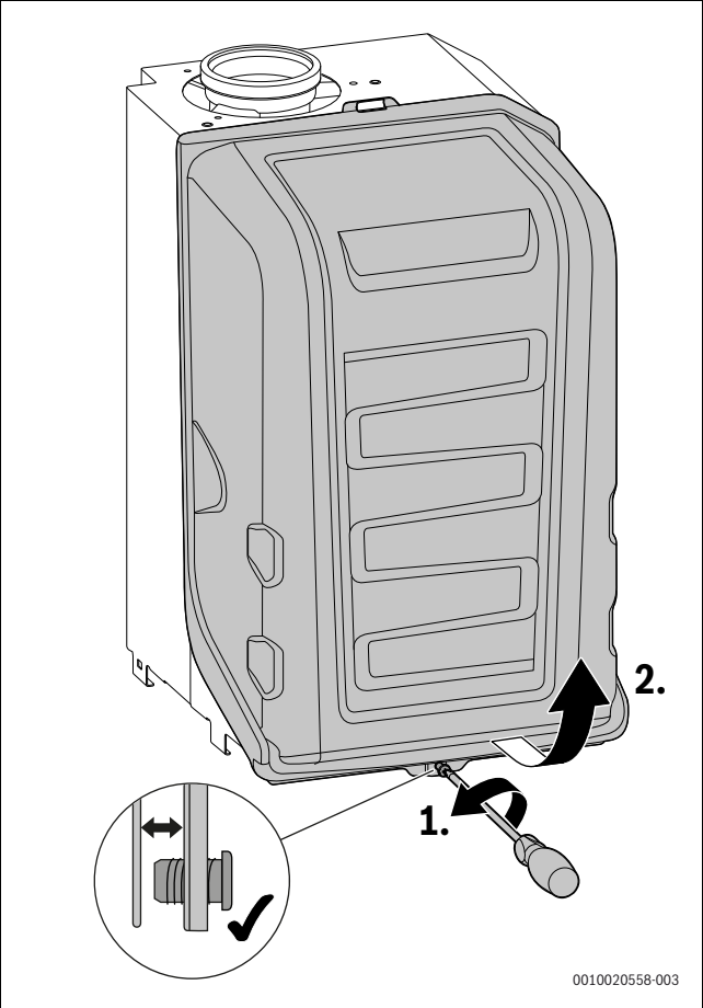
Afb. 33 Branderkap wegnemen
