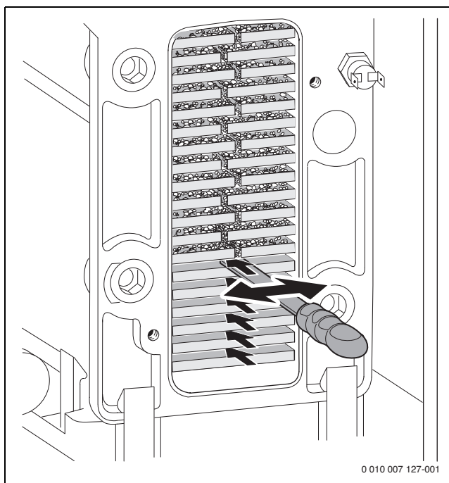
Afb. 45 Reinigingsgereedschap
