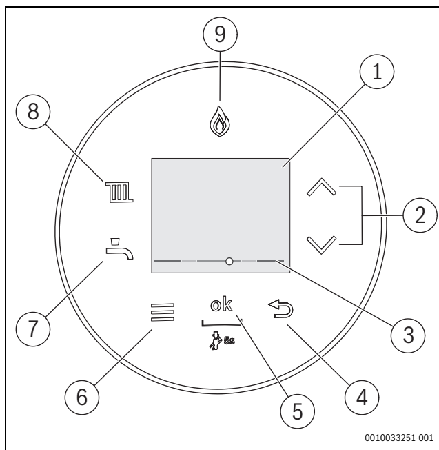
Afb. 31 Bedieningspaneel
