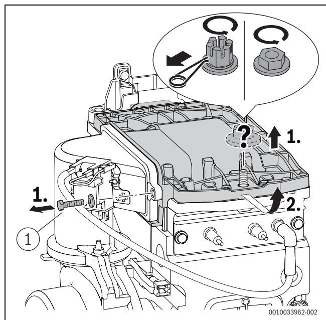
Afb. 39 Demonteer het branderdekseel
