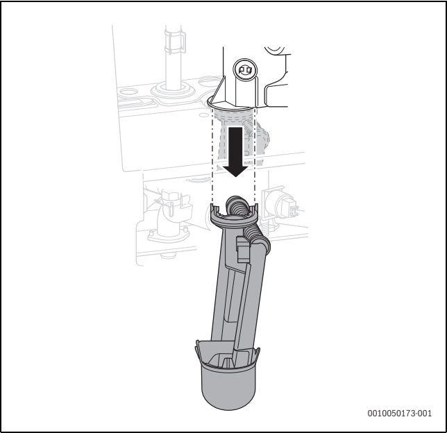
Afb. 49 Sifon
