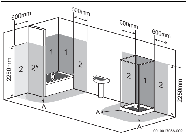
Afb. 13 Veiligheidszone (voorbeeldweergave)
