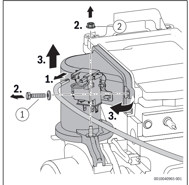
Afb. 42 Menginrichting demonteren
