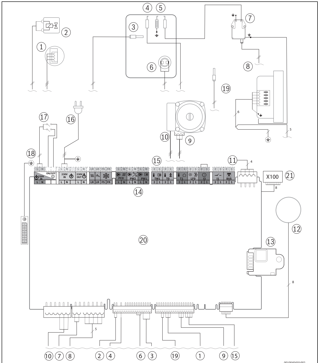
Afb. 55 Elektrische bedrading
