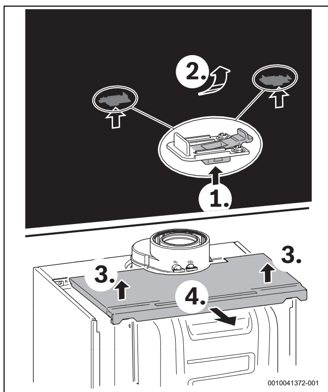
Afb. 30 Mantel (de)monteren
