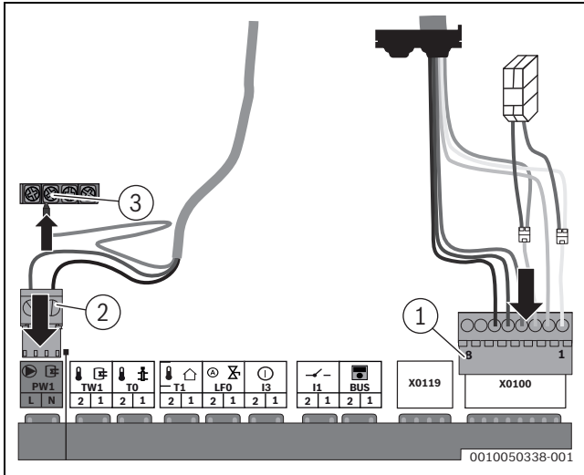
Afb. 23 Boiler aansluiten
