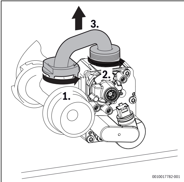
Afb. 50 Gasbuis demonteren
