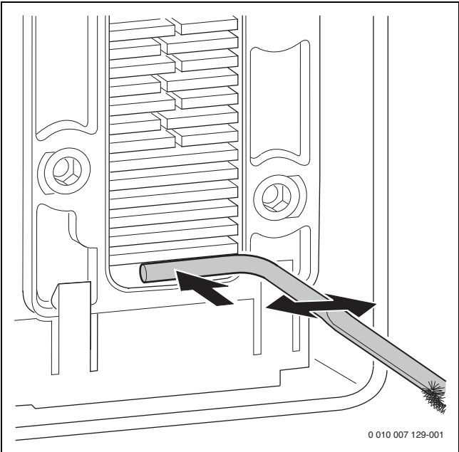
Afb. 48 Condensopvang reinigen
