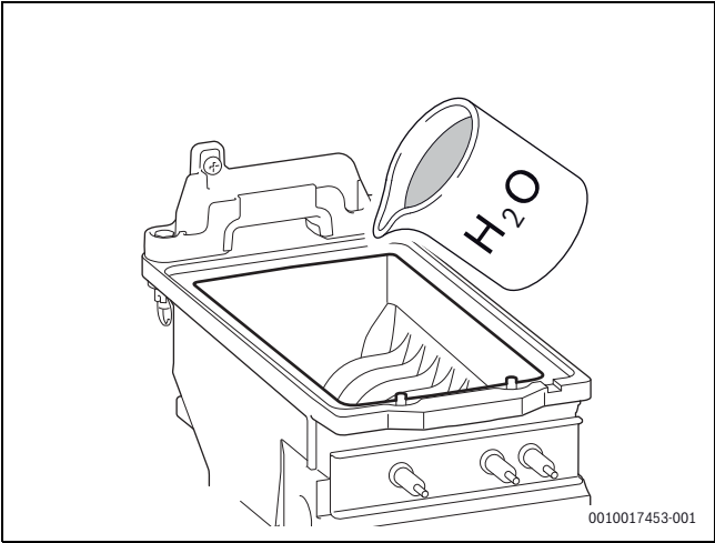
Afb. 47 Verwarmingslichaam spoelen
