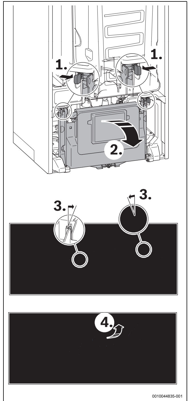
Afb. 24 Open branderautomaat
