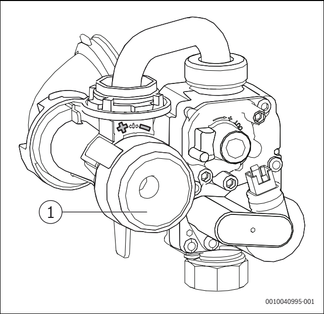
Afb. 34 Gas-luchtverhouding instellen
