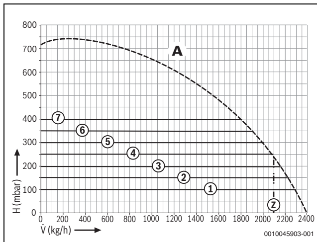
Afb. 54 9700i Aquapower plus HRC 45/CW6: pompkarakteristieken en pompcurves
