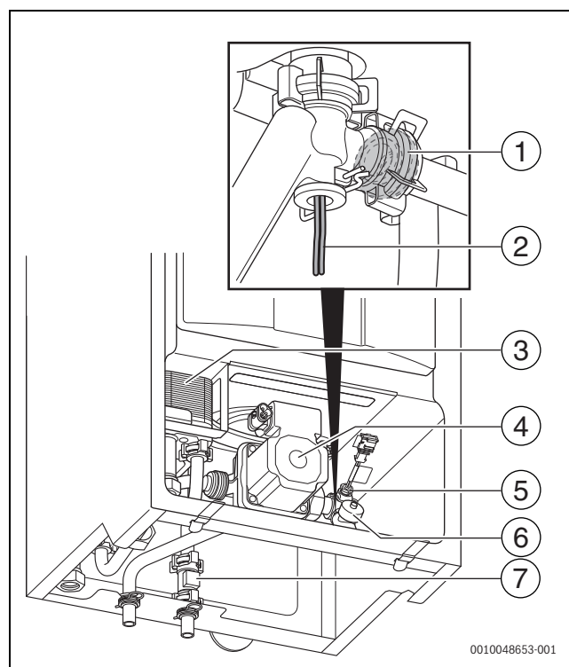
Afb. 11 Toestelsamenstelling T40S
