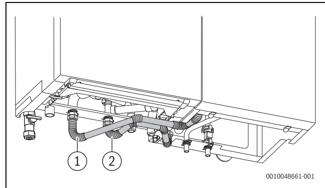
Afb. 18 Boiler en toestel verbinden
