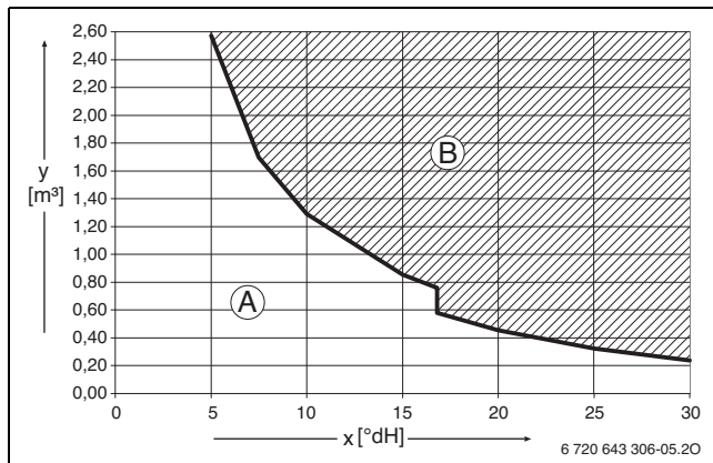
Afb. 14 Eisen aan het vul- en bijvulwater in °dH voor toestellen < 50 kW
