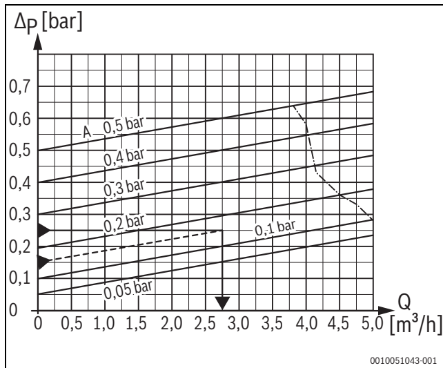
Afb. 46 Instelbereik overstroomventiel
