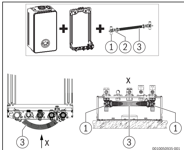
Afb. 26 Bypass/open verdeler (LLH) in het montageframe, optie 3
