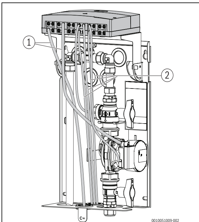
Afb. 29 Elektrische kabels door de bodemplaat installeren (isolatie niet weergegeven, hydraulisch leidingwerk conform optie 2)
