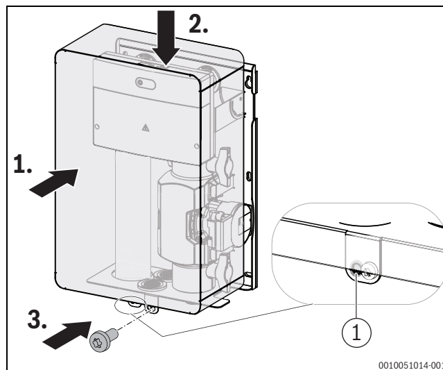
Afb. 39 Voorwand monteren
