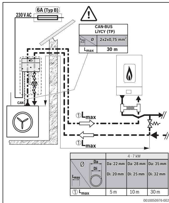
Afb. 10 Eisen aan de kabellengtes (voorbeeldweergave: aan achterkant door de wand)
