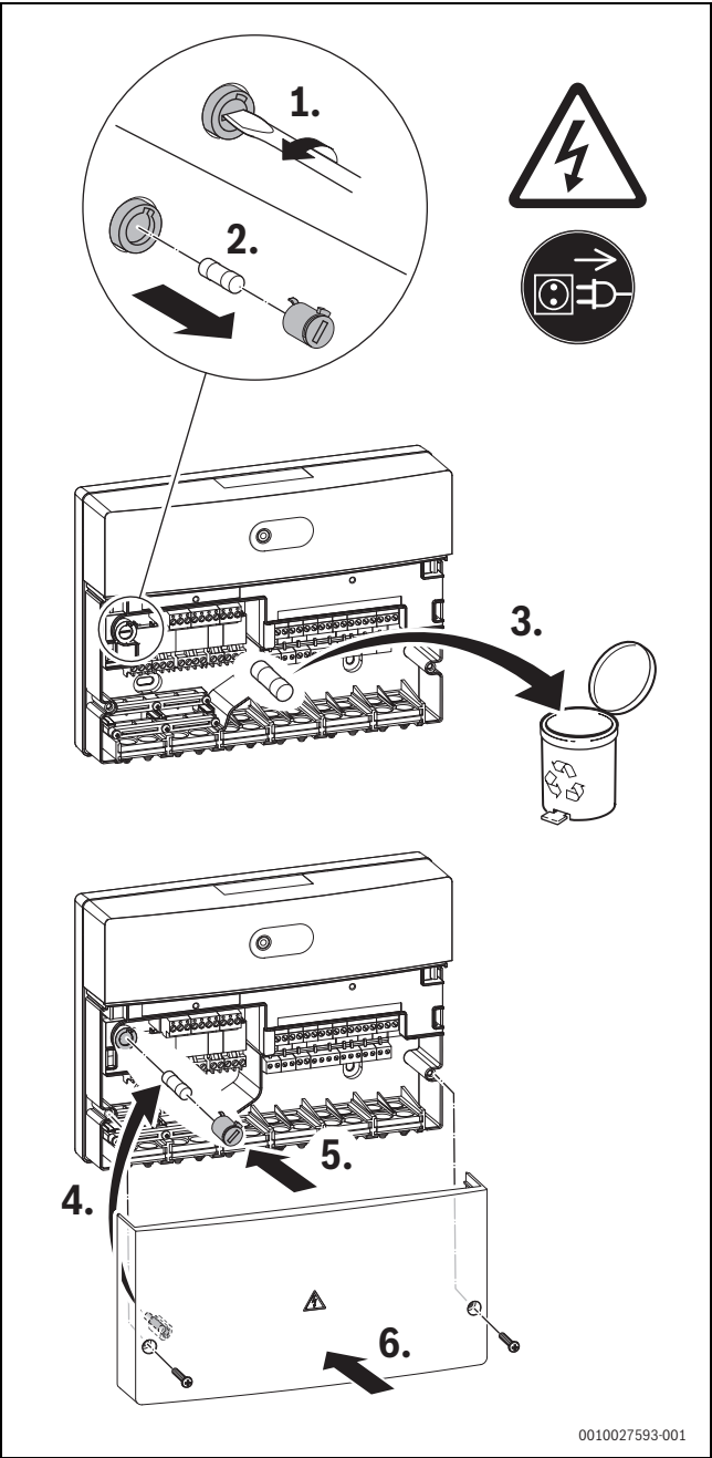
Afb. 55 Zekering vervangen
