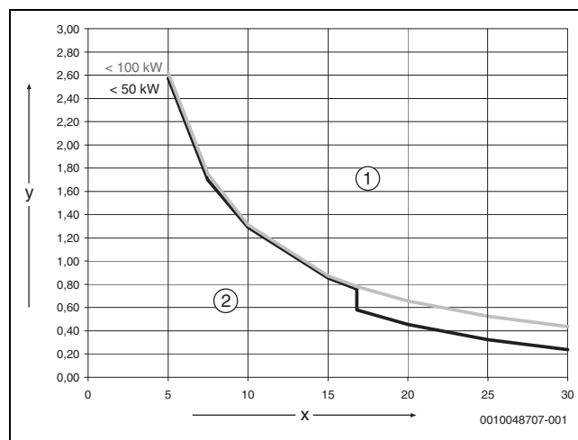
Afb. 40 Warmtebronnen < 50 kW < 100 kW
