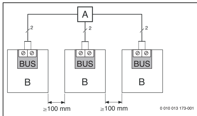
Afb. 36 Verdeeldoos aansluiten
