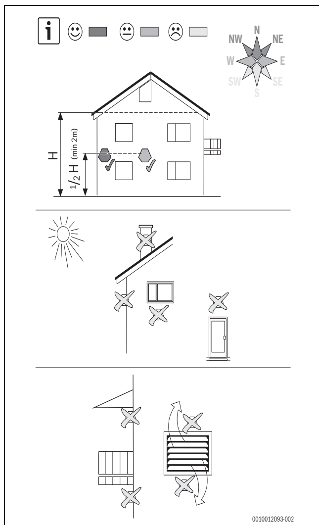
Afb. 35 Plaatsing van de buitentemperatuursensor
