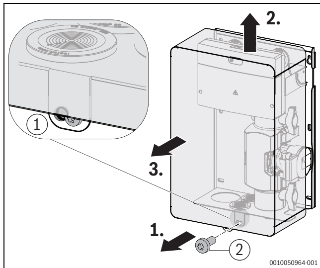
Afb. 14 Voorwand verwijderen
