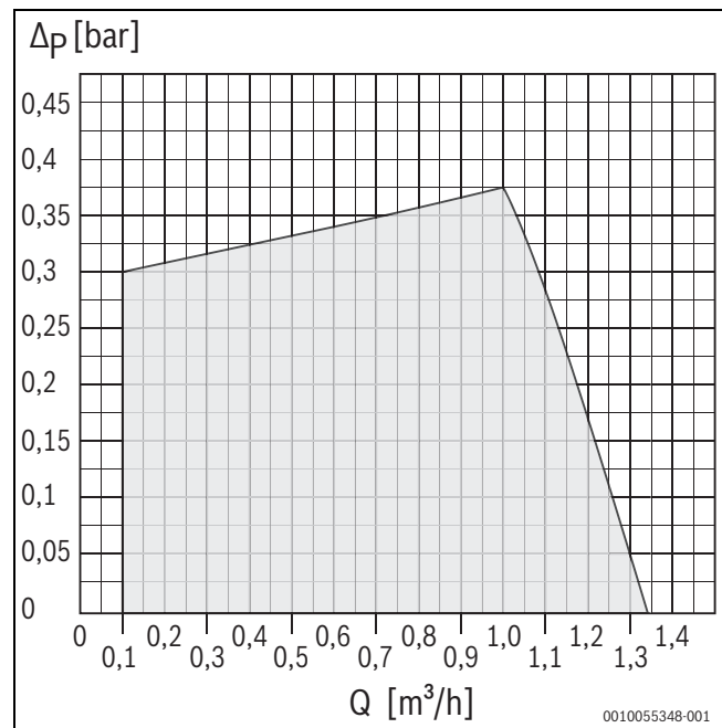
Afb. 49 Restopvoerhoogte pomp, 0,3 bar (300 mbar)
