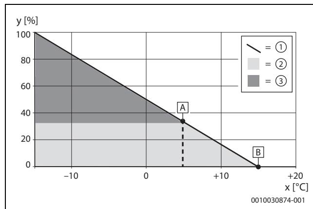
Afb. 41 Regelstrategie aandeel hernieuwbare energie maximaliseren
