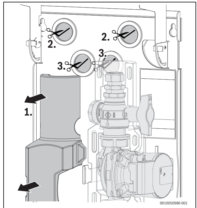
Afb. 20 Isolerende halfschaal verwijderen, doorvoertules insnijden (hybride manager is niet afgebeeld)
