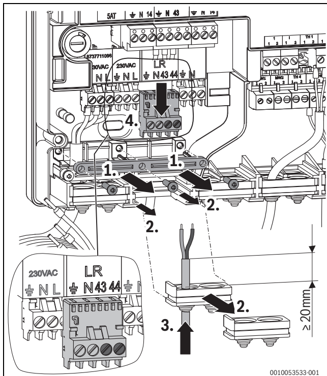
Afb. 32 Aansluiting voedingsspanning 230 V externe regelaar (PH0-leiding niet weergegeven)
