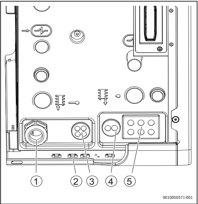
Afb. 25 Kabeldoorvoer naar de binnenunit
