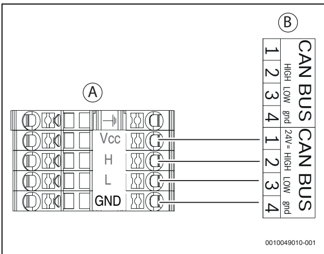
Afb. 20 CAN-BUS warmtepomp - binnenunit
