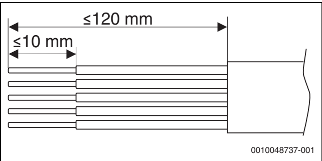
Afb. 24 Aders strippen aansluiting voedingsspanning
