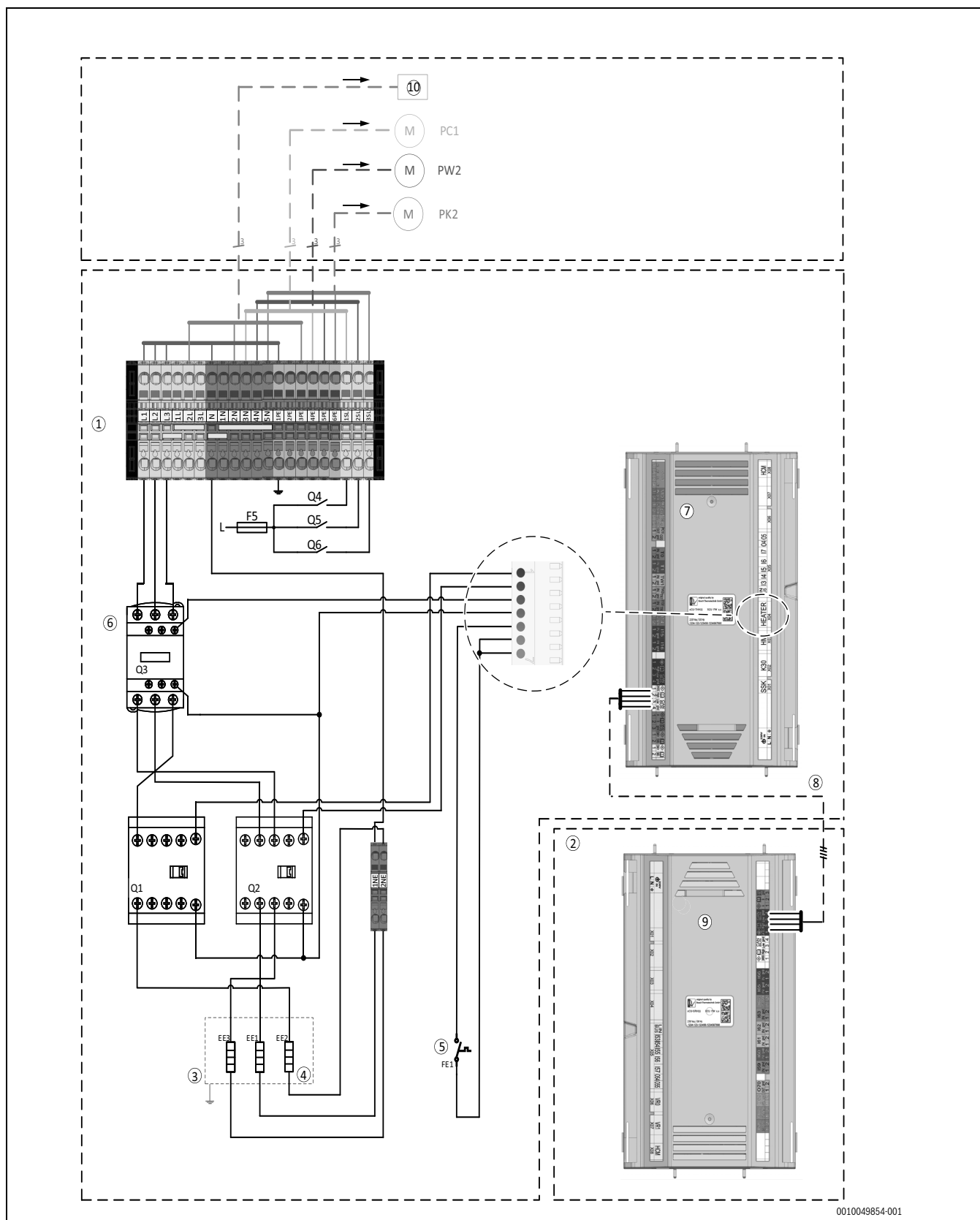
Afb. 41 Voedingsspanning binnenunit, standaard
