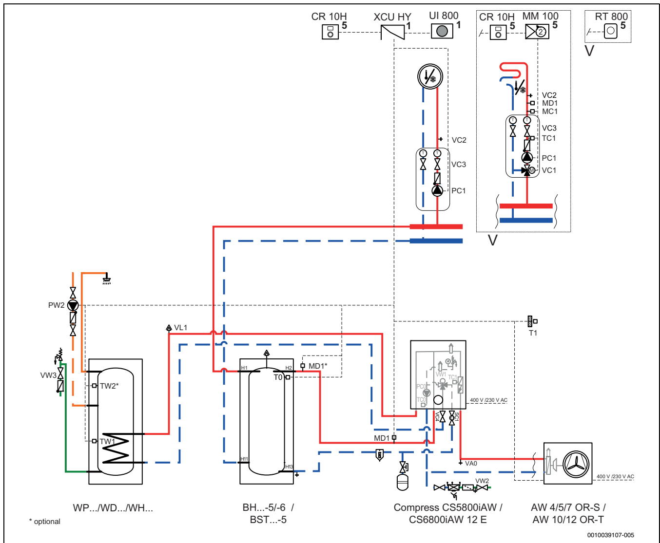
Afb. 37 Warmtepomp, binnenunit, buffervat en boiler
