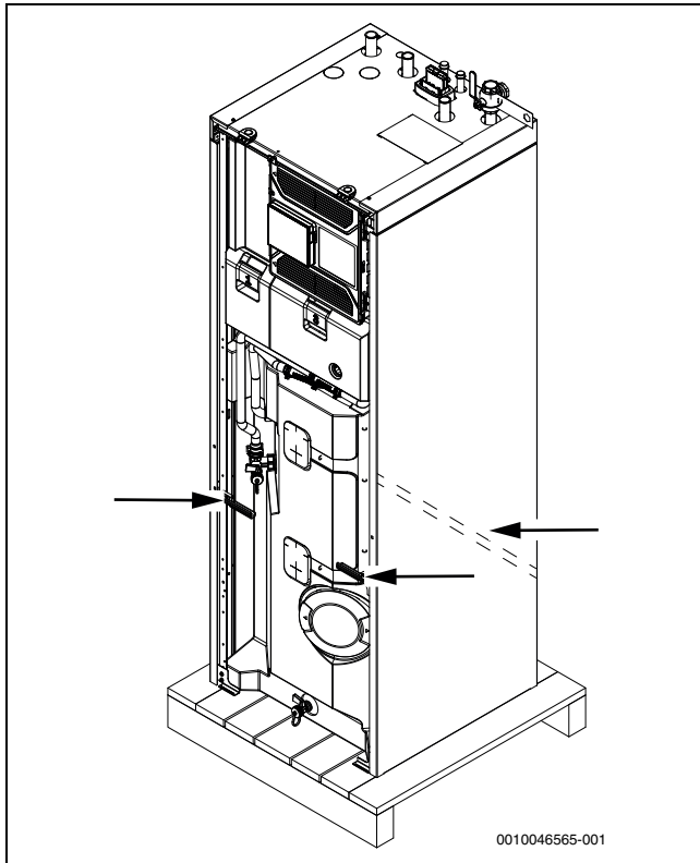
Afb. 10 Draagbeugels
