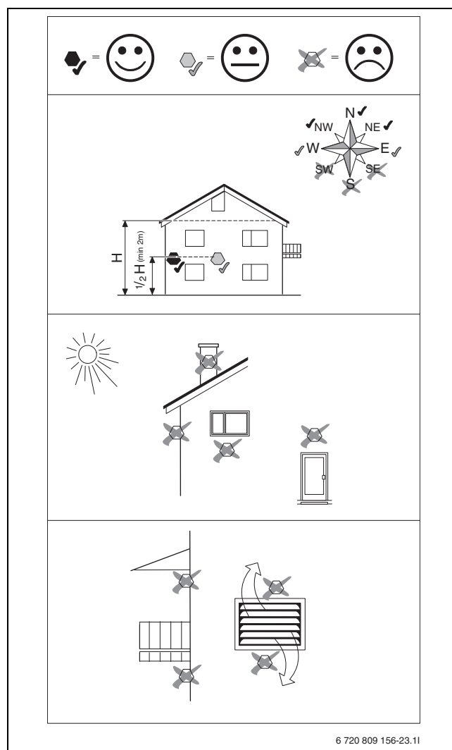
Afb. 28 Positie van de buitentemperatuursensor
