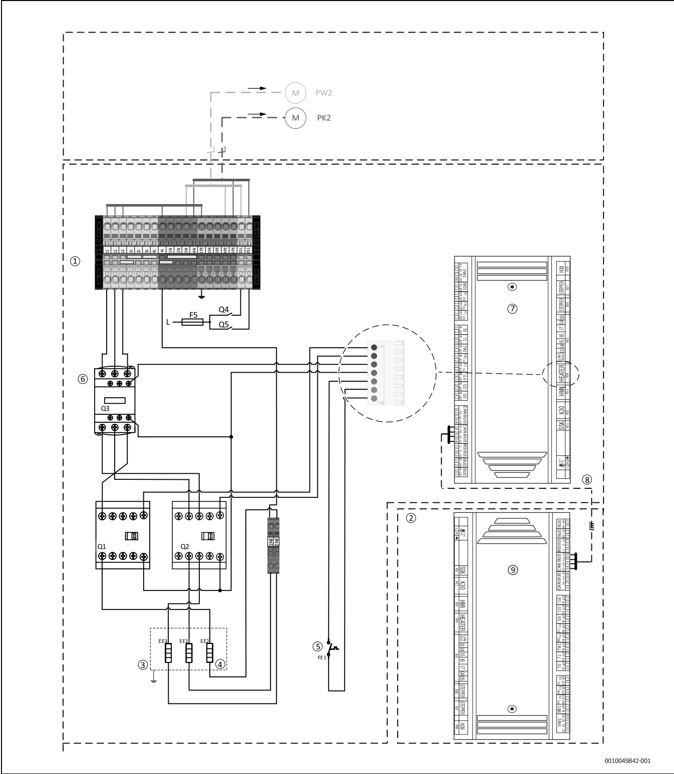
Afb. 45 Voedingsspanning binnenunit
