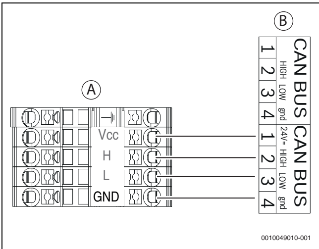
Afb. 25 CAN-BUS warmtepomp - binnenunit
