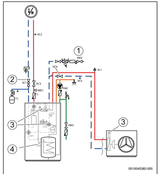
Afb. 24 Binnenunit, warmtepomp en cv-installatie
