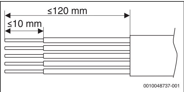
Afb. 29 Aders strippen aansluiting voedingsspanning
