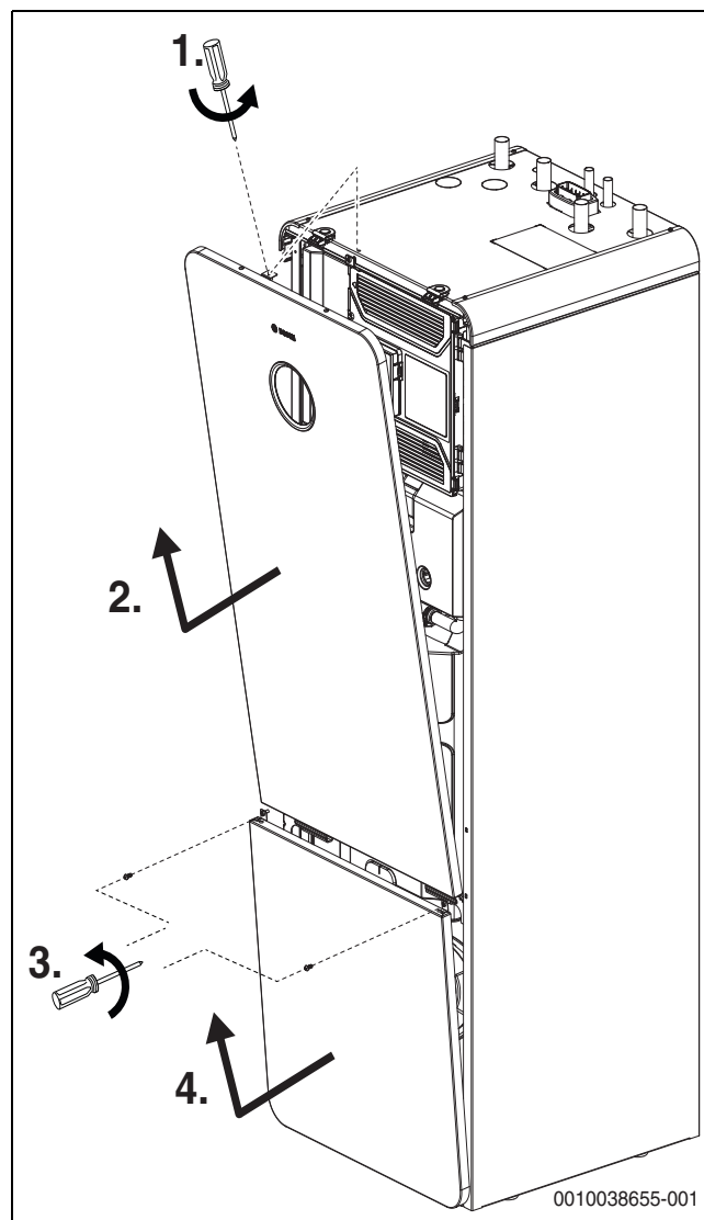
Afb. 16 Verwijder de voorkant
