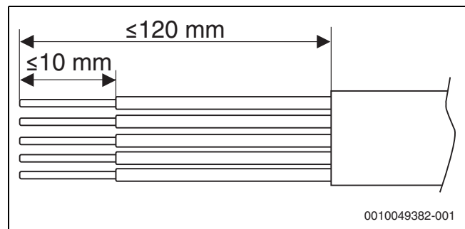
Afb. 33 Strippen van de aders voor de netaansluiting
