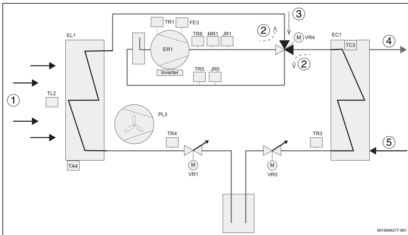
Afb. 42 Koelmiddelcircuit
