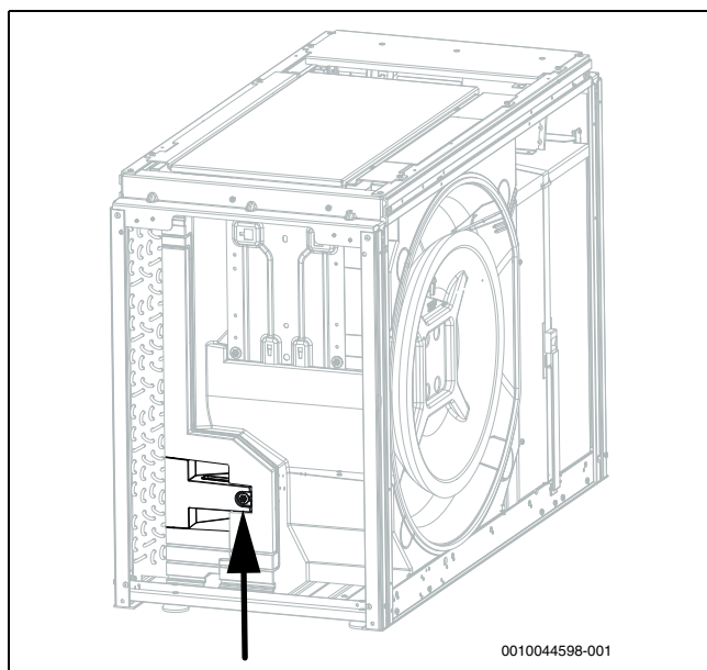
Afb. 36 Losschroeven
