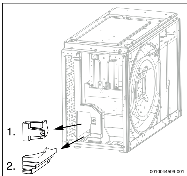
Afb. 37 EPP-onderdelen
