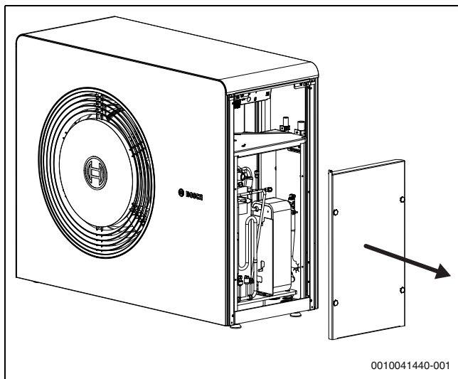
Afb. 28 Deksel koudemiddelmodule
