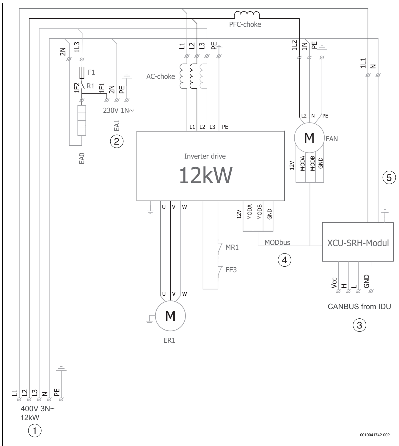
Afb. 43 Elektrisch schema
