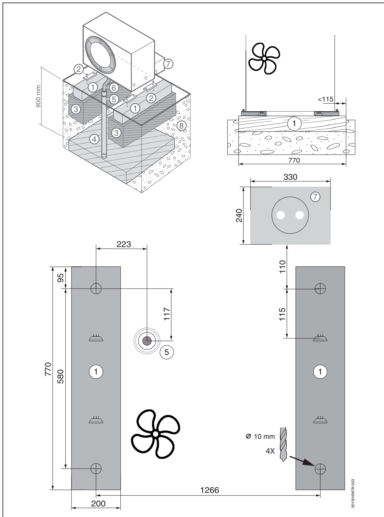
Afb. 21 Funderingsschema, alternatief 1
