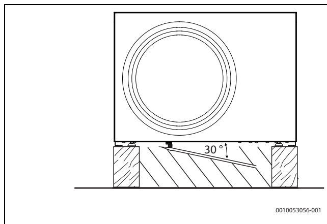
Afb. 23 Installatie van de kabel voor de druipschaalverwarming
