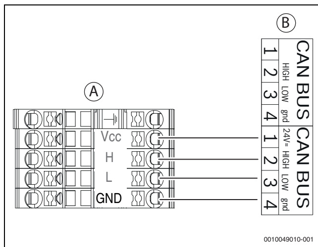
Afb. 30 CAN-BUS warmtepomp - binnenunit
