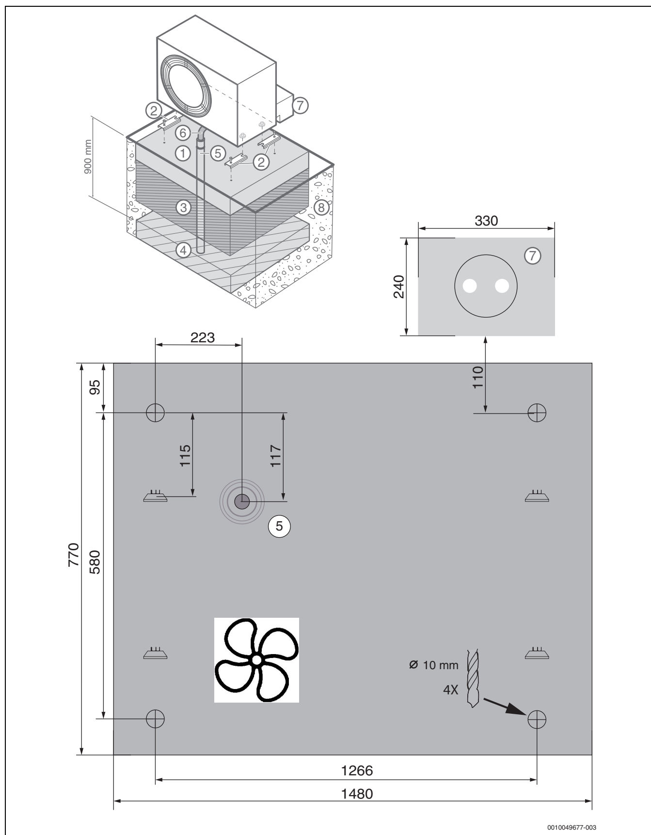
Afb. 22 Funderingsschema, alternatief 2
