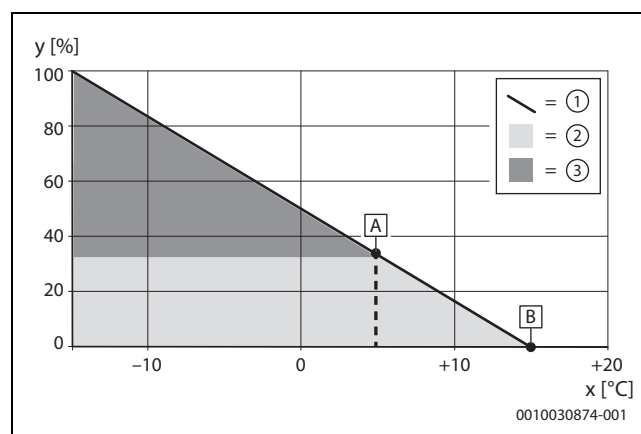
Afb. 31 Regelstrategie aandeel hernieuwbare energie maximaliseren
