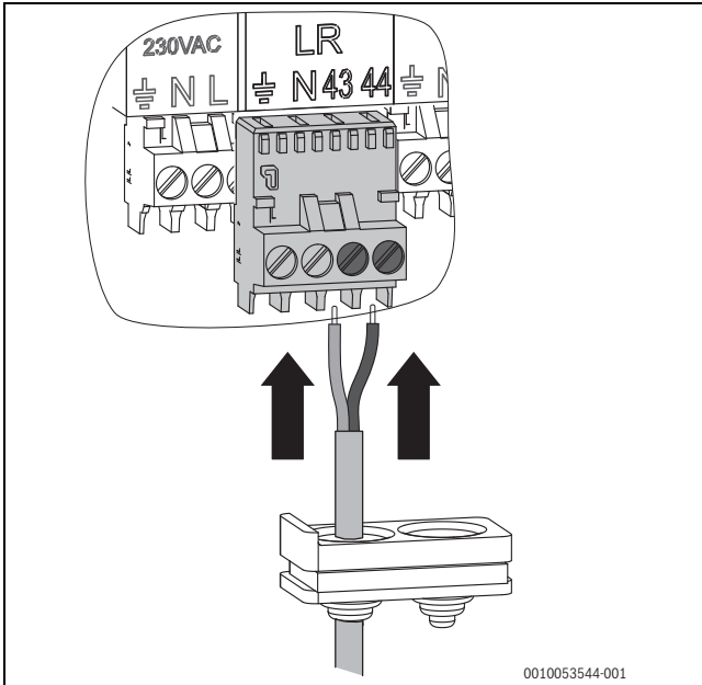
Afb. 25 Aansluitkabel externe regelaar op de klemmen aansluiten
