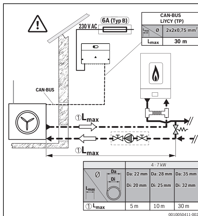
Afb. 8 Eisen aan de kabellengtes
