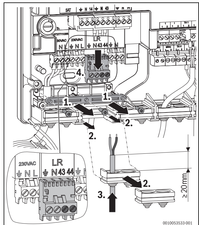
Afb. 24 Aansluiting voedingsspanning 230 V externe regelaar (PH0-leiding niet weergegeven)
