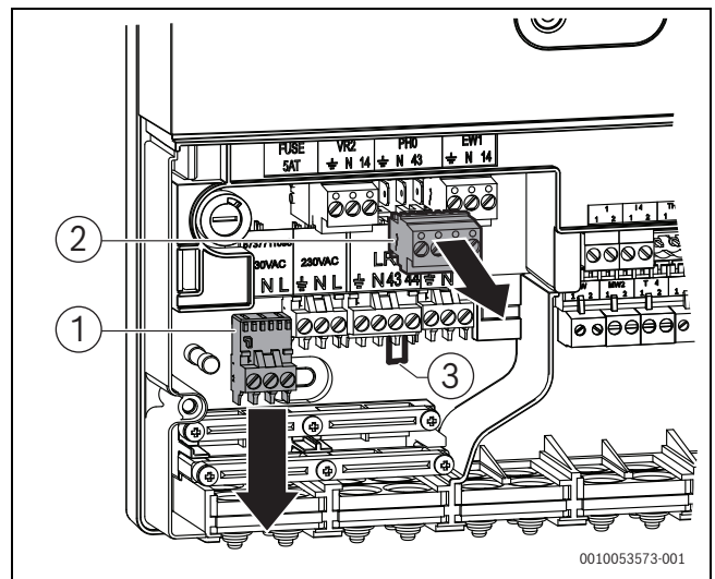
Afb. 21 Aansluitklemmen voedingsspanning 230 V lostrekken
