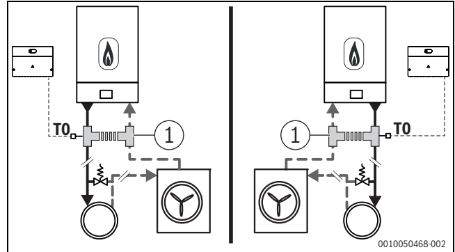
Afb. 10 Bypass/open verdeler (LLH) in de installatie, optie 1
