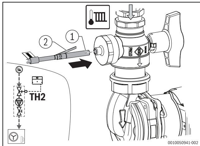
Afb. 14 Temperatuursensor TH2 monteren (voorbeeld)
