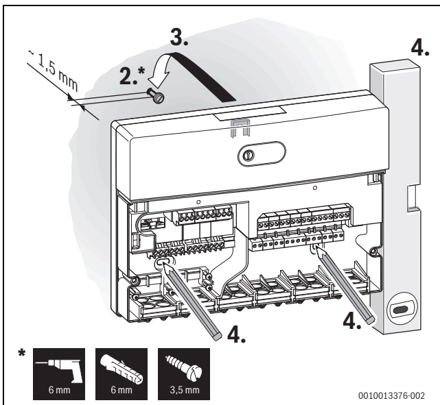
Afb. 17 Wandbevestiging markeren
