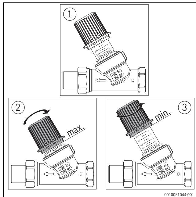
Afb. 37 Instelling overstroomventiel
