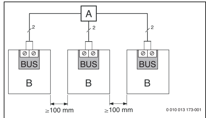
Afb. 28 Verdeeldoos aansluiten
