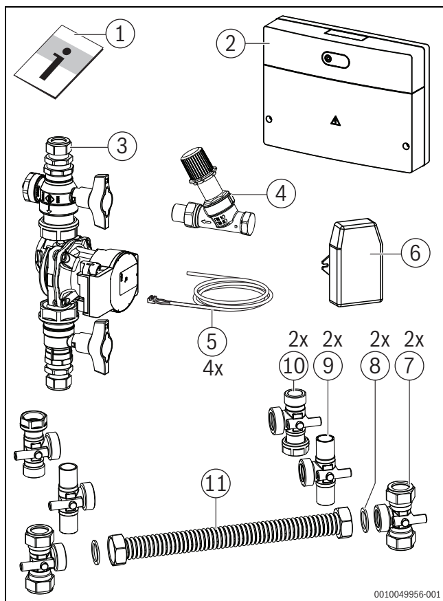
Afb. 1 Leveringsomvang CSH5800iAW
