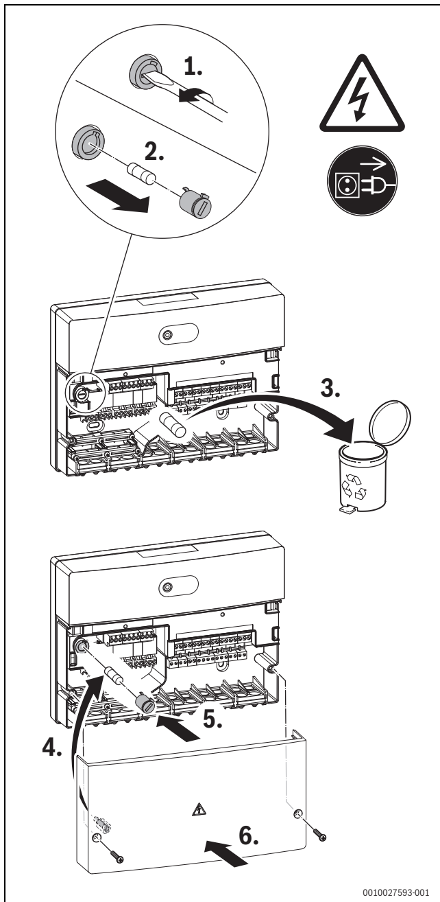
Afb. 45 Zekering vervangen
