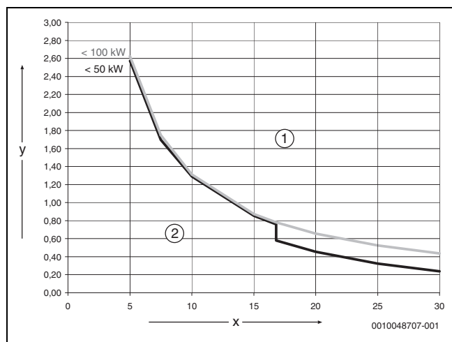
Afb. 30 Warmtebronnen &lt; 50 kW &lt; 100 kW
