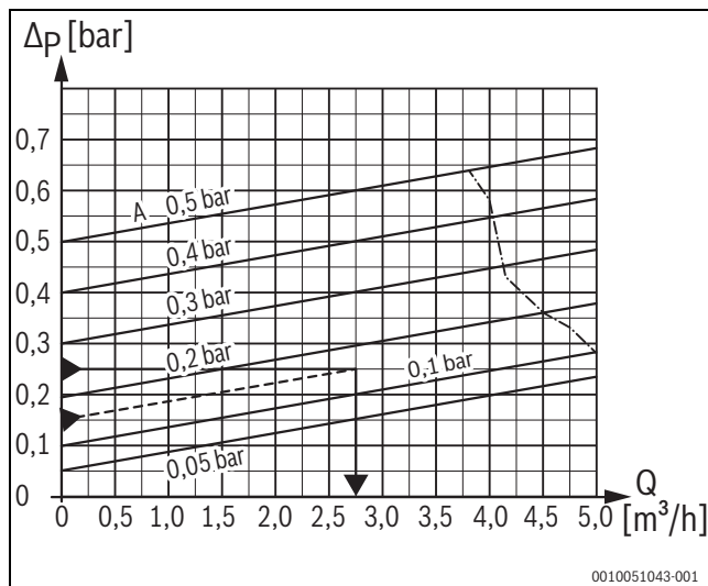
Afb. 36 Instelbereik overstroomventiel
