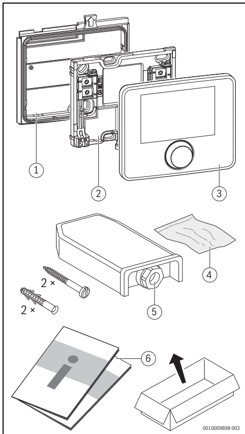
Afb. 3 Leveringsomvang
