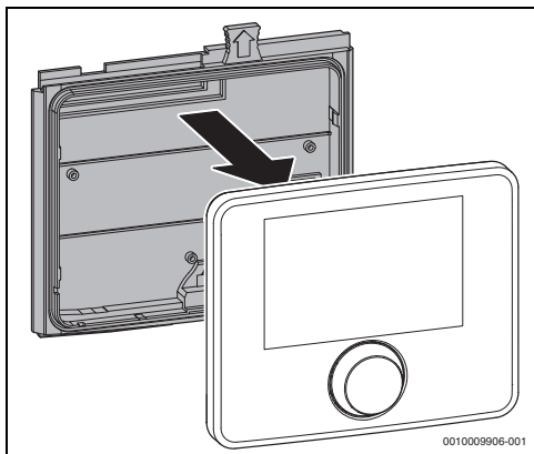
Afb. 12 Inbouwframe aan de achterzijde van de bedieningsunit aanbrengen
