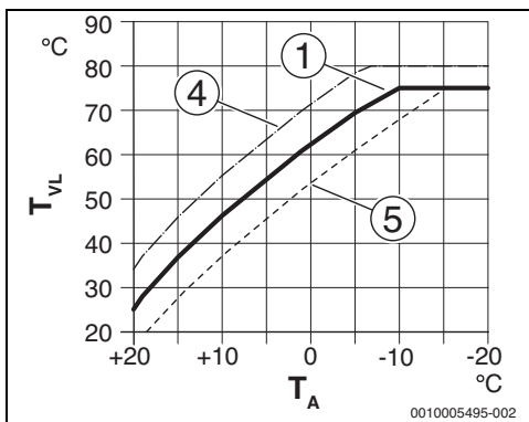
Afb. 19 Instelling van de stooklijn voor radiator Parallelverschuiving via Offset ruimtetemperatuur of gewenste kamertemperatuur
