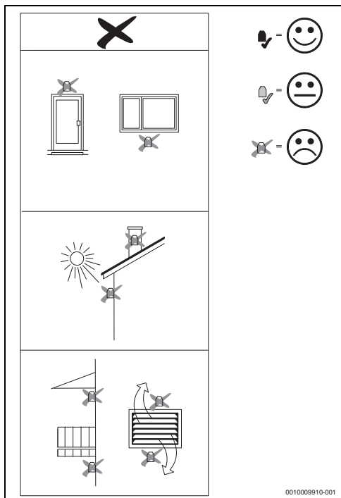
Afb. 14 Ongeschikte installatieplaats van de buitentemperatuursensor
