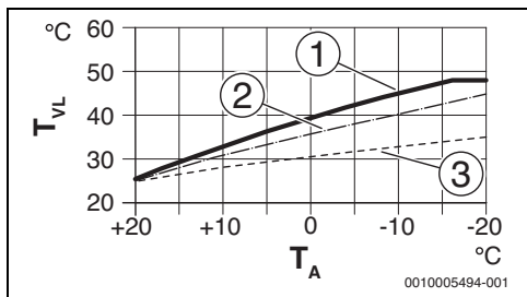
Afb. 16 Instelling van de stooklijn voor vloerverwarming Stijging via dimensioneringstemperatuur T_{AL} en minimale buitentemperatuur T_{A,min}
