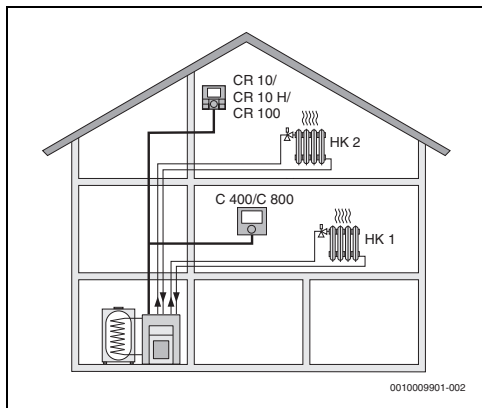
Afb. 2 CR 10/CR 10 H/CR 100 als afstandsbediening voor de tweede cv-groep (HK 2) en C 400/C 800 als regelaar voor de eerste cv-groep (HK 1)
