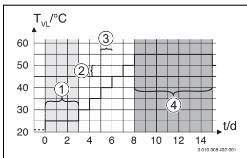
Afb. 20 Verloop van het drogen afwerkvloer met de fabrieksinstellingen in de opwarmfase
