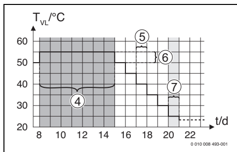
Afb. 21 Verloop van het drogen afwerkvloer met de fabrieksinstellingen in de afkoelfase
