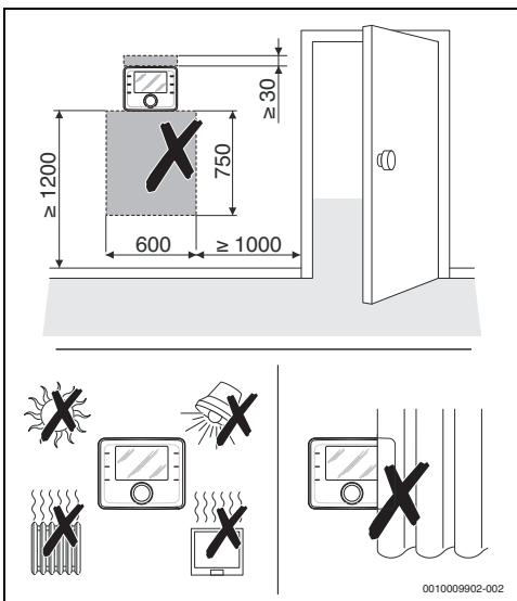
Afb. 5 Installatieplaats in de referentieruimte
