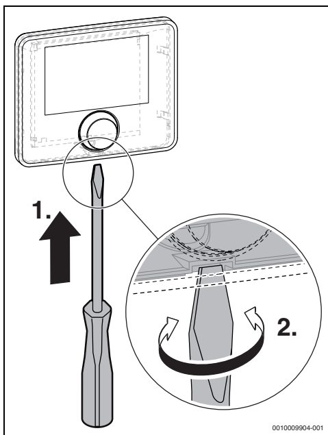
Afb. 10 Afdekking aan de achterzijde van de bedieningsunit losmaken
