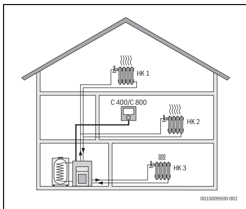
Afb. 1 C 400/C 800 als regelaar voor meerdere (hier drie) cv-groepen
