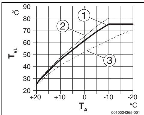
Afb. 18 Instelling van de stooklijn voor radiator Stijging via dimensioneringstemperatuur T_{AL} en minimale buitentemperatuur T_{A,min}
