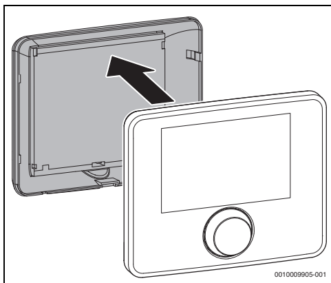
Afb. 11 Afdekking van de achterzijde van de bedieningsunit verwijderen
