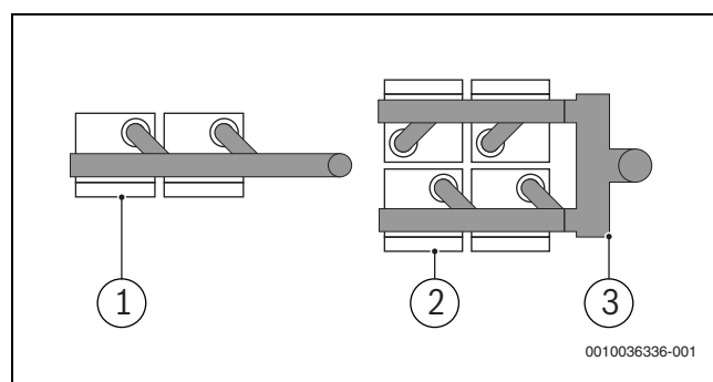
Afb. 22 Bovenanzicht cascadeopstelling
