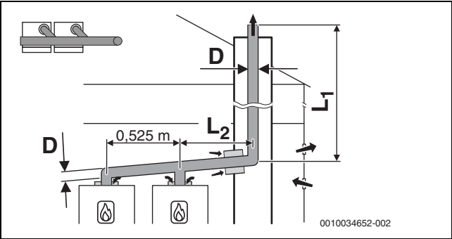
Afb. 23 B 23p /B 53p
