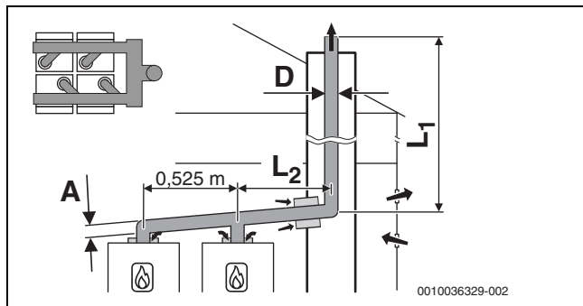
Afb. 26 B 23p /B 53p
