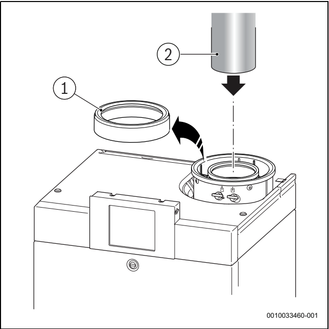
Afb. 5 Enkele buisaansluiting (open systeem)
