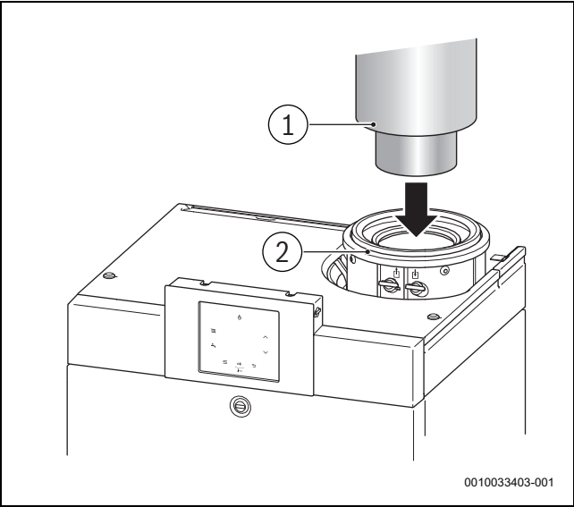
Afb. 1 Concentrische buis (gesloten systeem)
