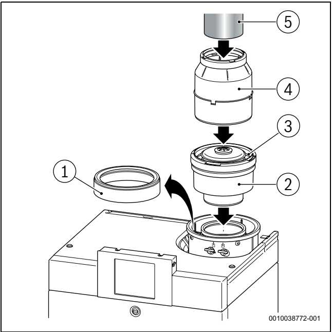
Afb. 6 Monteren externe rookgaskeerklep
