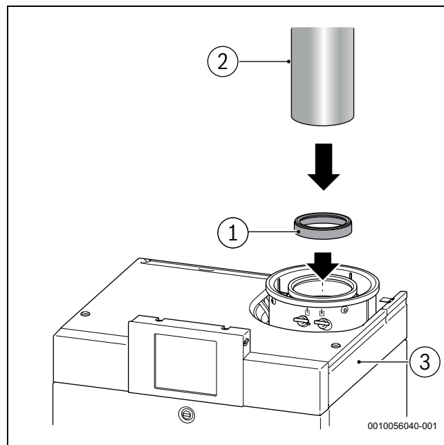
Afb. 4 Monteren rookgasafvoeradapter Ø 110-100
