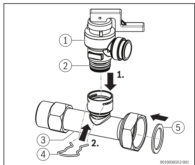
Afb. 6 Montage overstortventiel
