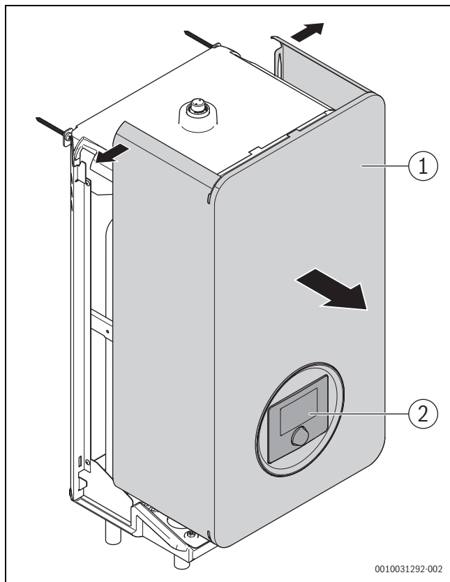
Afb. 13 Afdekkap verwijderen
