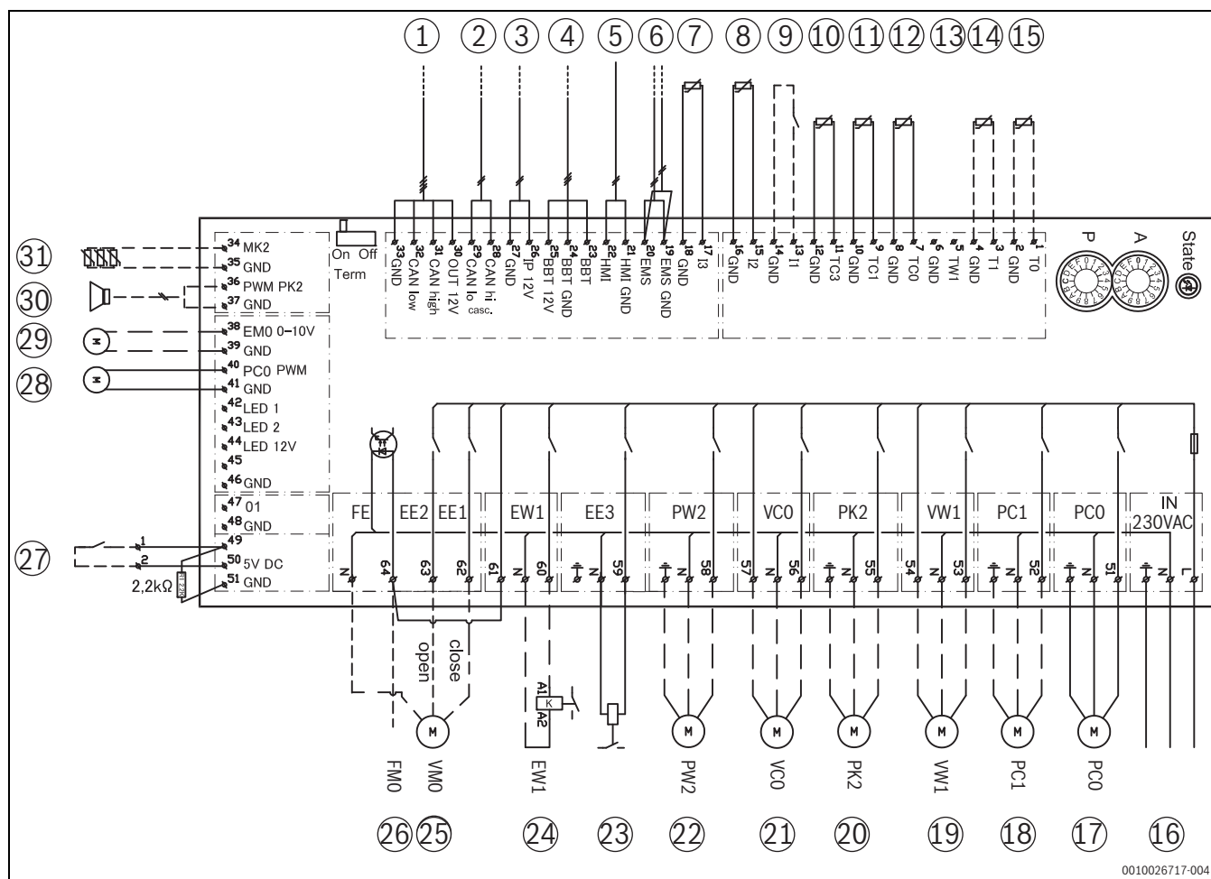
Afb. 45 Aansluitschema installatiemodule
