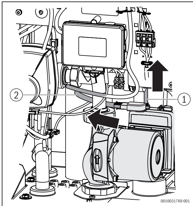
Afb. 37 Stekker aftrekken
