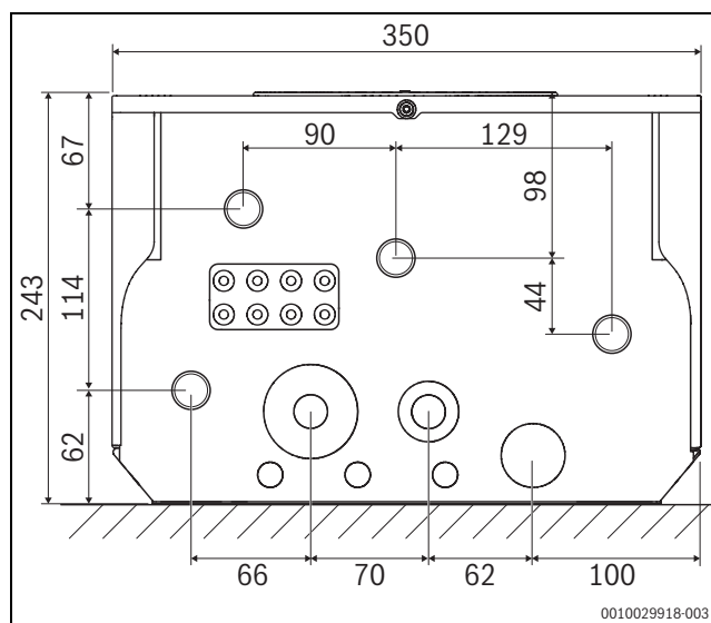
Afb. 5 Afstanden aansluitingen (mm)
