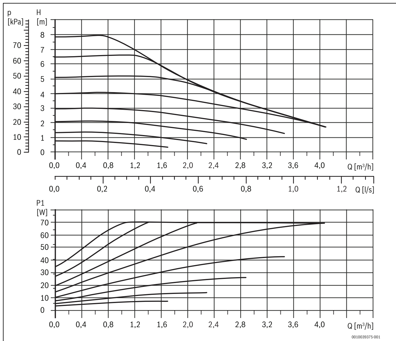
Afb. 20 Opvoercharacteristieken
