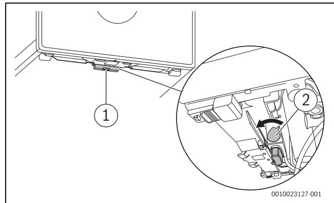
Afb. 4 Key borgen
