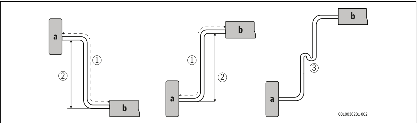
Afb. 10 Leidinglengthe en opvoerhoogte
