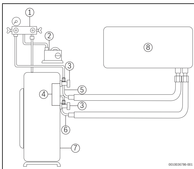
Afb. 18 Vacuüm, vullen en dichtheidstest
