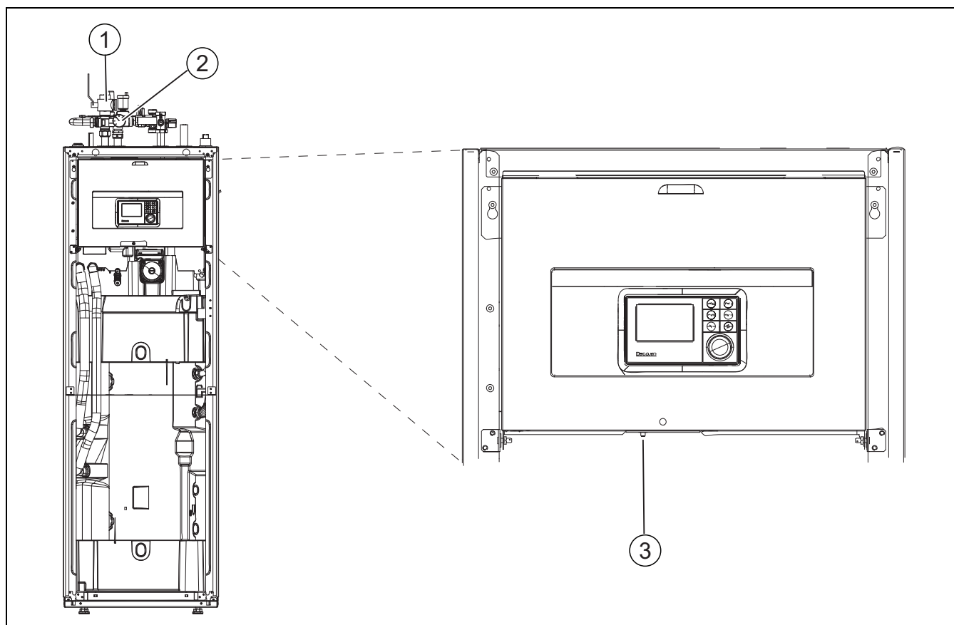
Afb. 6 Binnenunit IDU T/IDU TS
