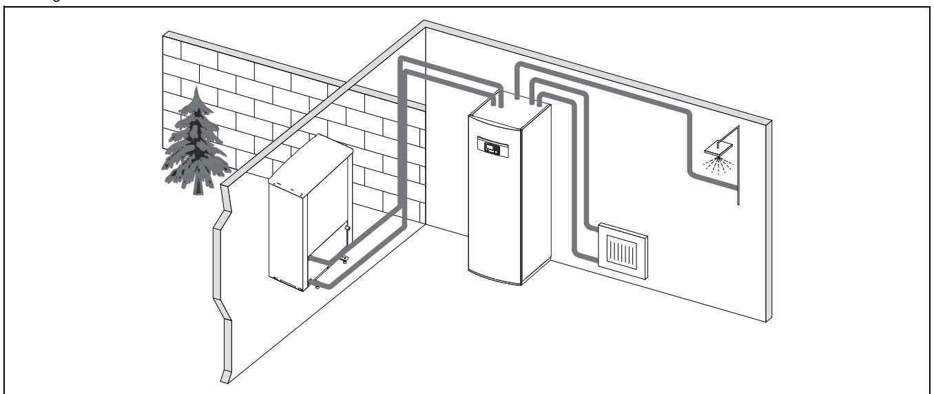
Afb. 3 Warmtepomp ODU Monoblock A/W, binnenunit IDU T/IDU TS-geïntegreerde boiler en elektrische bijverwarming
