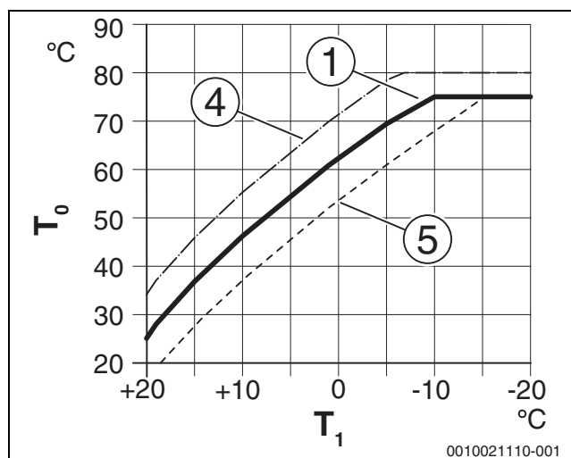
Afb. 5 Instelling van de stooklijn voor radiator Parallelschuiving via Offset ruimtetemperatuur of gewenste kamertemperatuur
