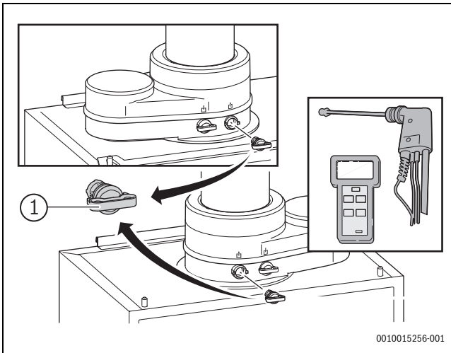
Afb. 53 Verwijderen afdekdop
