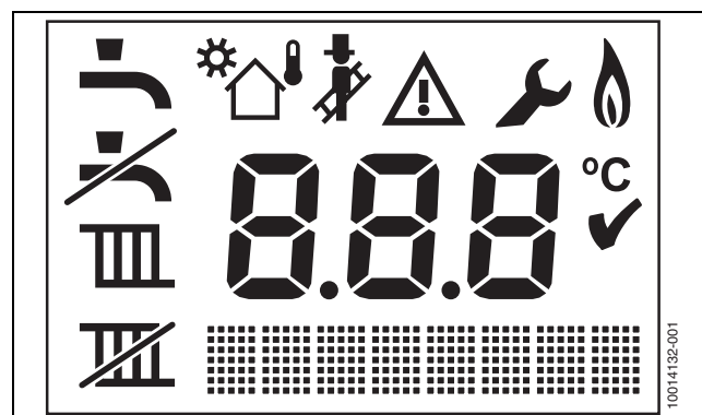
Afb. 36 Overzicht symbolen
