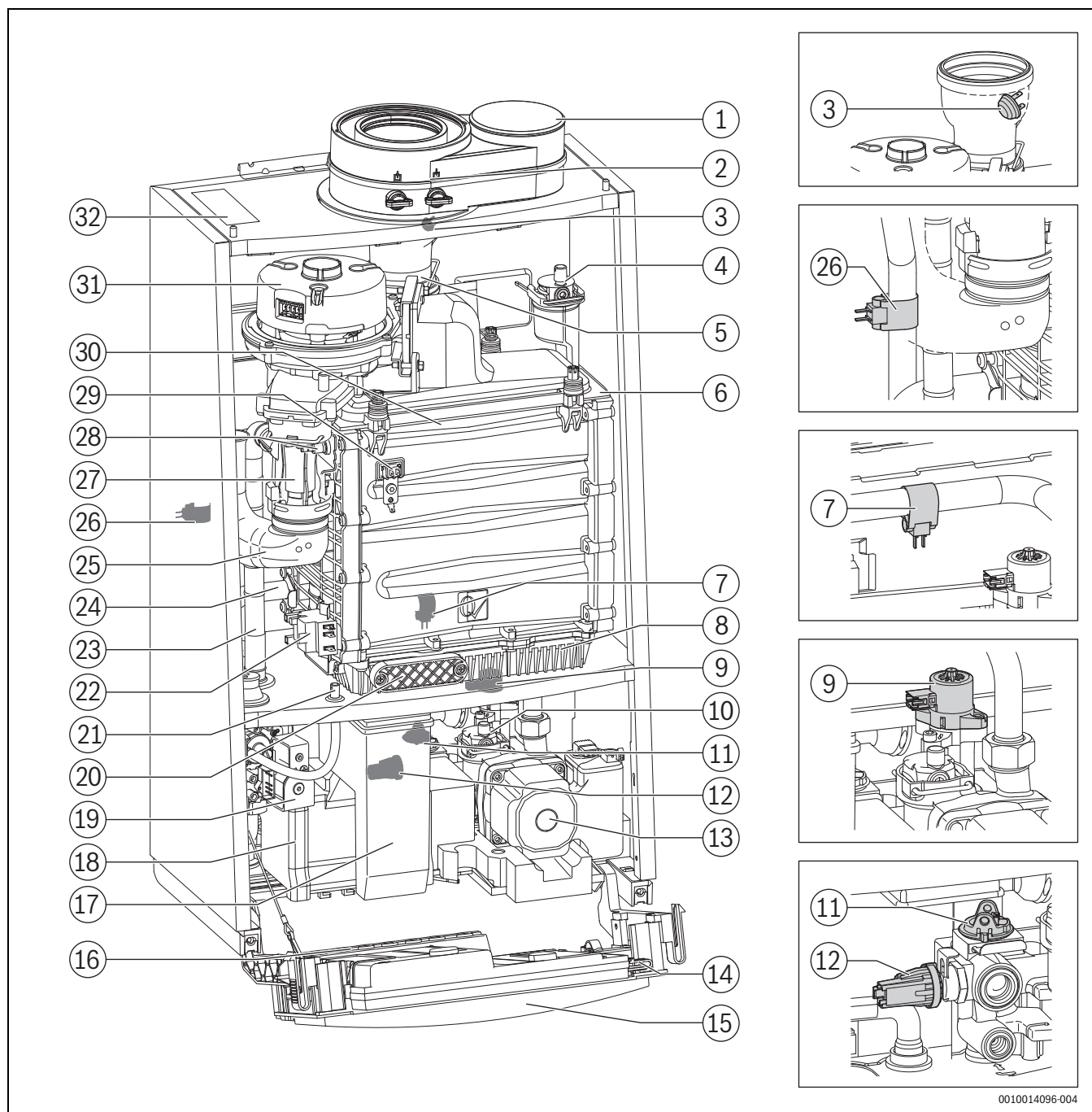
Afb. 1 Overzichtstekening
