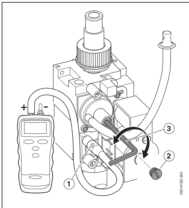
Afb. 56 Instellen gas-luchtverhouding
