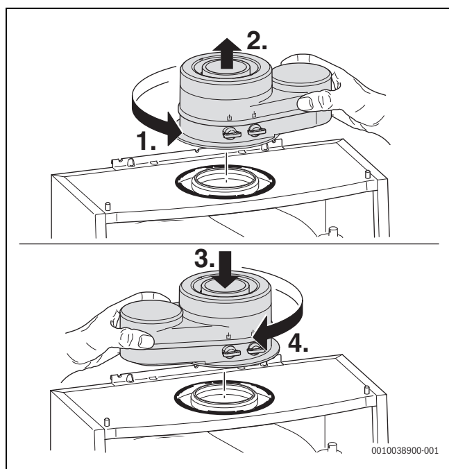
Afb. 6 Omdraaien rookgasafvoeradapter
