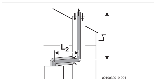
Afb. 13 Star rookgasafvoersysteem conform C93x in een schacht en concentrisch luchttoevoer- en rookgasafvoersysteem in opstellingsruimte
