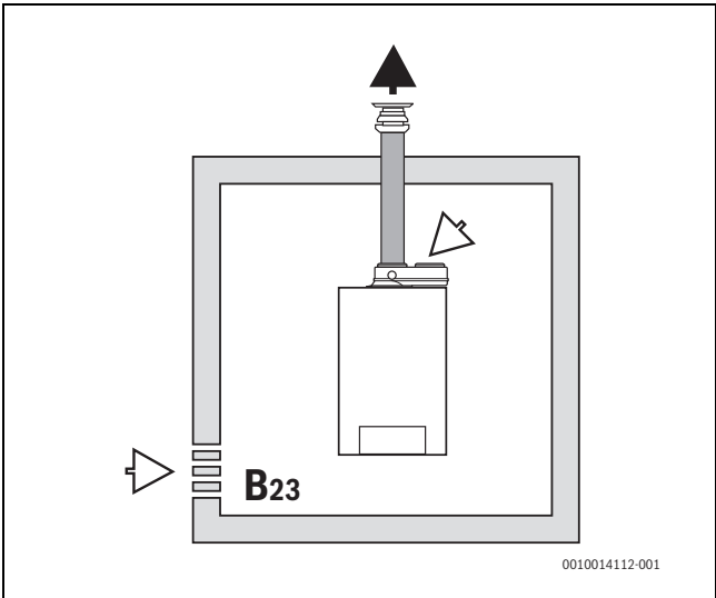
Afb. 8 Situatietekening rookgasafvoer type B 23
