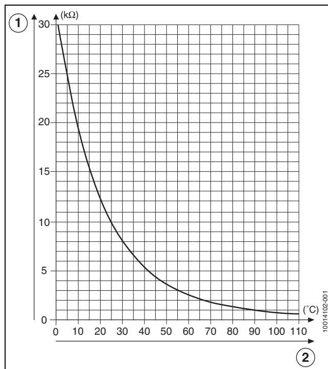
Afb. 62 Weerstandsgrafiek temperatuursensoren
