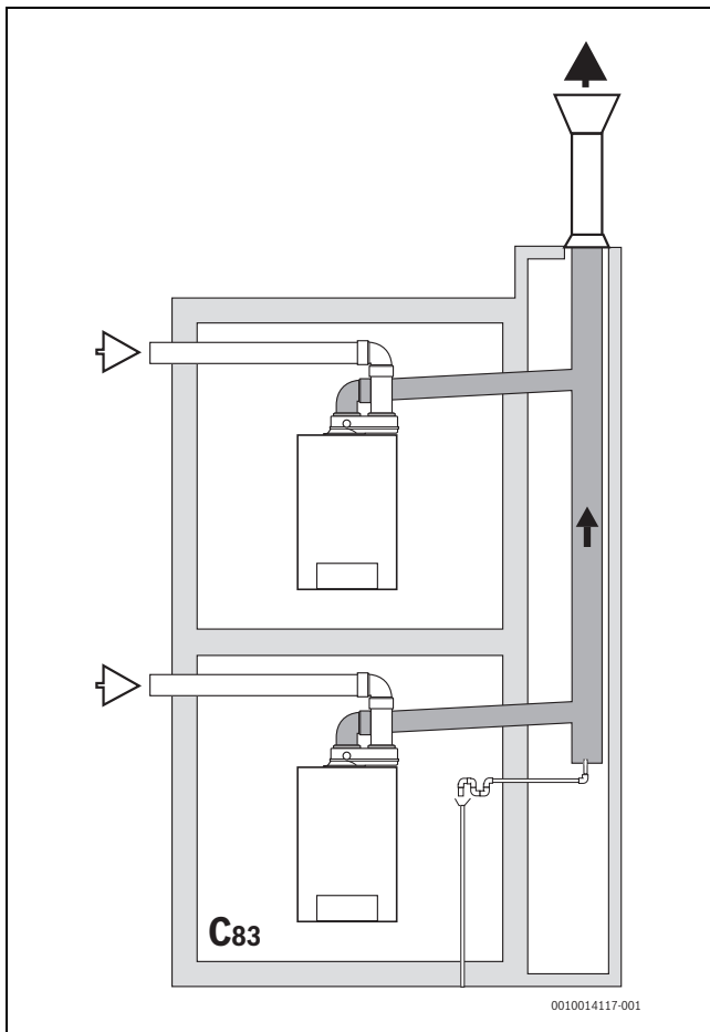
Afb. 16 Situatietekening rookgasafvoer type C 83
