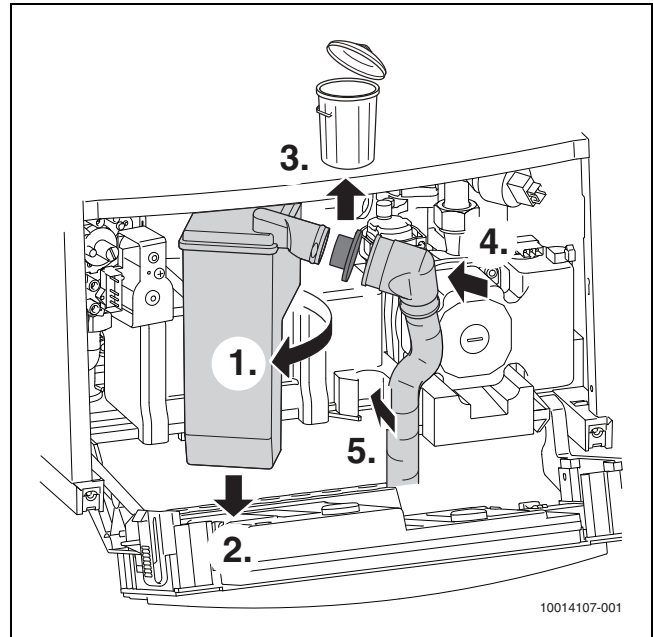
Afb. 21 Vullen toestelsifon
