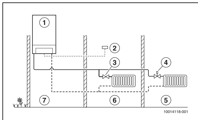
Afb. 23 Regelprincipe ruimteregeling
