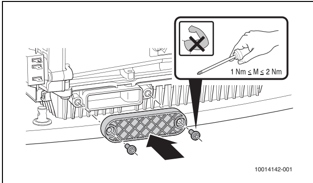
Afb. 43 Plaatsen servicedeksel
