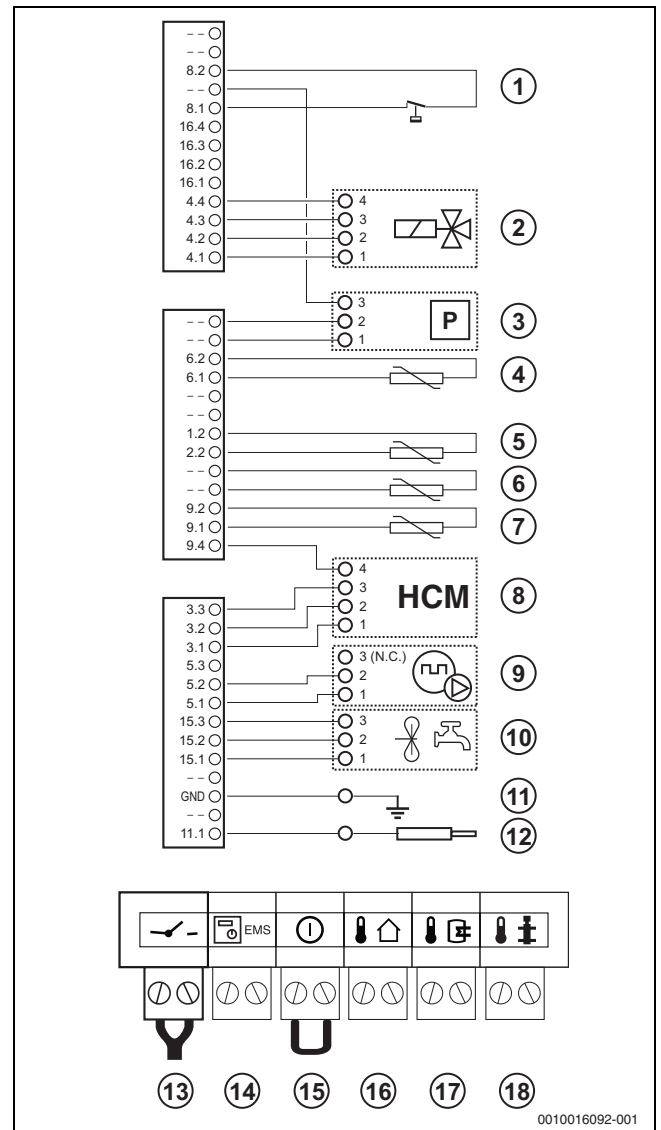
Afb. 60 Elektrisch schema 24 V-deel
