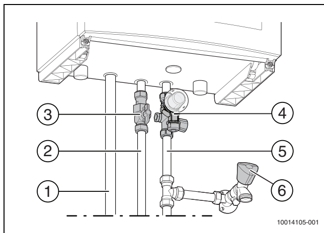
Afb. 19 Aansluiten gasleiding en waterleidingen
