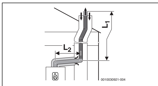
Afb. 14 Flexibel rookgasafvoersysteem conform C93x in een schacht en concentrisch luchttoevoer- en rookgasafvoersysteem in opstellingsruimte
