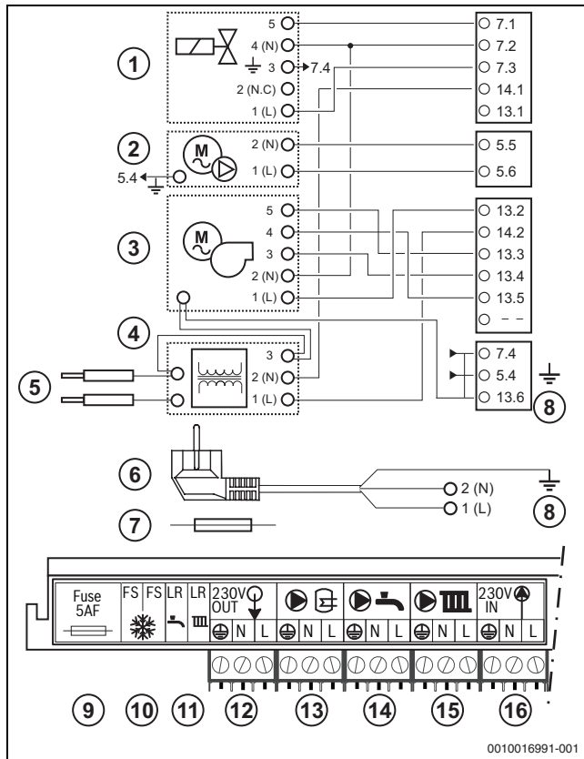
Afb. 59 Elektrisch schema 230 V-deel
