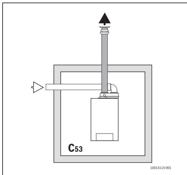
Afb. 12 Situatietekening rookgasafvoer type C 53
