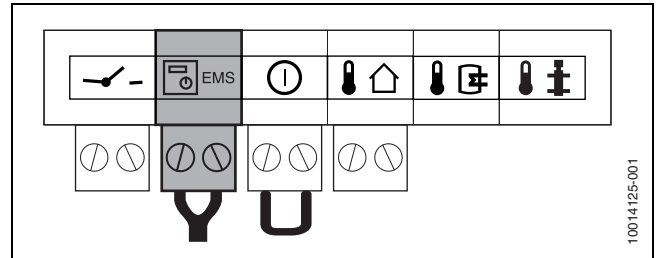
Afb. 30 Aansluiten modulerende kamerthermostaat (oranje)
