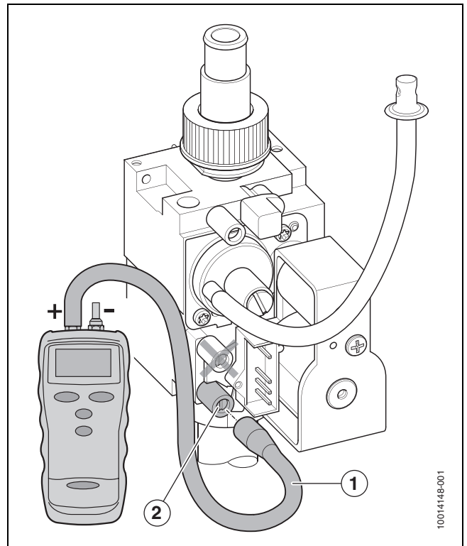
Afb. 52 Meten dynamische gasvoordruk
