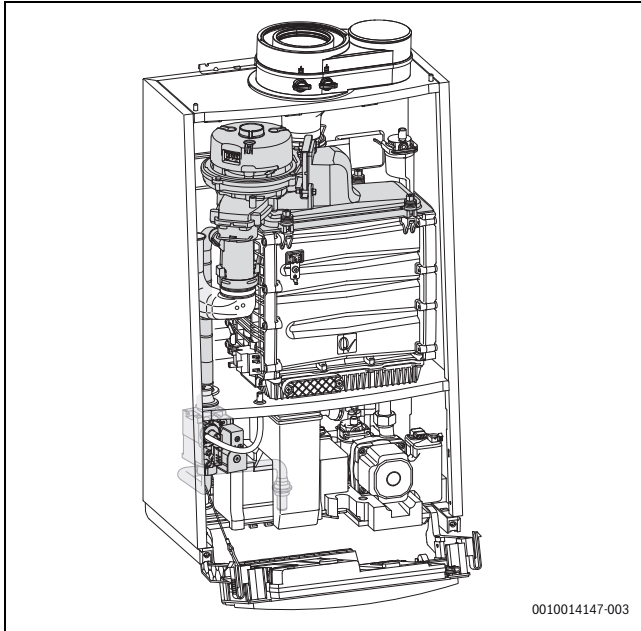
Afb. 50 Gasstraat
