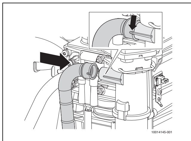
Afb. 49 Plaatsen gasslang
