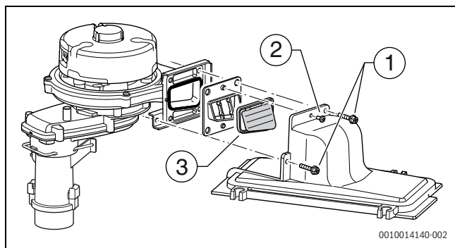
Afb. 46 Vervangen keerklep
