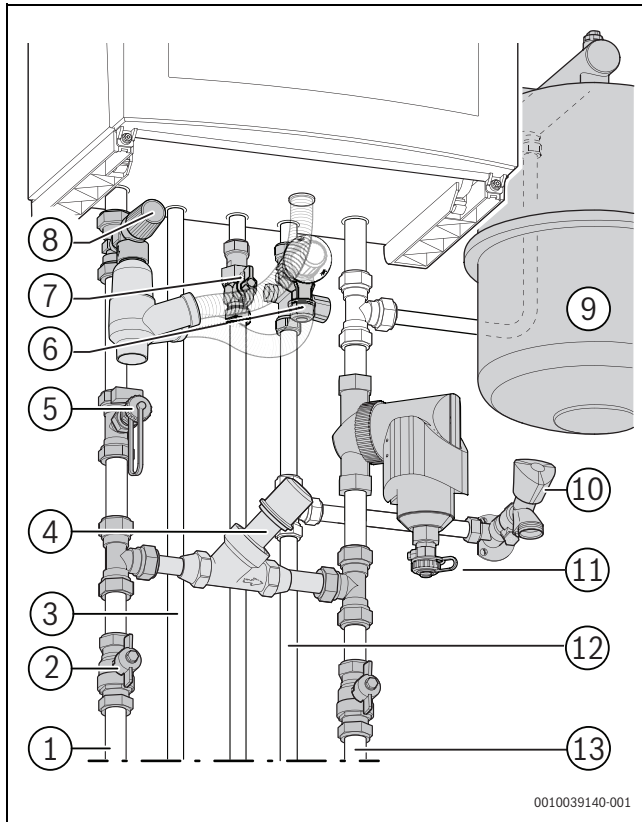
Afb. 20 Overzicht aansluitingen
