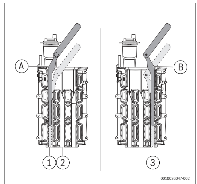
Afb. 42 Gebruik reinigingsmes
