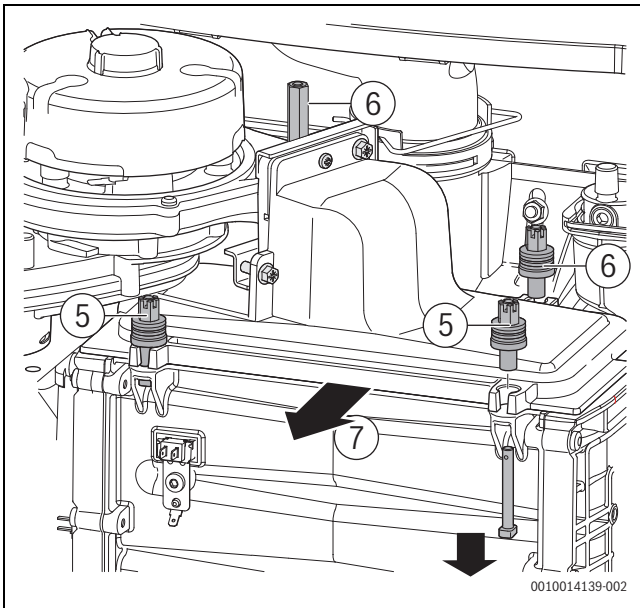
Afb. 40 Demonteren branderdekseel
