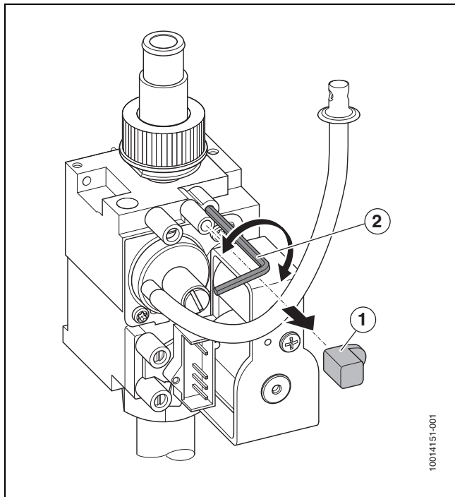
Afb. 55 Instellen zuurstofgehalte
