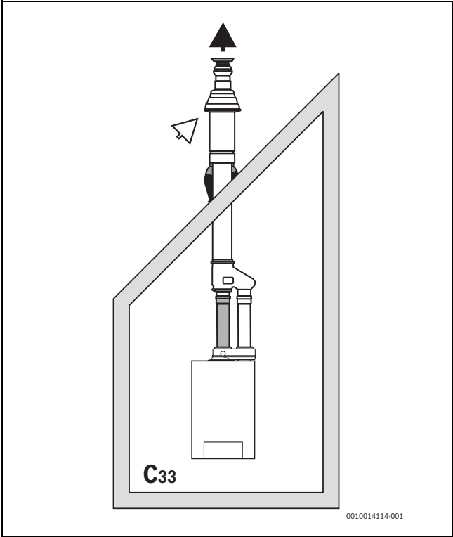
Afb. 11 Situatietekening rookgasafvoer type C 33
