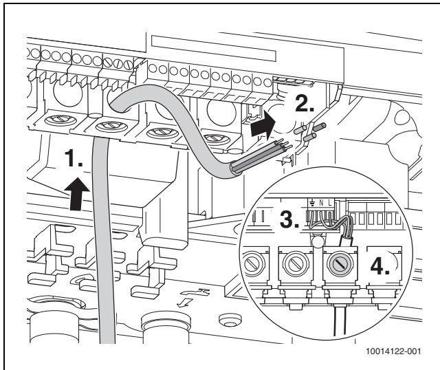
Afb. 27 Trekontlasting
