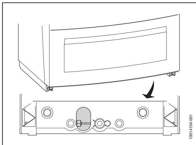
Afb. 18 Serviceopening warmwatertemperatuursensor
