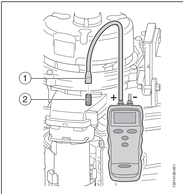
Afb. 51 Drukmeting
