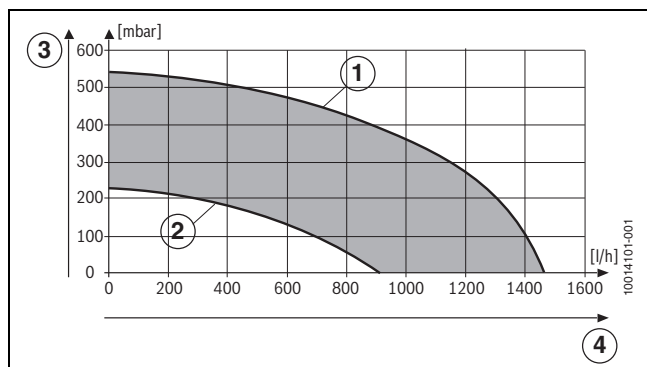
Afb. 61 Restopvoerhoogte cv-water
