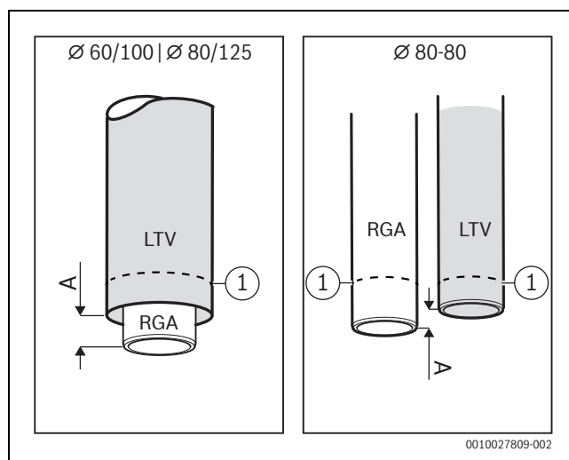
Afb. 7 Lengteverschil luchttoevoer-, rookgasafvoerbuizen [A]
