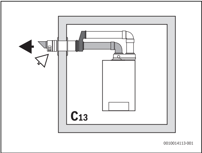
Afb. 10 Situatietekening rookgasafvoer type C 13
