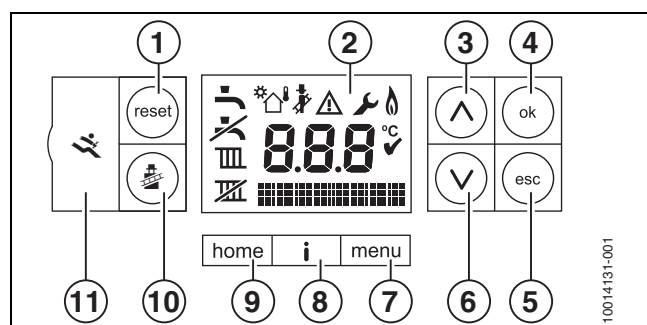
Afb. 35 Bedieningspaneel
