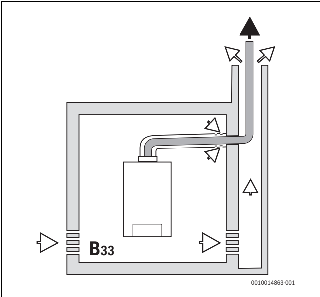
Afb. 9 Situatietekening rookgasafvoer type B 33
