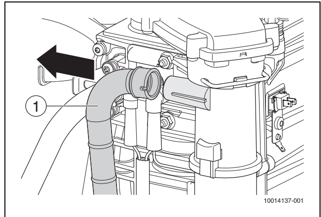
Afb. 38 Verwijderen gasslang
