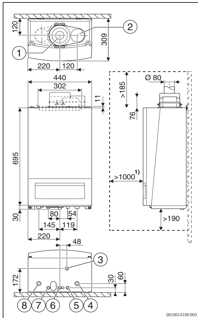
Afb. 4 Afmetingen [mm] 1)
