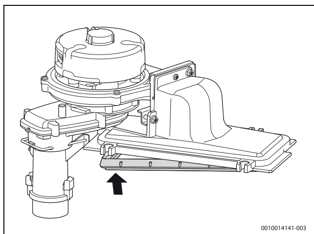
Afb. 47 Plaatsen branderpakking
