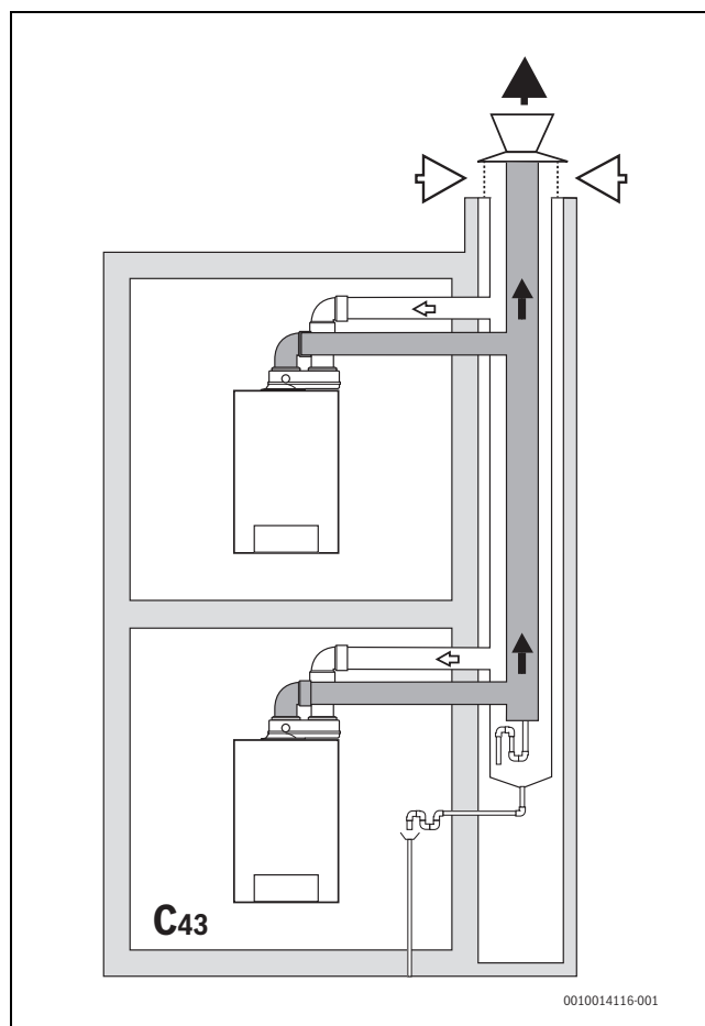
Afb. 15 Situatietekening rookgasafvoer type C 43
