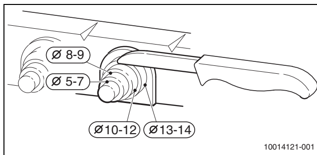
Afb. 26 Diameters kabeldoorvoeren
