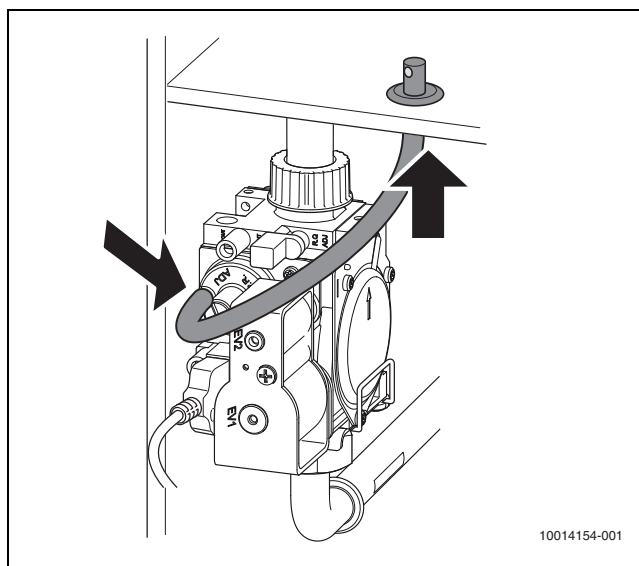
Afb. 58 Positie drukvereffeningsslang
