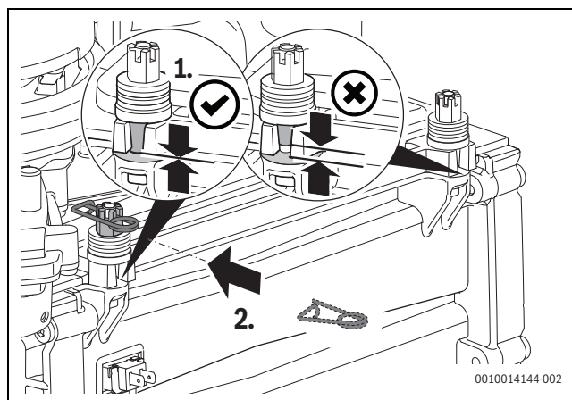
Afb. 48 Aandraaien moeren
