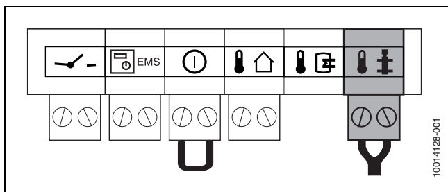
Afb. 33 Aansluiten Nefit Solarsensor (bruin)
