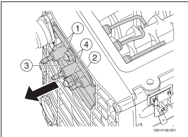
Afb. 41 Verwijderen ontstekingsunit
