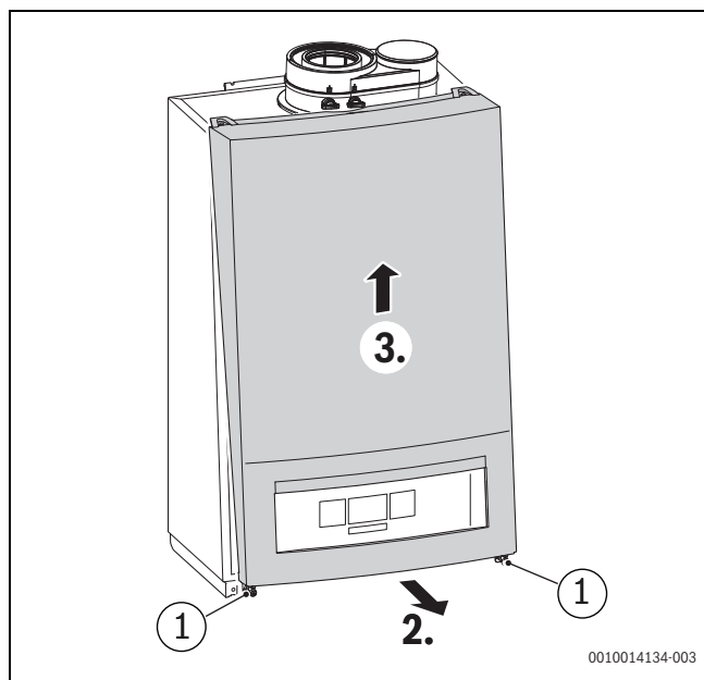
Afb. 3 Openen voorpaneel
