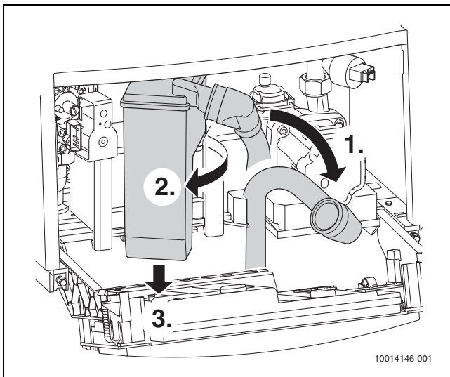
Afb. 44 Verwijderen toestelsifon
