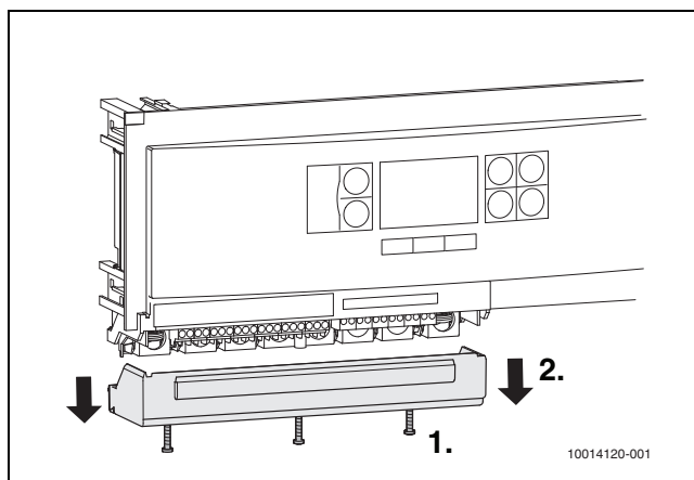
Afb. 25 Verwijderen beschermkap
