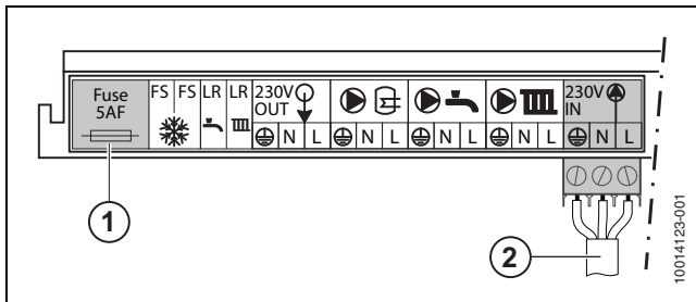
Afb. 28 Netspanningsaansluitingen
