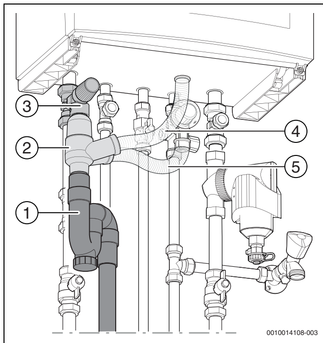
Afb. 22 Aansluiten condensafvoer
