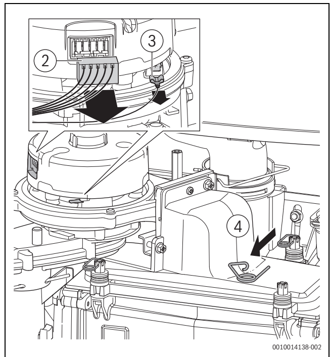
Afb. 39 Demonteren branderdekseel
