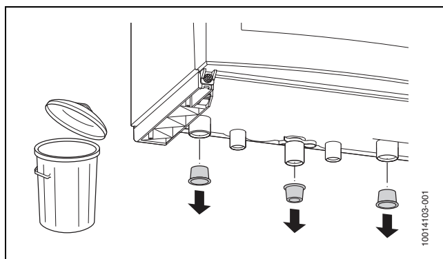
Afb. 17 Verwijderen beschermdoppen
