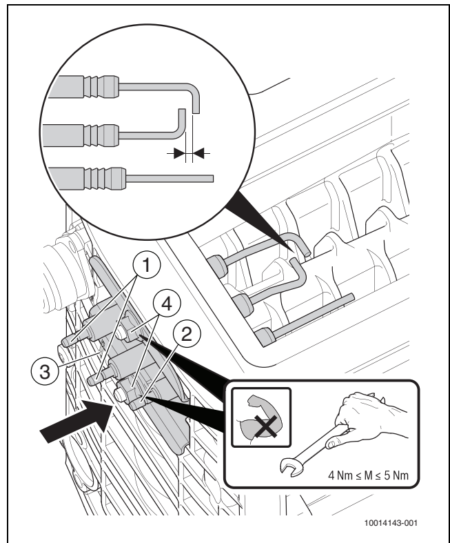
Afb. 45 Controleren en inbouwen ontstekingsunit
