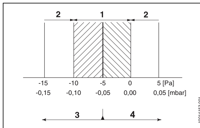
Afb. 57 Instellen drukverschil (op laaglast)
