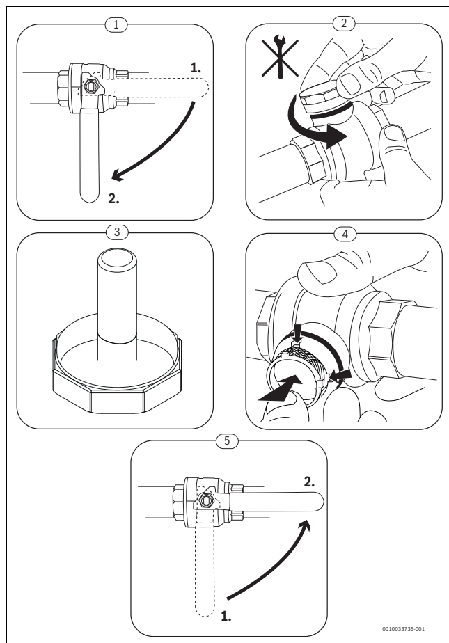
Afb. 6 Filterreiniging
