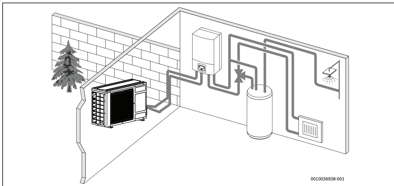
Afb. 2 Warmtepomp buitenunit, AWS E binnenunit met elektrische bijverwarming en externe boiler
