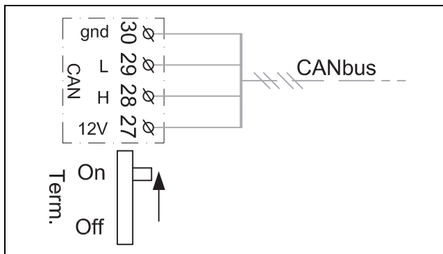
Afb. 16 CAN-BUS-afsluiting
