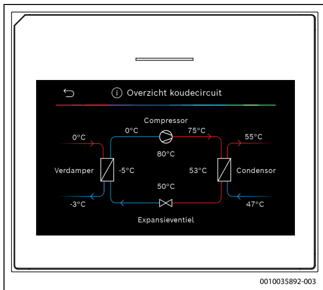
Afb. 11 Overzicht koelcircuit
