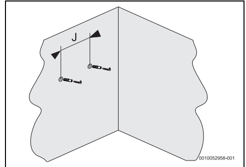
Bild 9 Befestigungsschrauben
