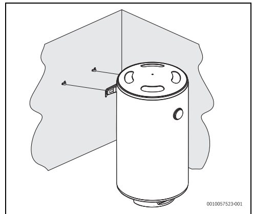
Bild 10 Senkrechte Installation (Wandmontage)
