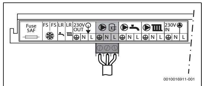
Afb. 27 Tapwaterpompaansluiting
