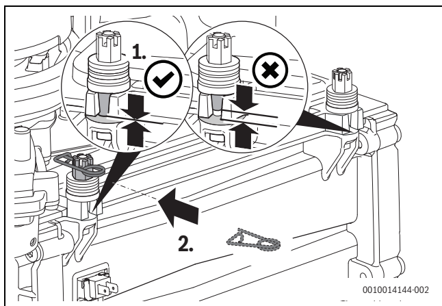
Afb. 52 Aandraaien moeren
