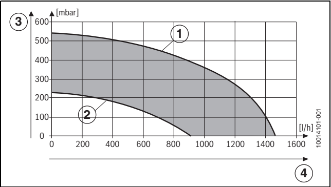
Afb. 65 Restopvoerhoogte cv-water
