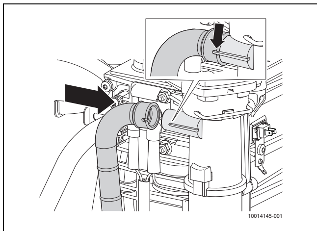
Afb. 53 Plaatsen gasslang
