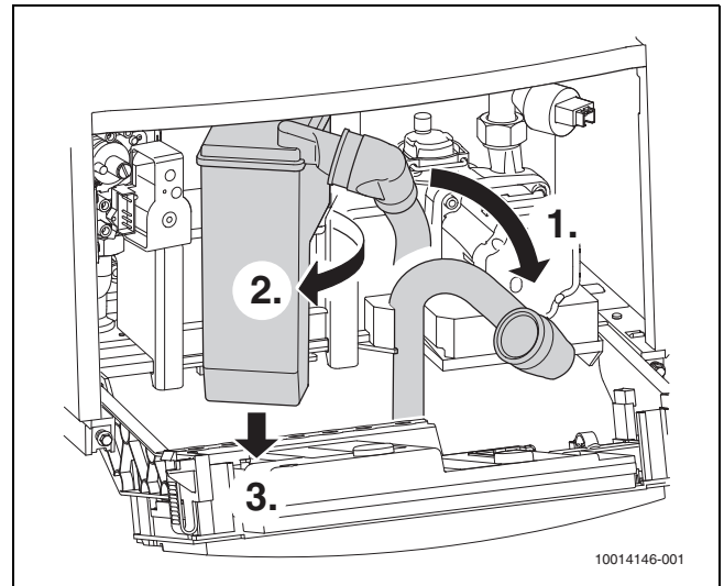
Afb. 48 Verwijderen toestelsifon
