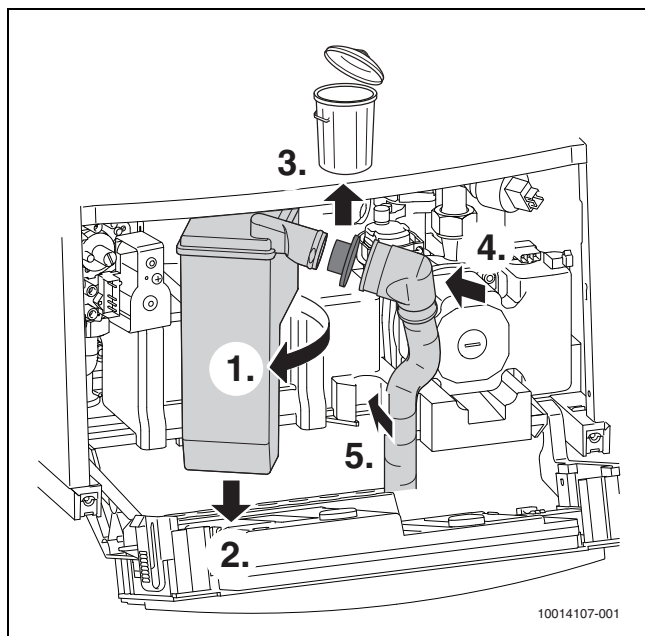
Afb. 19 Vullen toestelsifon
