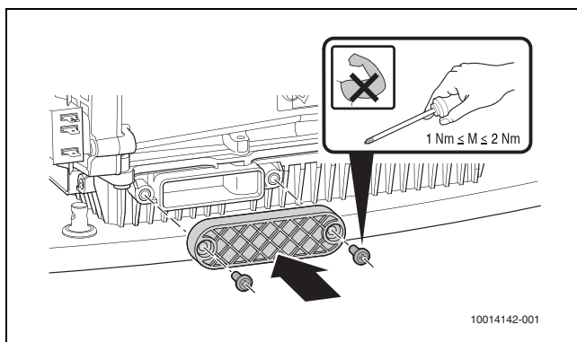
Afb. 47 Plaatsen servicedeksel
