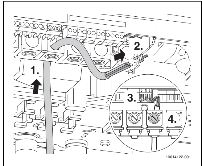
Afb. 26 Trekontlasting
