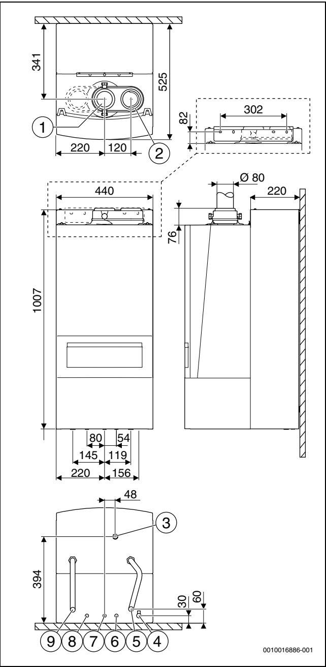
Afb. 4 Afmetingen [mm]
