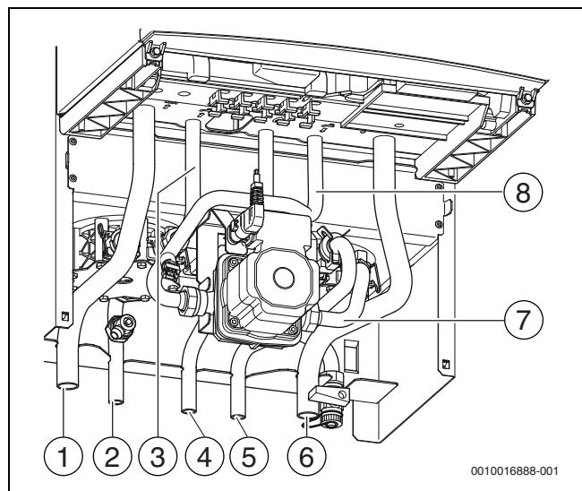
Afb. 15 Verbindingsstukken
