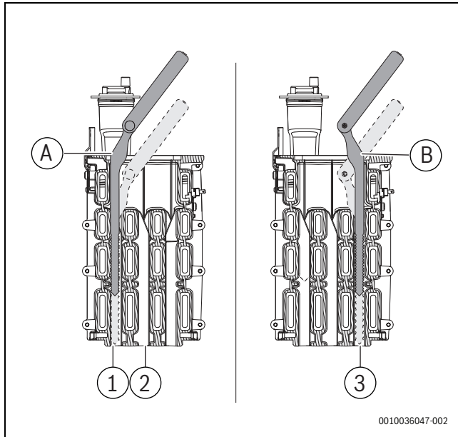
Afb. 46 Gebruik reinigingsmes
