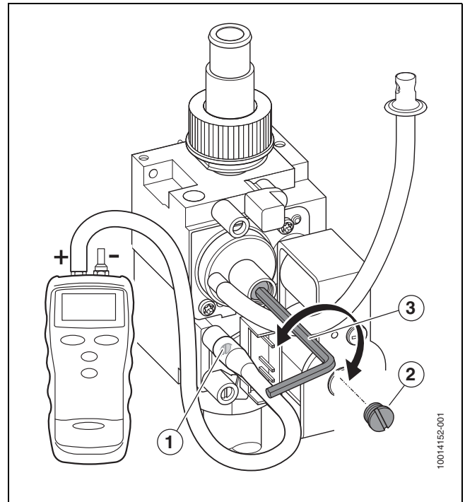
Afb. 60 Instellen gas-luchtverhouding
