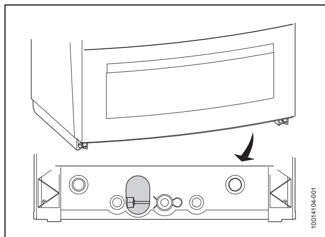
Afb. 14 Serviceopening warmwatertemperatuursensor
