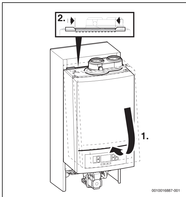
Afb. 12 Ophangen cv-toestel
