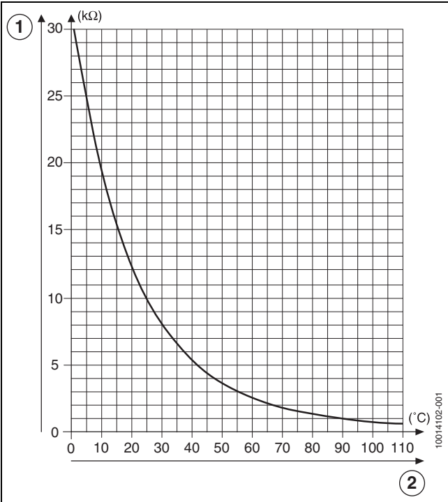
Afb. 66 Weerstandsgrafiek temperatuursensoren
