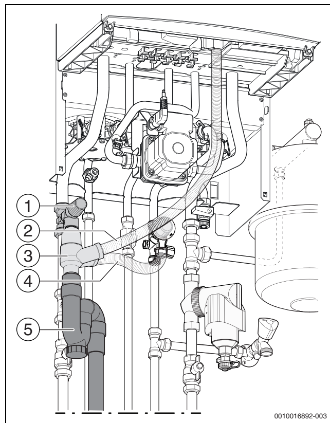
Afb. 20 Aansluiten condensafvoer
