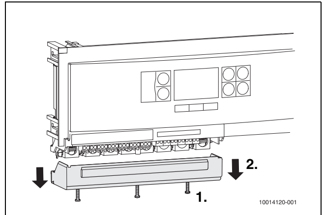
Afb. 20 Verwijderen beschermkap
