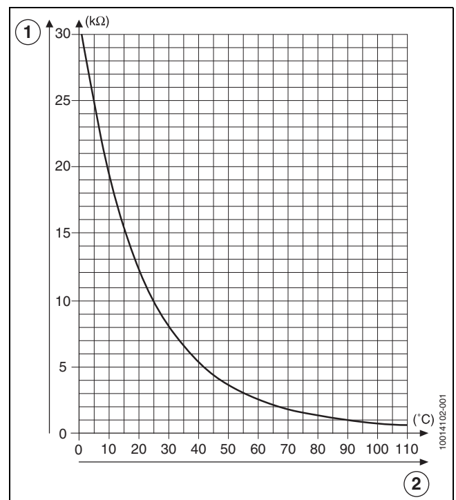
Afb. 58 Weerstandsgrafiek temperatuursensoren
