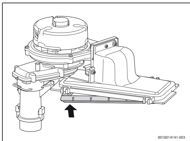
Afb. 43 Plaatsen branderpakking
