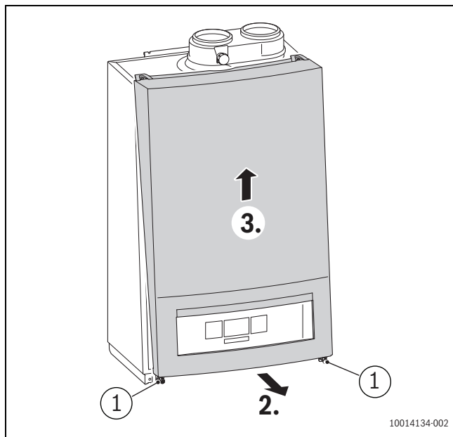
Afb. 33 Openen voorpaneel
