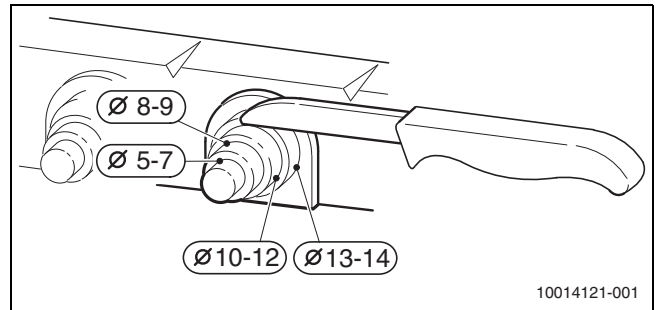
Afb. 21 Diameters kabeldoorvoeren
