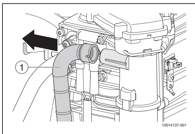
Afb. 34 Verwijderen gaslang
