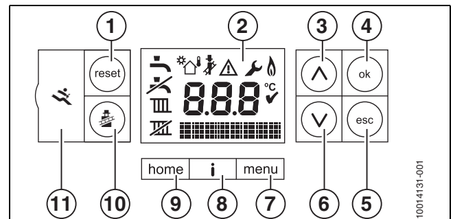
Afb. 30 Bedieningspaneel
