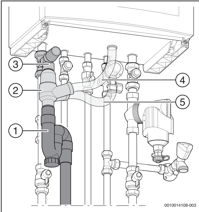
Afb. 16 Aansluiten condensafvoer
