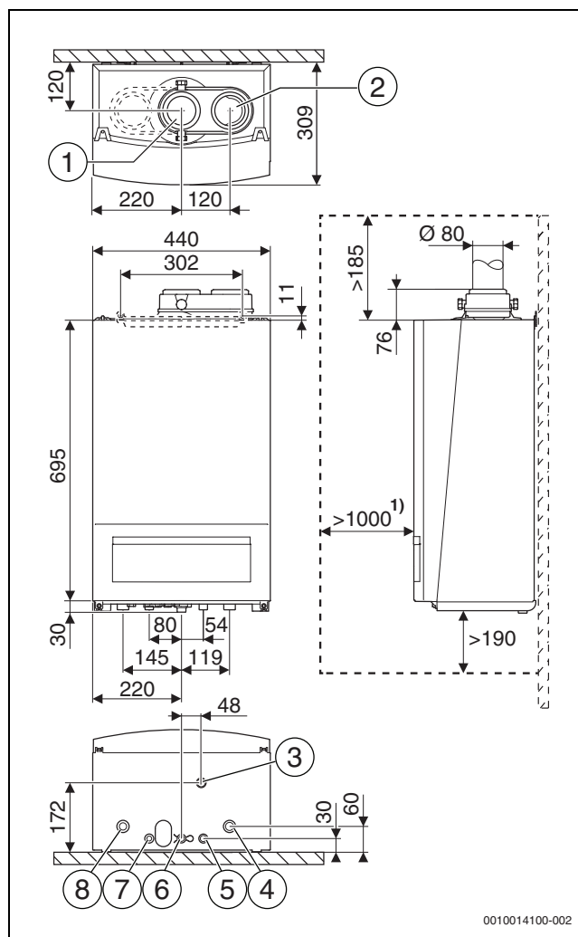
Afb. 3 Afmetingen [mm] 1)
