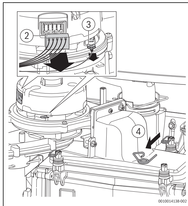
Afb. 35 Demoneren branderdeksel
