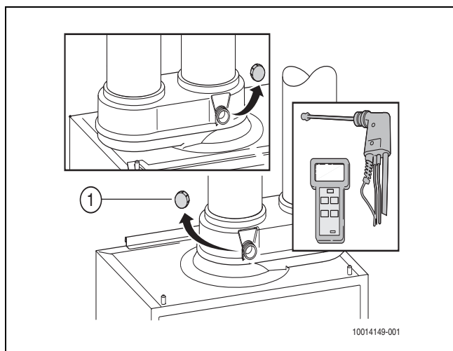
Afb. 49 Verwijderen afdekdop
