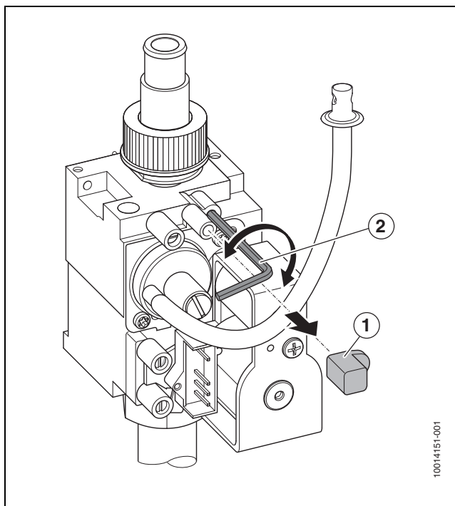
Afb. 51 Instellen zuurstofgehalte
