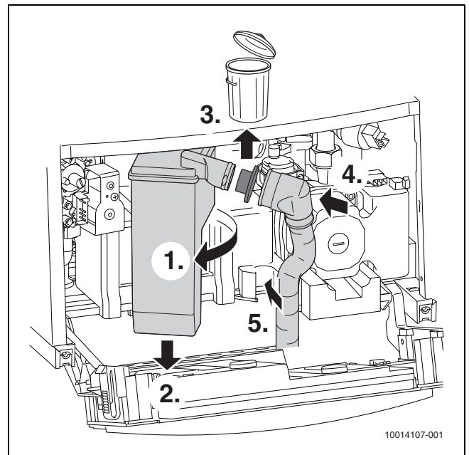
Afb. 15 Vullen toestelsifon
