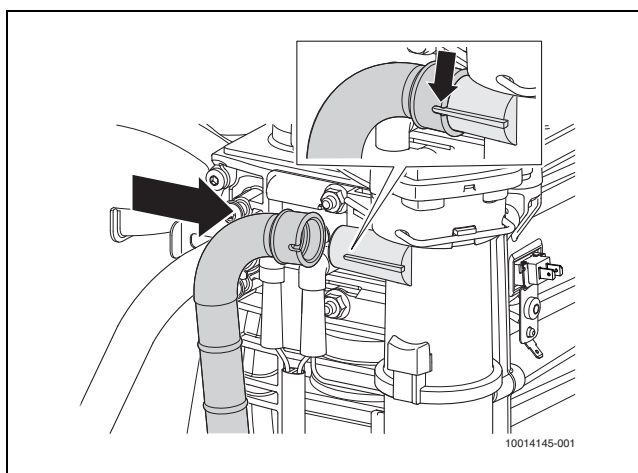
Afb. 45 Plaatsen gasslang
