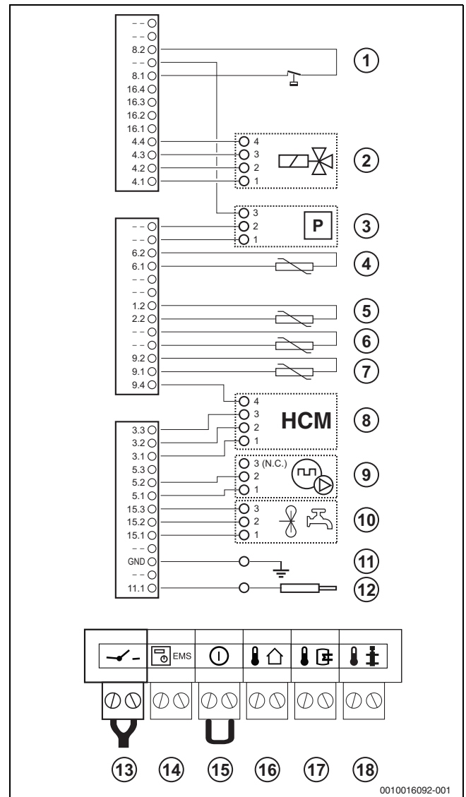
Afb. 56 Elektrisch schema 24 V-deel
