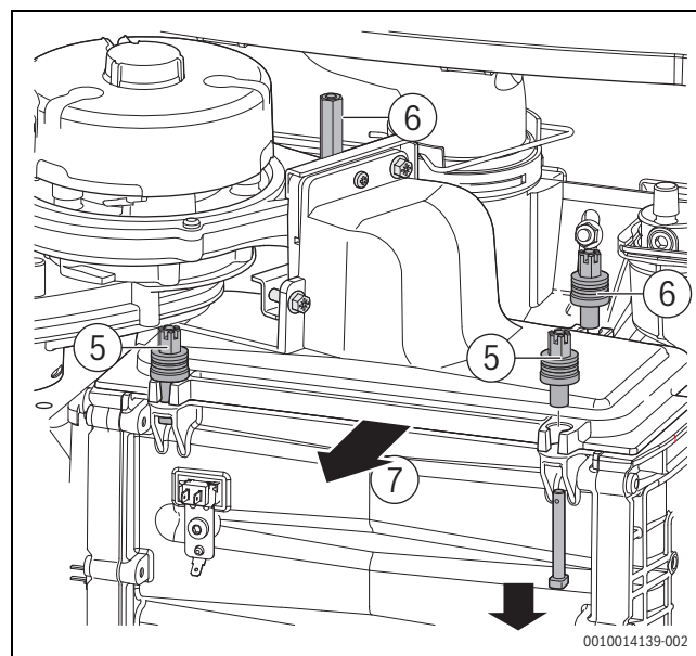
Afb. 36 Demoneren branderdeksel
