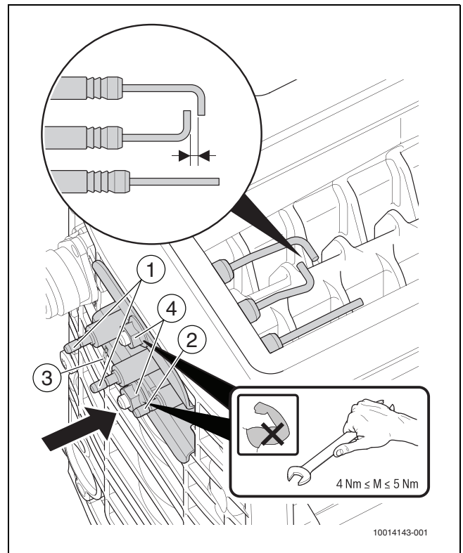
Afb. 41 Controleren en inbouwen ontstekingsunit
