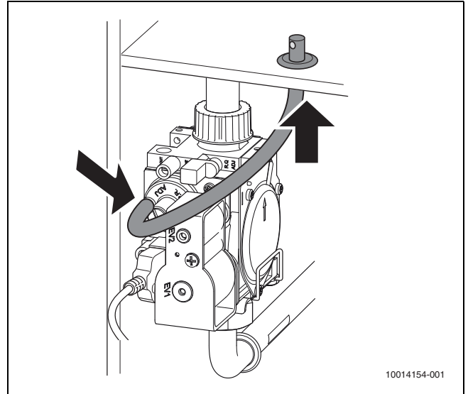
Afb. 54 Positie drukvereffeningsslang
