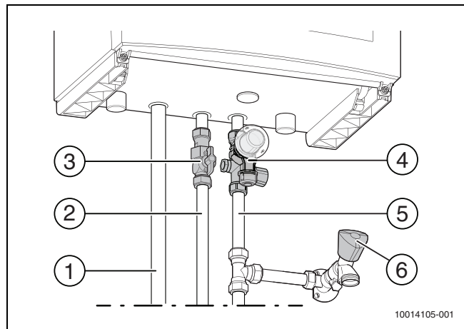
Afb. 13 Aansluiten gasleiding en waterleidingen
