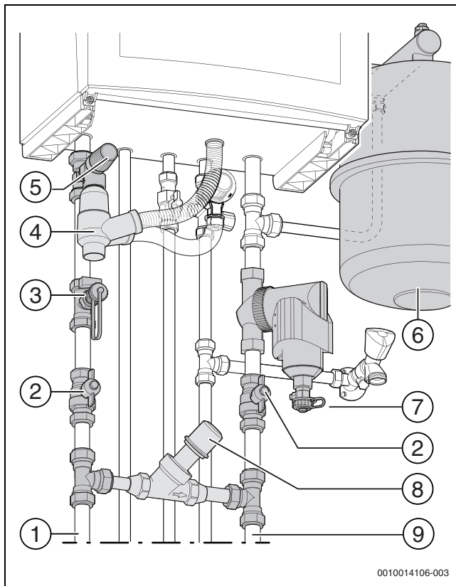
Afb. 14 Aansluiten cv-leidingen
