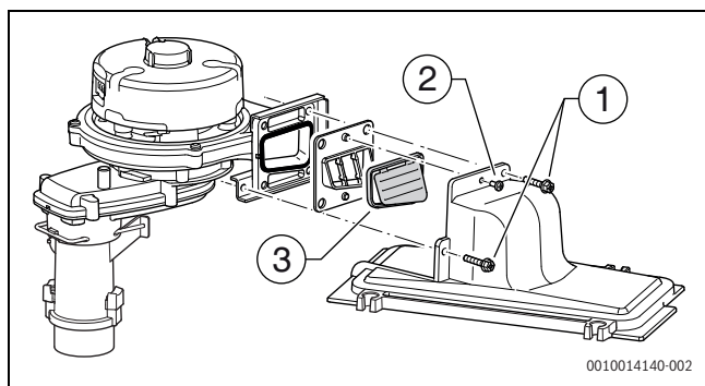
Afb. 42 Vervangen keerklep
