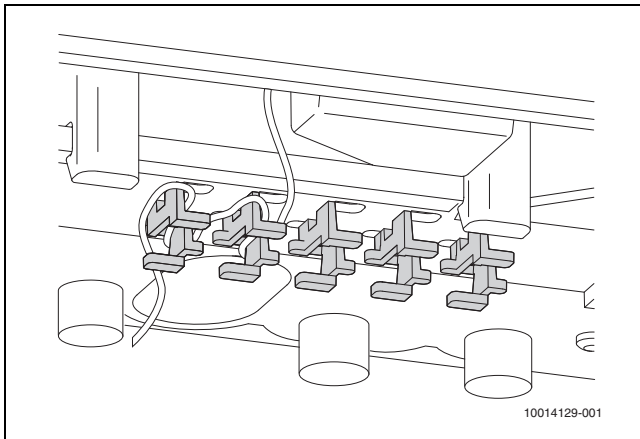
Afb. 29 Kabelbinder
