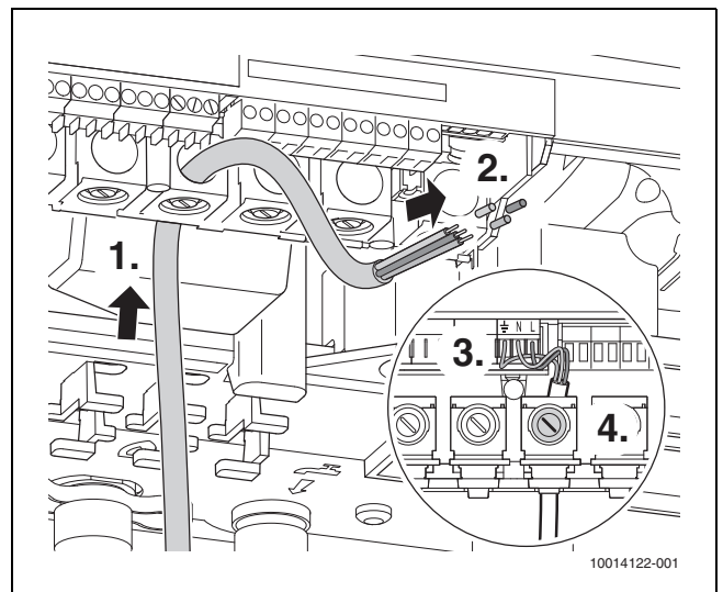
Afb. 22 Trekontlasting
