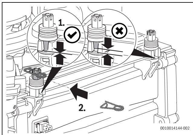
Afb. 44 Aandraaien moeren
