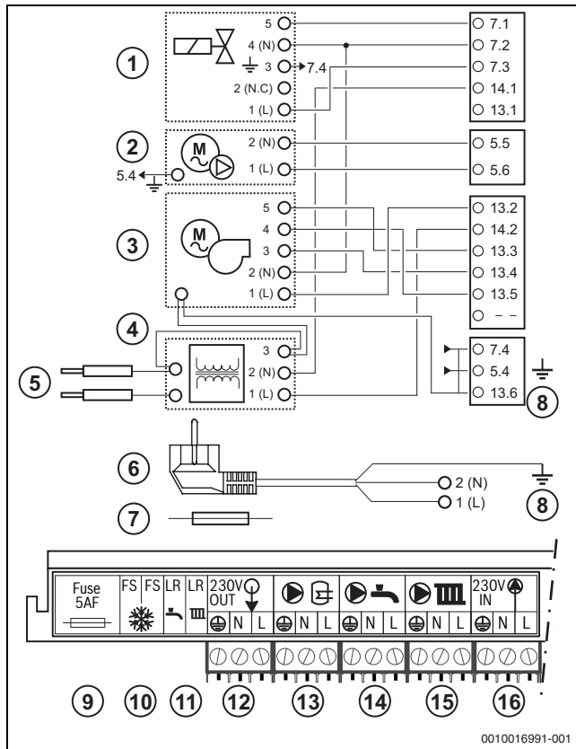
Afb. 55 Elektrisch schema 230 V-deel
