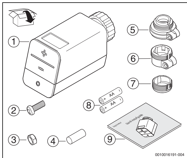
Afb. 2 Leveringsomvang
