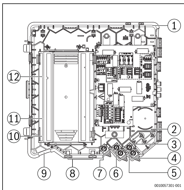
Rys. 154 Prowadzenie przewodów w skrzynce zaciskowej (główne zasilanie, osprzęt dodatkowy i niskie napięcie)
