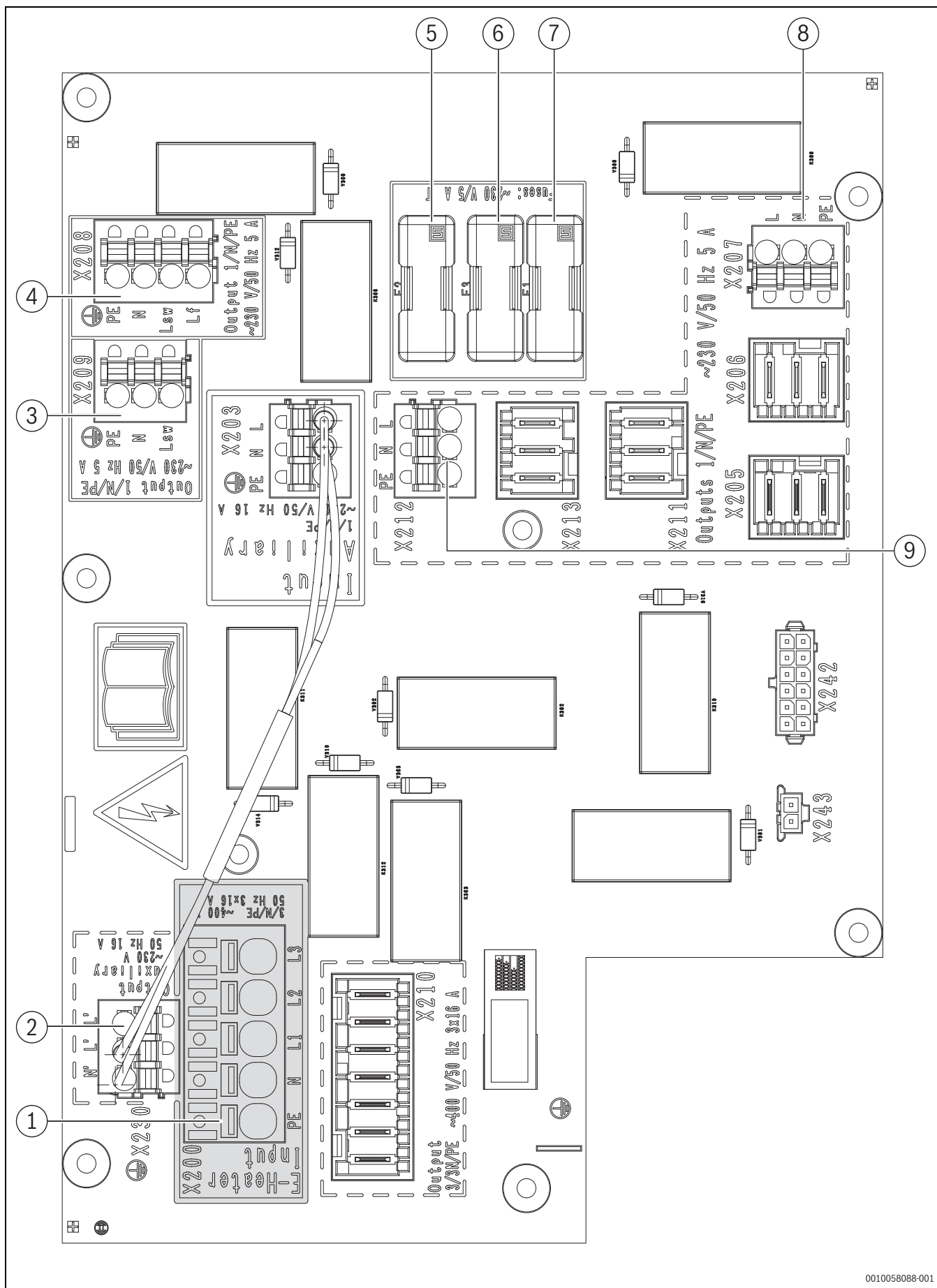
Rys. 145 Przyłącza na XCU-SEH
