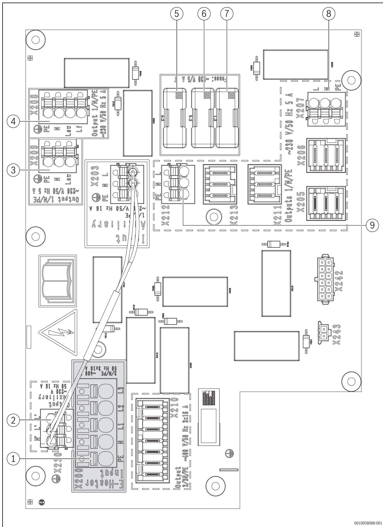
Fig. 88 Collegamenti su XCU-SEH
