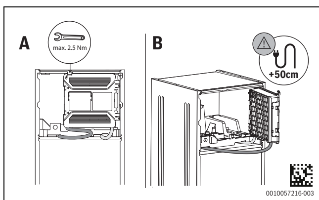
Afb. 43 Kabeldoorvoeren naar de binneneenheid
