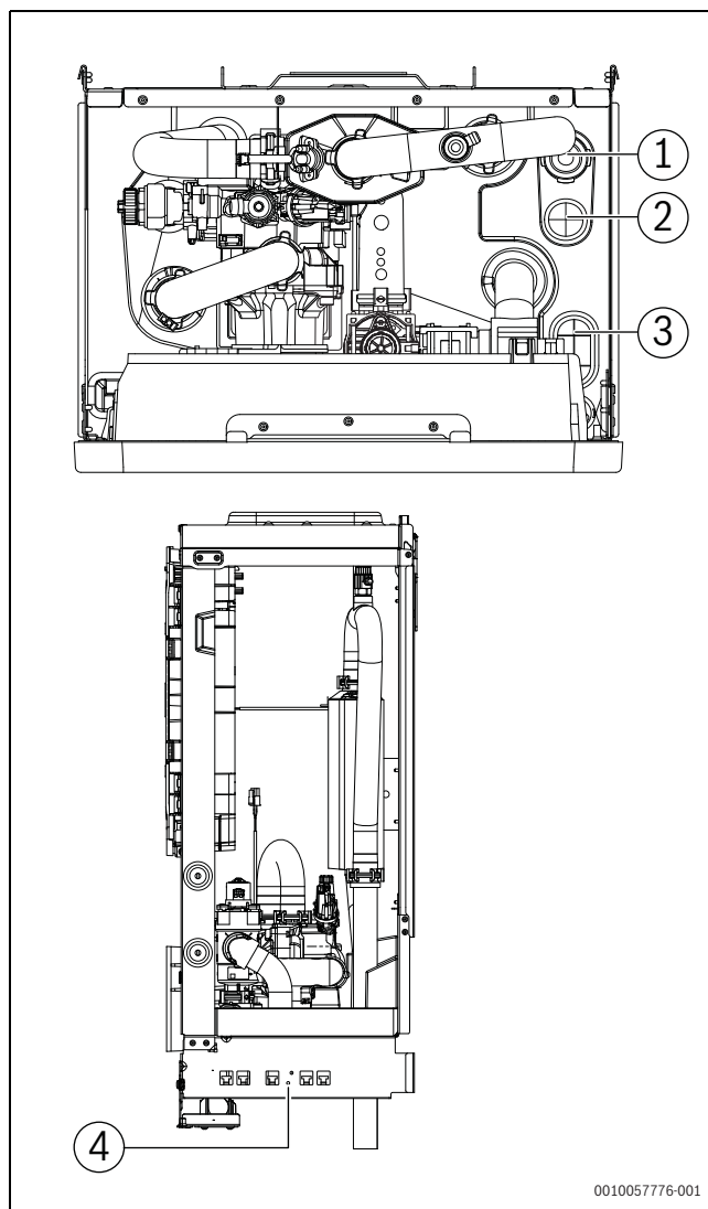
Fig. 97 Pressacavi e gommini per l'unità interna (alimentazione principale, accessori e bassa tensione)
