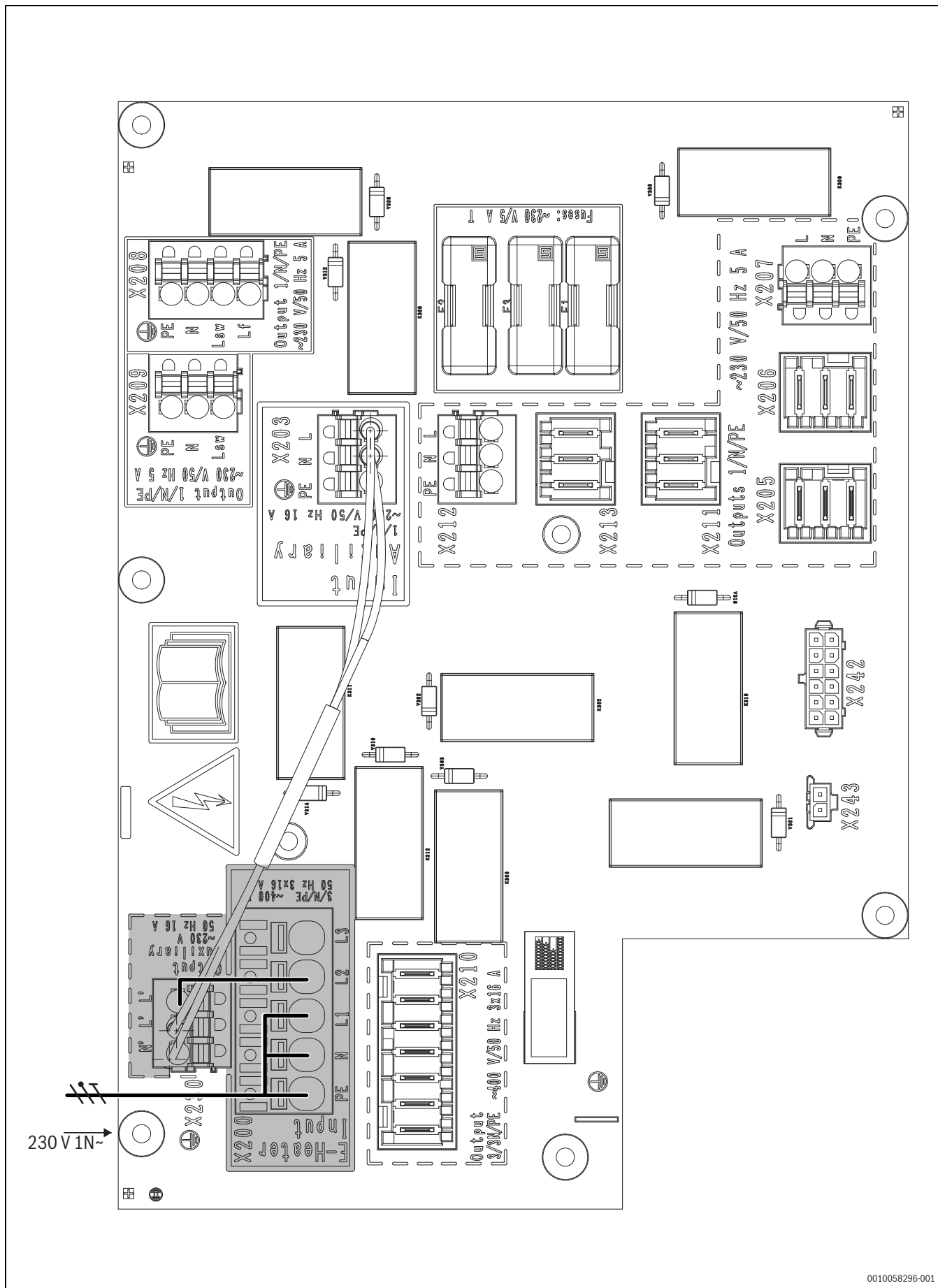
Fig. 62 Raccordement 230 V pour le chauffage d'appoint électrique avec pontage 230 V pour la commande et les pompes
