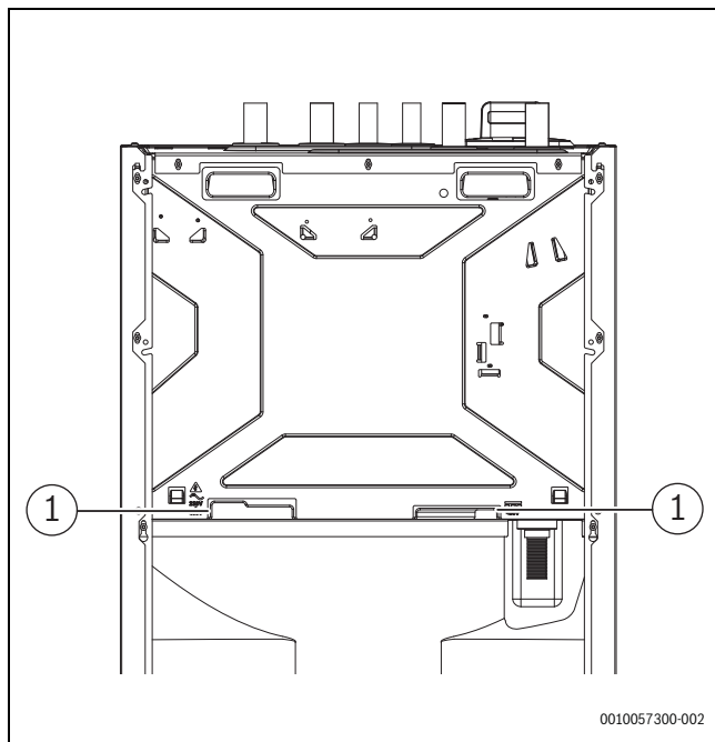
Afb. 128 Kabeldoorvoeren naar de binnenunit
