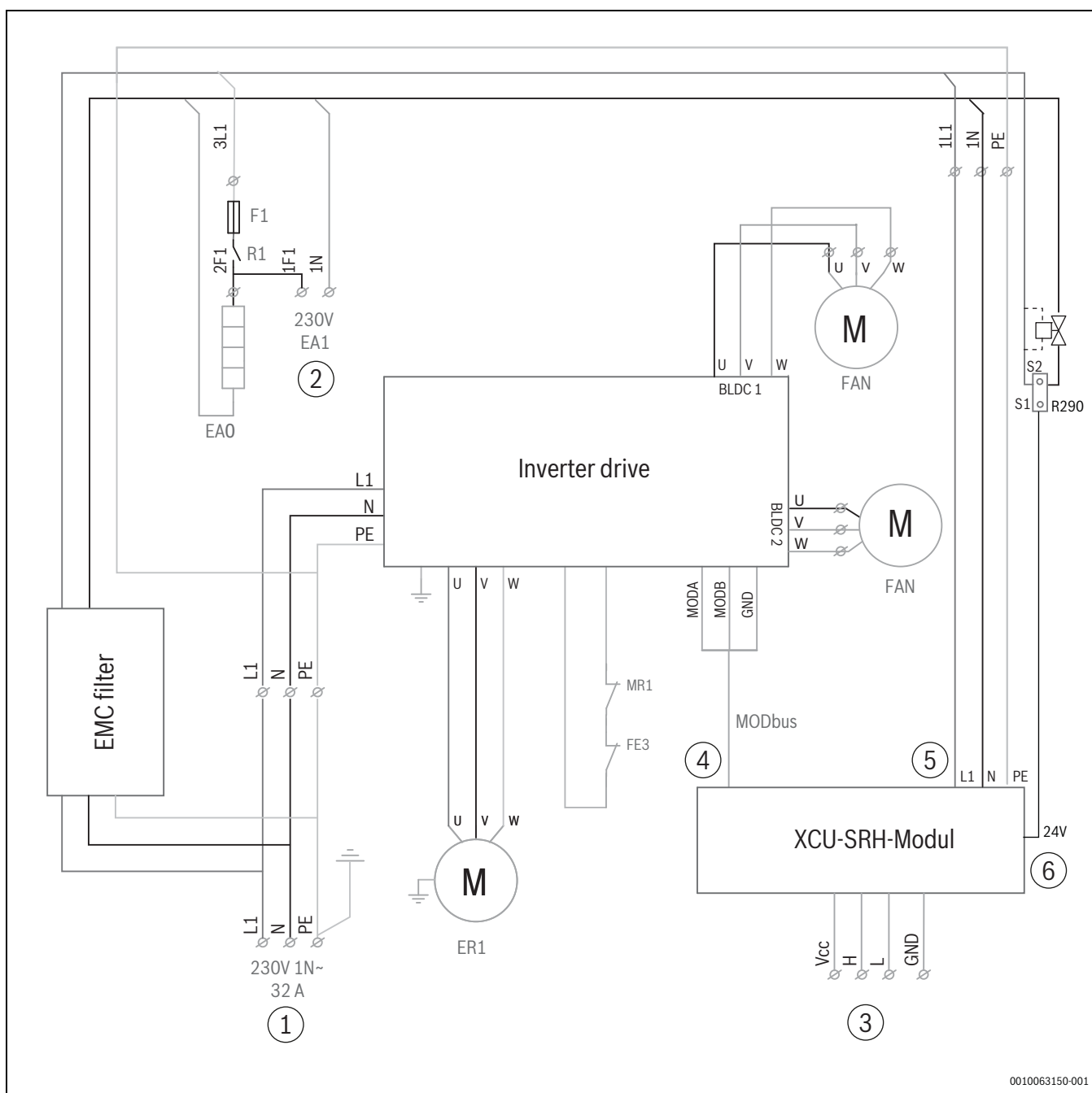
Afb. 140 Aansluitschema 1 fase (houdt rekening met pre-installatie van de druppelvangerverwarming)
