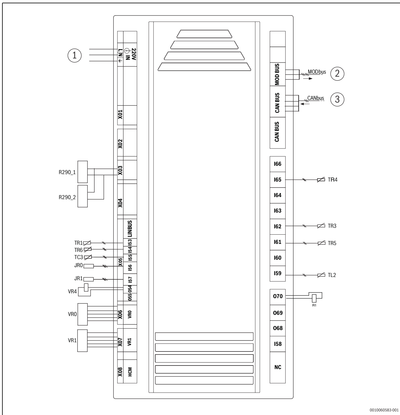
Fig. 115 Schema elettrico XCU-SRH (XCU-HP)
