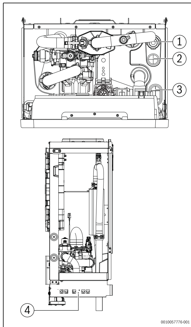
Fig. 68 Presse-étoupe et gaines vers l'unité intérieure (alimentation principale, accessoires et basse tension)
