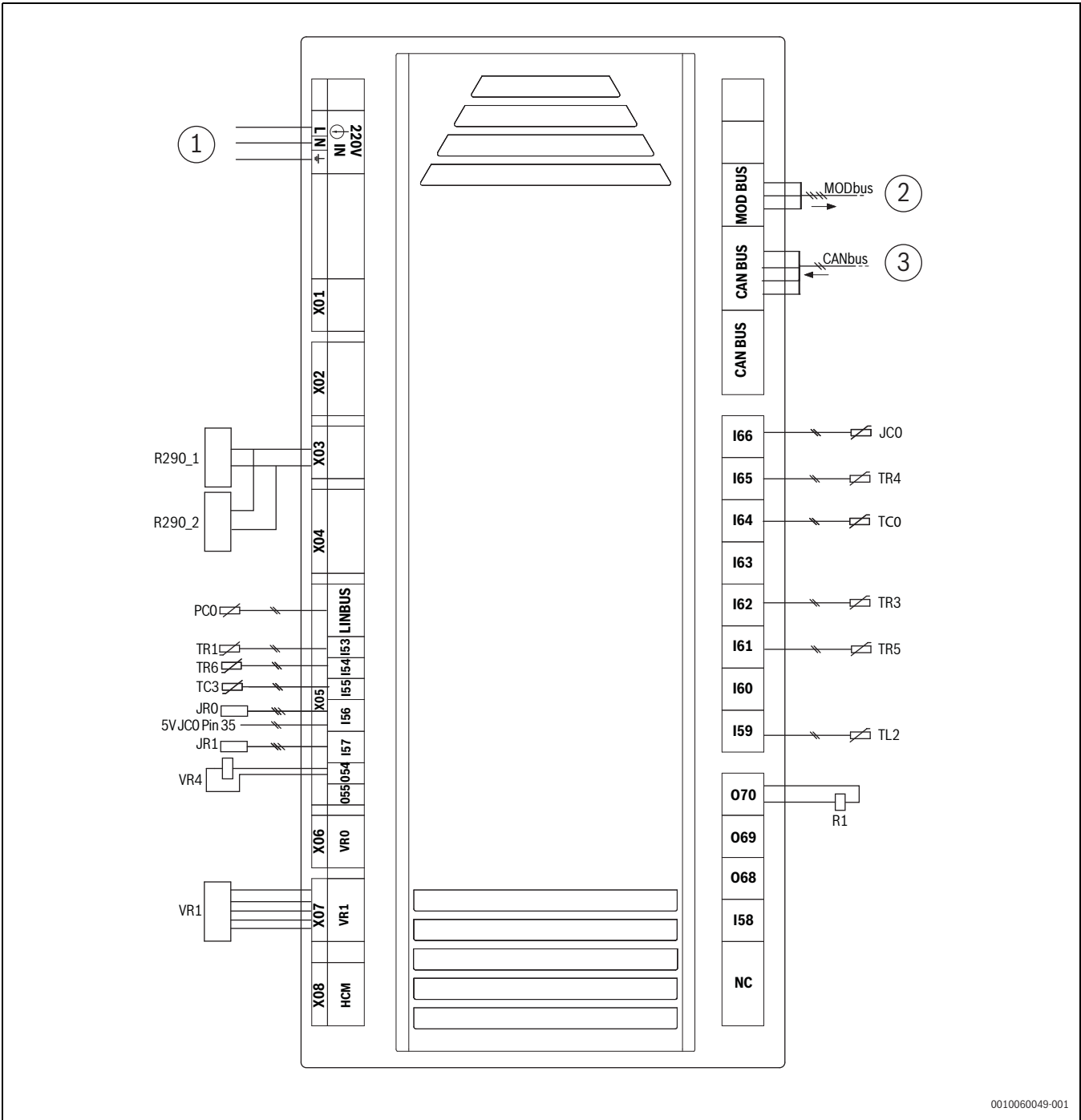
Fig. 110 Schema elettrico XCU-SRH (XCU-HP) con circolatore (ibrido)
