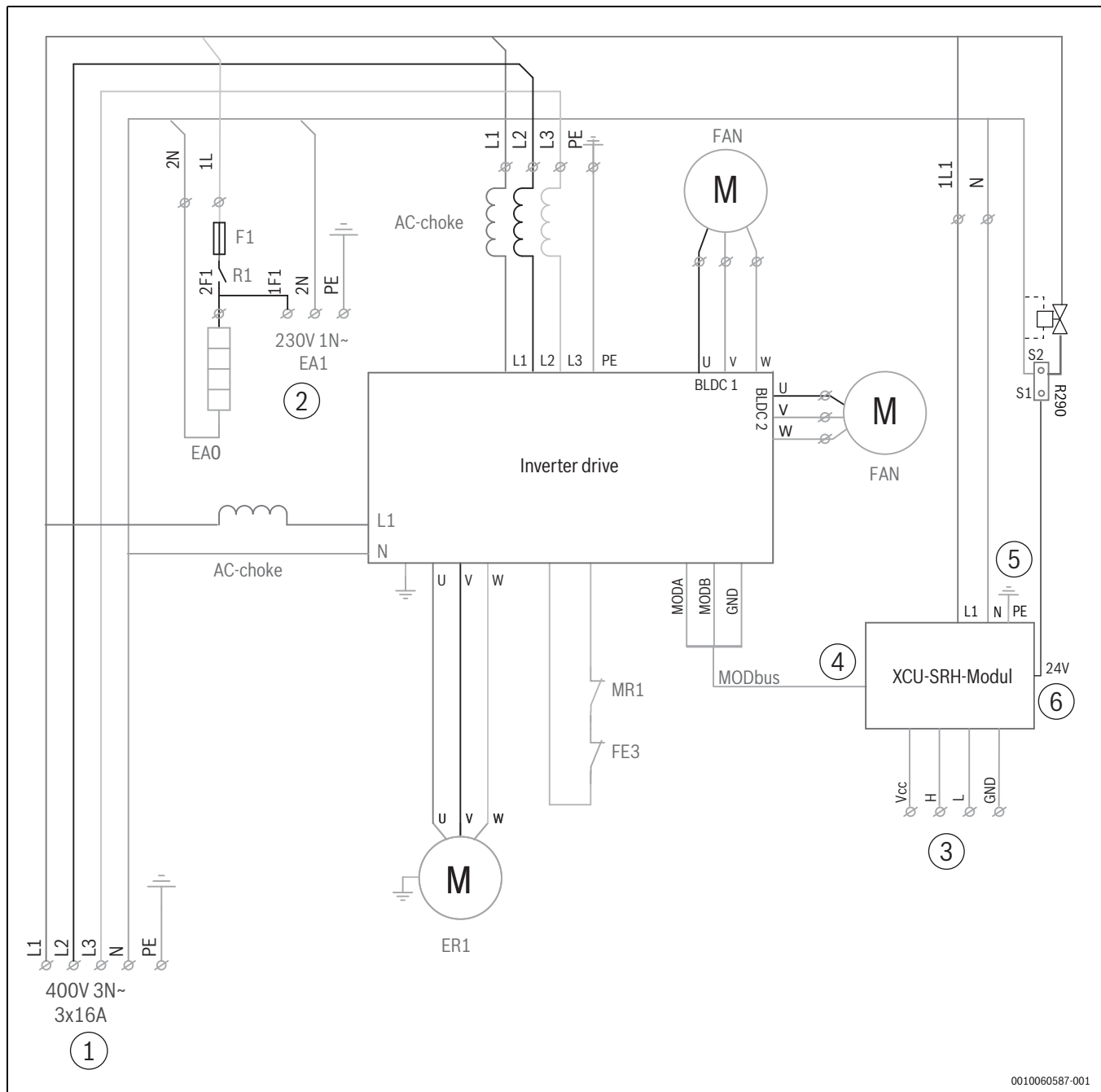
Afb. 56 Stroomkring 3 fase (houdt rekening met pre-installatie van de lekbakverwarming)
