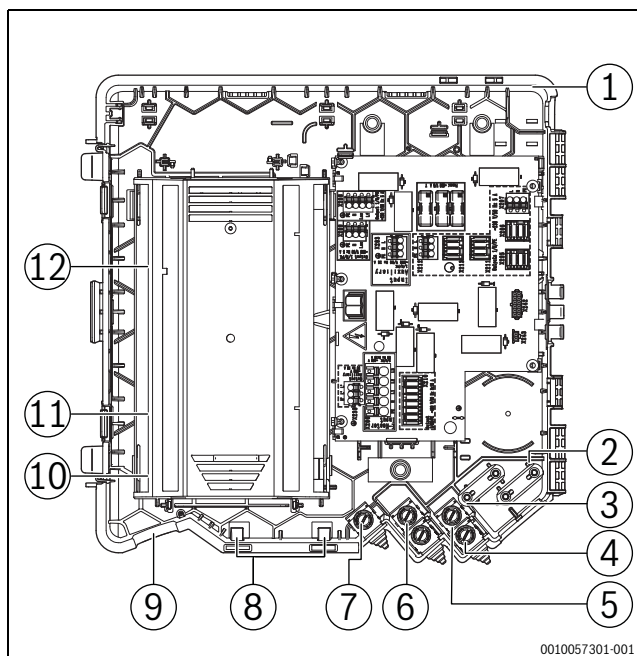
Bild 16 Kabelführung im Klemmenkasten (Netzanschluss, Zubehör und Kleinspannung)
