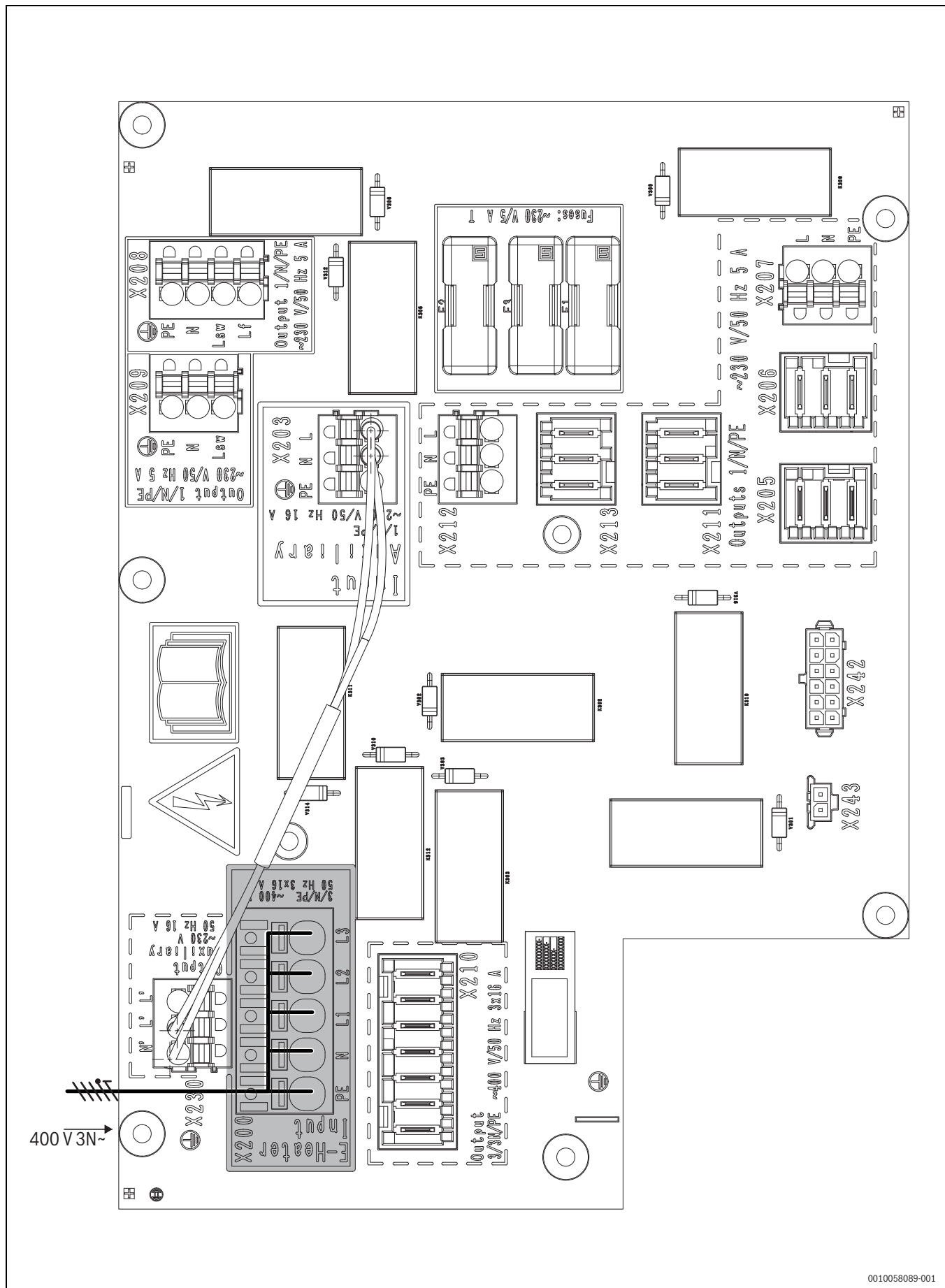
Bild 4 400 V-Anschluss für den elektrischen Zuheizer mit gebrücktem 230 V-Anschluss für die Steuerung und Pumpen
