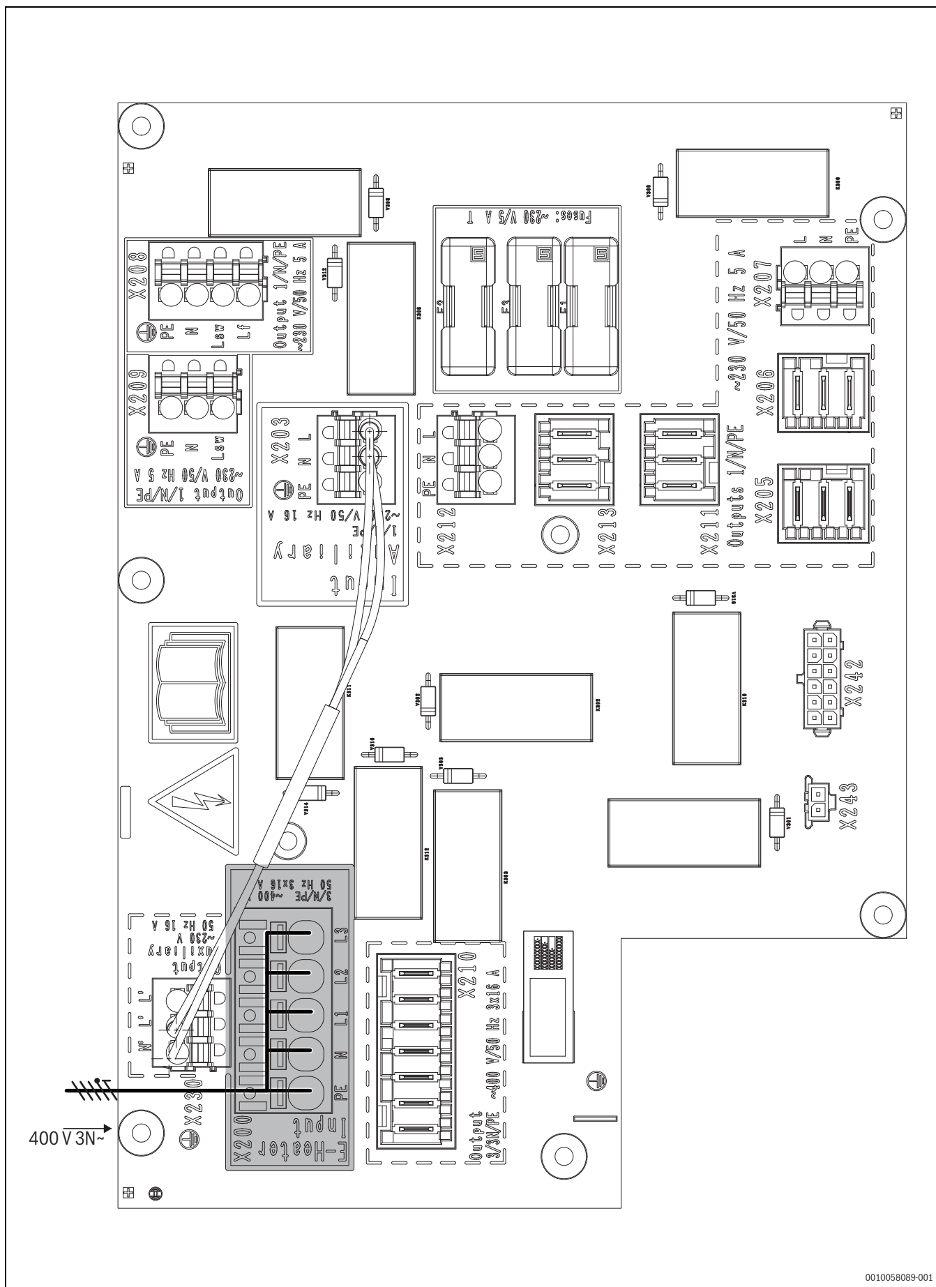
Afb. 32 400 V aansluiting voor de elektrische bijverwarming met overbrugde 230 V aansluiting voor de regeling en pompen.
