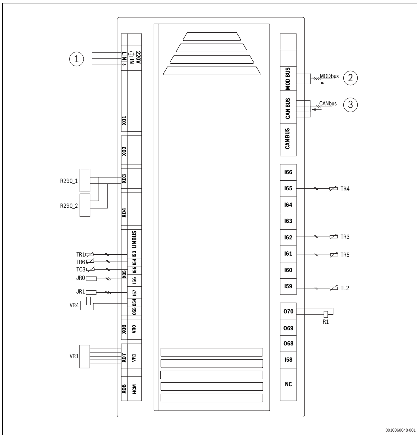
Fig. 109 Schema elettrico XCU-SRH (XCU-HP) senza circolatore (silenzioso)
