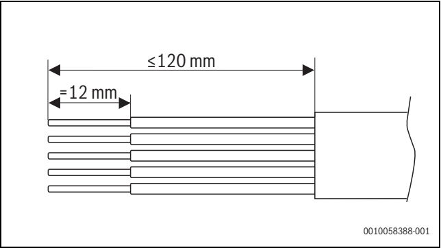
Afb. 30 Striplengte ader voedingsaansluiting
