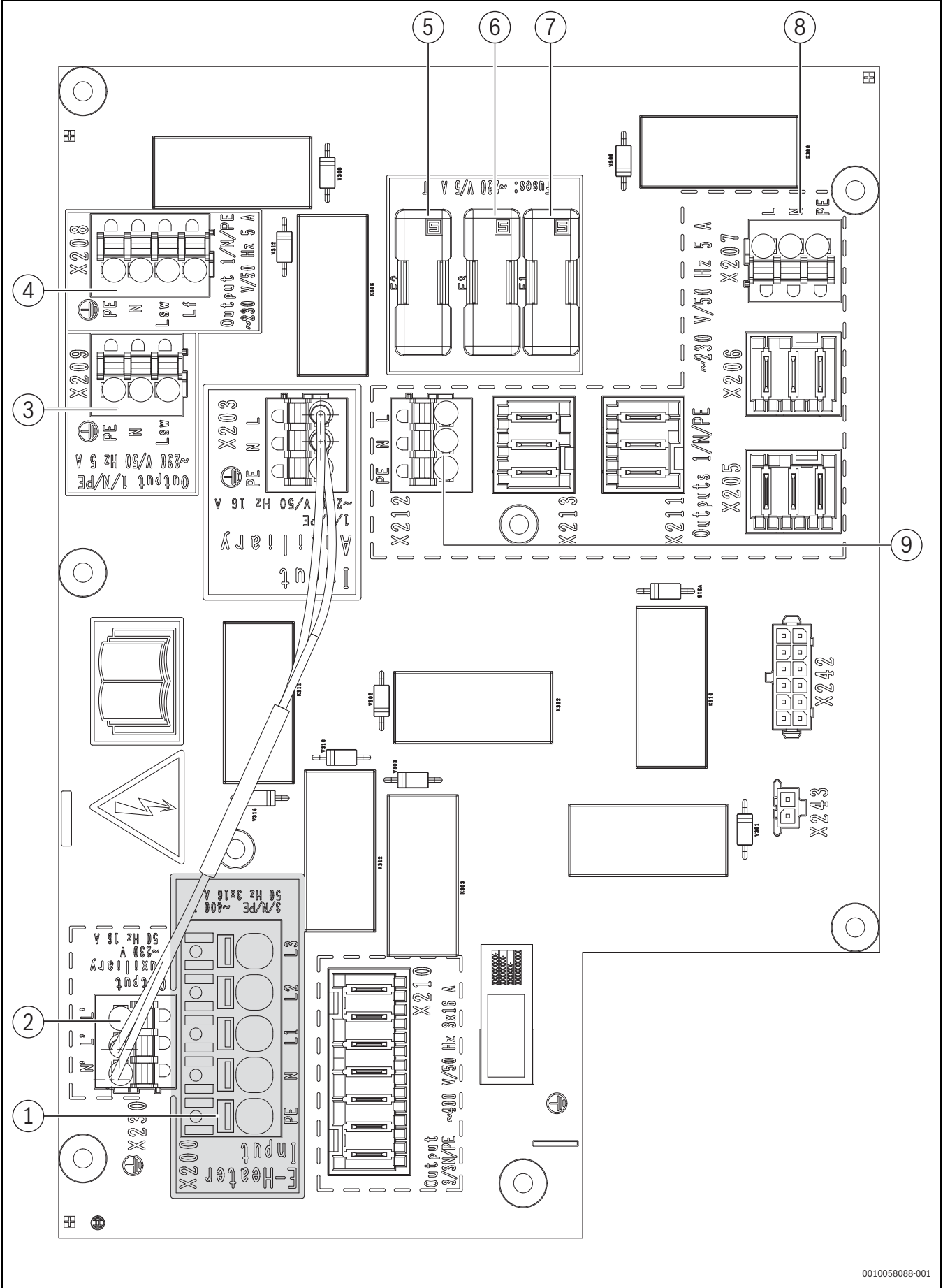
Fig. 59 Raccordements sur XCU-SEH
