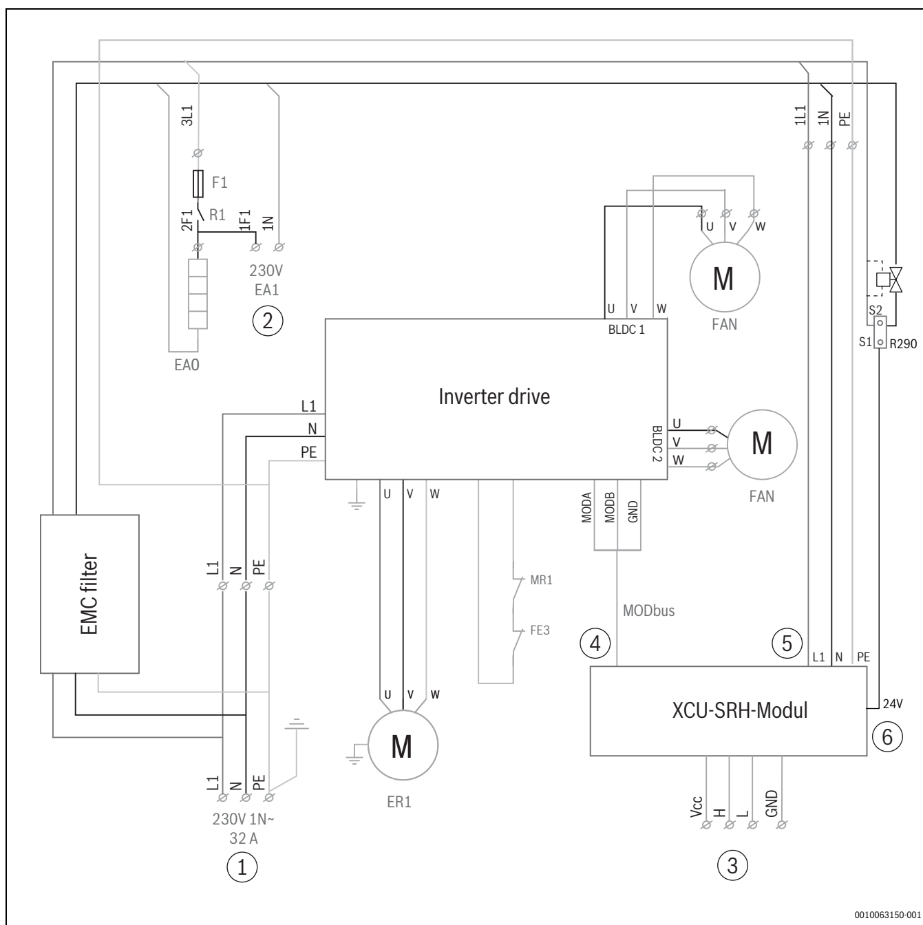
Rys. 168 Schemat elektryczny 1-fazowy (uwzględnić wstępną instalację podgrzewacza tacy skroplin)
