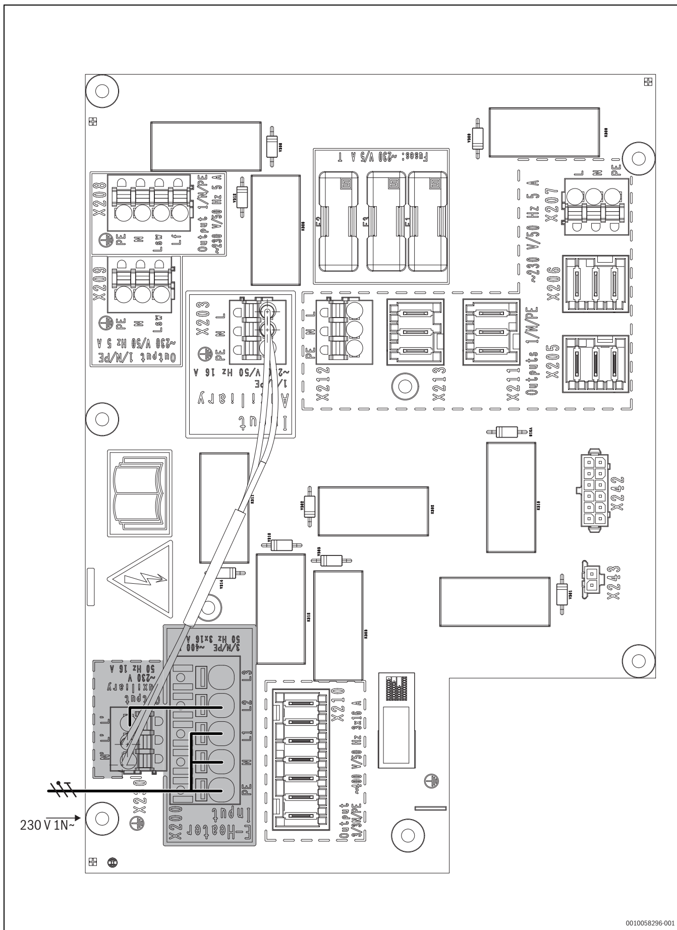
Afb. 33 230 V aansluiting voor de elektrische bijverwarming met overbrugde 230 V aansluiting voor de regeling en pompen.
