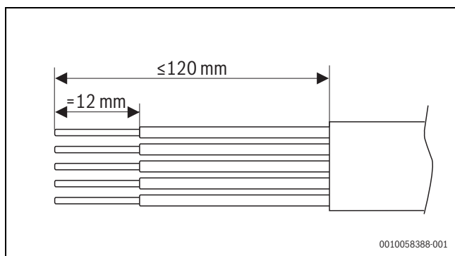
Fig. 87 Spellamento del cavo di alimentazione principale
