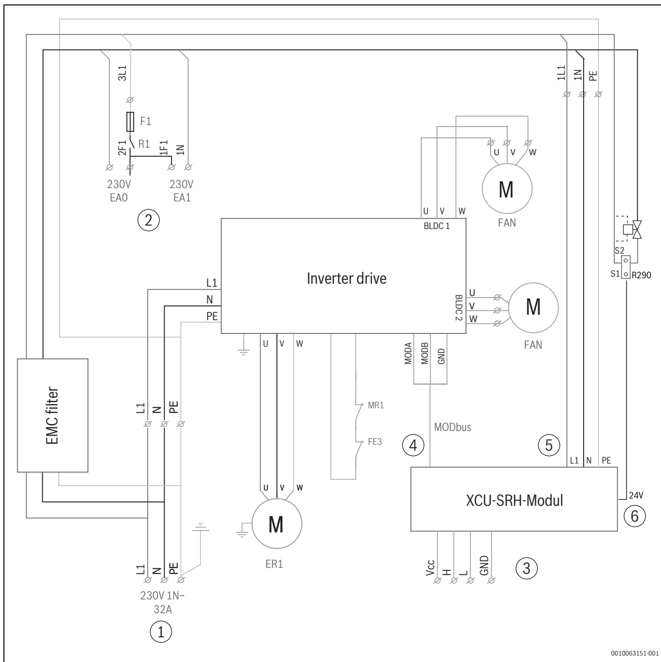
Fig. 111 Schema elettrico monofase (non considera la preinstallazione della resistenza della bacinella di raccolta condensa)
