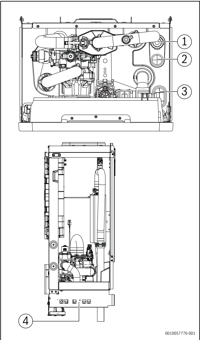
Afb. 125 Kabelwartels en doorvoeren naar de binnenunit (voedingsspanning, accessoires en laagspanning)
