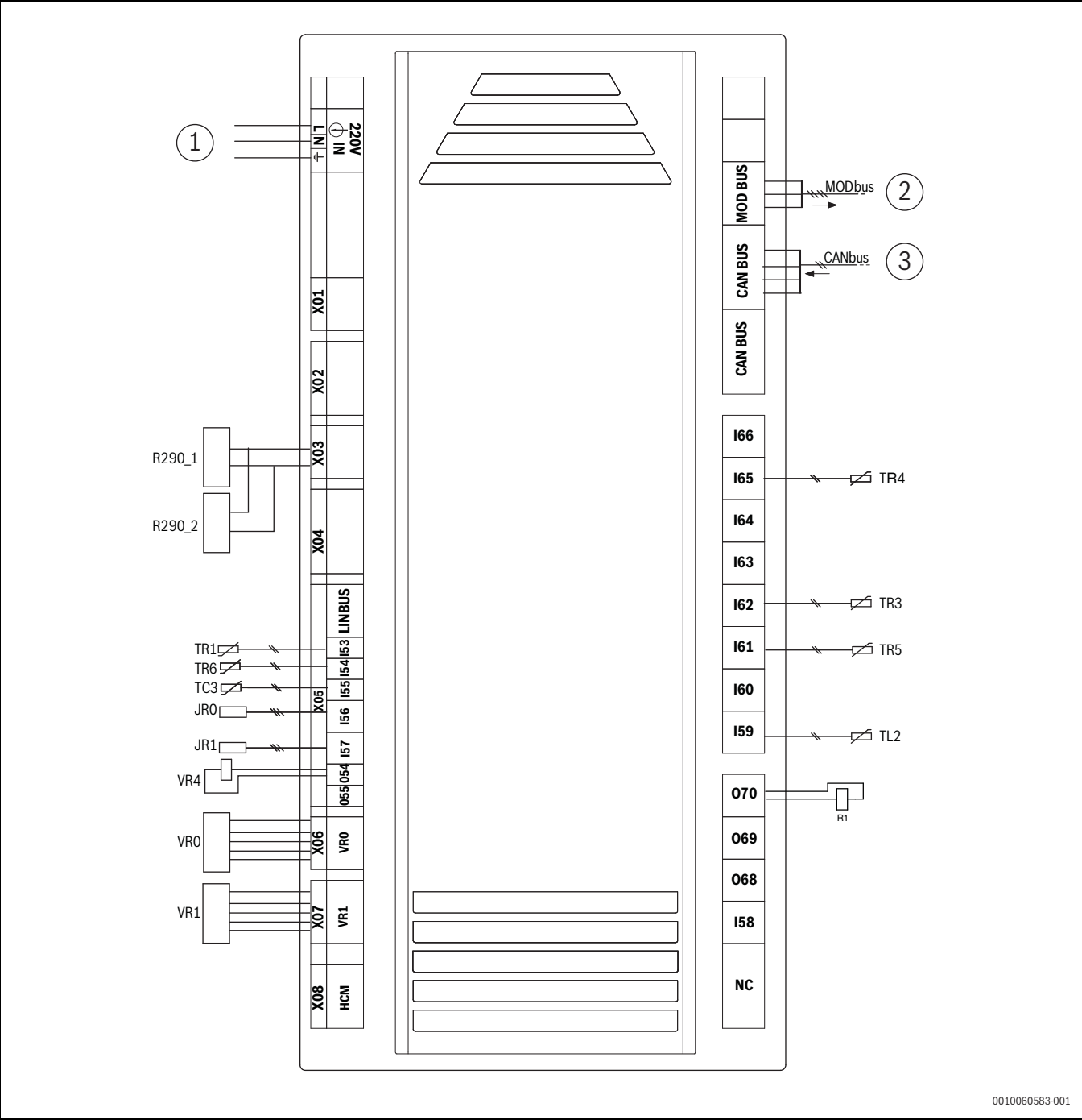
Fig. 86 Schéma du circuit XCU-SRH (XCU-HP)
