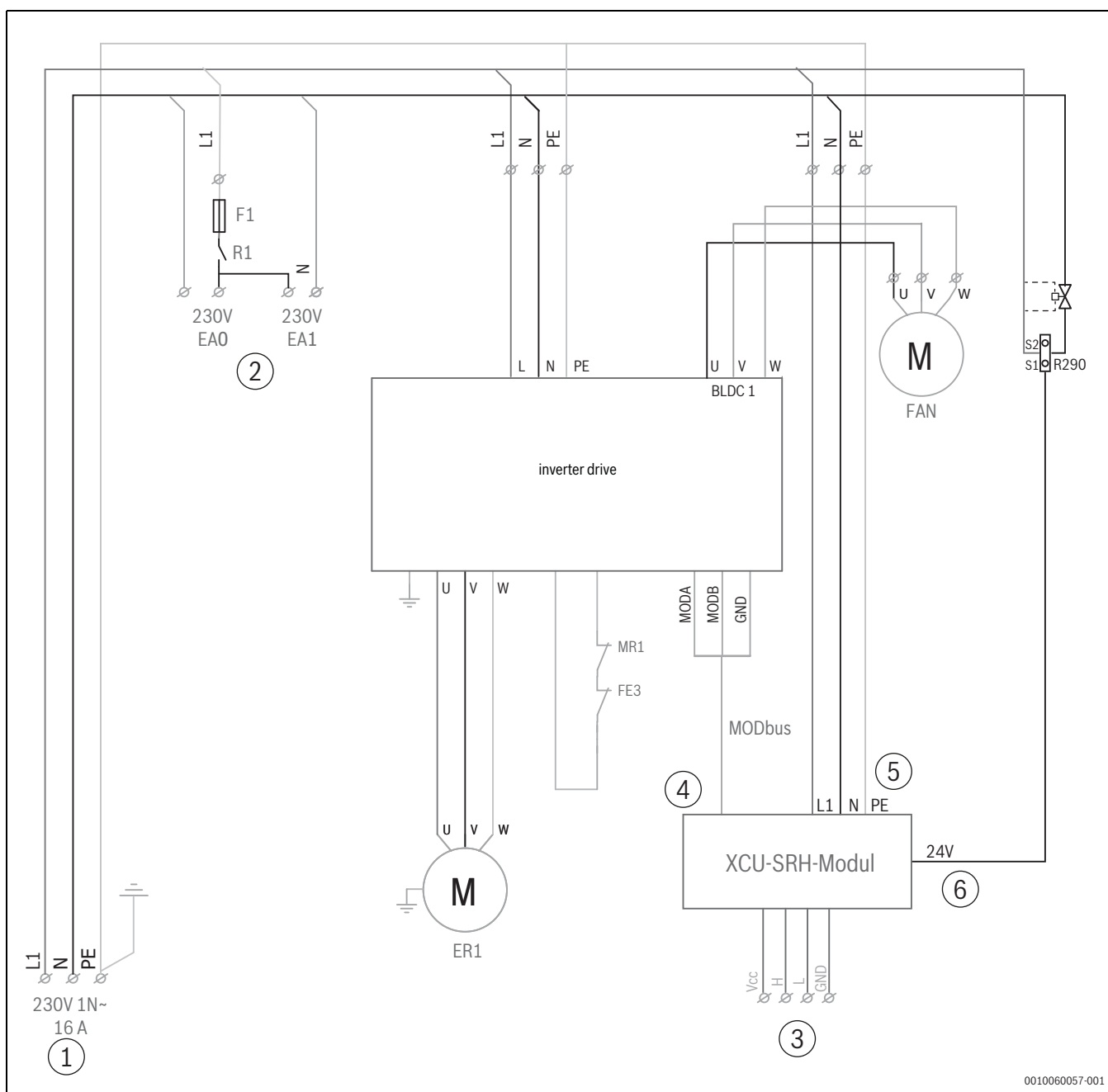
Afb. 134 Stroomkring zonder circulatiepomp (stil) met verwarmingskabel aangesloten in de fabriek
