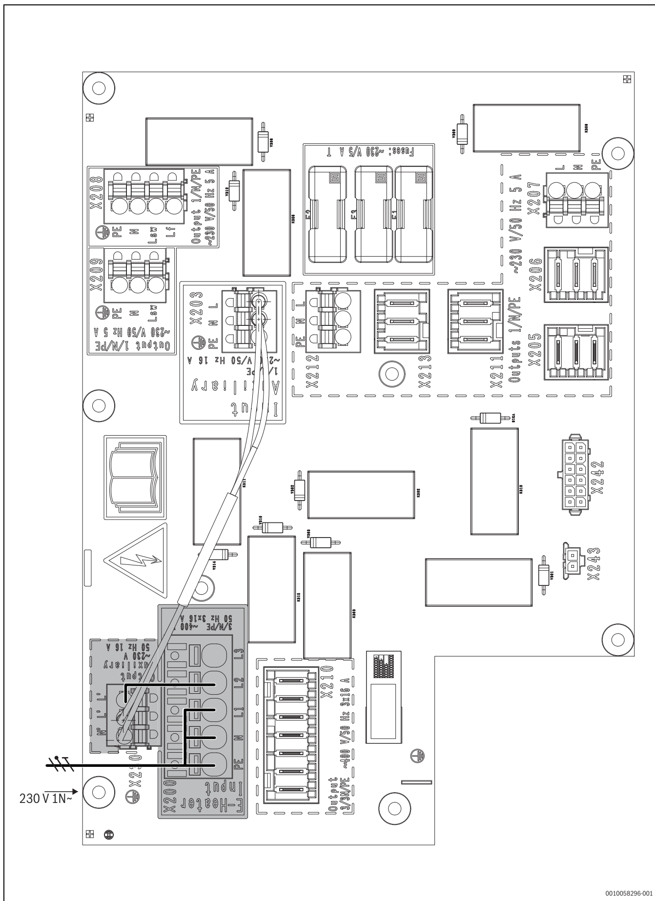
Rys. 147 Przyłącze 230 V ogrzewacza elektrycznego z połączeniem mostkowym 230 V na potrzeby sterowania i pomp
