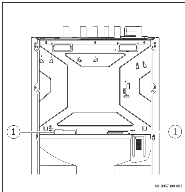
Rys. 156 Wejścia kablowe do jednostki wewnętrznej
