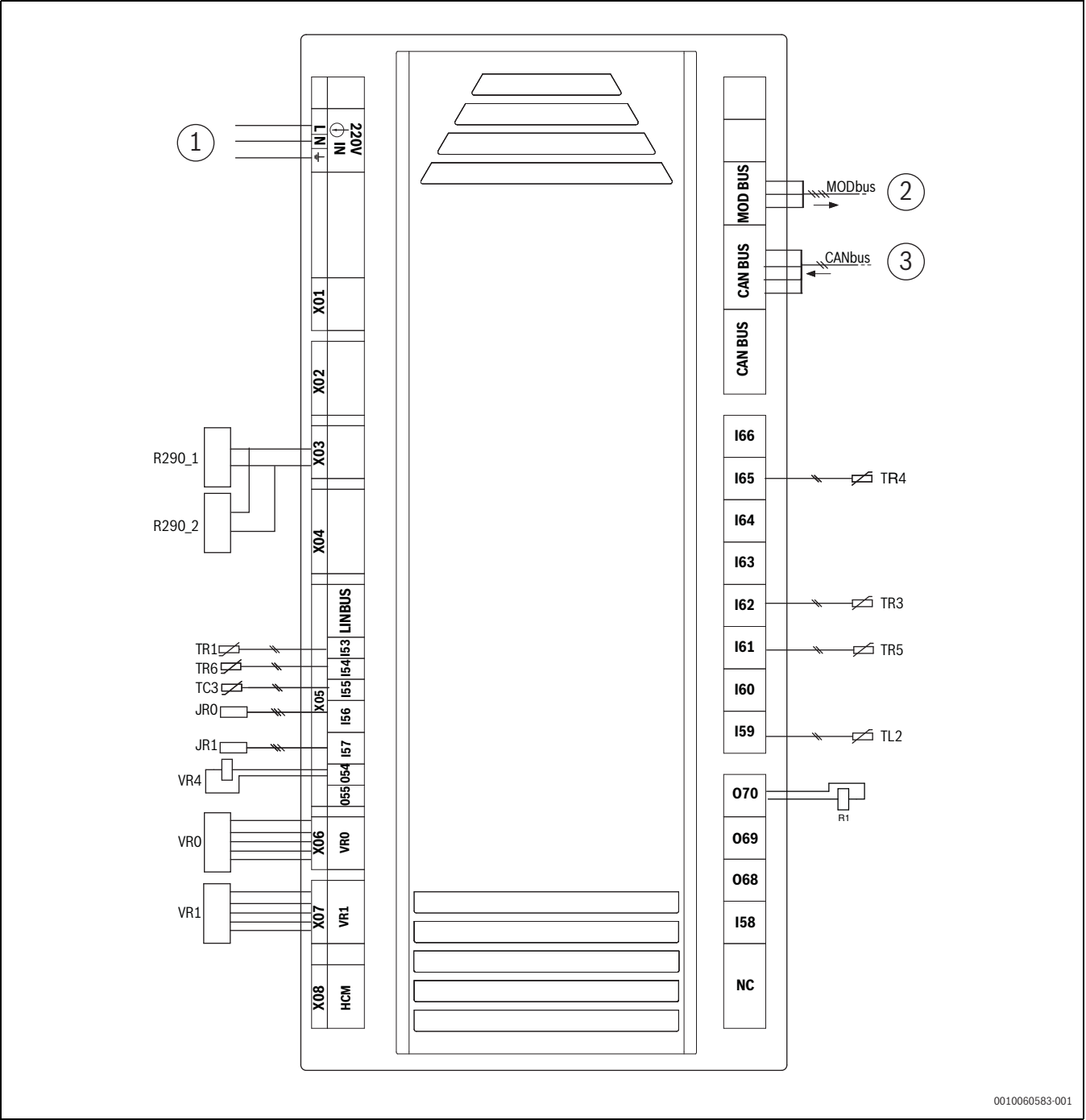
Afb. 143 Stroomkring XCU-SRH (XCU-HP)
