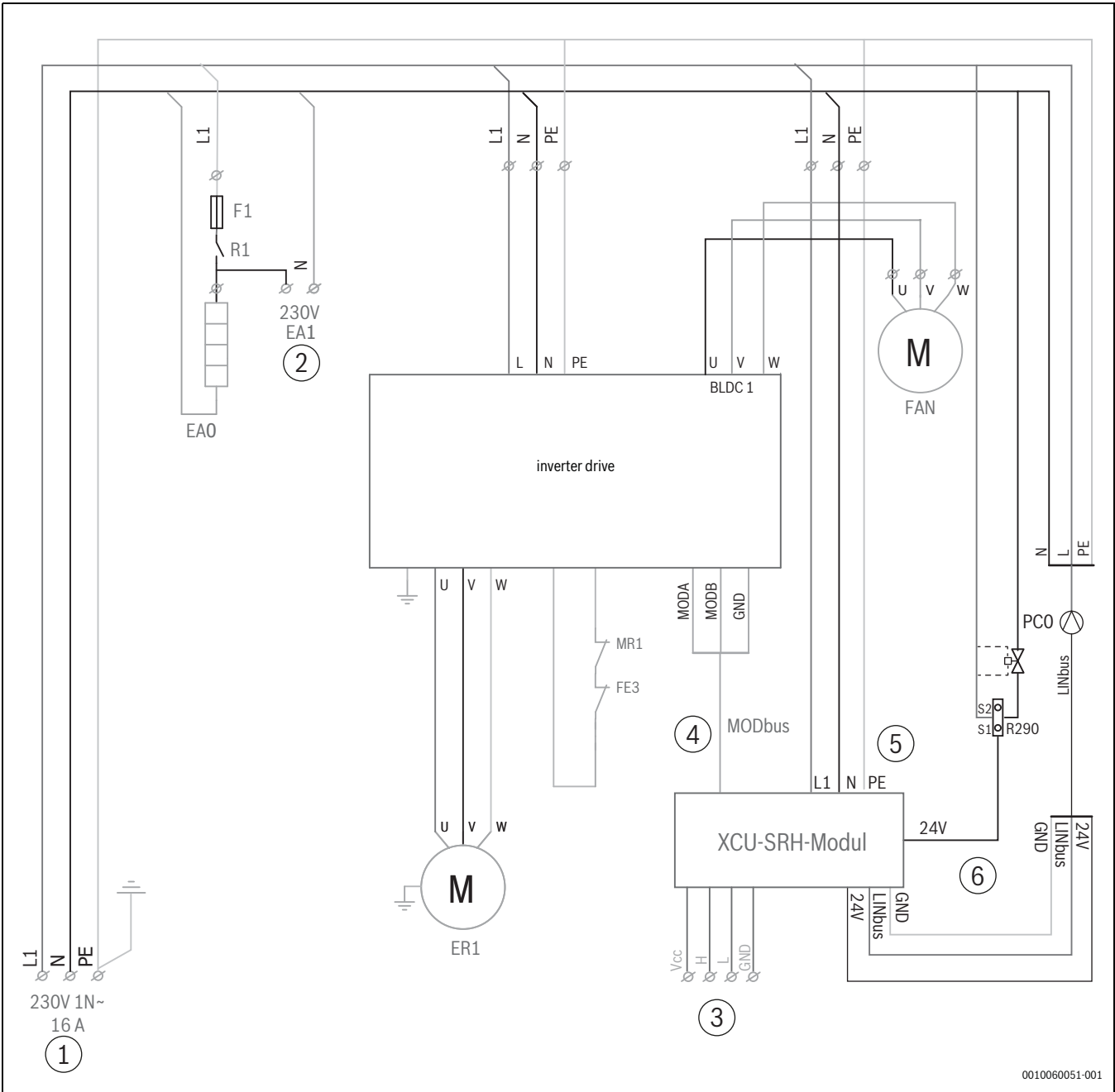
Afb. 135 Stroomkring met circulatiepomp (hybride) met verwarmingskabel aangesloten in de fabriek
