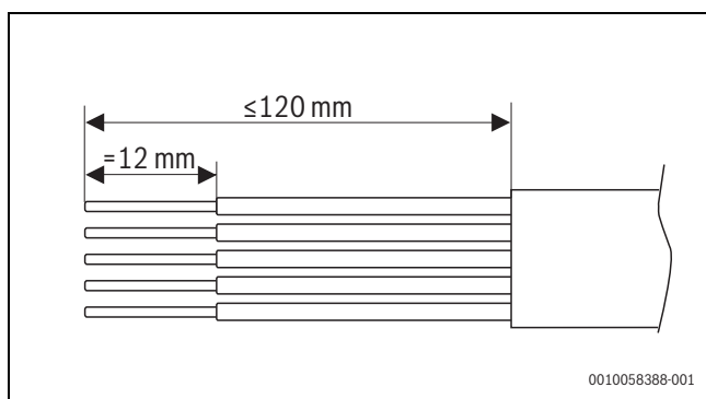
Fig. 58 Raccordement à l'alimentation secteur avec dénudage des fils
