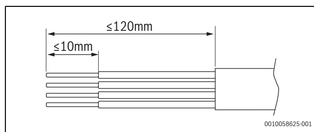
Bild 9 Abisolierung CAN-BUS
