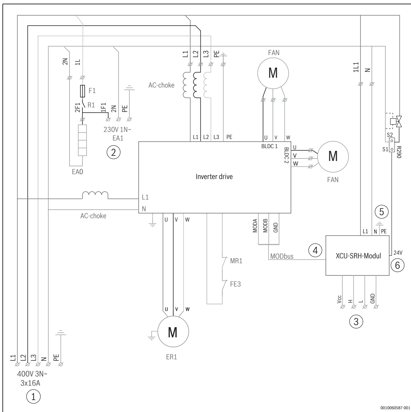
Fig. 85 Schéma électrique triphasé (avec prise en compte du pré-équipement du chauffage de bac à condensats)
