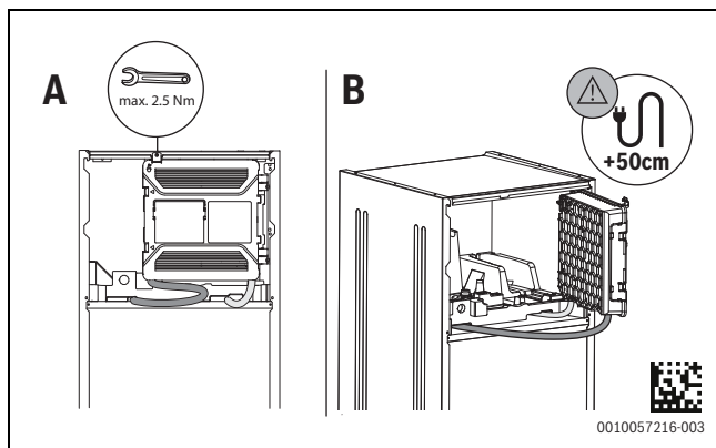
Fig. 101 Passaggio dei cavi all'unità interna
