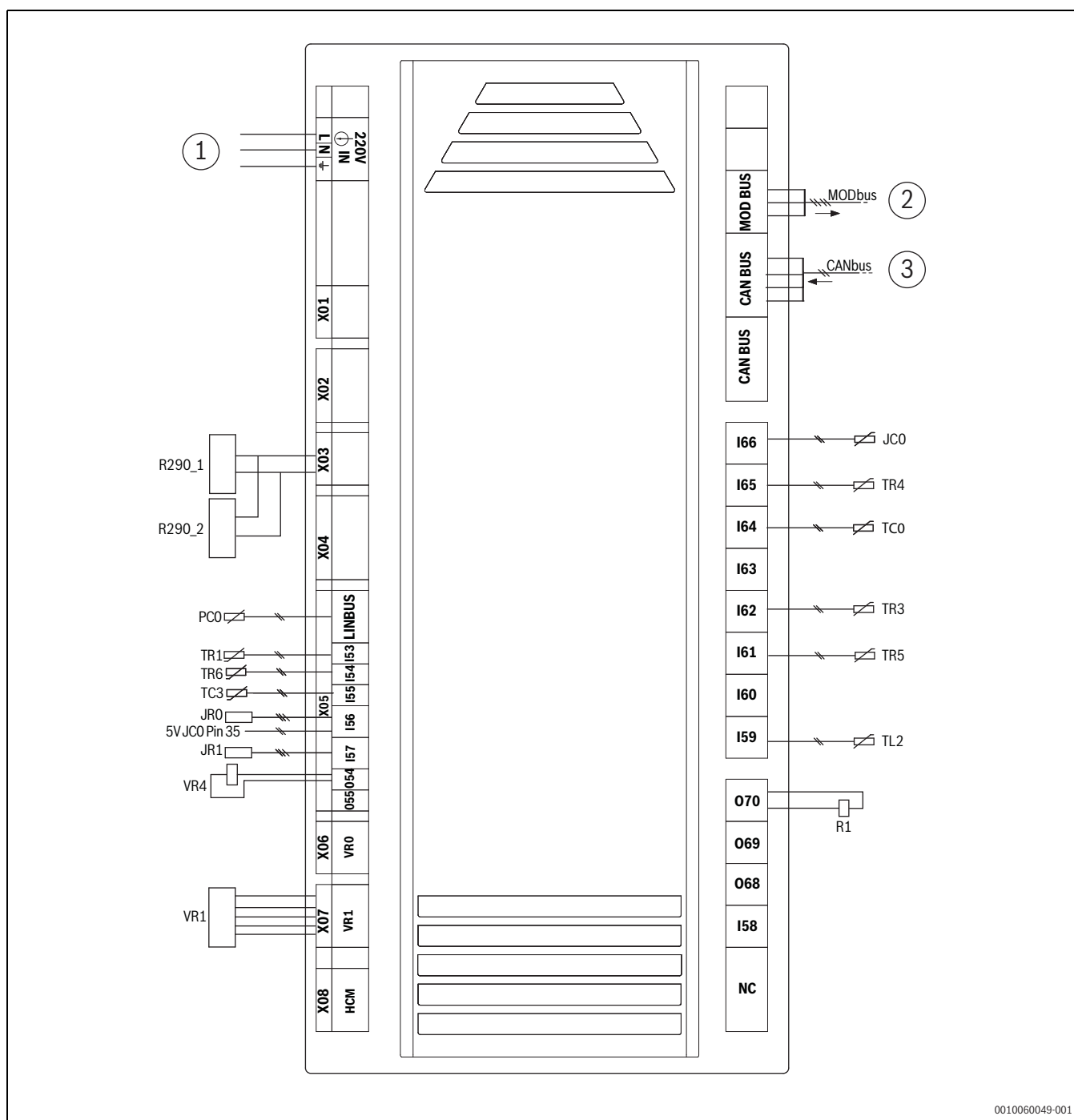
Rys. 166 Schemat elektryczny XCU-SRH (XCU-HP) z pompą cyrkulacyjną (system hybrydowy)
