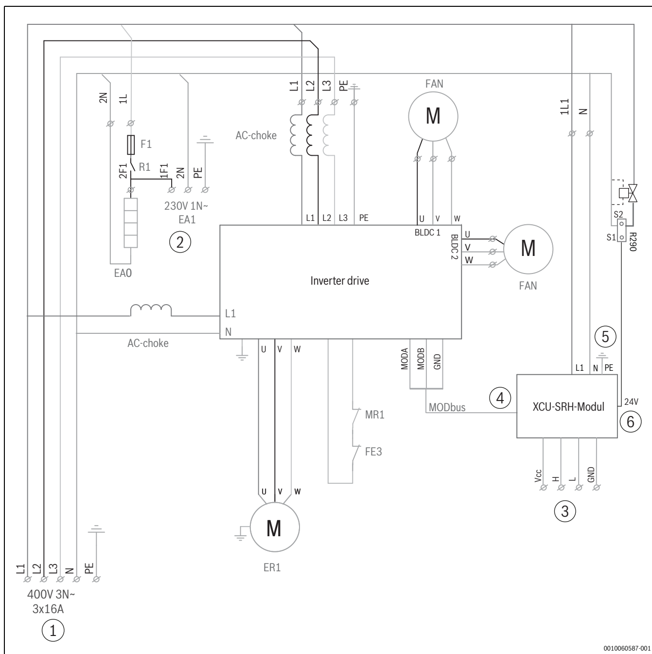
Rys. 170 Schemat elektryczny 3-fazowy (uwzględnia wstępną instalację podgrzewacza tacy skroplin)
