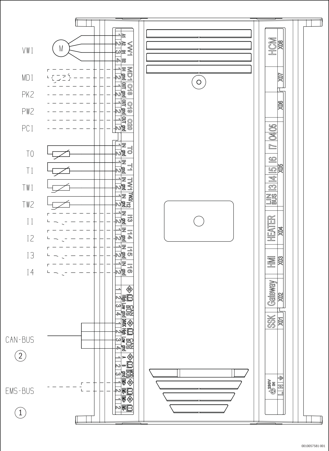
Fig. 103 Collegamenti XCU-THH
