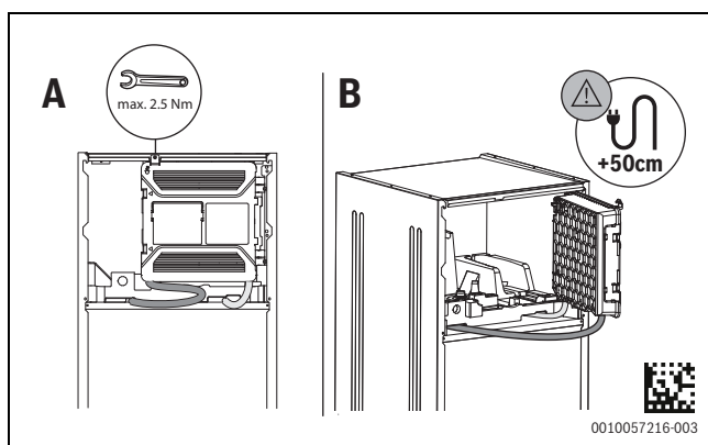
Afb. 129 Kabeldoorvoeren naar de binnenunit
