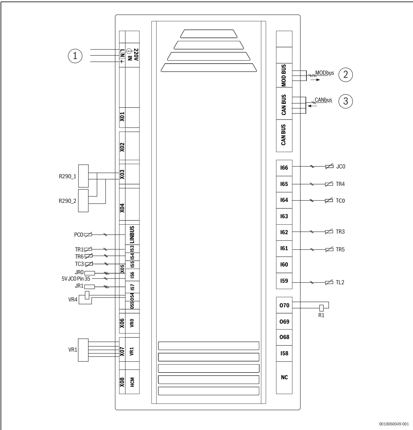
Fig. 81 Schéma du circuit XCU-SRH (XCU-HP) avec pompe de circulation (hybride)
