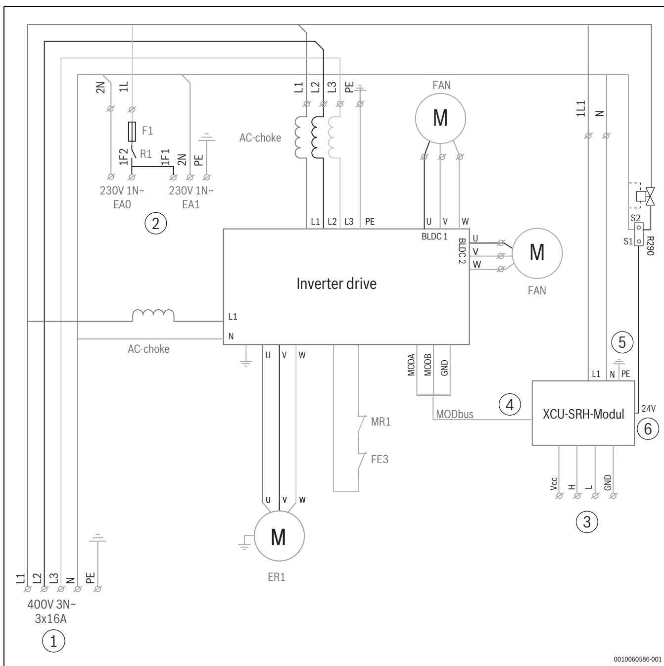
Rys. 169 Schemat elektryczny 3-fazowy (nie uwzględnia wstępnej instalacji podgrzewacza tacy skroplin)
