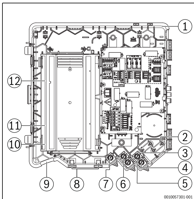
Afb. 130 Kabelinstallatie in de aansluitdoos (voedingsspanning, accessoires en laagspanning)
