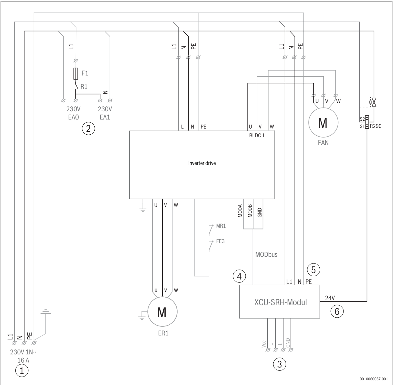
Fig. 106 Schema elettrico senza circolatore (silenzioso) senza cavo scaldante collegato in fabbrica
