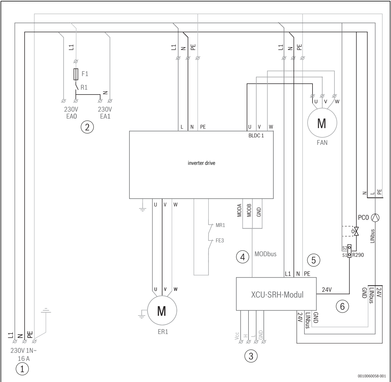
Afb. 50 Stroomkring met circulatiepomp (hybride) zonder verwarmingskabel aangesloten in de fabriek
