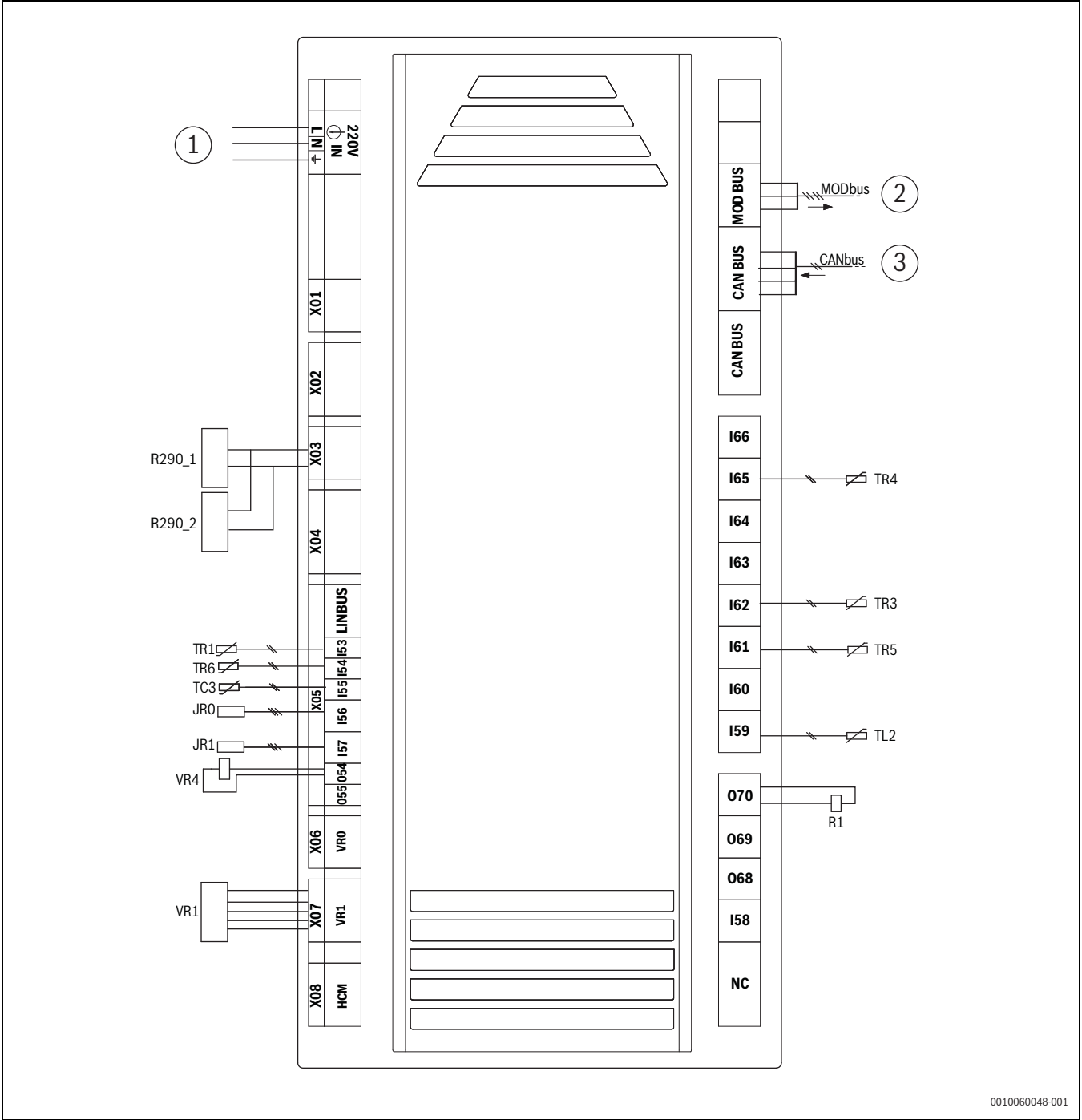
Afb. 137 Stroomkring XCU-SRH (XCU-HP) zonder circulatiepomp (stil)
