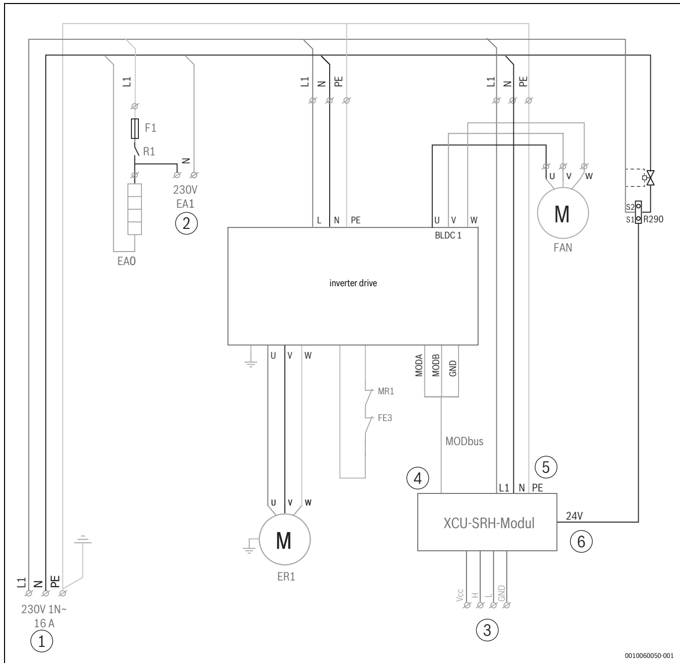
Afb. 133 Stroomkring SC zonder circulatiepomp (stil) met verwarmingskabel aangesloten in de fabriek
