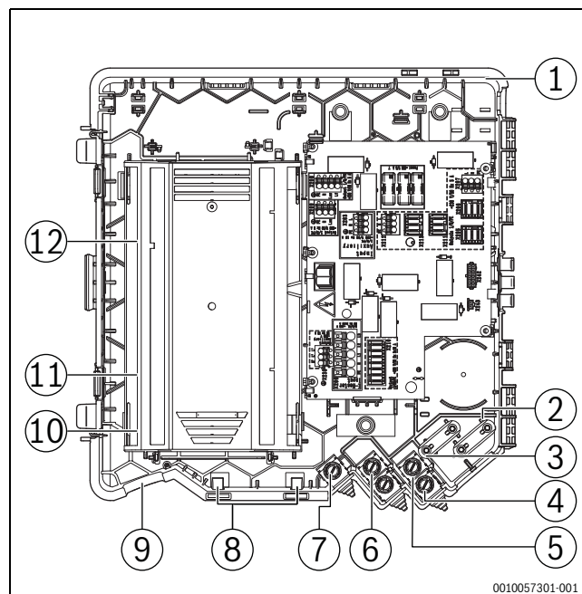
Rys. 158 Prowadzenie przewodów w skrzynce zaciskowej (główne zasilanie, osprzęt dodatkowy i niskie napięcie)
