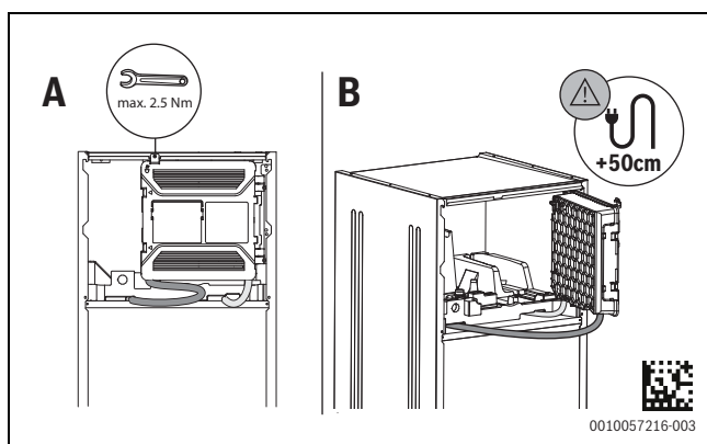
Fig. 72 Passe-câbles vers l'unité intérieure
