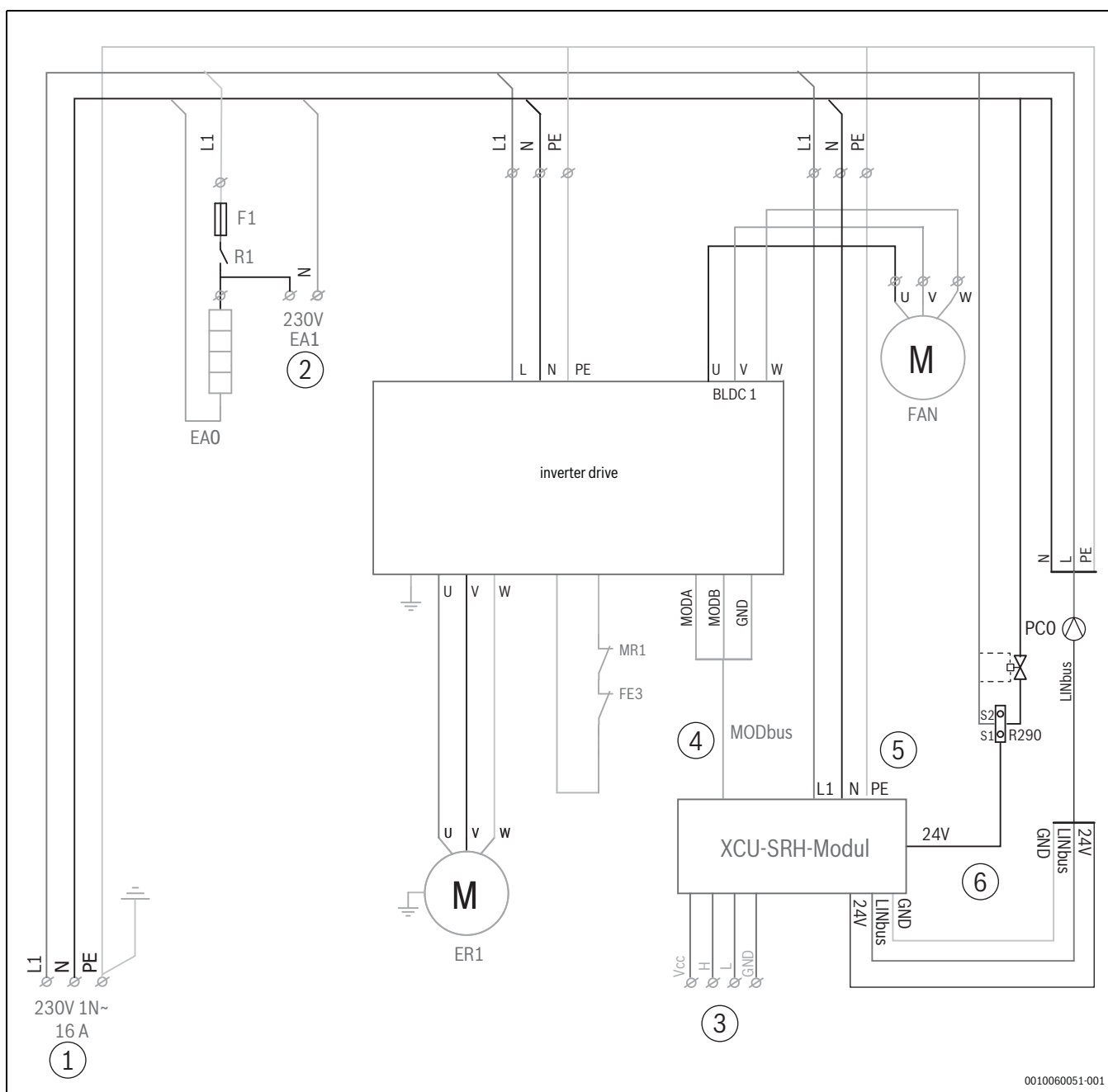
Fig. 78 Schéma du circuit avec pompe de circulation (hybride) avec câble chauffant raccordé en usine
