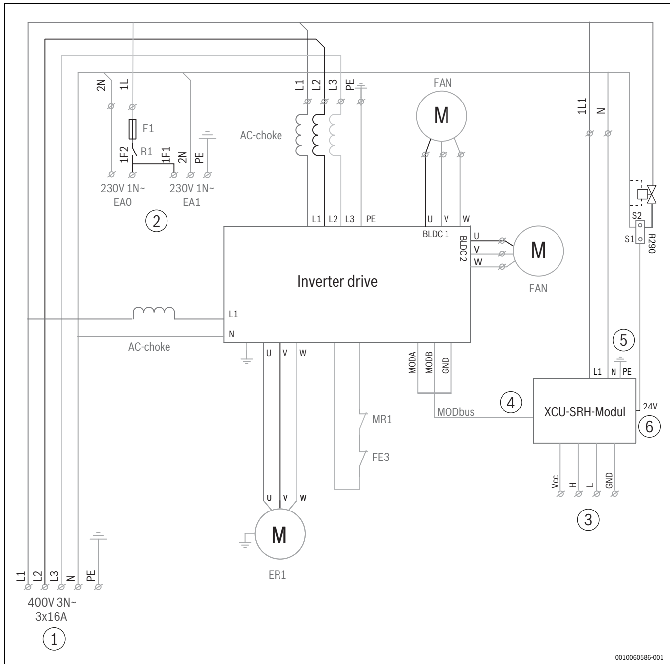
Bild 27 Schaltplan 3-phasig (berücksichtigt nicht die Vorinstallation der Kondensatwannenheizung)
