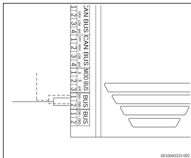
Bild 10 EMS-Anschluss
