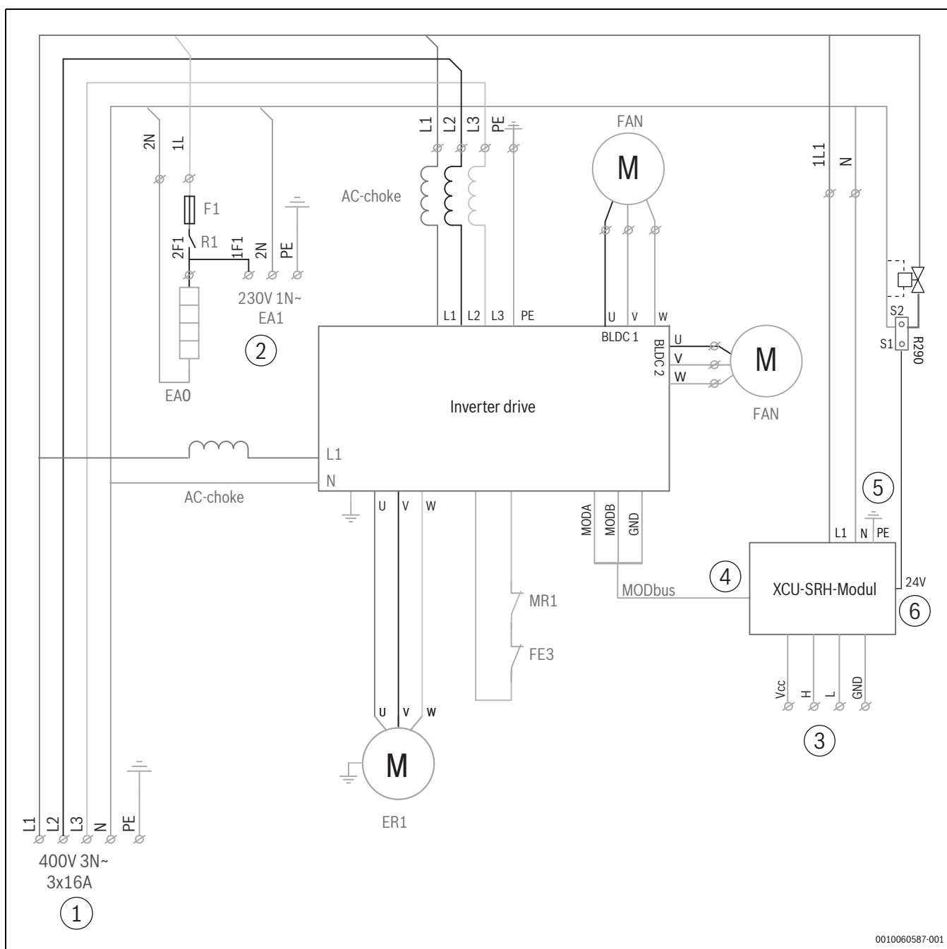
Afb. 142 Aansluitschema 3 fase (houdt rekening met pre-installatie van de druppelvangerverwarming)
