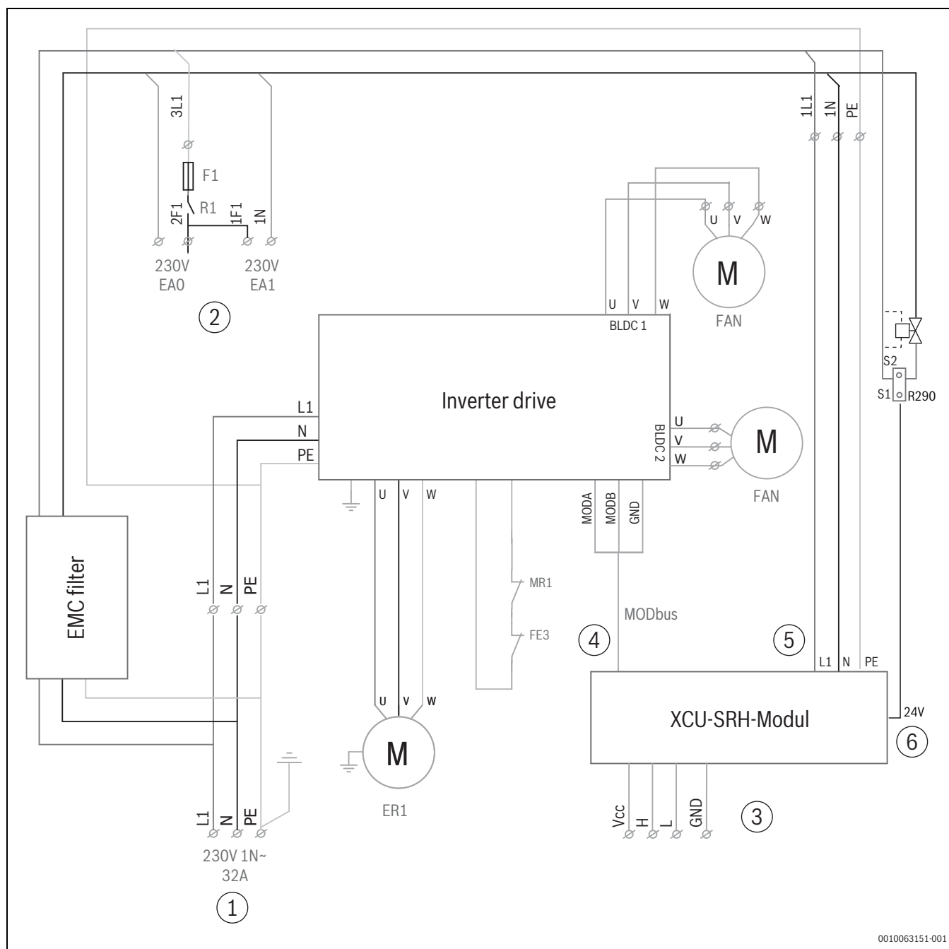
Afb. 53 Stroomkring 1 fase (houdt geen rekening met pre-installatie van de lekbakverwarming)
