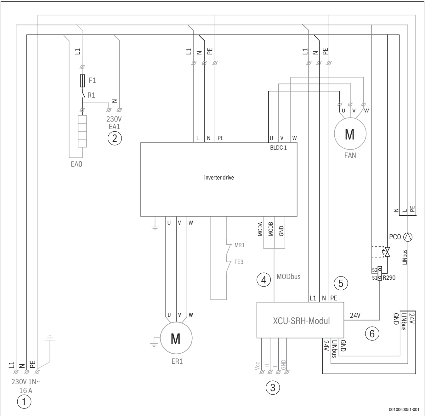
Bild 21 Schaltplan mit Zirkulationspumpe (Hybrid) mit werkseitig angeschlossenen Heizkabel
