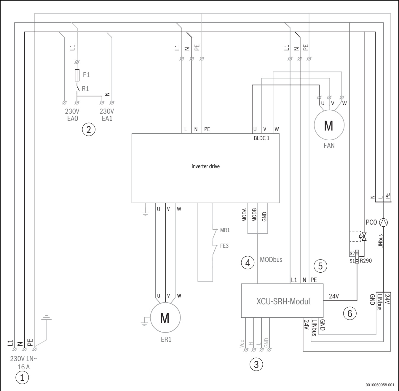
Fig. 79 Schéma du circuit avec pompe de circulation (hybride) sans câble chauffant raccordé en usine
