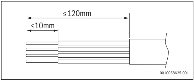
Rys. 151 Zdejmowanie izolacji z przewodów magistrali CAN BUS
