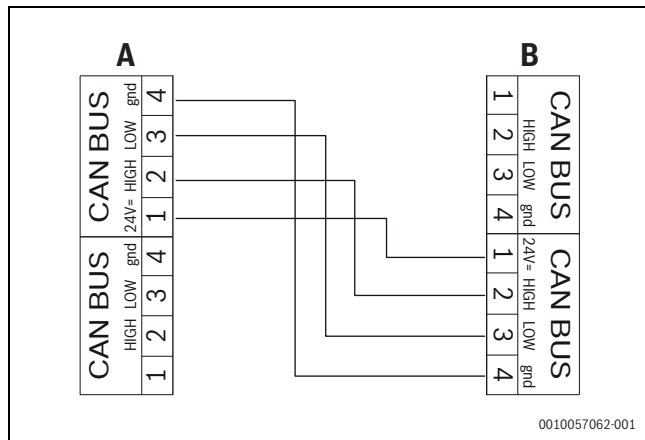
Fig. 64 BUS CAN, unité extérieure - unité intérieure
