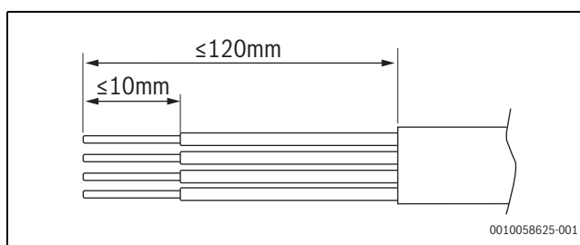
Fig. 66 Dénudage CAN-BUS
