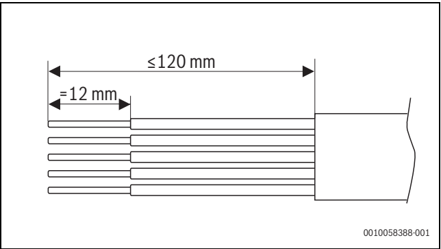
Rys. 144 Usuwanie izolacji z przewodu zasilania sieciowego
