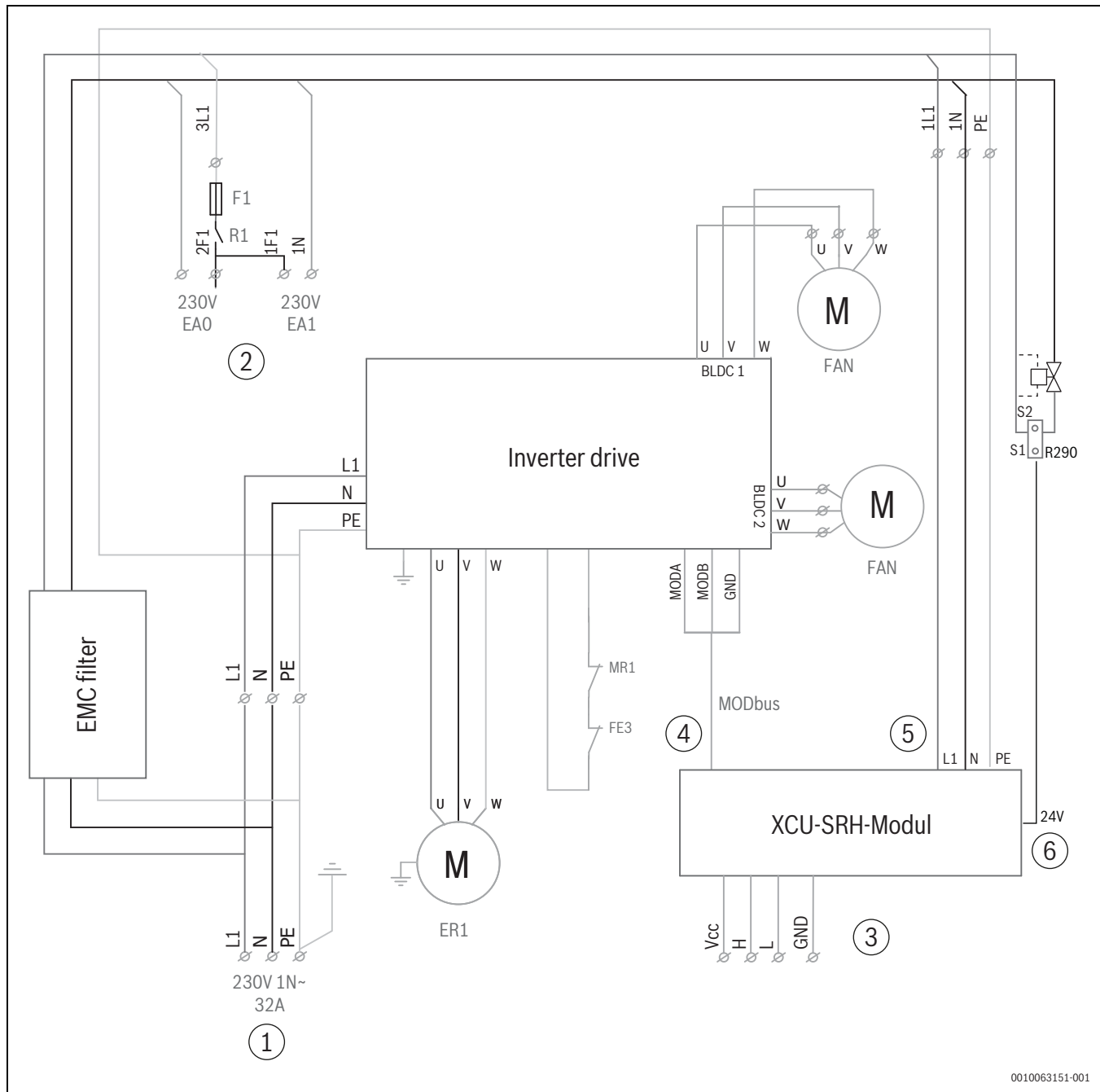
Afb. 139 Aansluitschema 1 fase (houdt geen rekening met pre-installatie van de druppelvangerverwarming)
