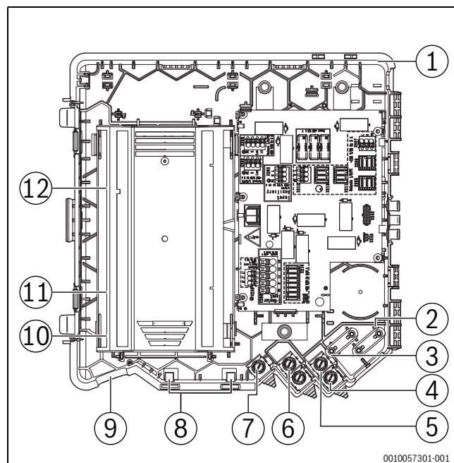
Fig. 73 Chemin de câbles dans le boîtier électrique (alimentation principale, accessoires et basse tension)
