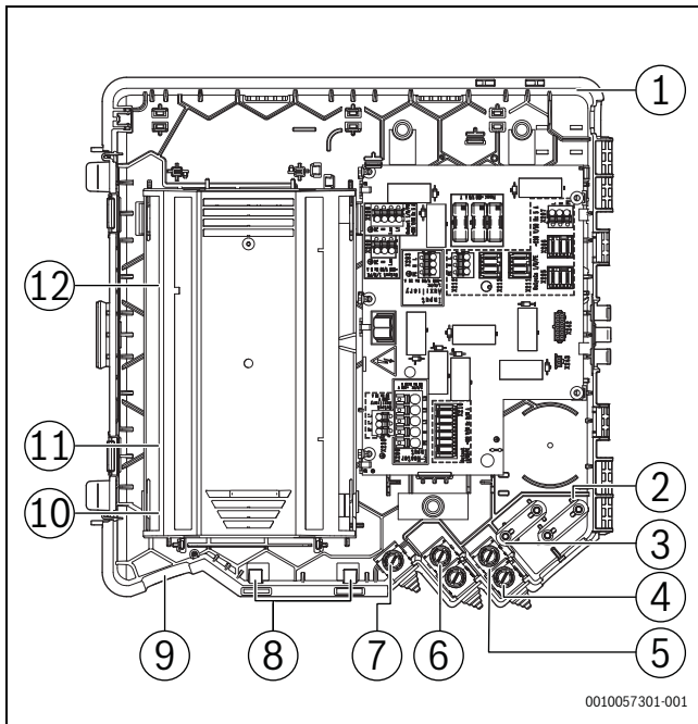
Afb. 40 Kabeldoorvoering in de aansluitdoos (voedingsspanning, accessoires en laagspanning)
