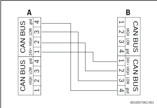
Fig. 93 CAN-BUS unità esterna - unità interna
