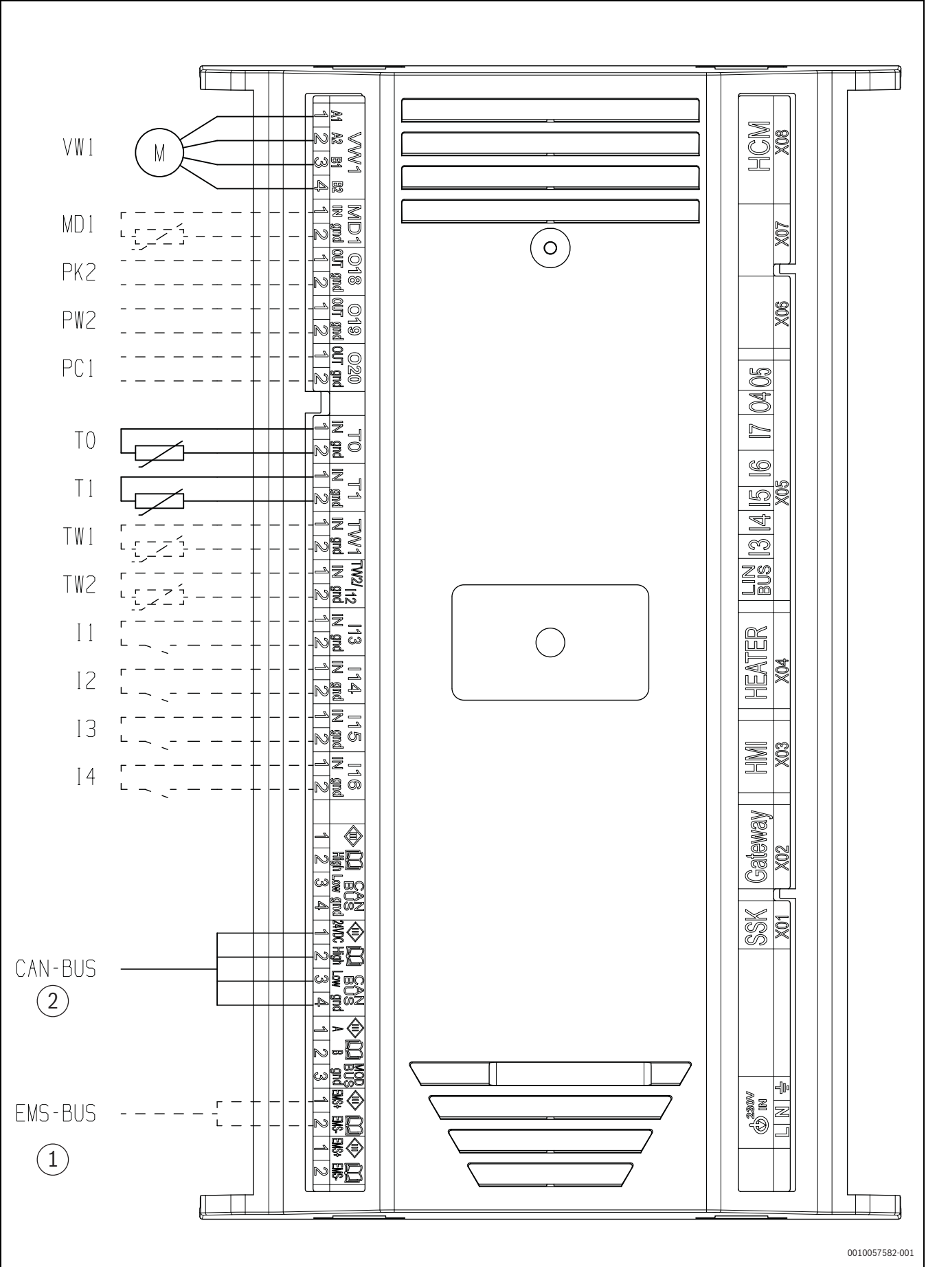
Bild 13 Anschlüsse XCU-THH [VW1]3-Wege-Ventil Heizung/Warmwasserspeicher [MD1]Kondensationsfühler (Zubehör für Kühlbetrieb)
