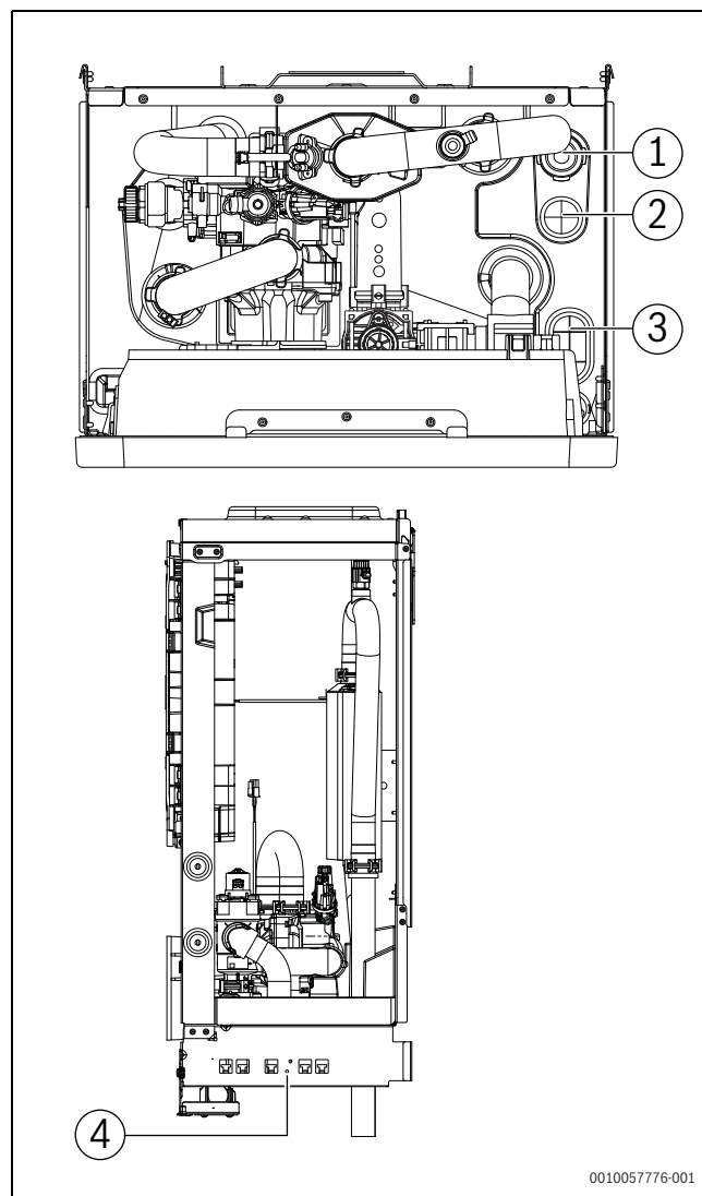
Rys. 153 Dławnica kablowa i tulejki do jednostki wewnętrznej (główne zasilanie, akcesoria i niskie napięcie)
