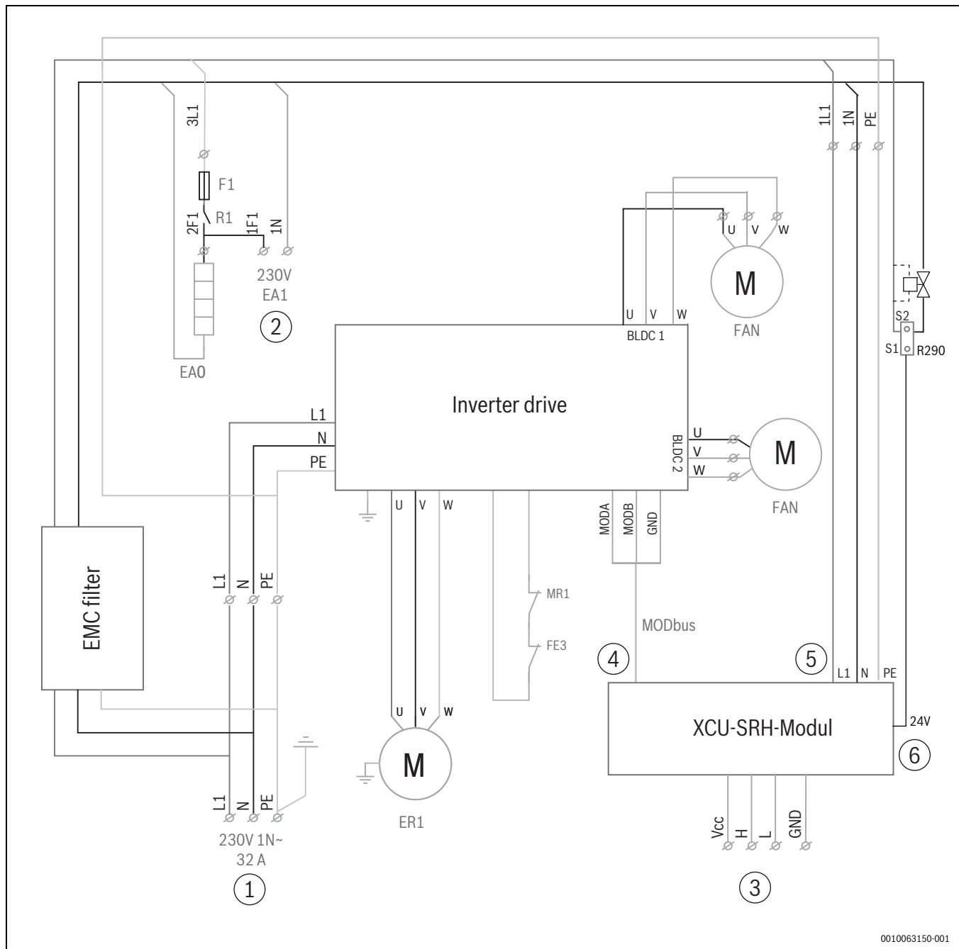
Afb. 54 Stroomkring 1 fase (houdt rekening met pre-installatie van de lekbakverwarming)
