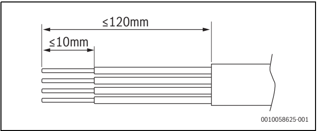
Afb. 37 Stripten CAN-BUS
