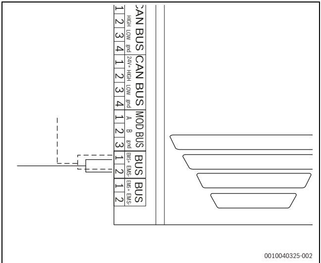
Rys. 152 Podłączanie EMS
