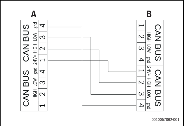
Rys. 149 Magistrala CAN-BUS jednostka zewnętrzna – jednostka wewnętrzna
