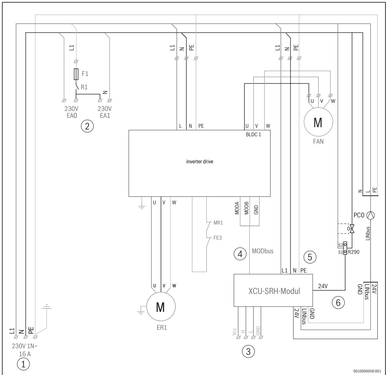
Afb. 136 Stroomkring met circulatiepomp (hybride) zonder verwarmingskabel aangesloten in de fabriek
