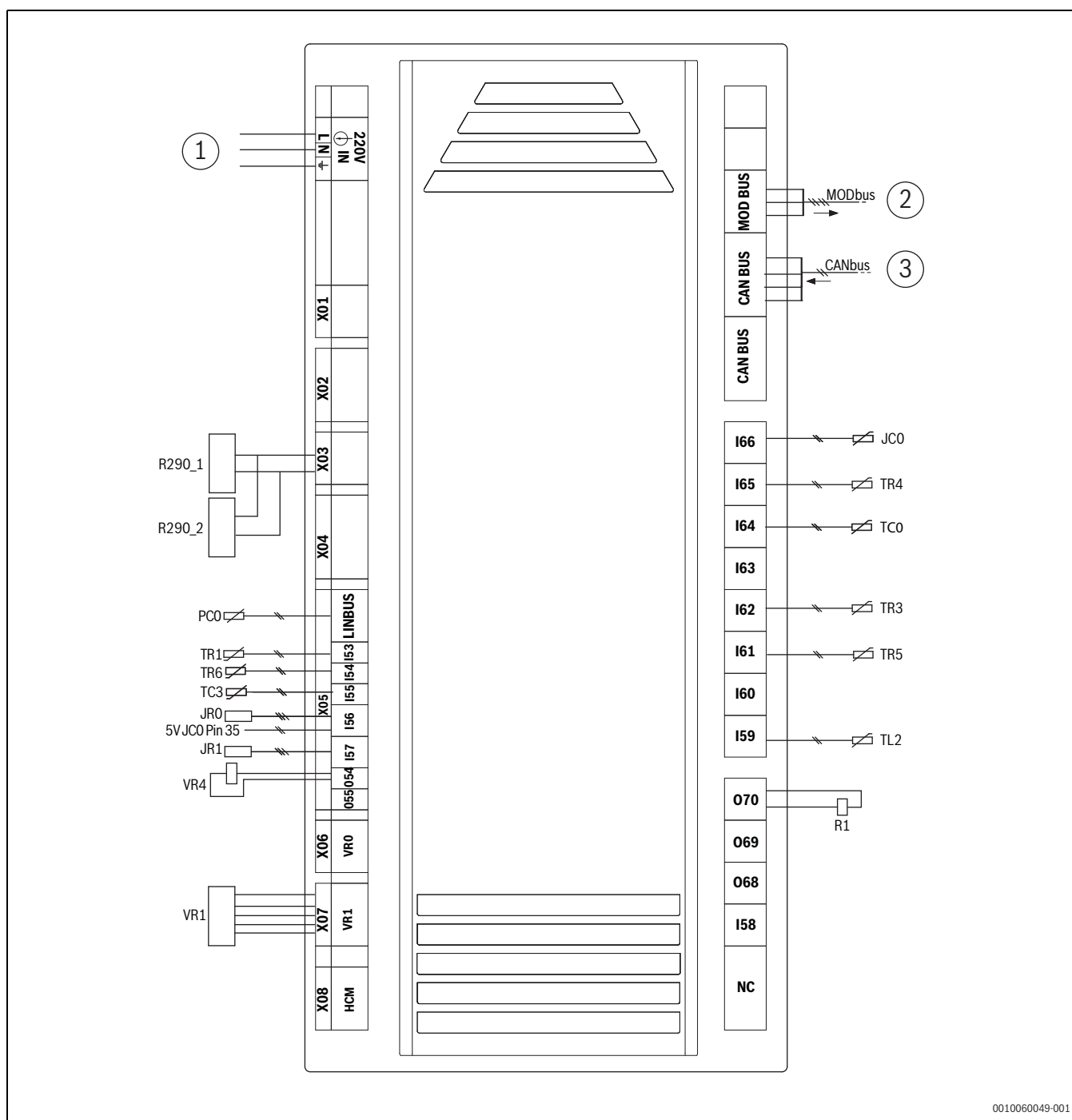
Afb. 52 Stroomkring XCU-SRH (XCU-HP) met circulatiepomp (hybride)
