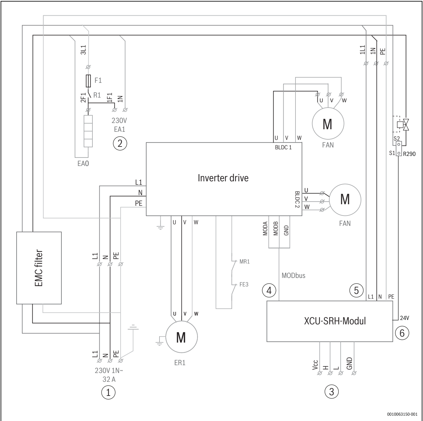
Fig. 112 Schema elettrico monofase (considera la preinstallazione della resistenza della bacinella di raccolta condensa)
