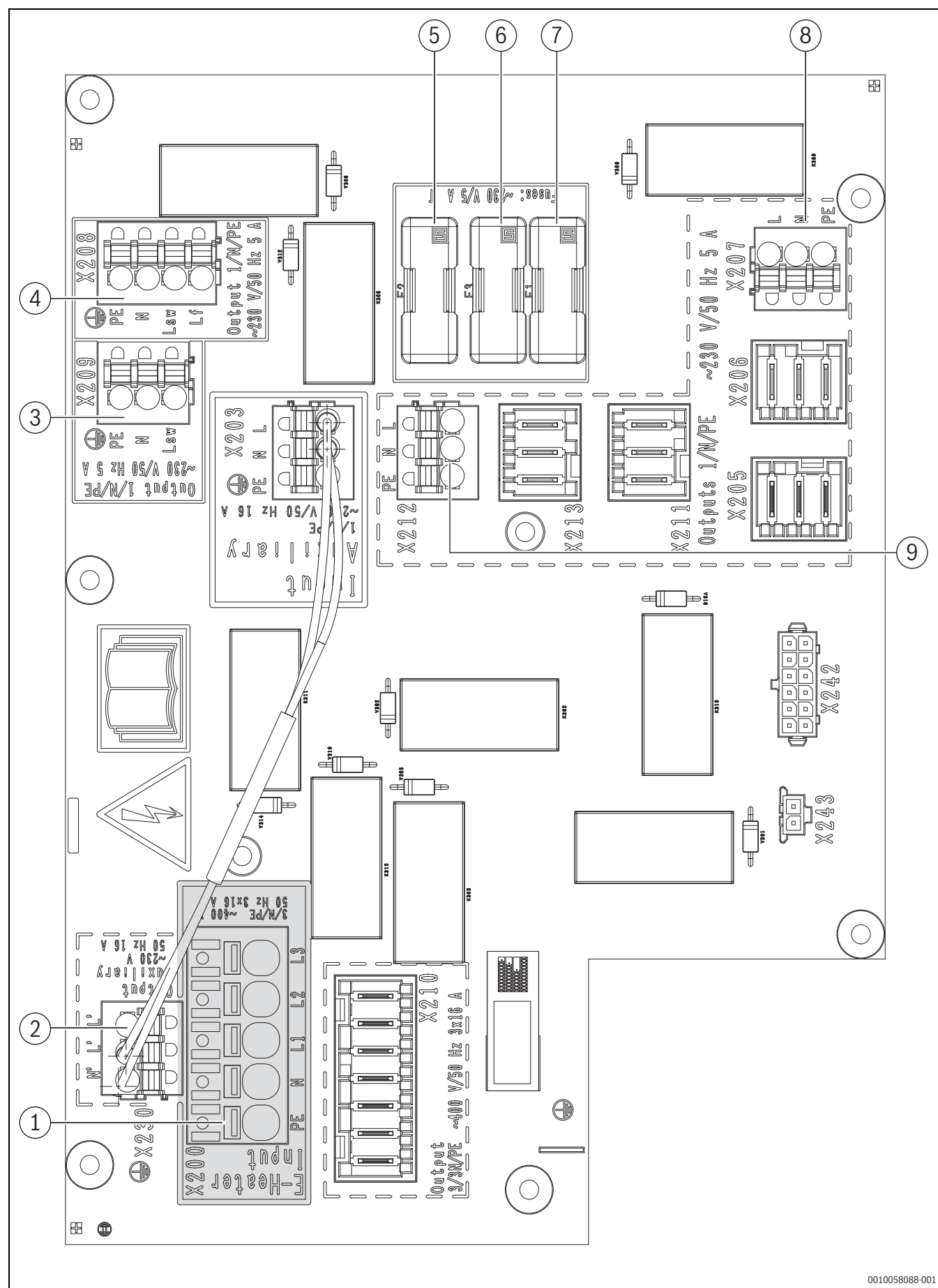
Afb. 117 Aansluitingen op de XCU-SEH
