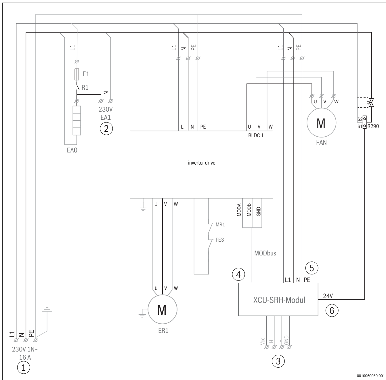
Rys. 161 Schemat elektryczny SC bez pompy cyrkulacyjnej (system cichy) z przewodem grzewczym podłączonym fabrycznie
