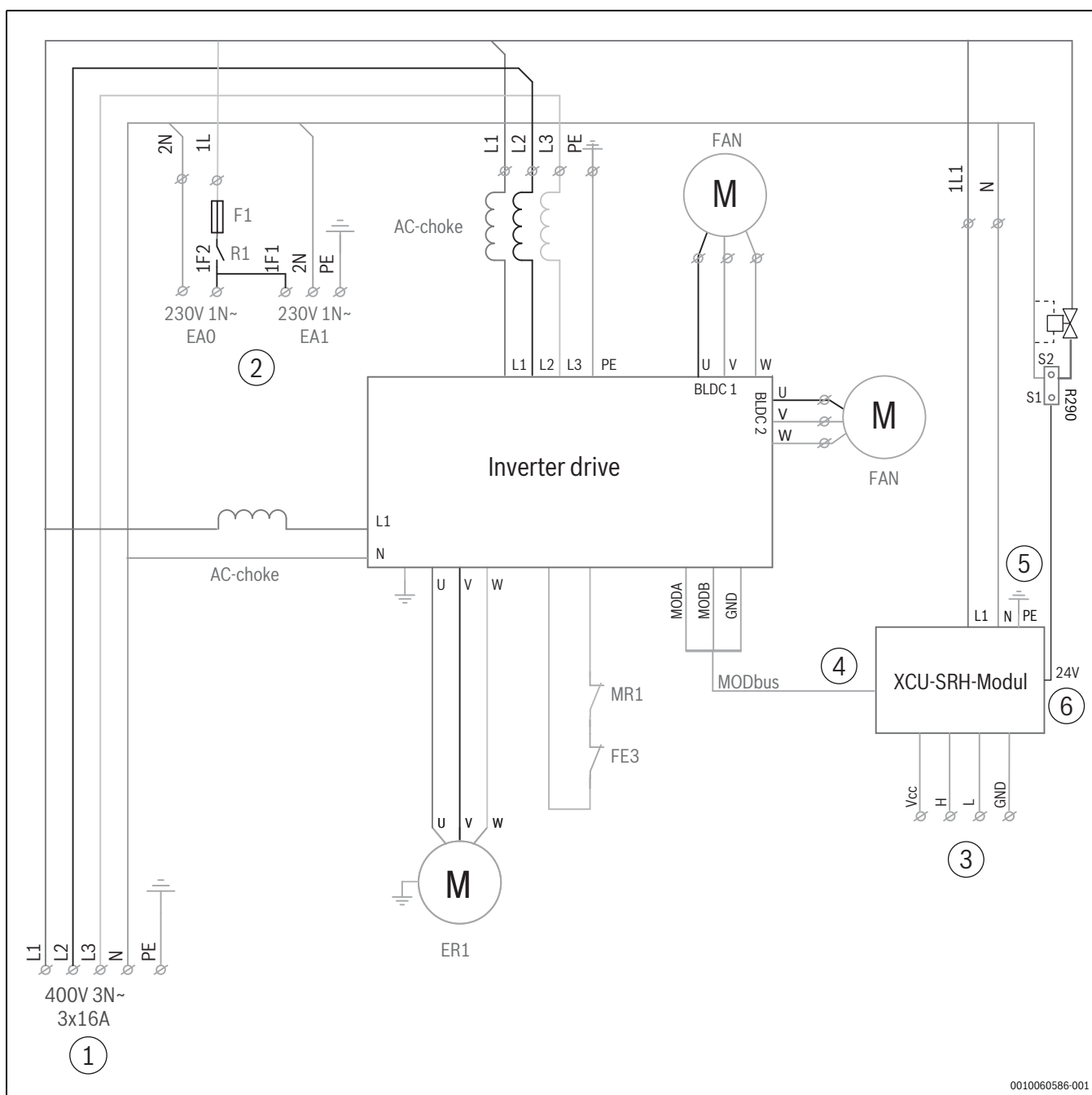
Afb. 55 Stroomkring 3fase (houdt geen rekening met pre-installatie van de lekbakverwarming)
