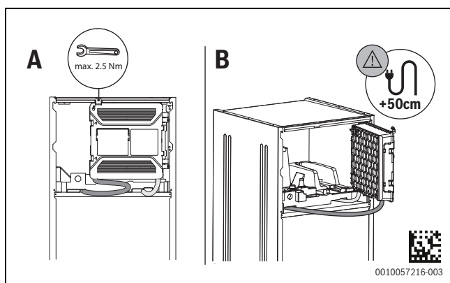
Rys. 157 Wejścia kablowe do jednostki wewnętrznej
