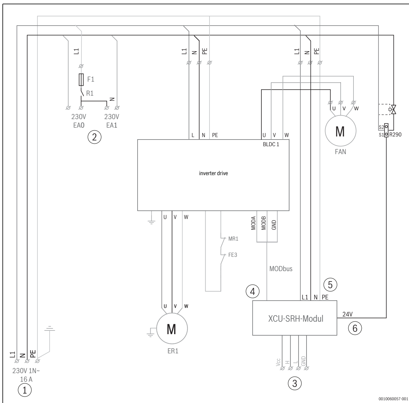
Rys. 162 Schemat elektryczny bez pompy cyrkulacyjnej (system cichy) i bez przewodu grzewczego podłączonego fabrycznie
