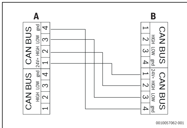
Afb. 121 CAN-BUS buitenunit - binnenunit
