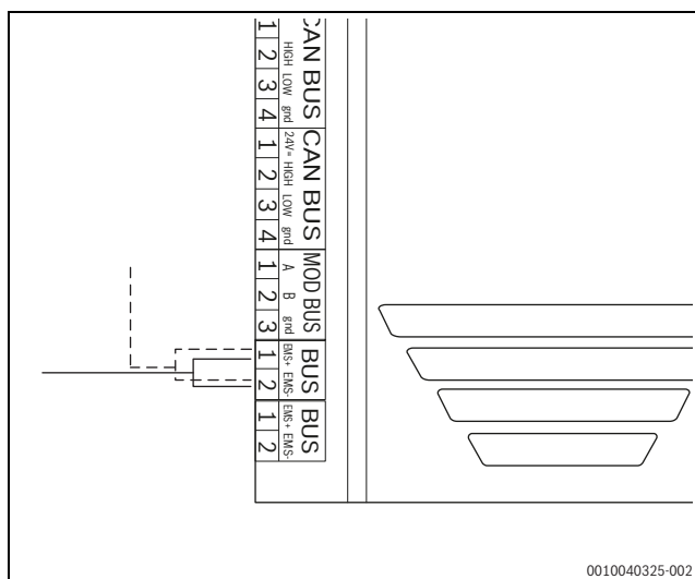
Fig. 67 Raccordement de EMS
