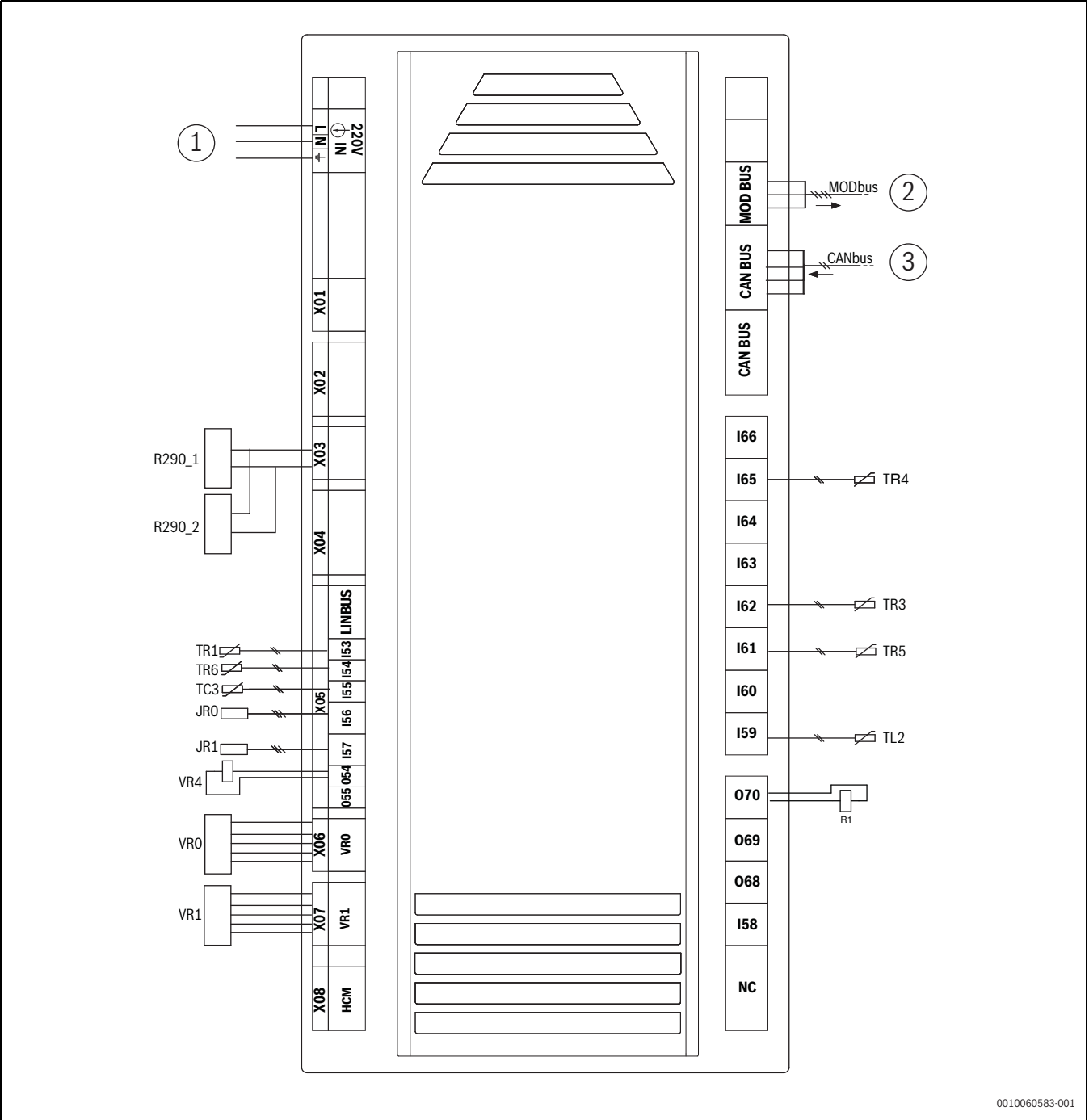
Bild 29 Schaltplan XCU-SRH (XCU-HP)
