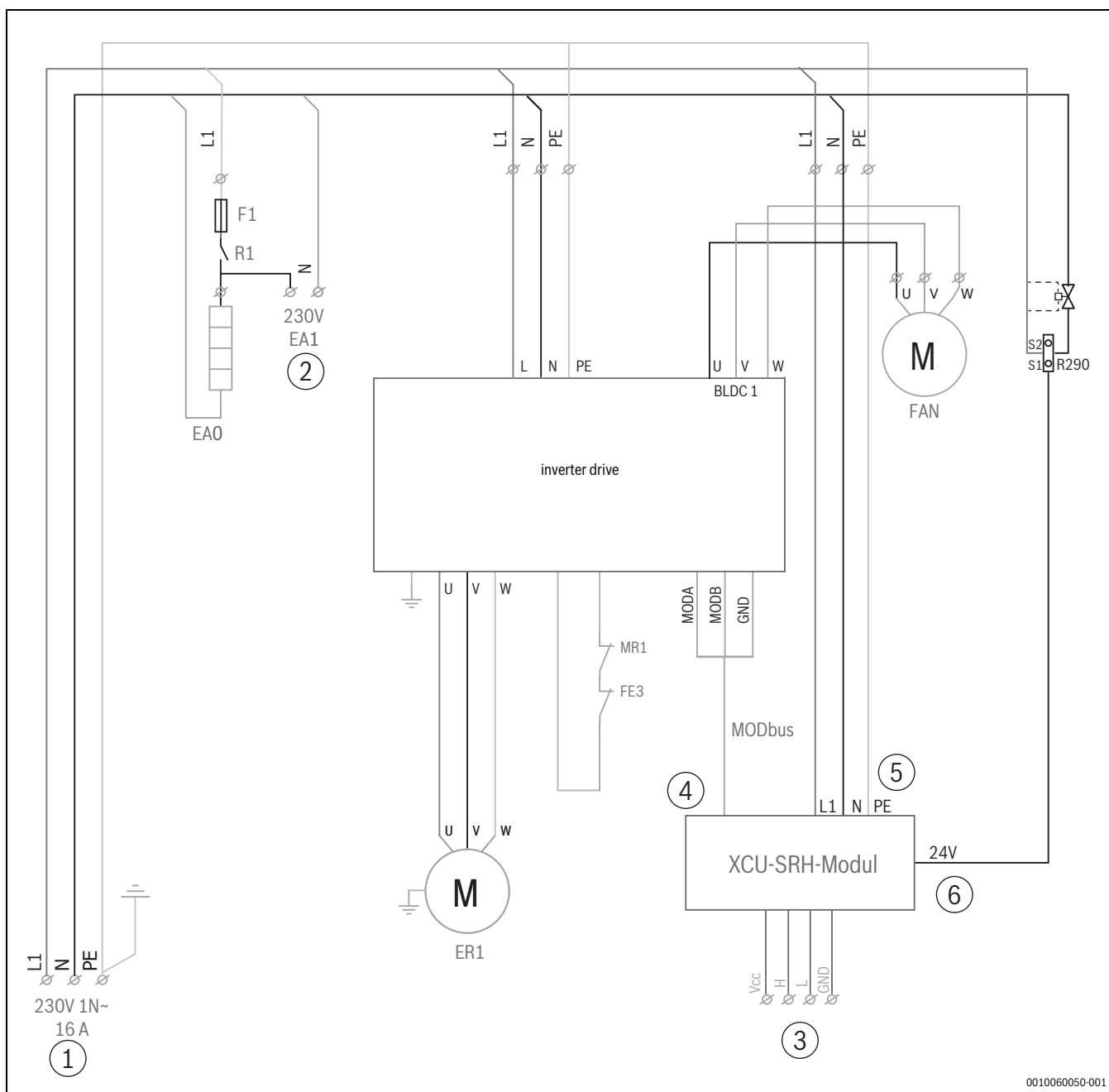
Afb. 47 Stroomkring SC zonder circulatiepomp (stil) met verwarmingskabel aangesloten in de fabriek
