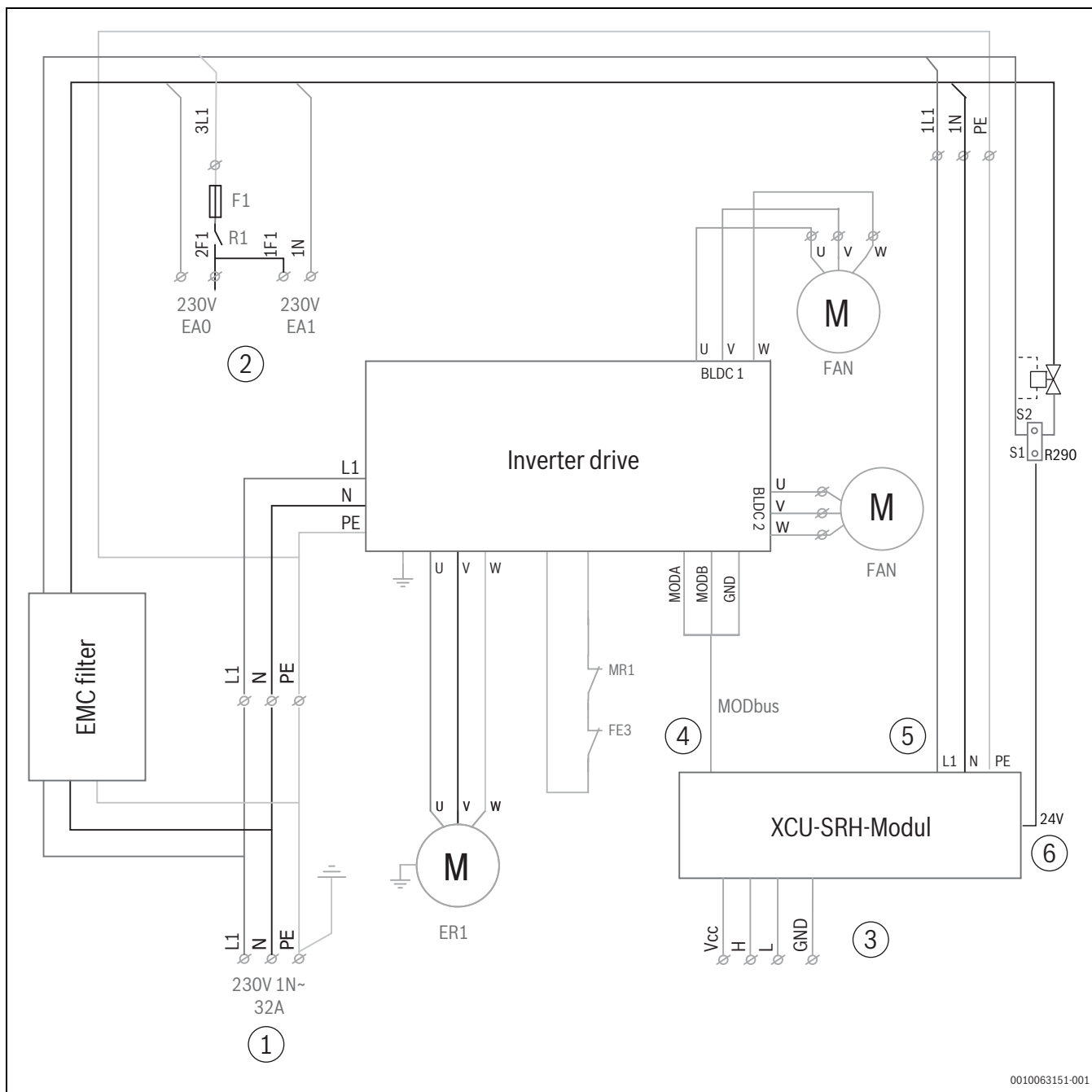
Rys. 167 Schemat elektryczny 1-fazowy (nie uwzględnia wstępnej instalacji podgrzewacza tacy skroplin)
