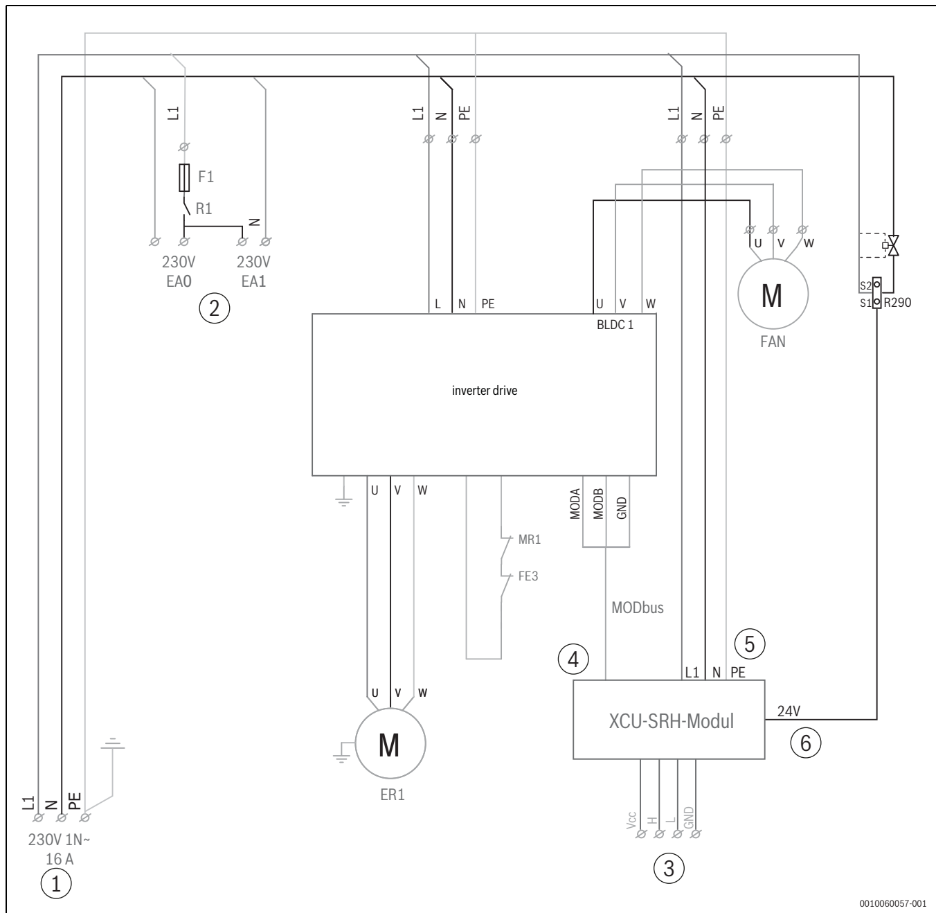
Afb. 48 Stroomkring zonder circulatiepomp (stil) met verwarmingskabel aangesloten in de fabriek
