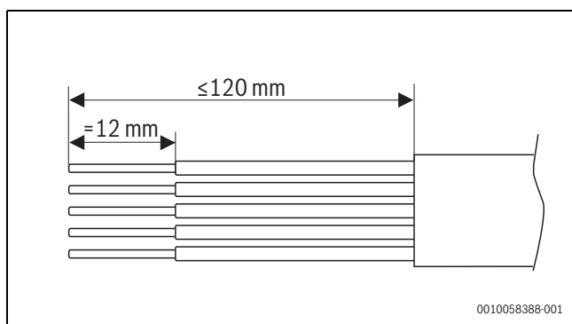
Afb. 116 Aders strippen aansluiting voedingsspanning
