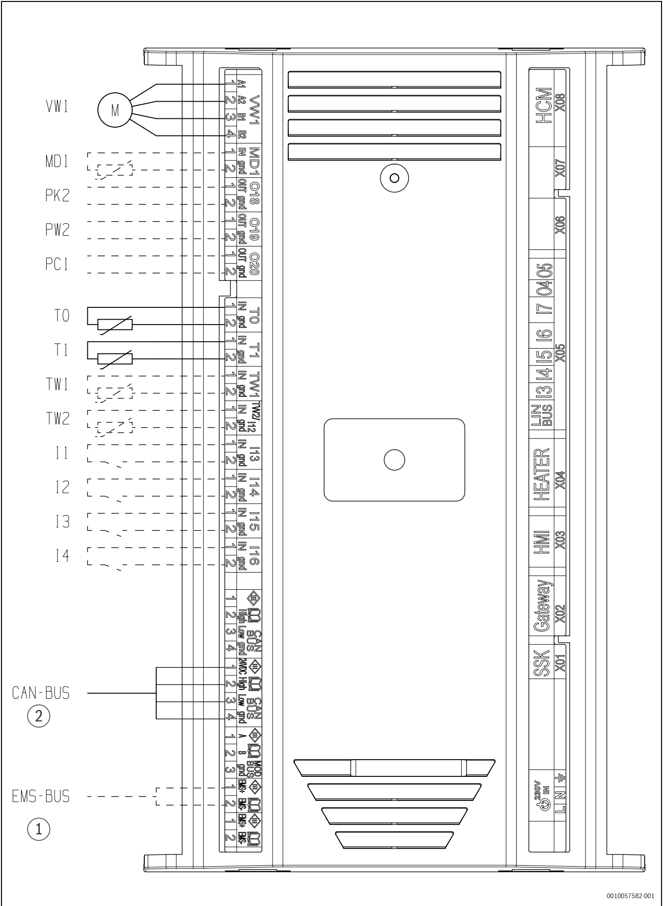
Afb. 127 Aansluitingen XCU-THH
