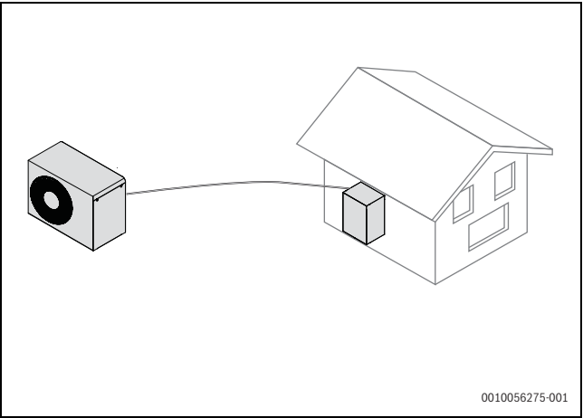
Afb. 36 CAN-BUS-aansluiting tussen binneneenheid en buiteneenheid
