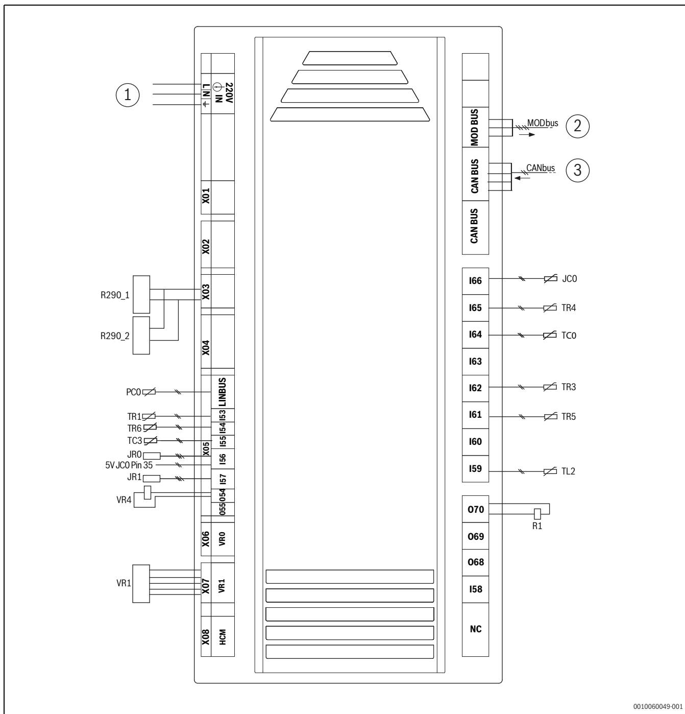
Afb. 138 Stroomkring XCU-SRH (XCU-HP) met circulatiepomp (hybride)
