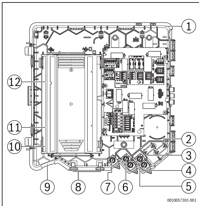
Afb. 126 Kabelinstallatie in de aansluitdoos (voedingsspanning, accessoires en laagspanning)
