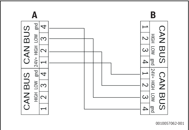
Afb. 35 CAN-BUS buiteneenheid - binneneenheid
