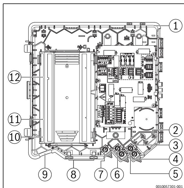
Afb. 44 Kabeldoorvoering in de aansluitdoos (voedingspanning, accessoires en laagspanning)
