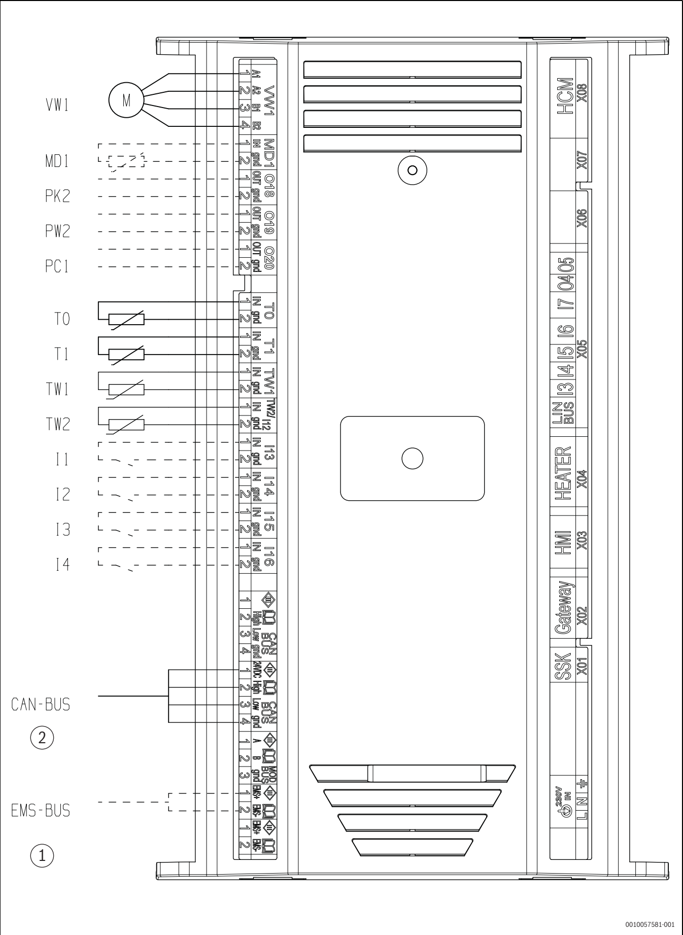
Bild 17 Anschlüsse XCU-THH
