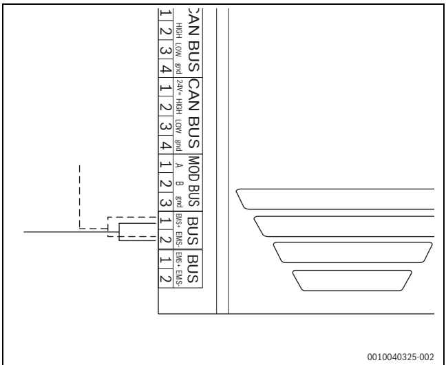
Fig. 96 Collegamento EMS
