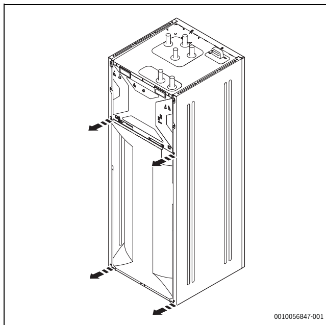
Afb. 9 Schroeven verwijderen voor demonteren zijpanelen
