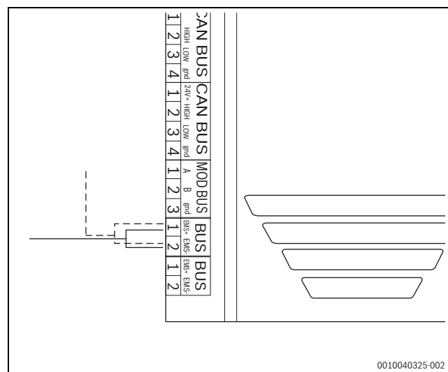
Afb. 33 EMS-verbinding
