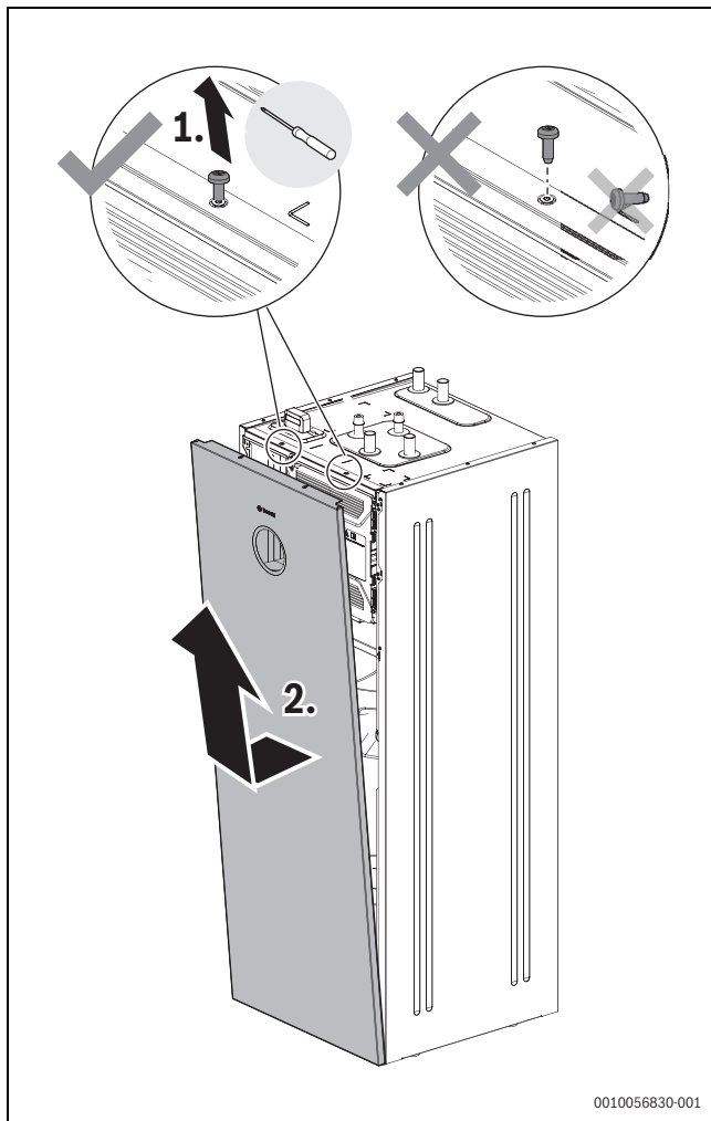
Afb. 12 Verwijder het frontmantel
