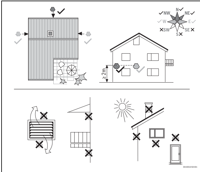
Afb. 34 Positie van de buitentemperatuursensor
