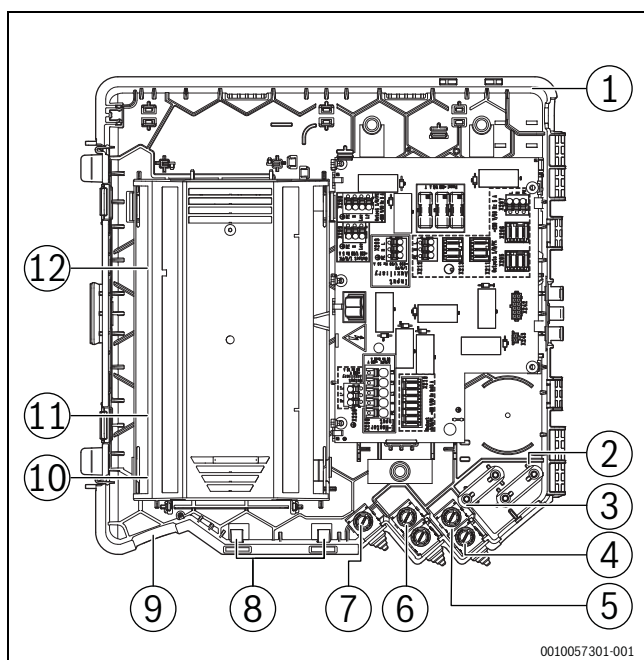
Afb. 23 Kabelinstallatie in de aansluitdoos (voedingsspanning, accessoires en laagspanning)
