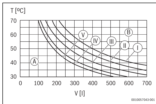
Afb. 11 Curven voor expansievat (12 l)
