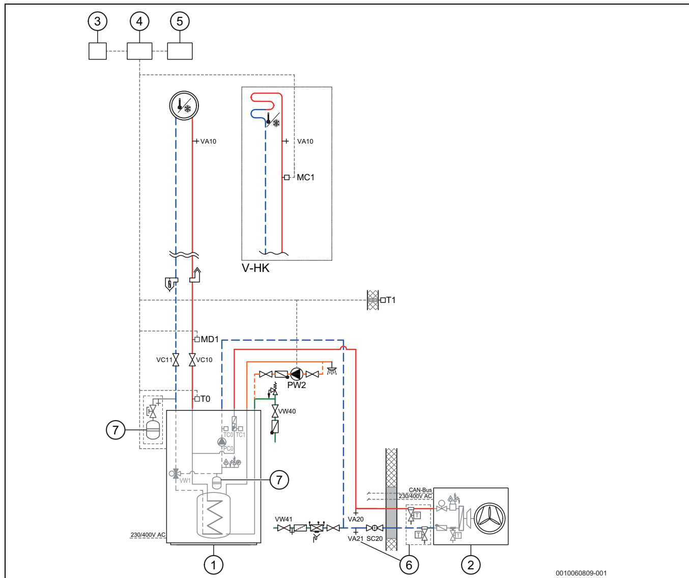
Afb. 40 Binnenunit Tower, warmtepomp (ODU) zonder ongemengde groep
