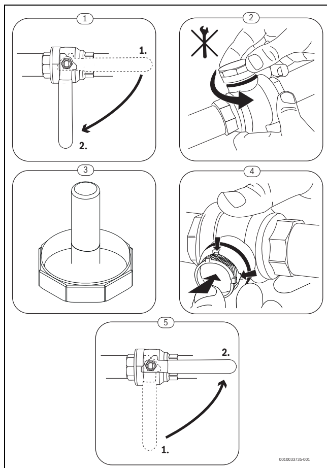
Afb. 39 Deeltjesfilter reinigen
