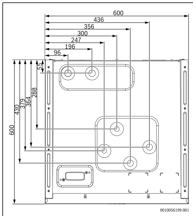
Afb. 4 Afmetingen, aansluitingen, bovenaanzicht
