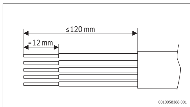
Afb. 20 Aders strippen aansluiting voedingsspanning
