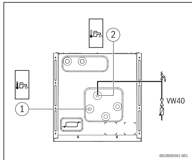
Afb. 18 Aansluitingen binnenunit drinkwater
