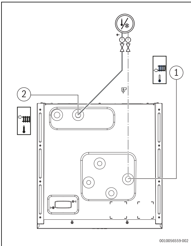
Afb. 16 Aansluitingen binnenunit op de cv-installatie
