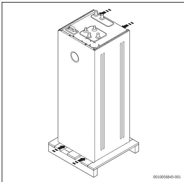
Afb. 7 Draaggrepen
