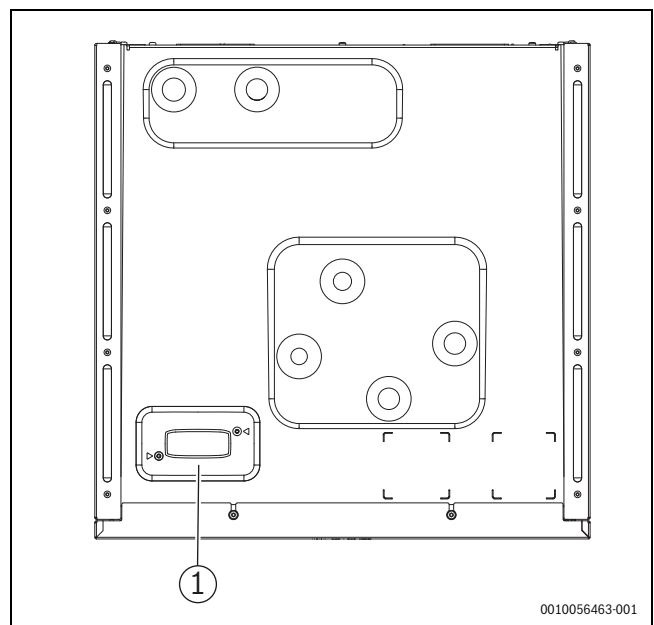
Afb. 13 Connect-Key plaatsing
