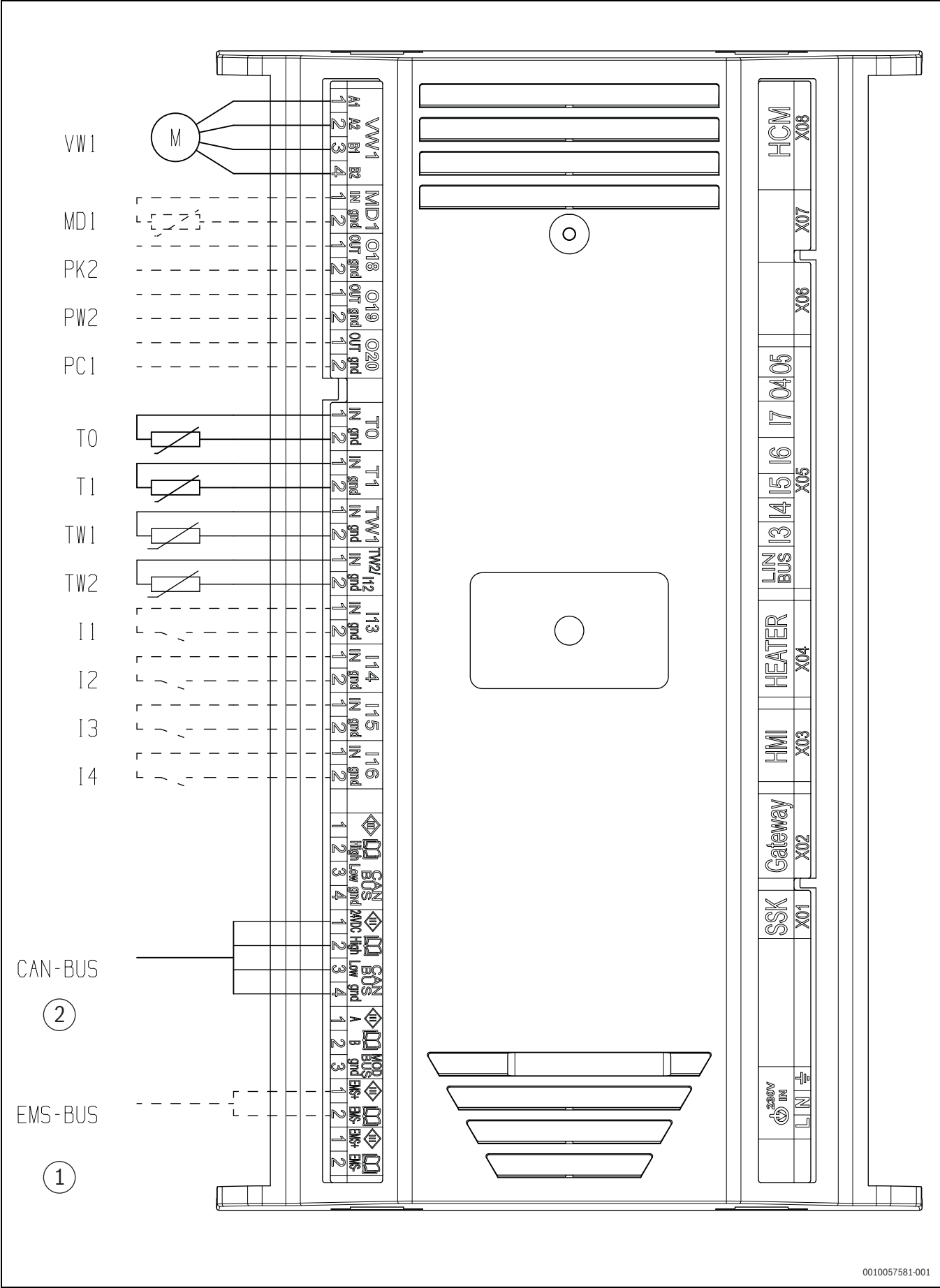
Afb. 29 Aansluitingen XCU-THH
