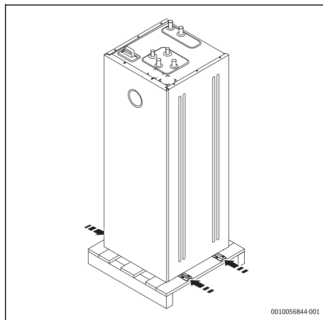
Afb. 6 Verwijder de bouten en de beugels
