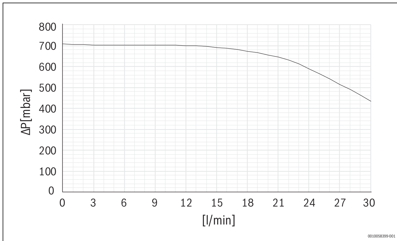
Afb. 41 Vermogenskaart voor PC0
