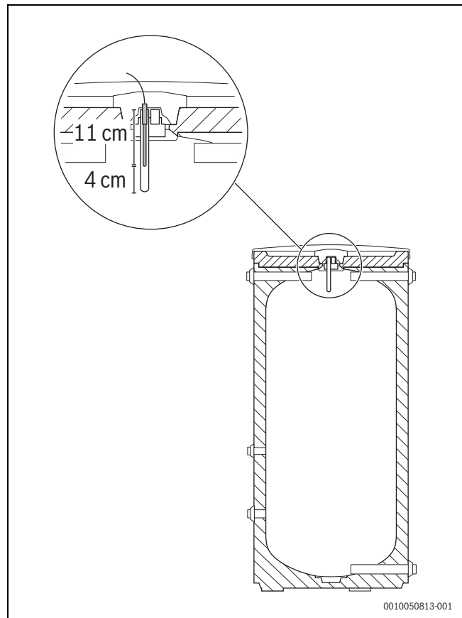
Afb. 35 Positioneren aanvoertemperatuursensor T0
