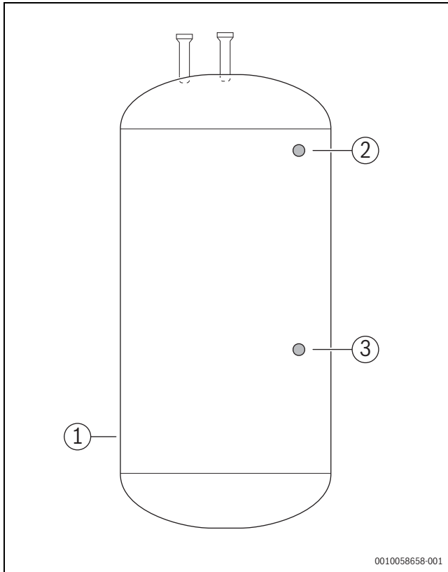
Afb. 38 Warmwatertemperatuursensoren
