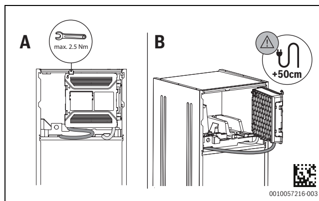
Afb. 22 Kabeldoorvoeren naar de binnenunit
