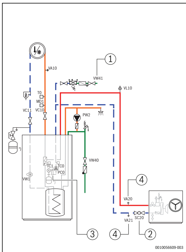
Afb. 19 Binnenunit, warmtepomp, boiler en een cv-installatie
