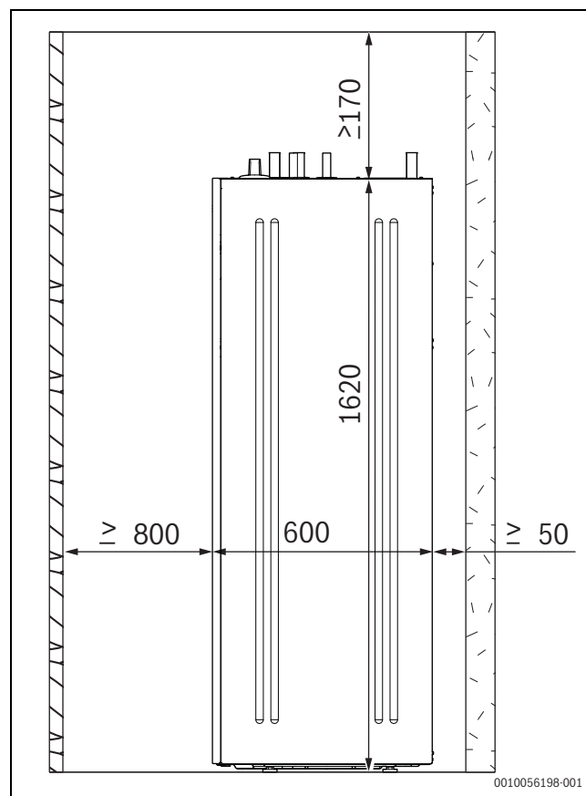
Afb. 2 Minimale afstand (mm)
