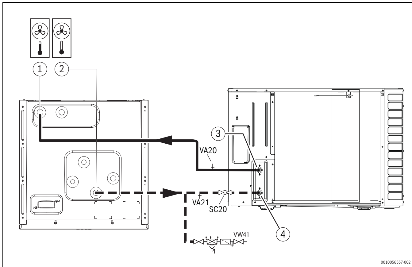
Afb. 15 Aansluiten van de binnenunit op de buitenunit
