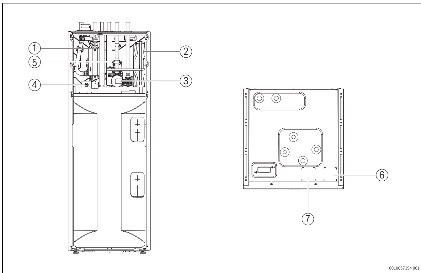
Afb. 5 Productoverzicht, voor- en bovenaanzicht
