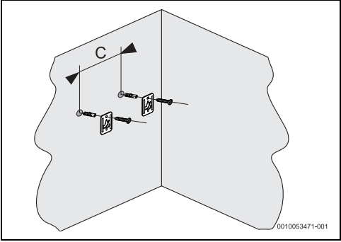
Bild 10 Montageplatten
