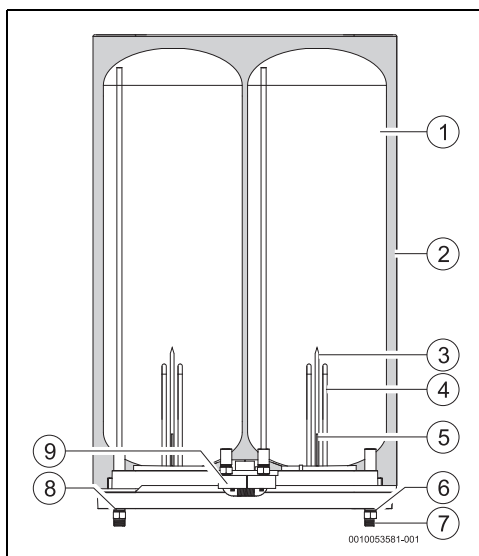
Fig. 4 Componenti dell'apparecchio
