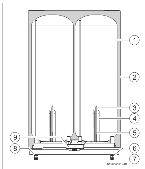
Afb. 4 Toestelcomponenten
