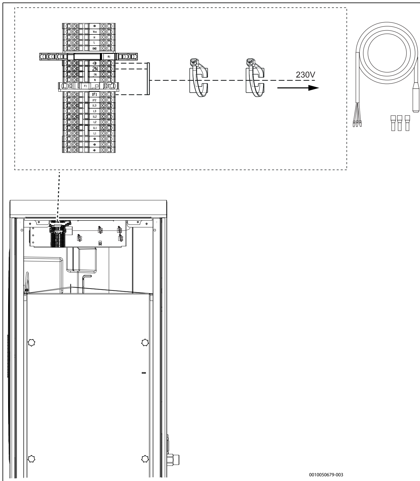
Afb. 44 Aansluiting verwarmingskabel (accessoire)
