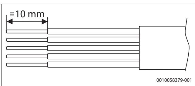
Afb. 42 Strippen van de aders voor de voedingsaansluiting
