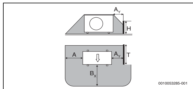
Afb. 9 Veiligheidszone met barrière rechts van een vloerstaande warmtepomp
