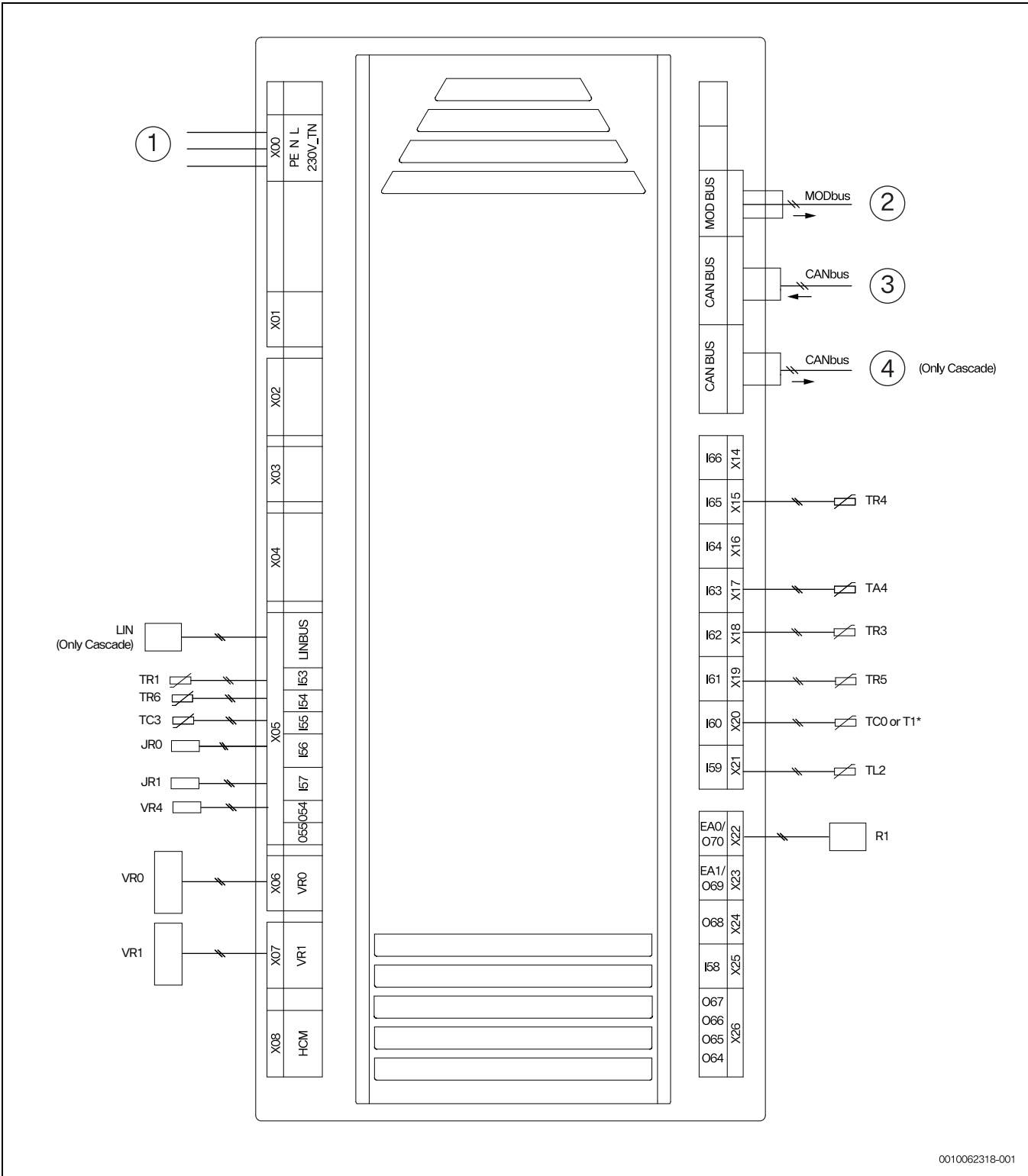
Afb. 53 Elektrisch schema XCU-SRH (XCU-HP)
