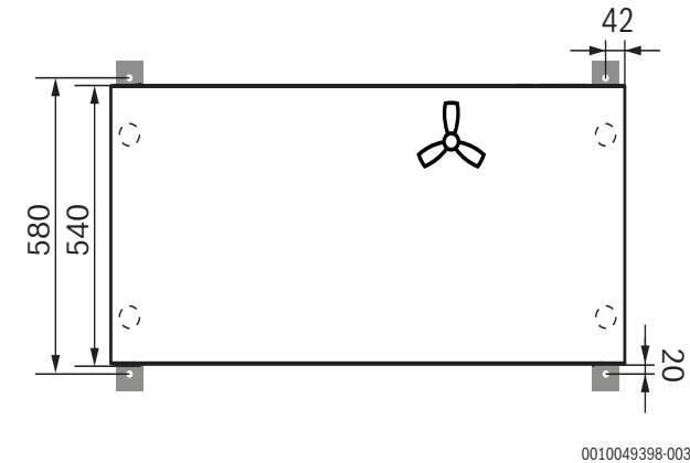
Afb. 5 Afmetingen warmtepomp, bovenkant
