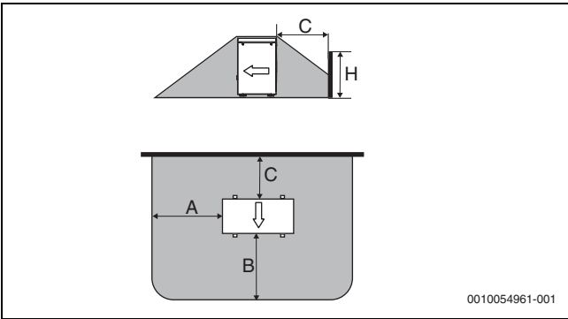
Afb. 13 Veiligheidszone met barrière achter een vloerstaande warmtepomp
