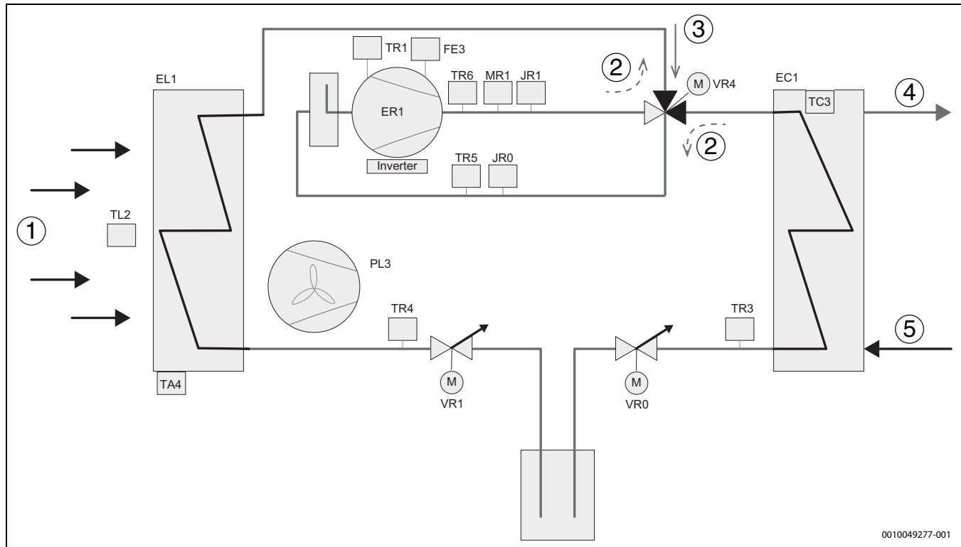
Afb. 51 Koelmiddelcircuit
