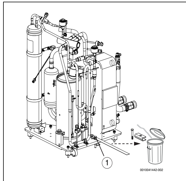
Afb. 38 Transportbeveiliging
