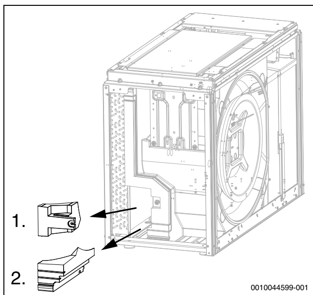
Afb. 46 EPP-onderdelen
