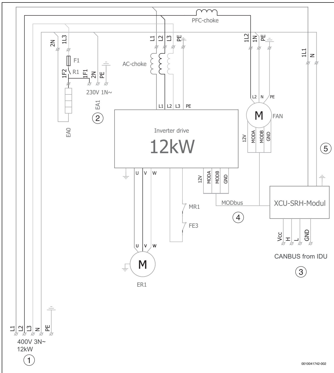
Afb. 52 Elektrisch schema
