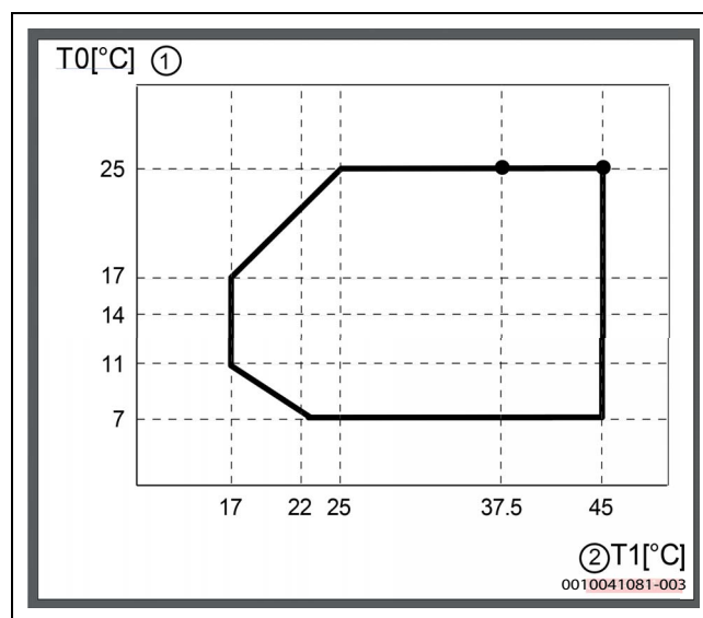
Afb. 50 Warmtepomp in koelmodus
