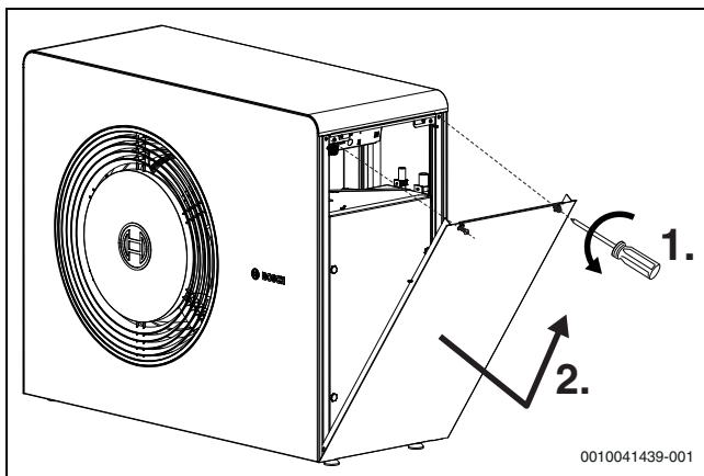
Afb. 36 Zijpaneel
