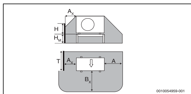
Afb. 10 Veiligheidszone met barrière links van een warmtepomp op vloerconsole
