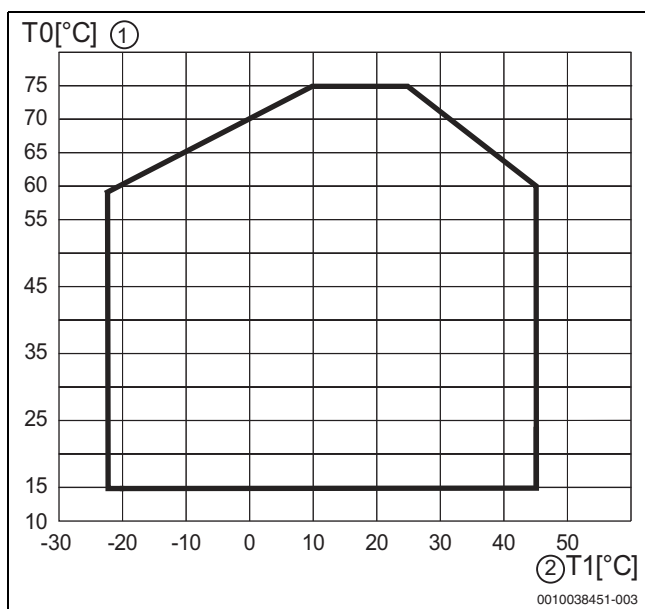
Afb. 49 Warmtepomp in verwarmingsmodus zonder boosterverwarming
