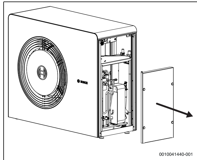
Afb. 37 Deksel koudemiddelmodule
