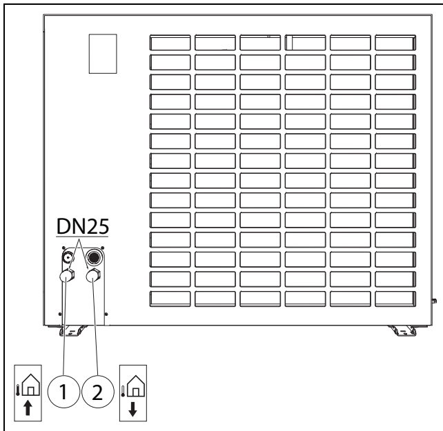
Afb. 35 Aansluitingen van de aanvoer en retour, beschrijving geldt voor alle grootten
