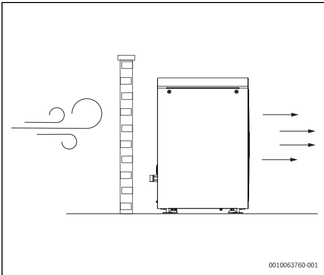
Afb. 22 Vrijstaande warmtepomp
