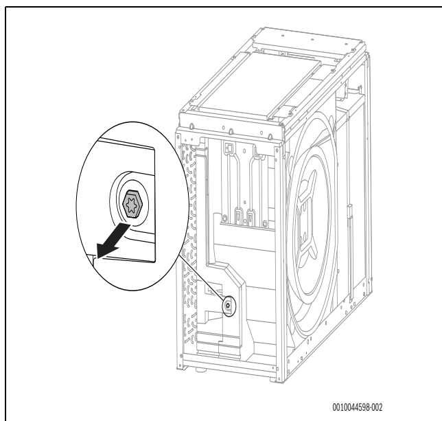
Afb. 45 Losschroeven
