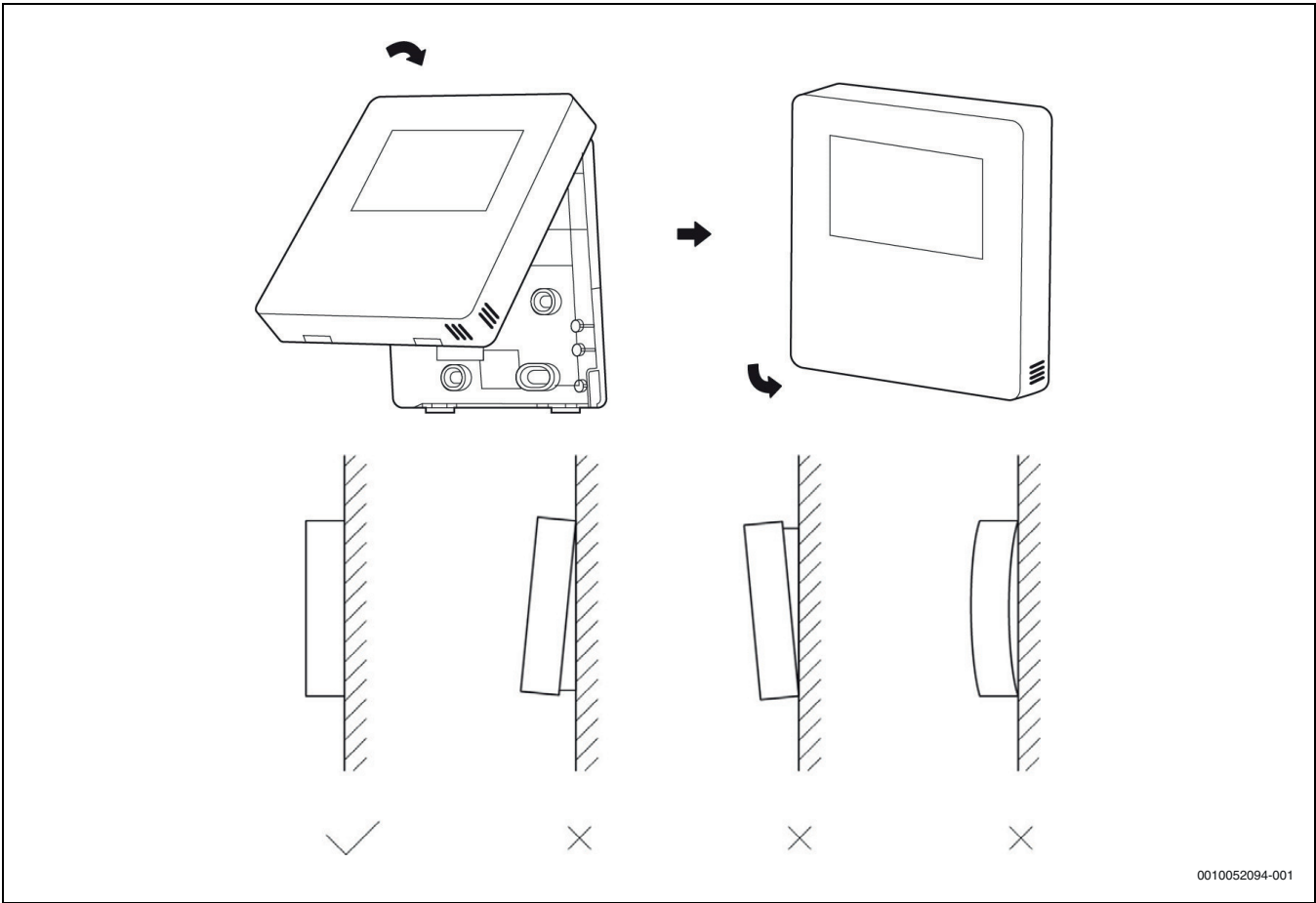
Afb. 100 De frontplaat installeren
