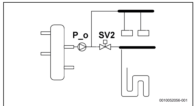
Afb. 81 Systeem met dubbele zone
