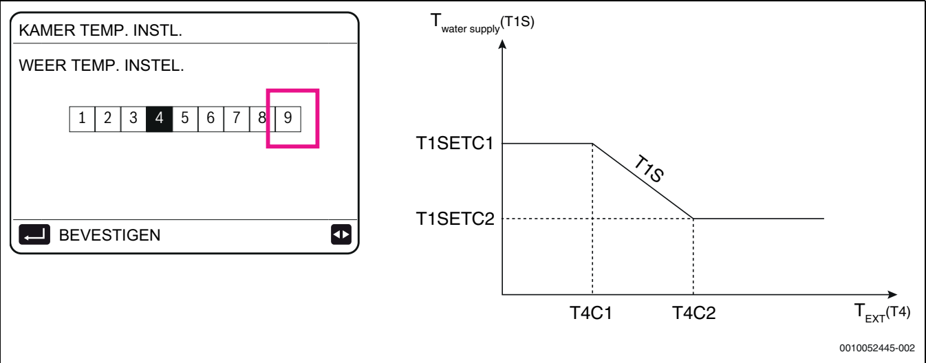
Afb. 150 Aanpasbare curve – buitenluchttemperatuur (T4C1, T4C2) en wateraanvoer (T1SETC1, T1SETC2).
