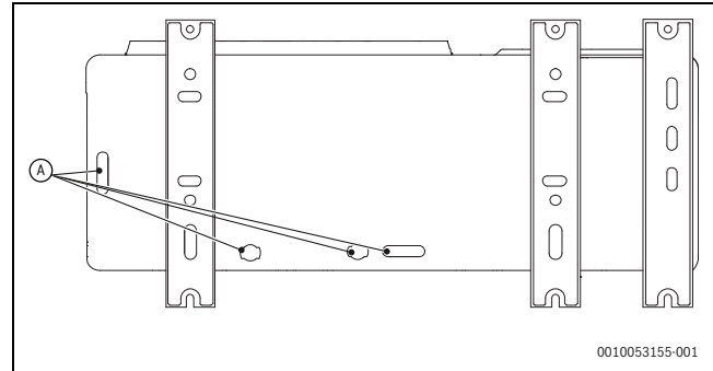
Afb. 47 Afvoeropeningen
