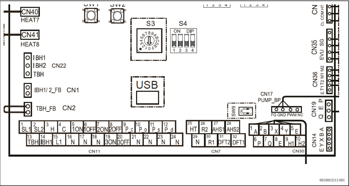
Afb. 73 Klemmenblok aansluiten
