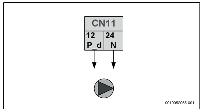
Afb. 80 Warmwaterpomp, type 2 regelsignaal
