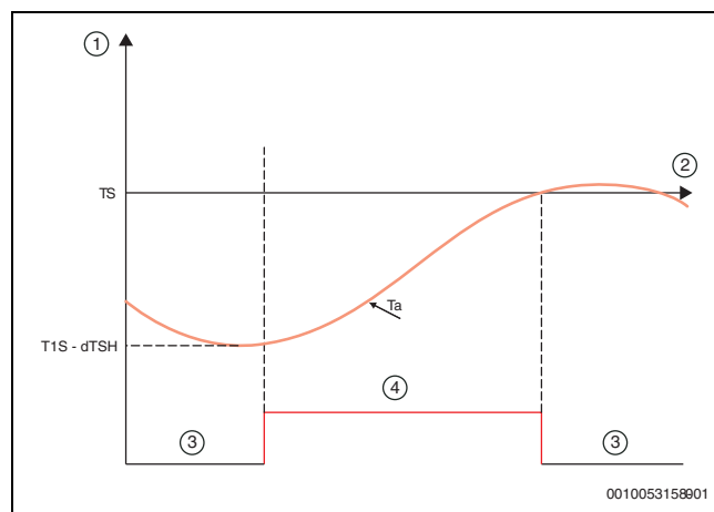
Afb. 126 Verwarmingsbedrijf - luchttemperatuur (Ta)
