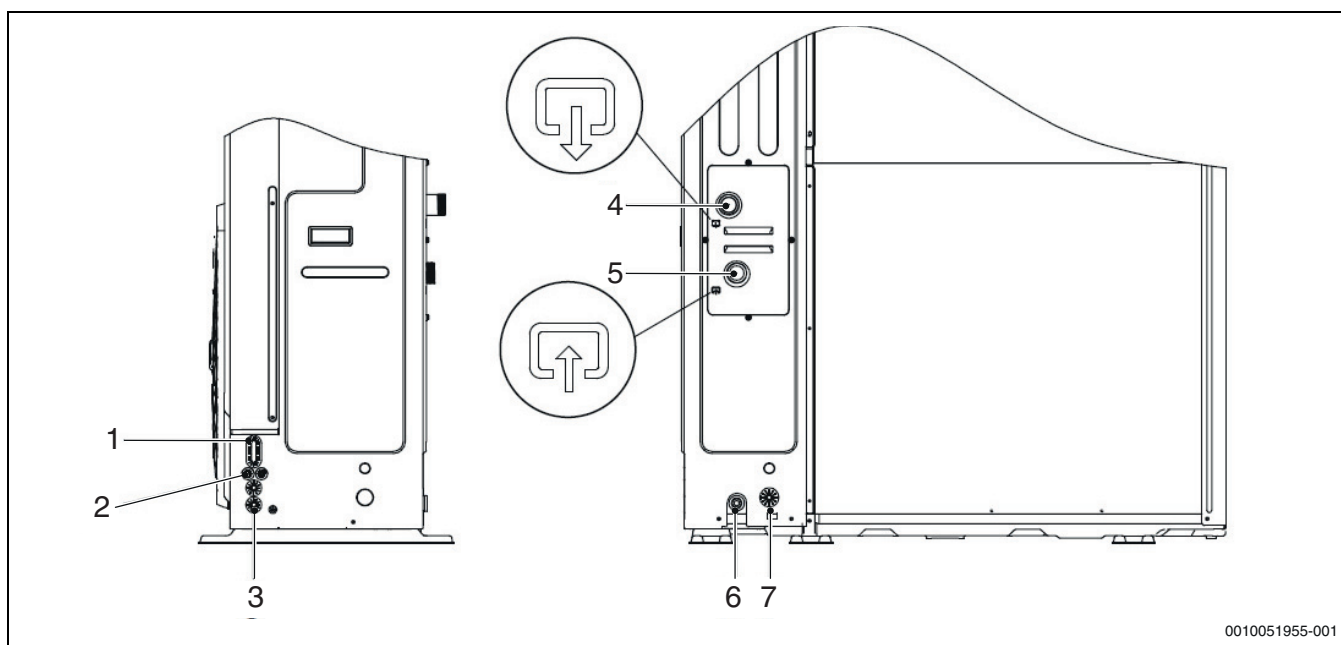
Afb. 66 Afmetingen CS2000AWF 18 R-T tot CS2000AWF 30 R-T
