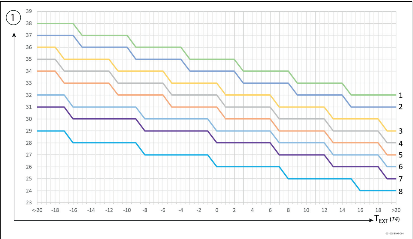
Afb. 145 Verwarmingsbedrijf op systemen met verdeling naar de stralingsbron
