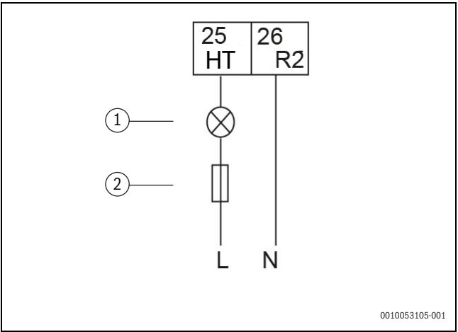
Afb. 74 TYPE 1 stuursignaal
