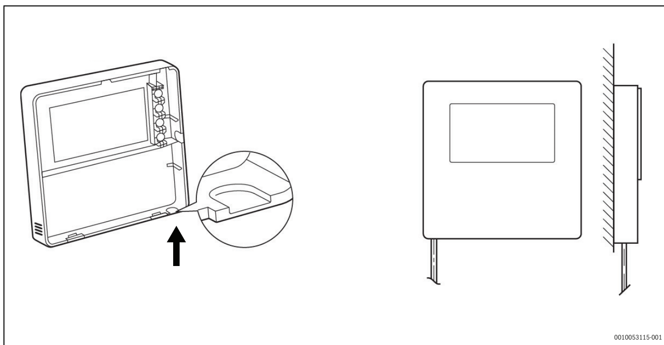
Afb. 96 Positioneren van de kabeluitlaat
