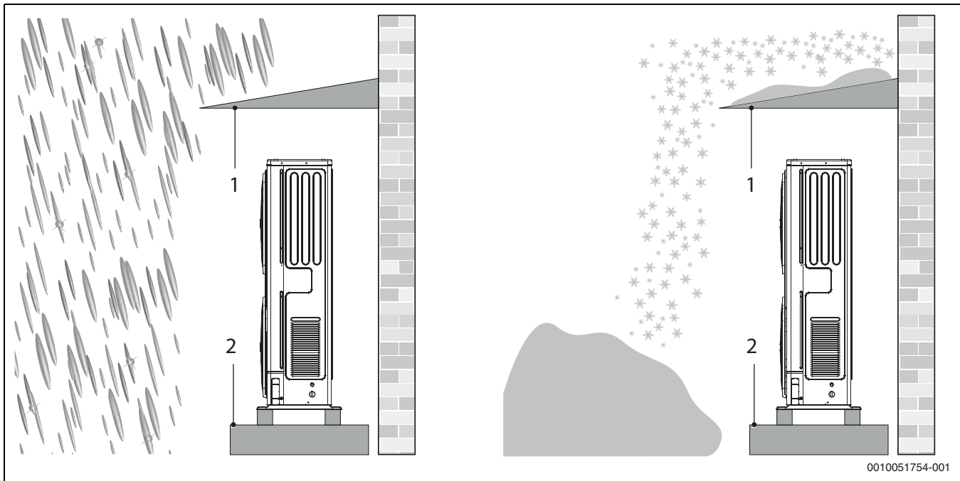
Afb. 40 Unit blootgesteld aan hevige regen of sneeuw
