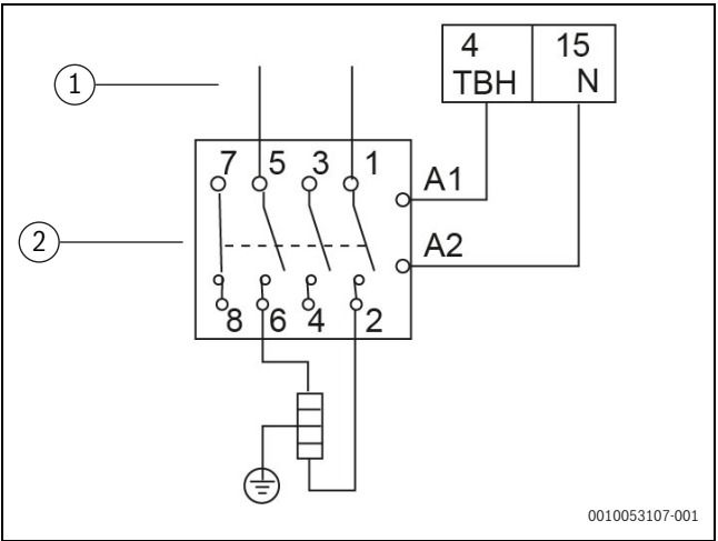
Afb. 75 TYPE 2 stuursignaal
