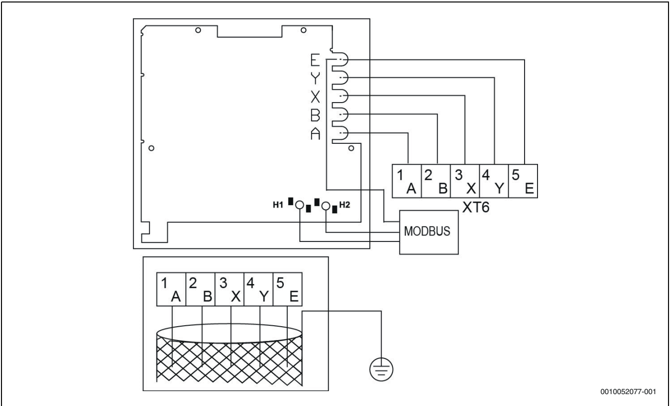
Afb. 94 Bedieningsunit
