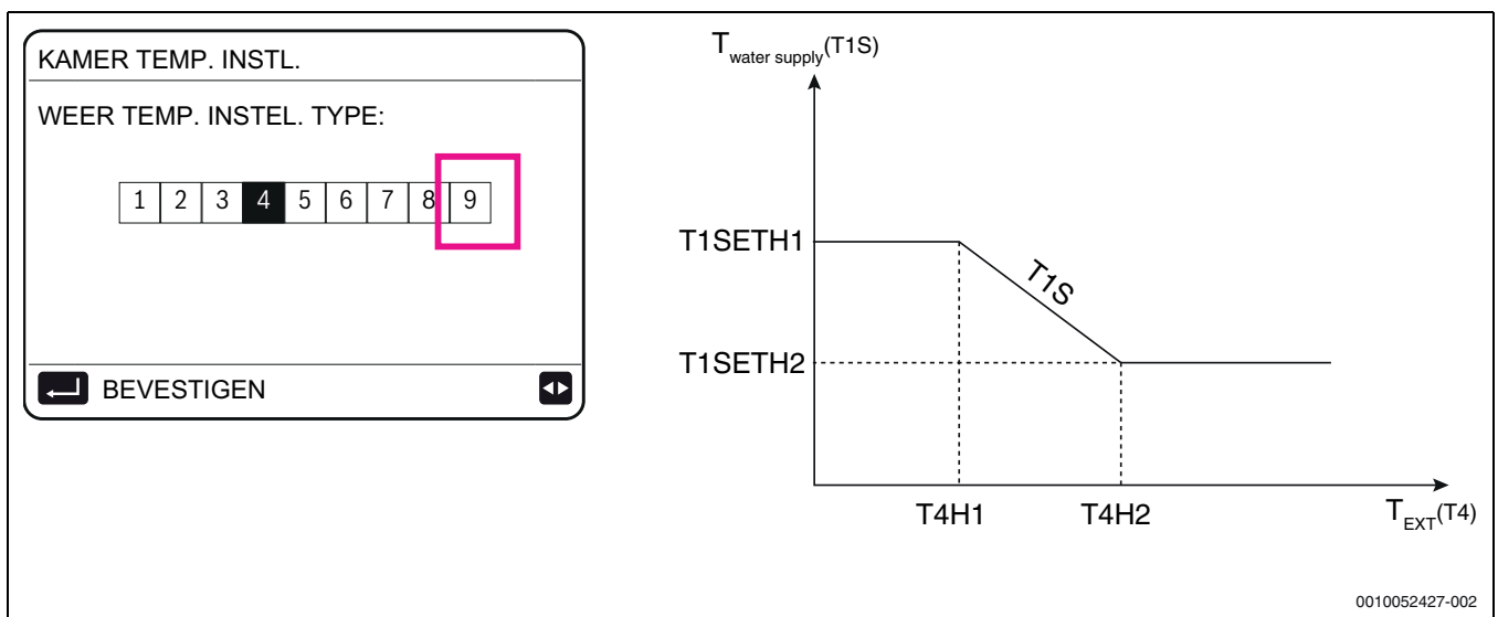
Afb. 147 Aanpasbare curve – buitenluchttemperatuur ( T_{4H1} , T_{4H2} ) en wateraanvoer ( T_{1SETH1} , T_{1SETH2} ).
