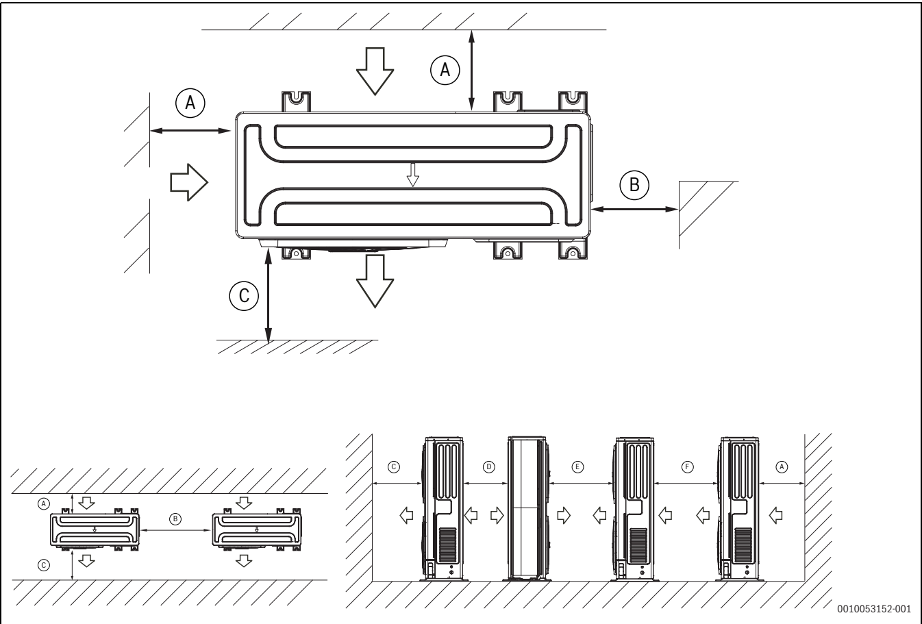
Afb. 36 Minimale afstanden
