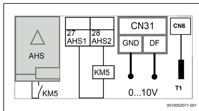
Afb. 92 Extra cv-toestel
