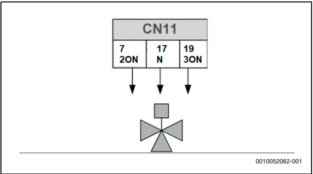
Afb. 86 3-wegventiel SV3, type 2 regelsignaal
