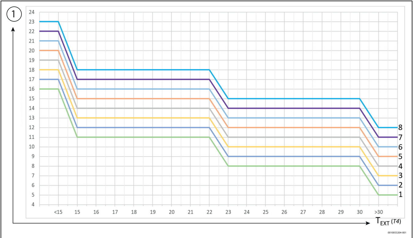
Afb. 149 Koelbedrijf op systemen met verdeling naar de eindapparaten
