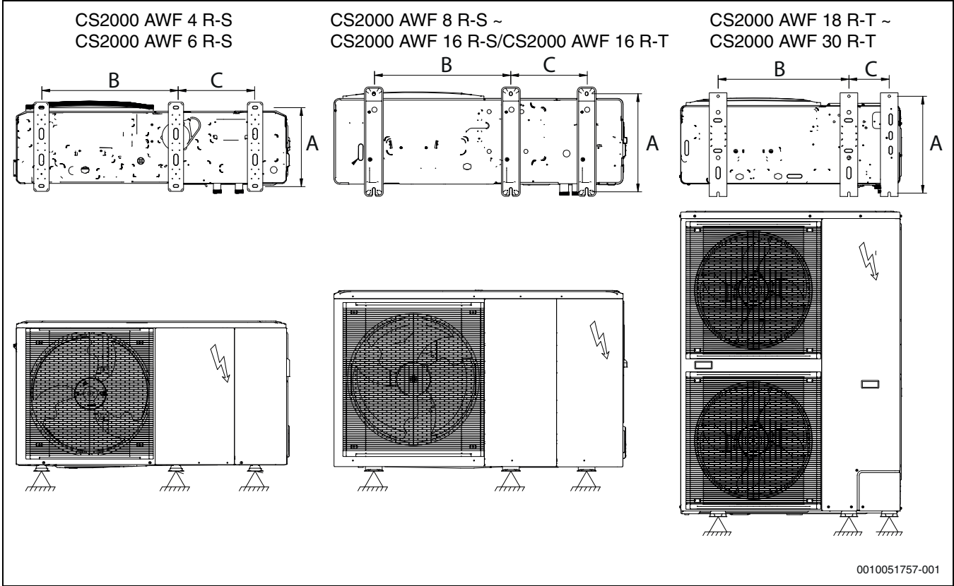
Afb. 42 Afmetingen voor bevestiging aan de grond
