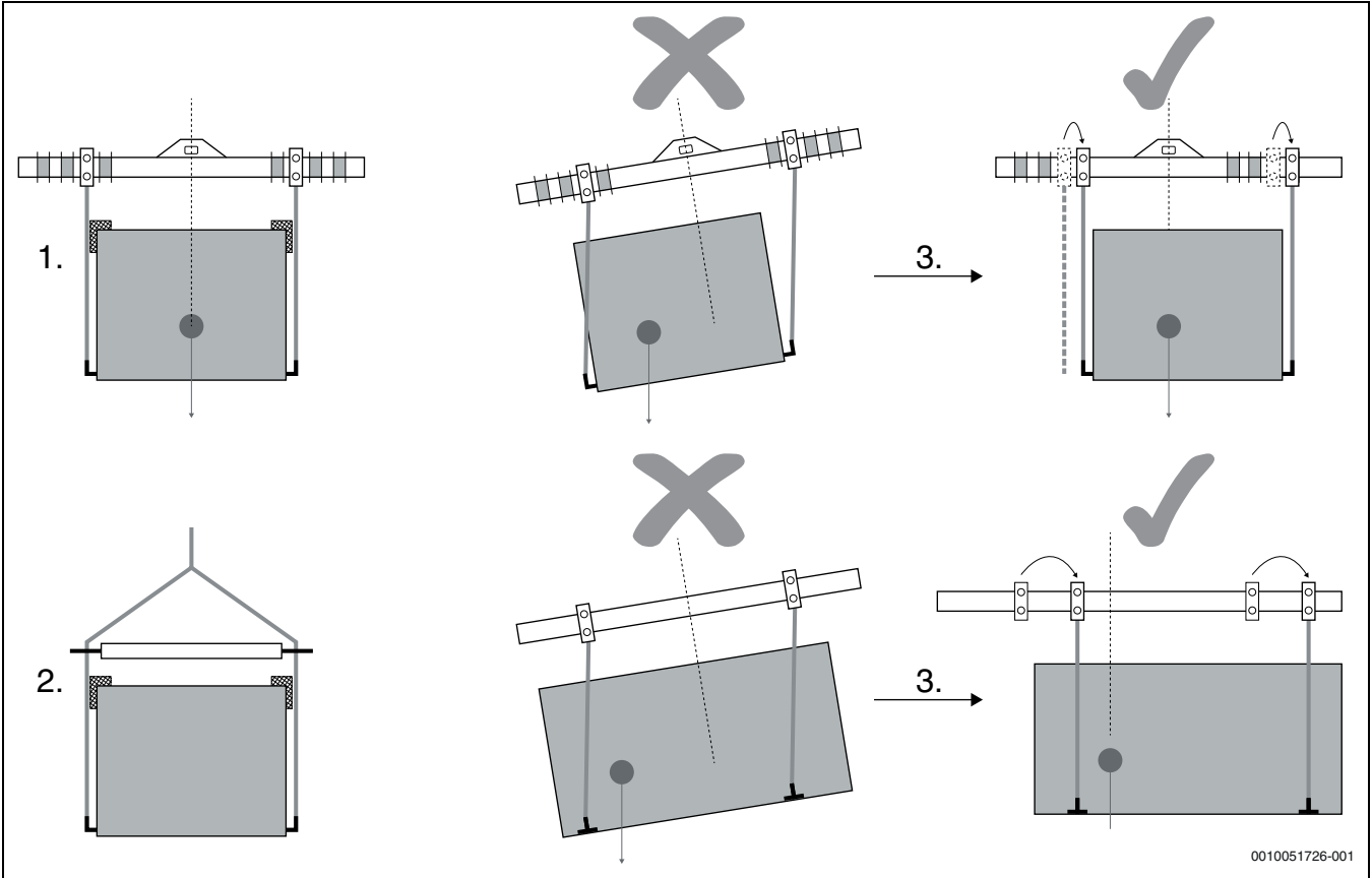
Afb. 29 Hijsen
