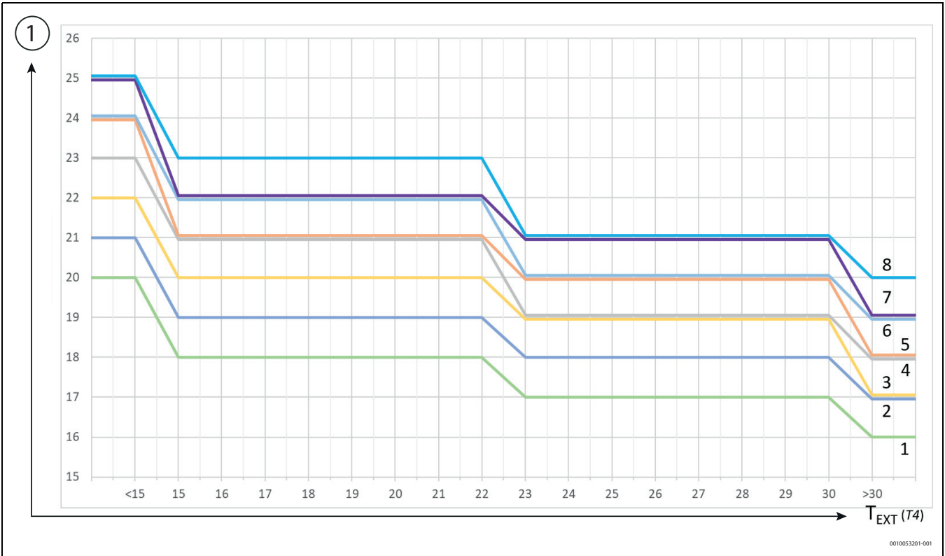
Afb. 148 Koelbedrijf op systemen met stralingsverdeling
