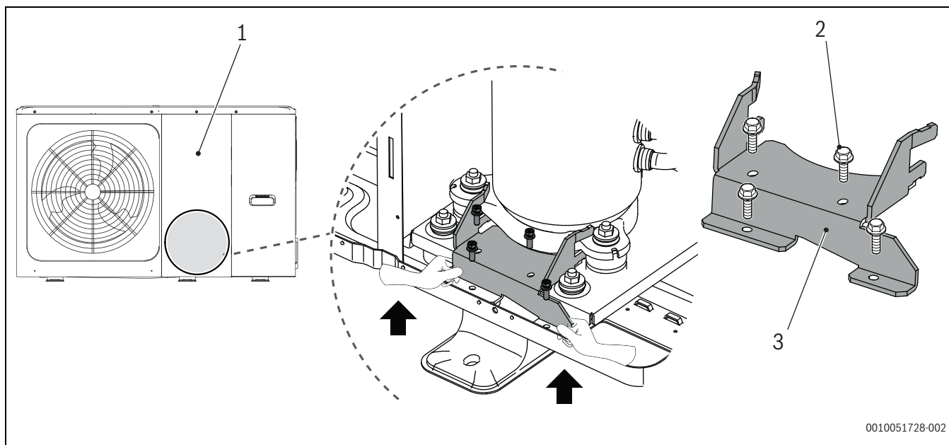
Afb. 31 De transportbeugel verwijderen
