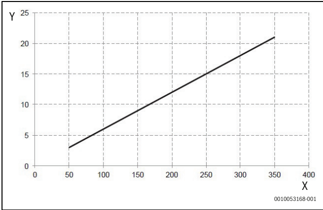
Afb. 56 Totale volume van het expansievat (afmetingen CS2000AWF 4 R-S tot CS2000AWF 16 R-S/CS2000AWF 16 R-T)
