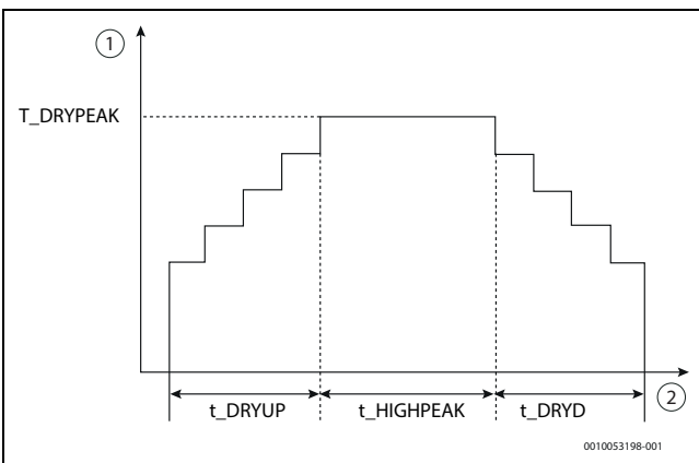
Afb. 143 Diagram droogcyclus
