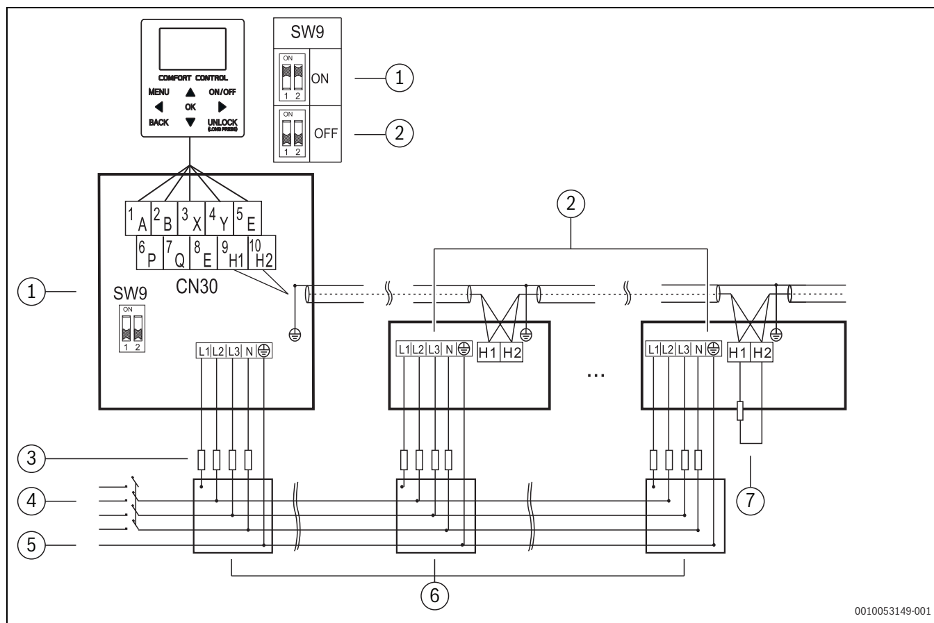
Afb. 68 Aansluitschema van het elektrische regelsysteem voor het cascadesysteem (3N ~)
