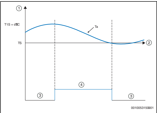
Afb. 123 Koelbedrijf - luchttemperatuur (Ta)
