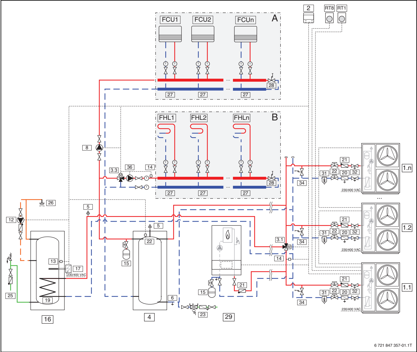
Afb. 27 Buitenunit met één of meerdere cv-groepen, externe bijverwarming, boiler en cascade (CS2000AWF 18-30 R-T)
