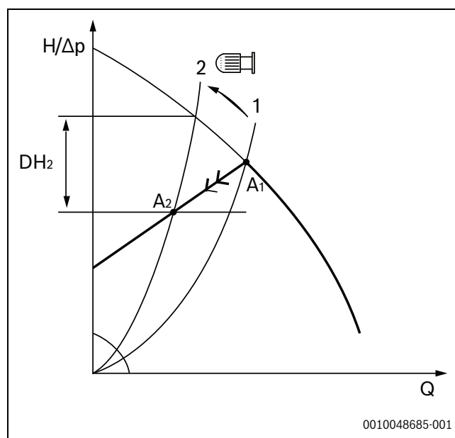
Afb. 51 Besturing met proportionele opvoer pomp. De opvoerhoogte wordt verminderd met DH2.
