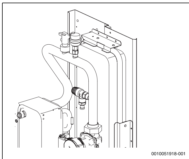
Afb. 60 Vullen / bijvullen met water
