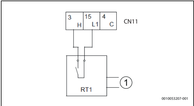
Afb. 102 Zonethermostaat – methode B
