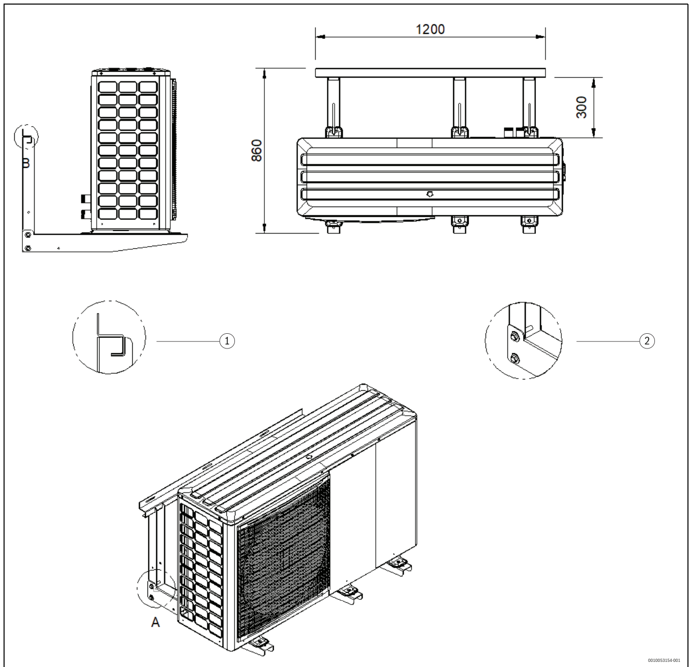
Afb. 44 Wandmontage
