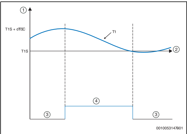
Afb. 122 Koelbedrijf - wateraanvoertemperatuur (T1)
