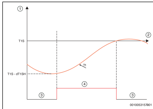
Afb. 125 Verwarmingsbedrijf - wateraanvoertemperatuur (T1)
