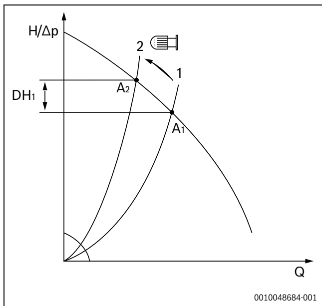
Afb. 50 Besturing met standaardpomp. Opvoerhoogte neemt toe met DH1.
