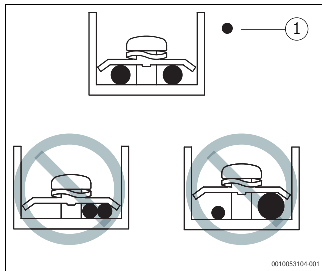
Afb. 70 Gevaar voor oververhitting door losse bedrading
