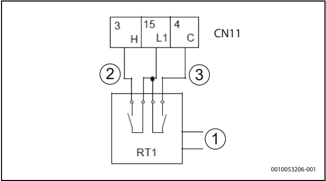
Afb. 101 Zonethermostaat – methode A
