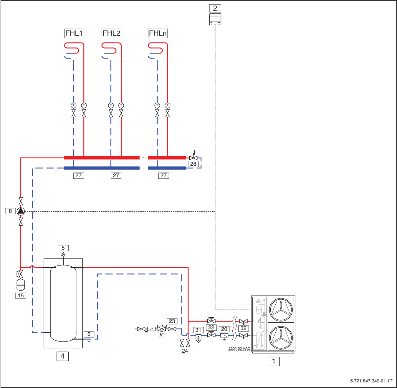
Afb. 19 Buitenunit met één of meerdere cv-groepen (CS2000AWF 18-30 R-T)
