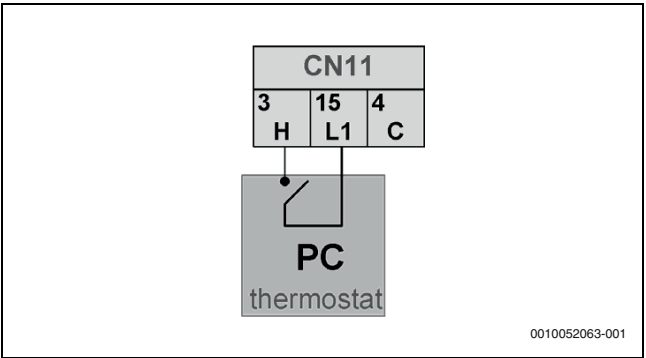
Afb. 87 Kamerthermostaat HMI-configuratie
