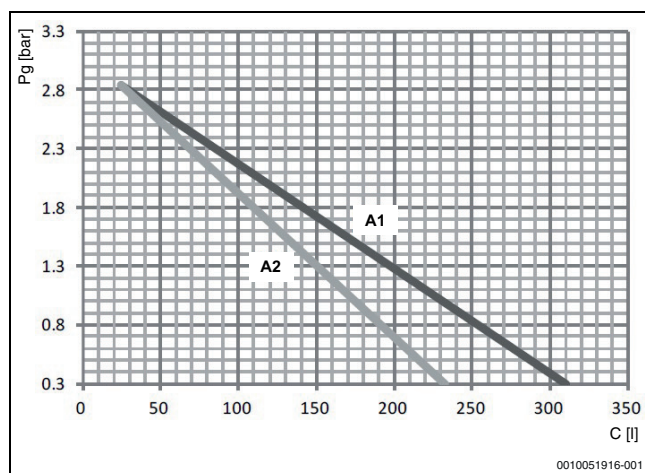
Afb. 57 Maximale waterinhoud
