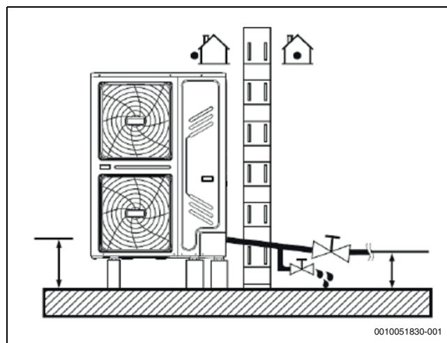
Afb. 54 Vorstbeveiliging watercircuit
