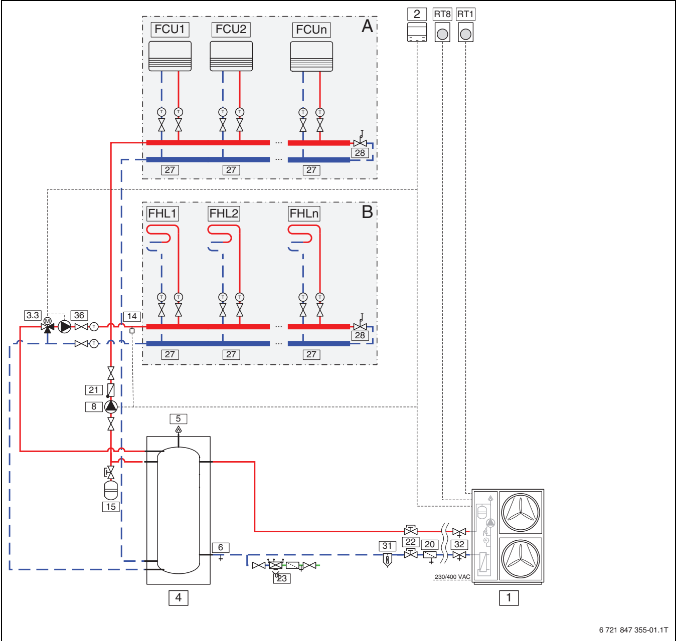
Afb. 25 Buitenunit met één of meerdere cv-groepen, vloerverwarming en radiatoren (CS2000AWF 18-30 R-T)
