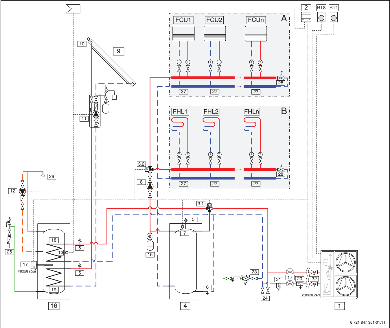
Afb. 21 Buitenunit met één of meerdere cv-groepen, elektrische back-up verwarming, boiler en zonnepsysteem (CS2000AWF 18-30 R-T)
