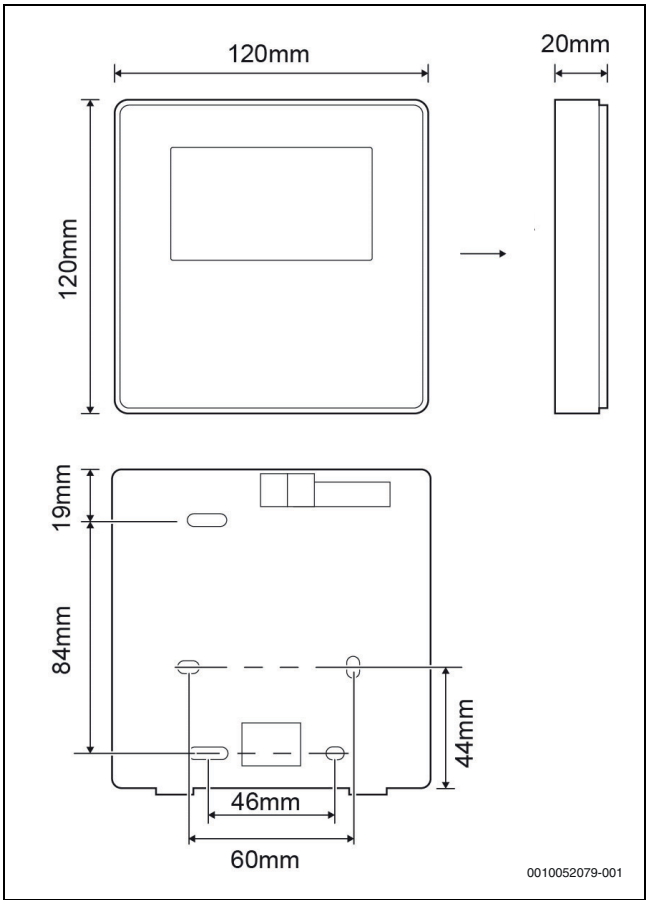
Afb. 95 Installatie de gebruikersinterface
