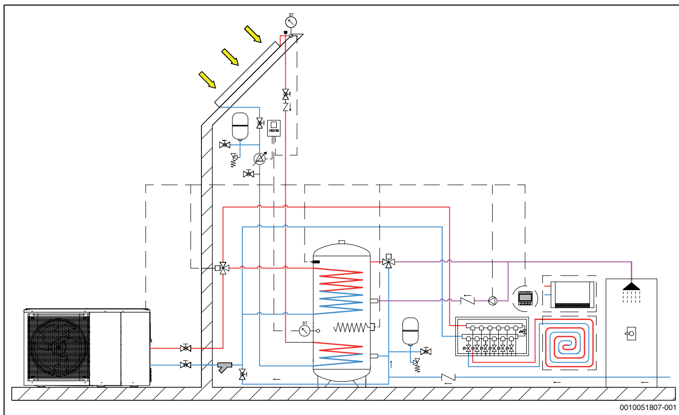
Afb. 52 Watersaansluitingen
