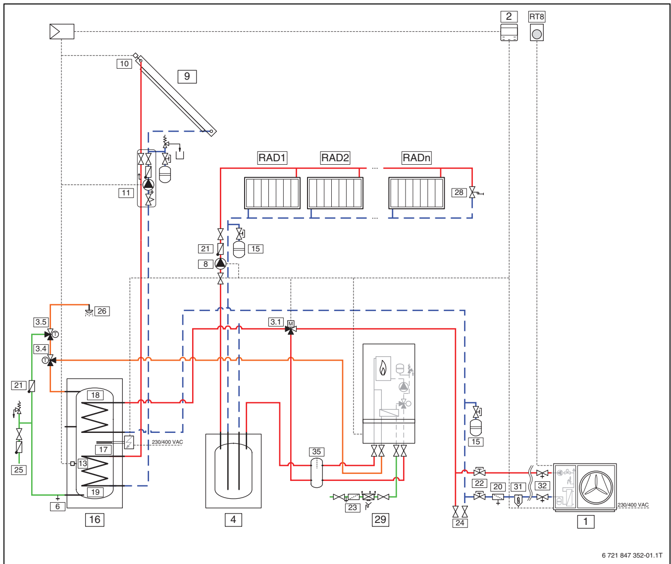
Afb. 22 Buitenunit met één of meerdere cv-groepen, externe bijverwarming, boiler en zonnepsysteem (CS2000AWF 4-6 R-S, CS2000AWF 8-10 R-S, CS2000AWF 12-16 R-S/T)
