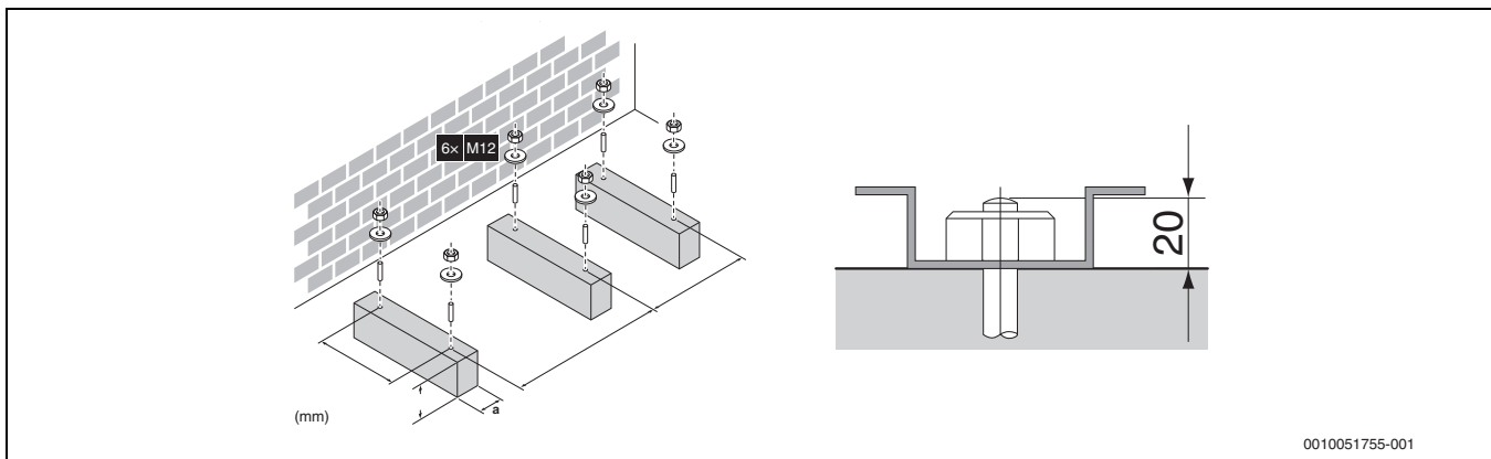
Afb. 41 Montage op de grond
