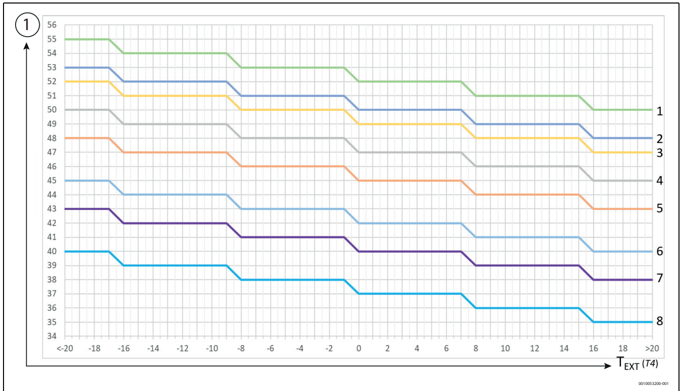
Afb. 146 Verwarmingsbedrijf op systemen met verdeling naar de eindapparaten
