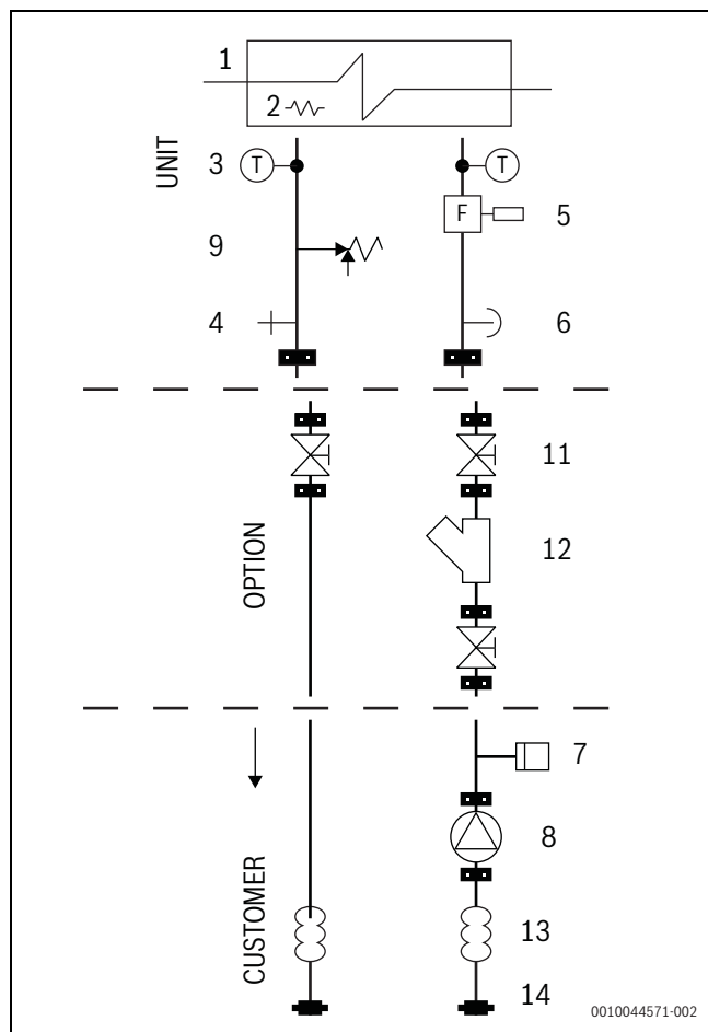
Afb. 23 Standaardeenheid
