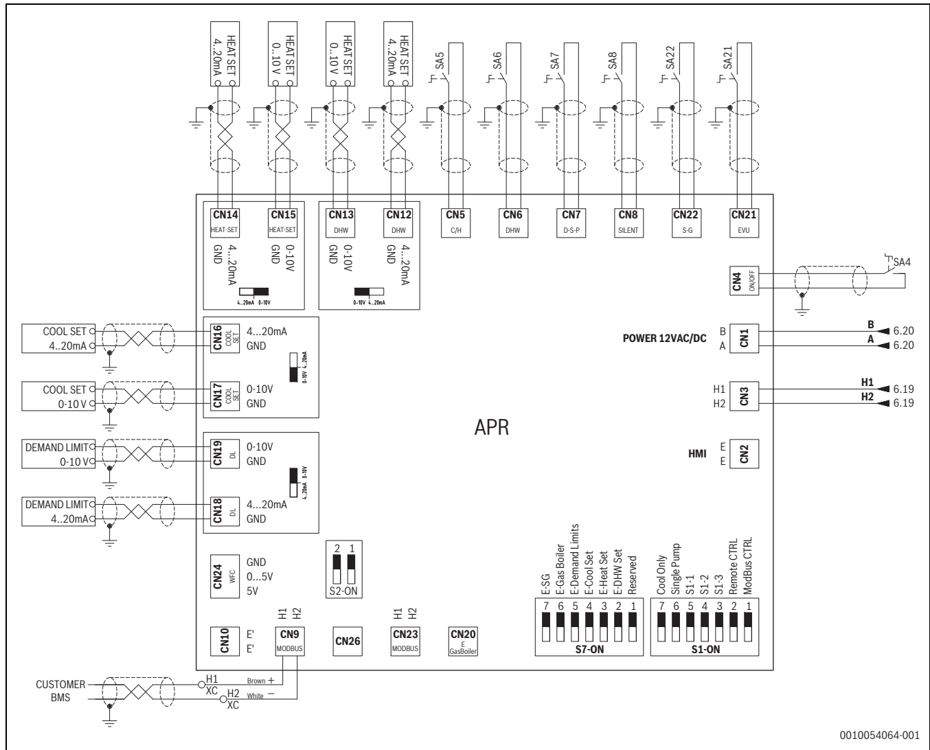
34. ábra AWP16 – AWP89
