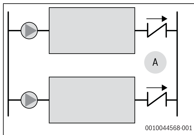
22. ábra Visszacsapó szelep
