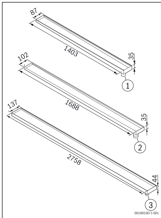
13. ábra Lefolyótálca az 1-4. alváz esetében
