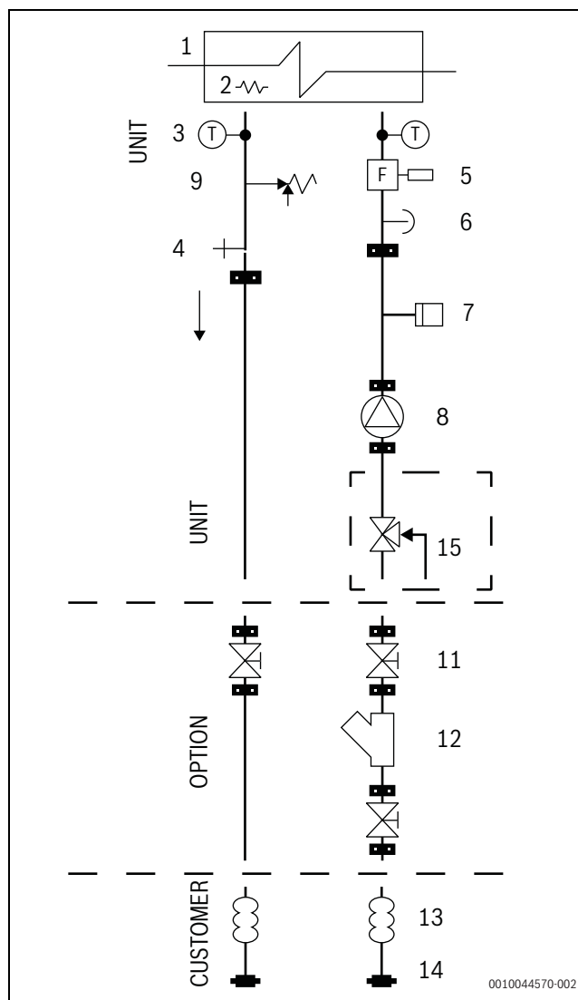
Rys. 26 Jednostka, pompa, zasobnik wody i zawór 3-drogowy do c.w.u. 15. Zawór c.w.u.
