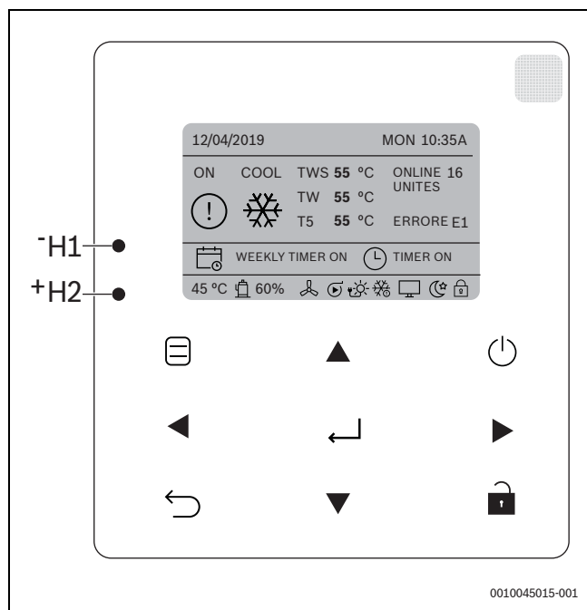
35. ábra HMI-kijelző áttekintése
