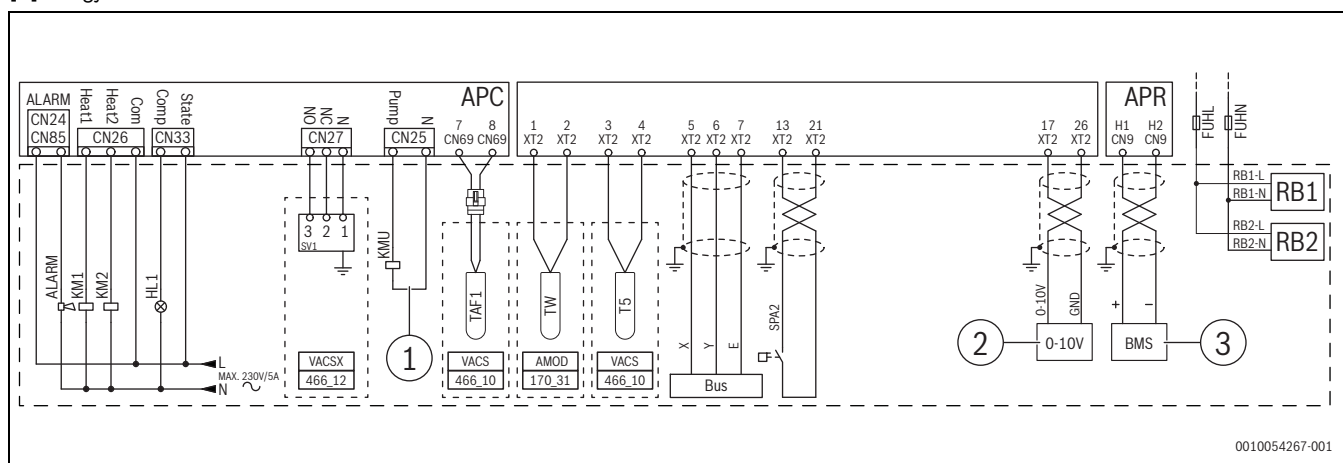
31. ábra AWP31 – AWP89 (≤ 2024.06.)
