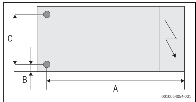
15. ábra Kondenzvíz-csatlakozó lefolyótálca
