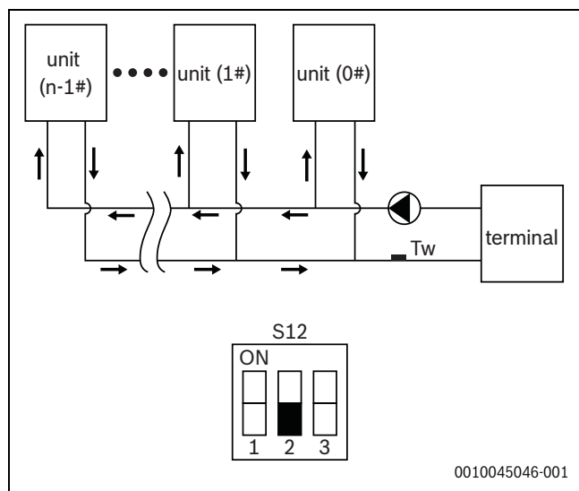
Rys. 72 Pojedyncza pompa wody
