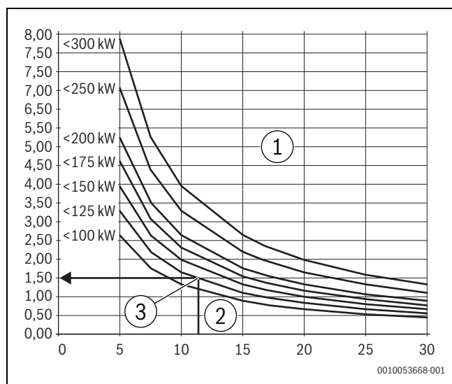
Rys. 17 Wymagania dotyczące objętości wody do napełniania i uzupełniania dla urządzeń grzewczych 100–300 kW
