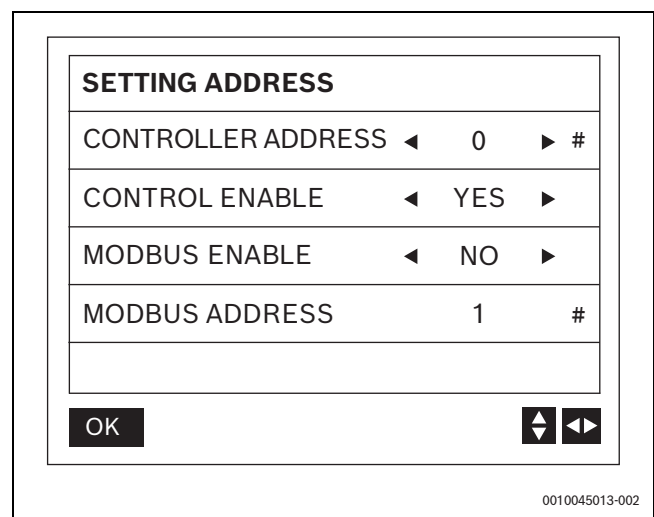
75. ábra Vezérlők cím kiosztása
