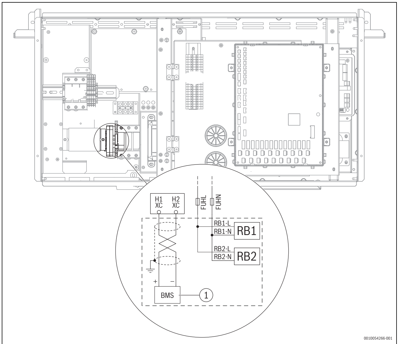
Afb. 30 AWP16 – AWP24(detail nieuwe installatie)
