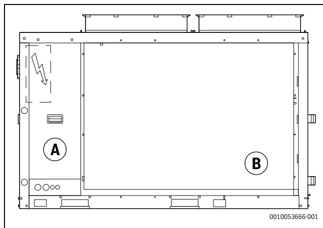
Rys. 3 Zakres dostawy – lokalizacja akcesoriów dostarczanych z jednostką
