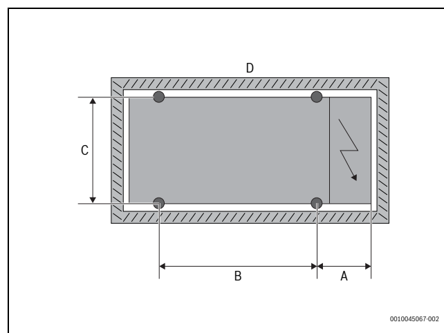
Rys. 12 Lokalizacja tłumików drgań
