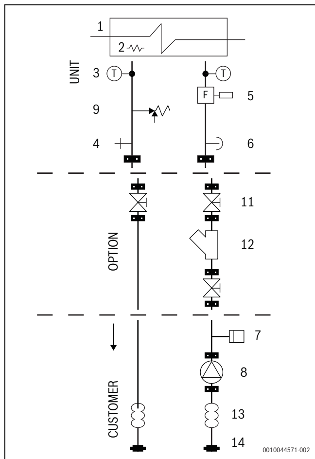
Rys. 23 Standardowa jednostka
