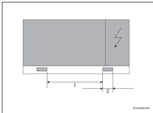
Sl.4 Upotrijebite viličar za AWP16 – AWP24AWP31 – AWP41
