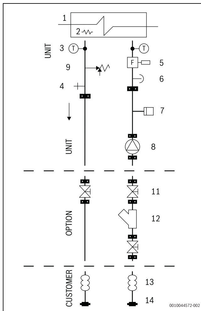
Afb. 24 Eenheid en pomp
