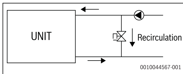
Rys. 21 Układ hydrauliczny: przepływność > maksymalny przepływ
