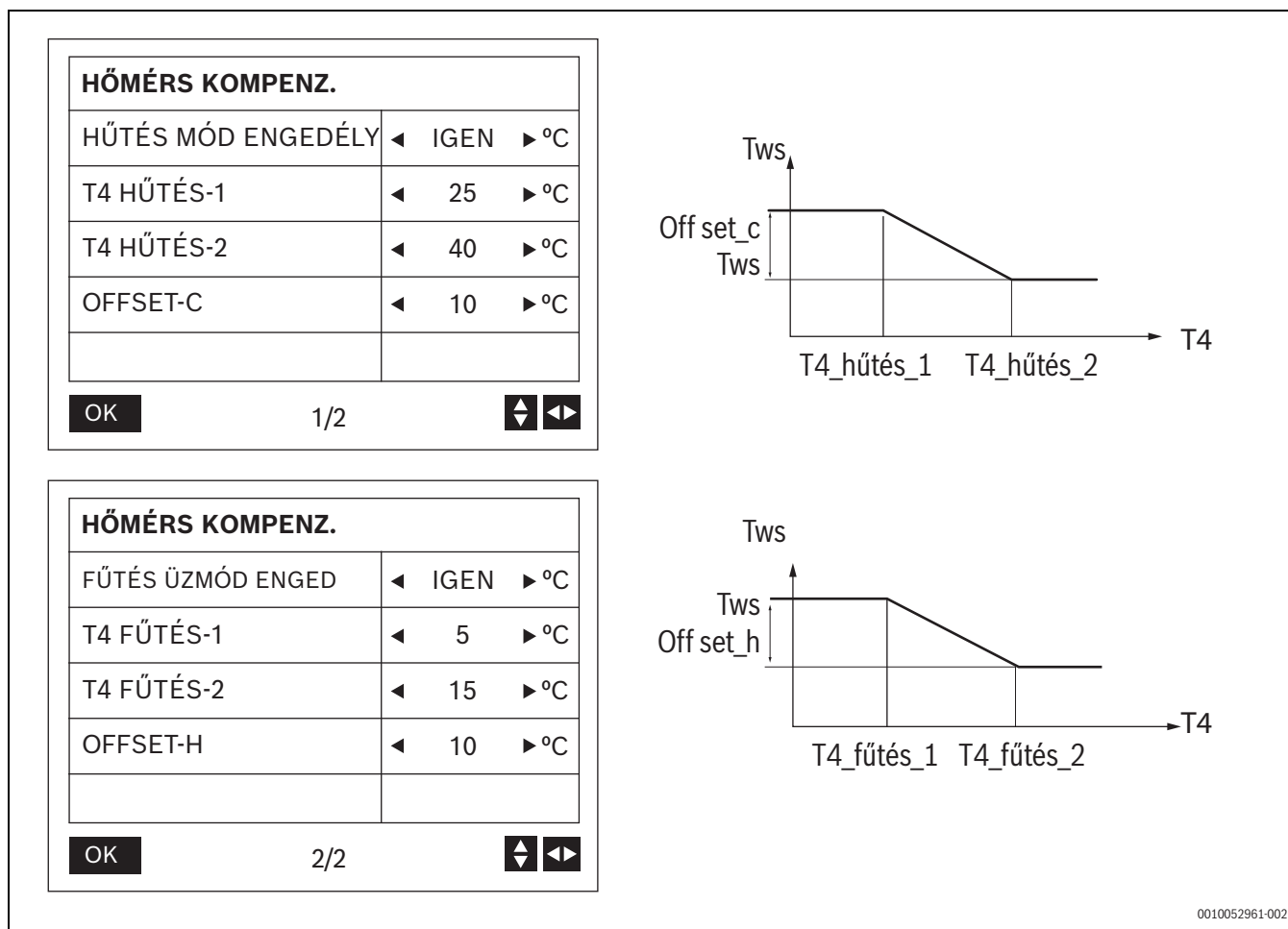
45. ábra Hőmérséklet-kompenzációs beállítások
