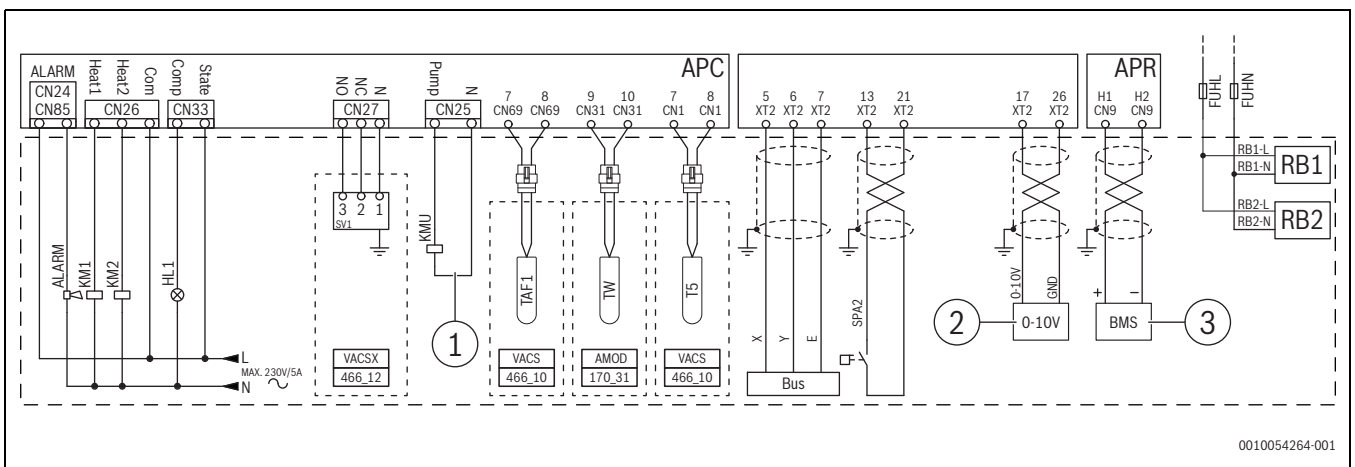
28. ábra AWP16 – AWP24 (≤ 2024.06.)
