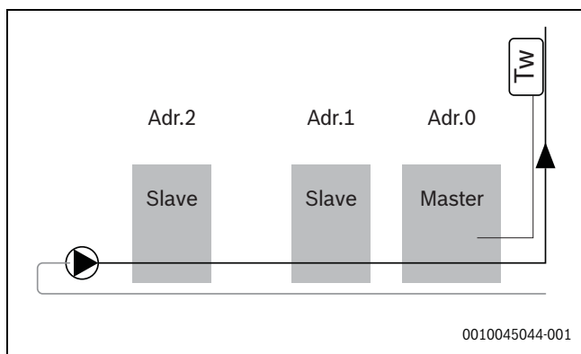
Rys. 69 Czujnik Tw
