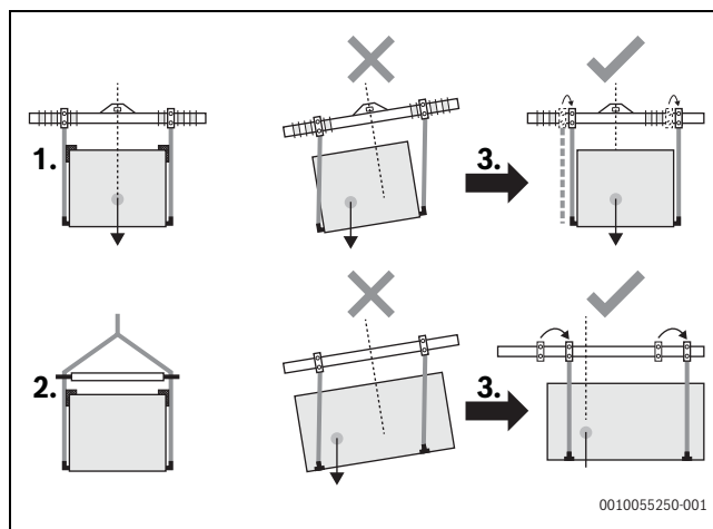
8. ábra Az egység felemelése
