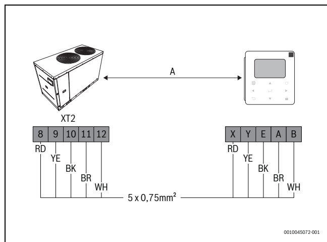
Sl.36 Maksimalna udaljenost 40 m. Snaga koju daje jedinica.
