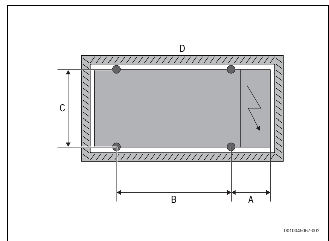
Afb. 12 Positie voor de anti-vibratiekoppelingen
