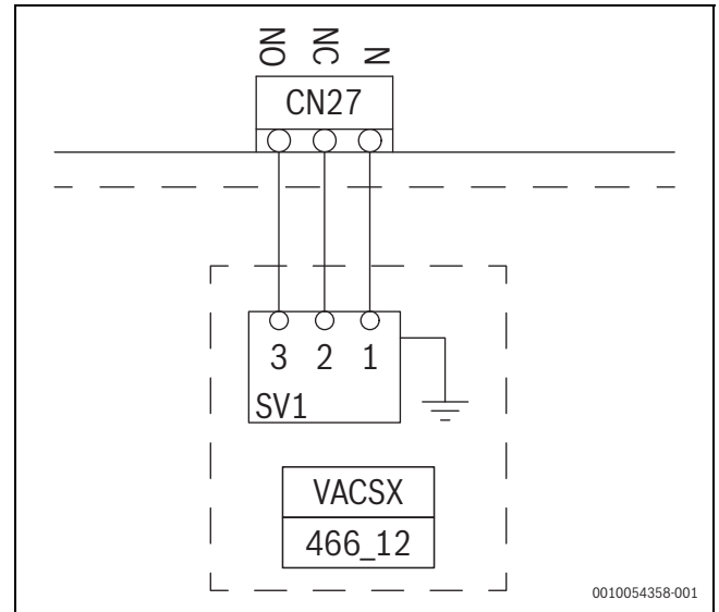
Afb. 43 Aansluiting van externe 3-wegklep voor warm tapwater
