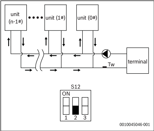
Afb. 72 Enkele waterpompen
