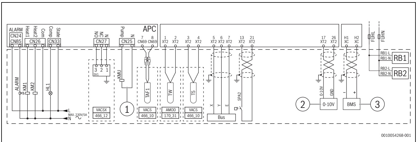
32. ábra AWP31 – AWP89 (≥ 2024.06.)
