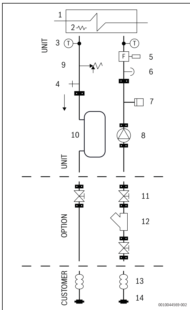
Afb. 25 Eenheid en opslagtank
