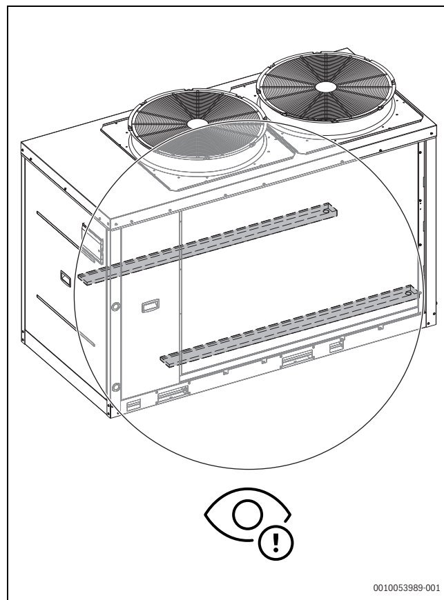
Afb. 14 Installatie condensbakken
