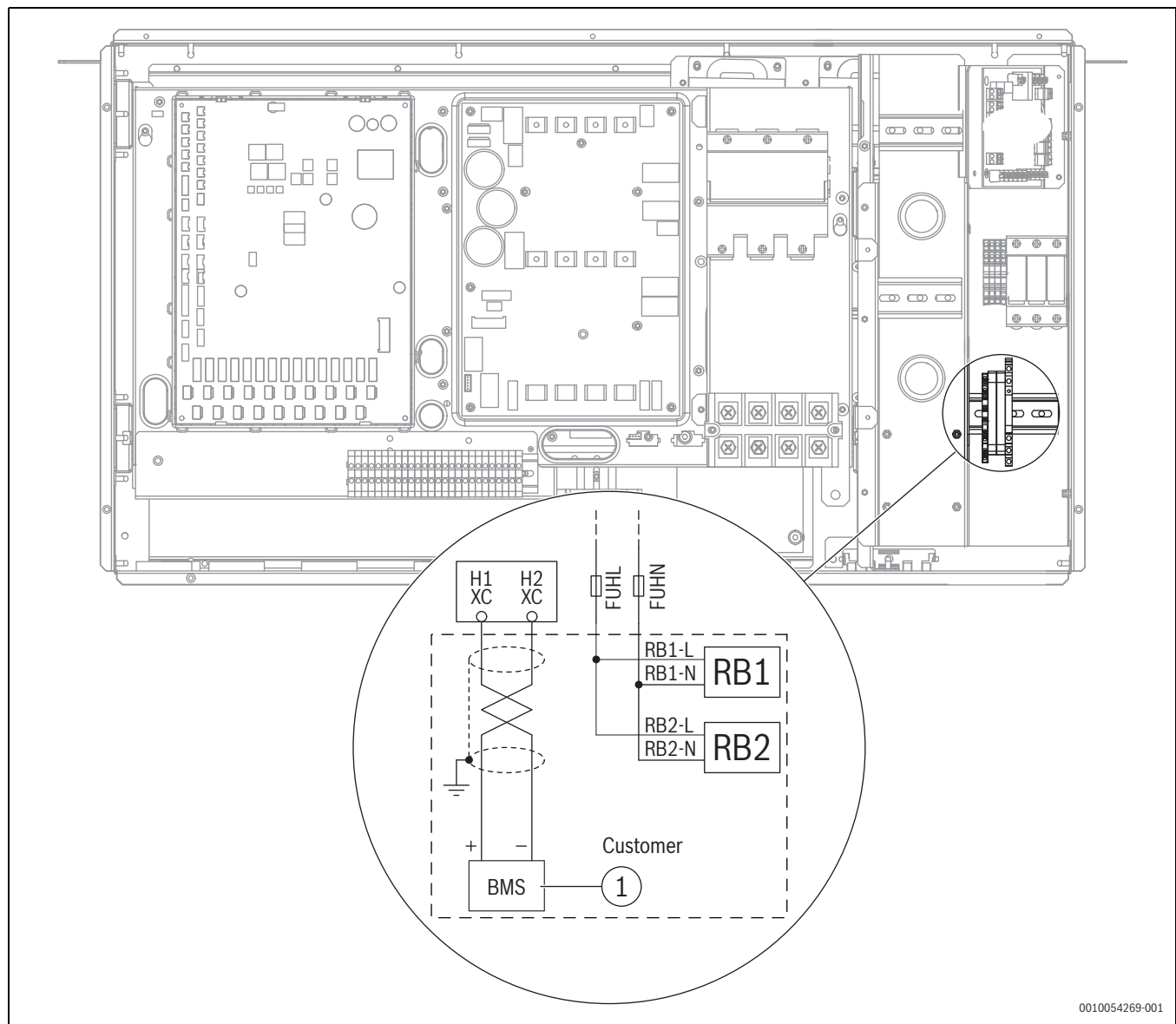
Sl.33 AWP31 – AWP89 (detaljni prikaz nove instalacije)
