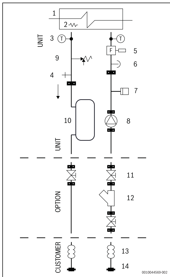
25. ábra Egység és tárolótartály
