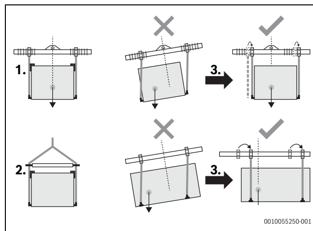
Rys. 8 Podnoszenie jednostki
