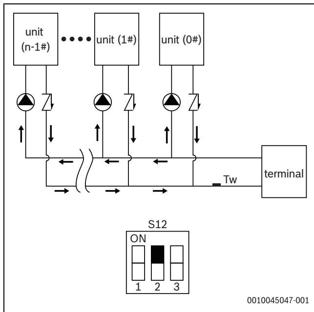
Afb. 73 Meervoudige waterpompen
