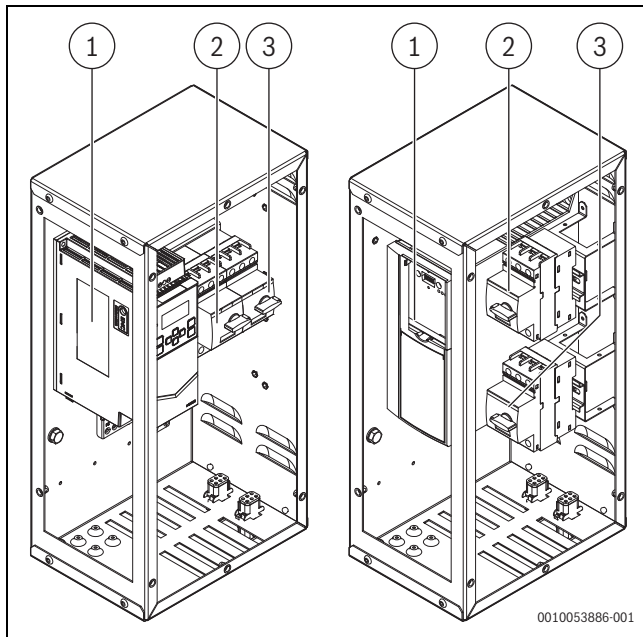
Afb. 41 Pompomvormer AWP65 – AWP89
