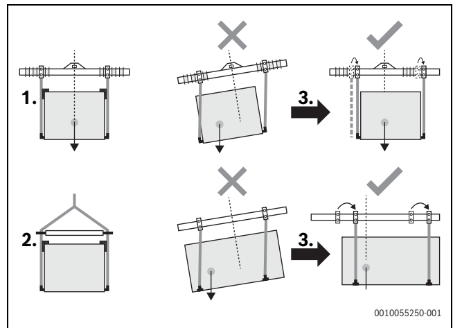
Afb. 8 Hijsen van de eenheid
