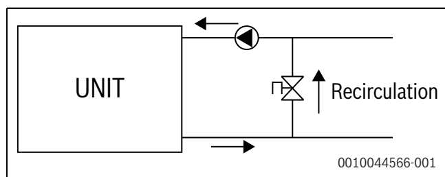
20. ábra Hidraulikus: Kapacitás < Maximális áramlás
