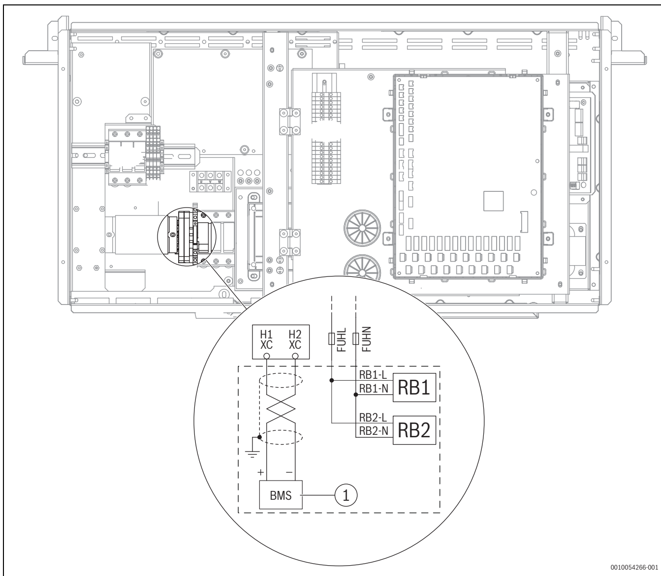
SI.30 AWP16 – AWP24(detaljni prikaz nove instalacije)
