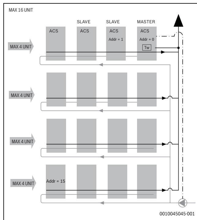
Rys. 71 Schemat układu z odwróconym przyłączem powrotnym
