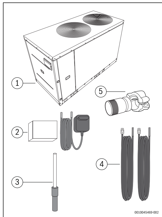
Afb. 2 Leveringsomvang - warmtepompeenheid
