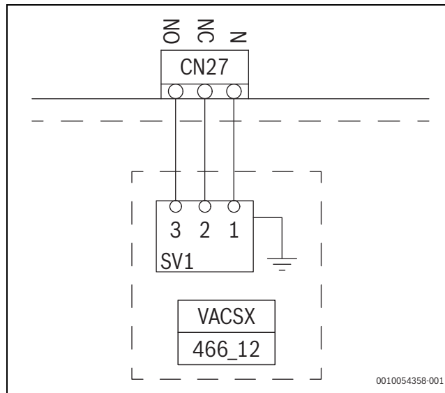
Rys. 43 Podłączenie zewnętrznego zaworu 3-drogowego do c.w.u.
