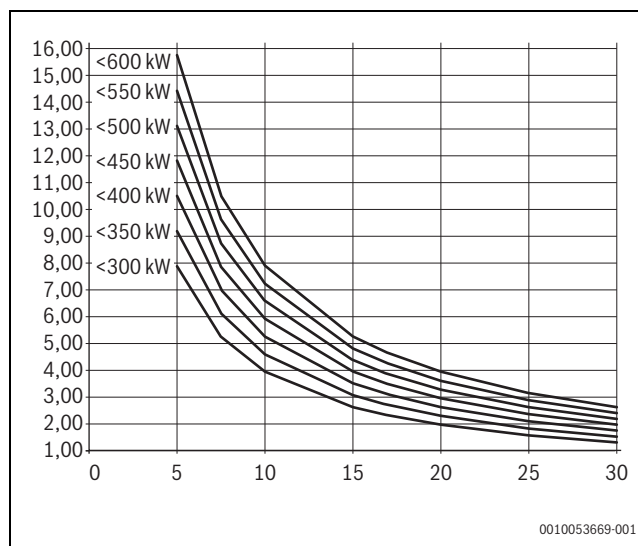
18. ábra A töltő- és pótvíz mennyiségére vonatkozó követelmények 300-600 kW hőtermelők esetén
