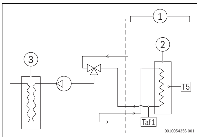
Afb. 42 Warmwaterhydraulica en positionering temperatuursensoren
