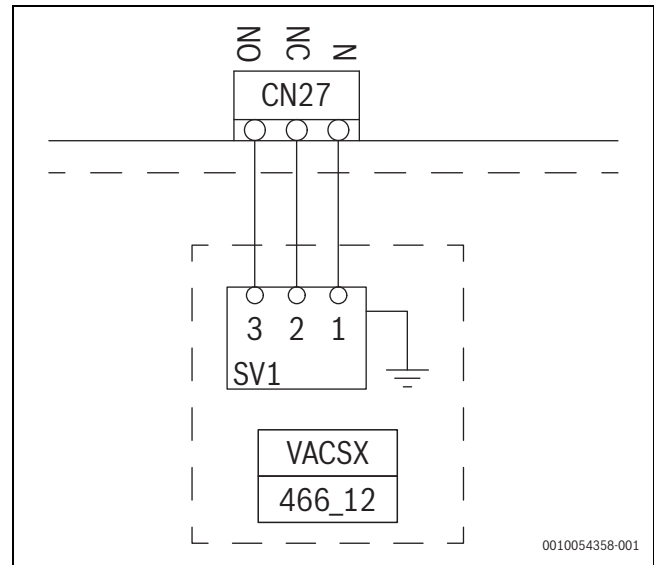
43. ábra Egy külső háromutas szelep csatlakoztatása a melegvízhez
