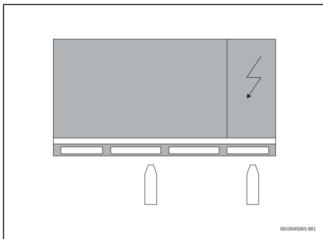
Rys. 5 Jednostka AWP53 – AWP59 na paletach
