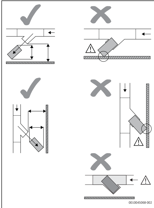
Sl.19 Upute za instalaciju filtra
