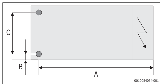
Afb. 15 Condensaataansluiting condensbak
