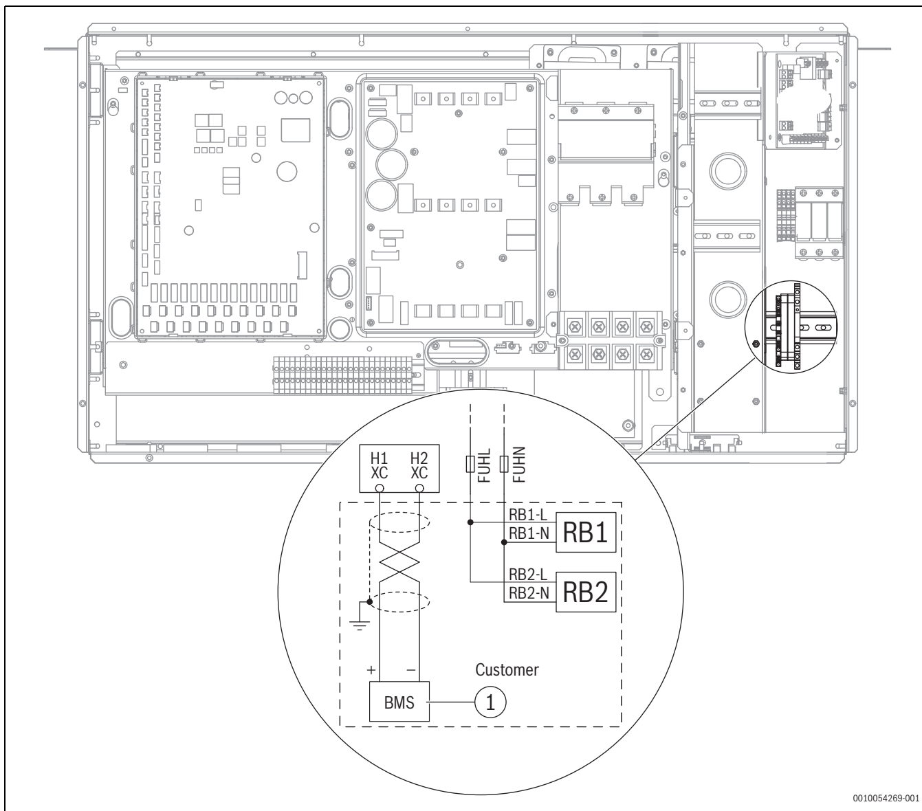
Rys. 33 AWP31 – AWP89 (szczegółowy widok nowej instalacji)
