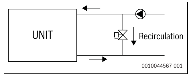
Sl.21 Hidraulika: kapacitet > maksimalni protok
