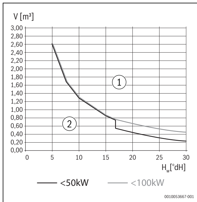
Rys. 16 Wymagania dotyczące objętości wody do napełniania i uzupełniania dla pomp ciepła ≤ 100 kW
