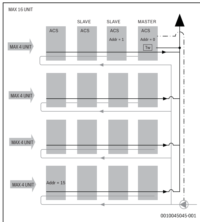
71. ábra Rendszerábra fordított visszatérő csatlakozással
