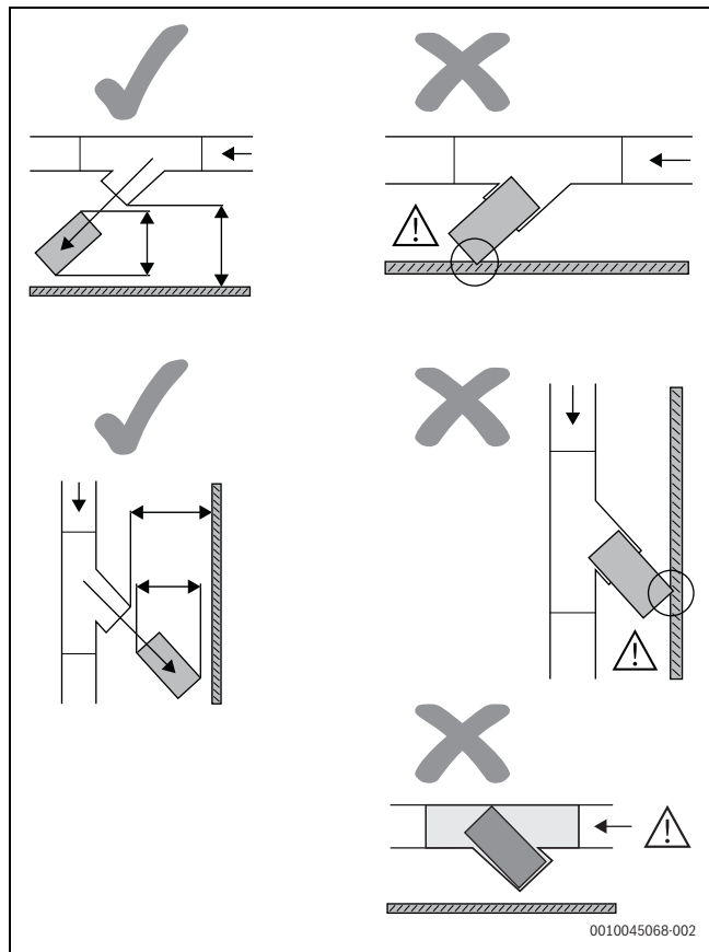
Rys. 19 Instrukcja montażu filtra
