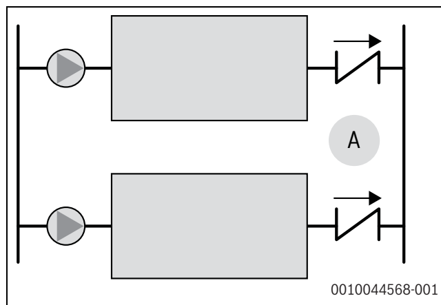
Rys. 22 Zawór jednokierunkowy
