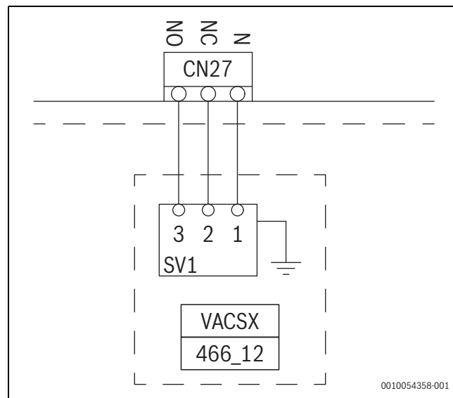
SI.43 Priključivanje vanjskog troputnog ventila za toplu vodu
