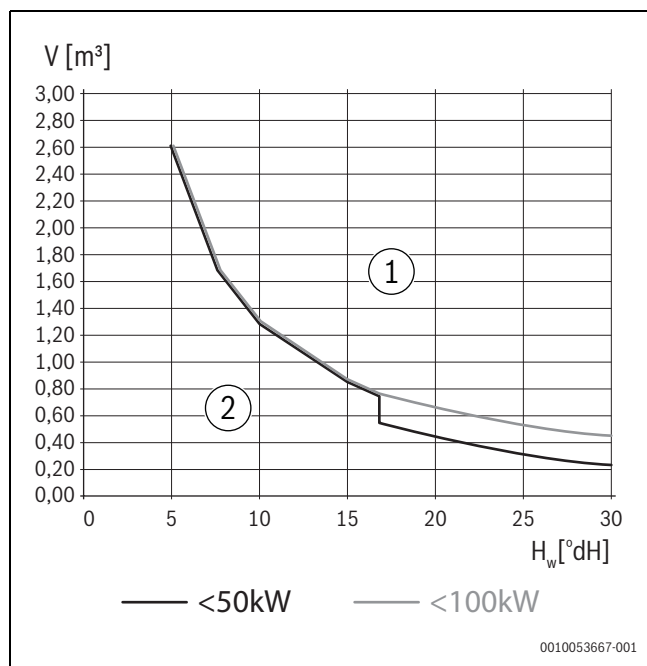
16. ábra A töltő- és pótvíz mennyiségére vonatkozó követelmények \leq 100 kW hőtermelők esetén
