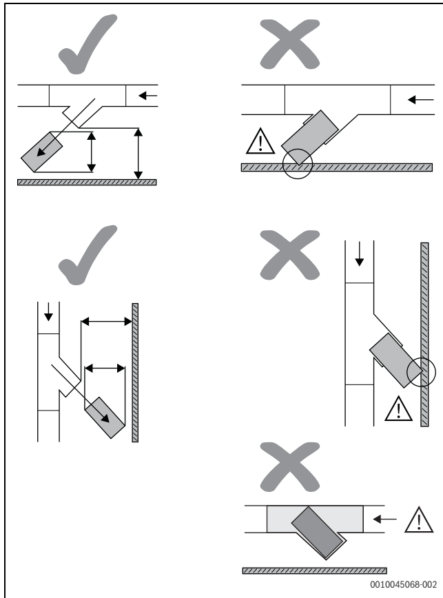
Afb. 19 Instructies filterinstallatie
