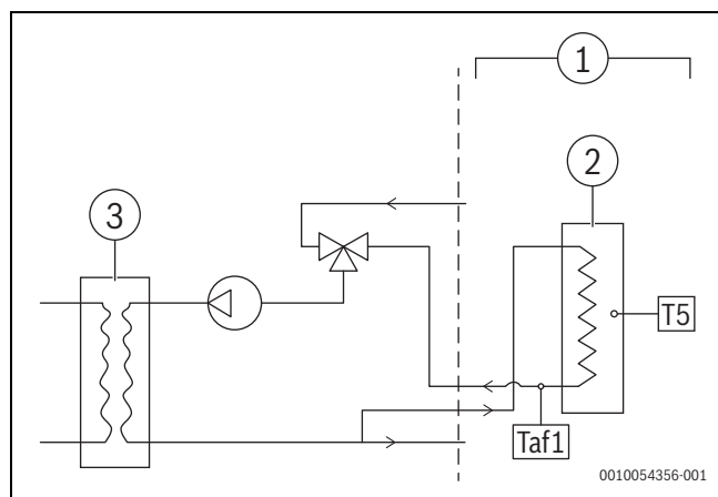
Rys. 42 Układ hydrauliczny c.w.u. i umieszczenie czujnika temperatury
