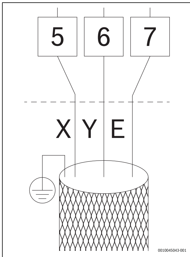
Rys. 70 Magistrala komunikacyjna jednostki modułowej
