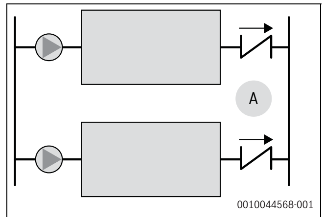
Afb. 22 terugslagklep
