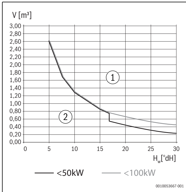
Afb. 16 Voorwaarden voor het vul- en bijvulwatervolume van warmtepompen met een vermogen van \leq 100 kW
