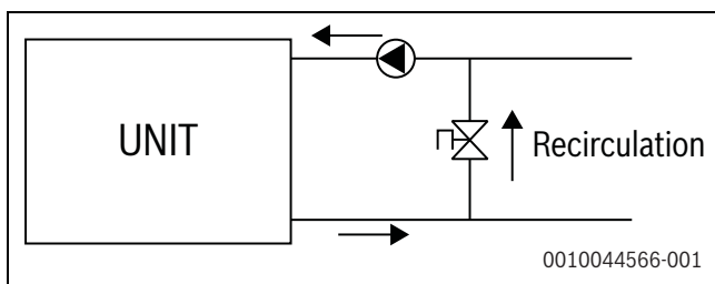
Afb. 20 Hydrauliek: capaciteit < maximale aanvoer
