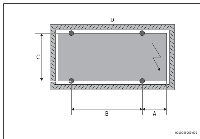
12. ábra A rezgéscsillapító csatlakozók helye
