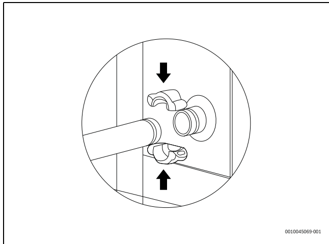
27. ábra Victaulic csatlakozás: csatlakozókötés, csatlakozó és bilincs (alkatrészek balról jobbra)
