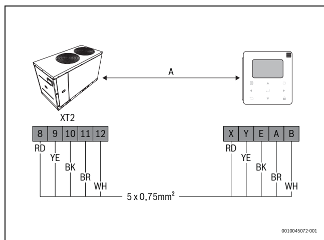
36. ábra A maximális távolság 40 m. A tápellátást az egység biztosítja.
