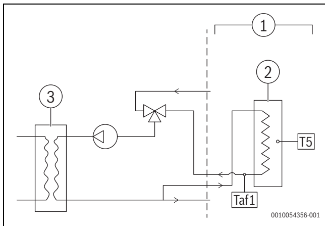
42. ábra DHW hidraulikus és hőmérséklet-érzékelők elhelyezése
