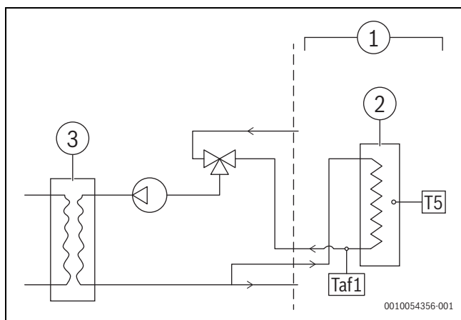
SI.42 Položaj hidrauličkog priključka za toplu vodu i temperaturnih osjetnika
