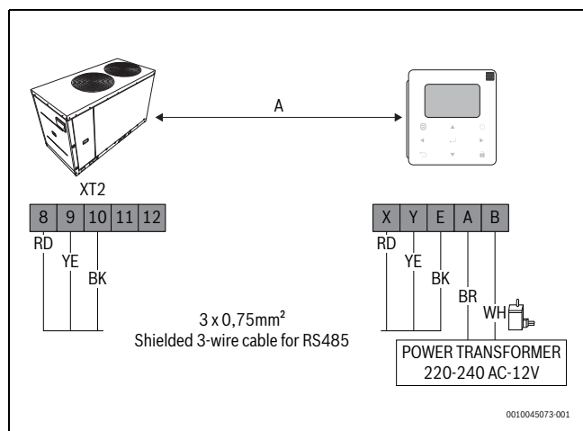
Sl.37 Maksimalna udaljenost 300 m. Odvojeni mrežni modul - mrežni modul isporučen s jedinicom.
