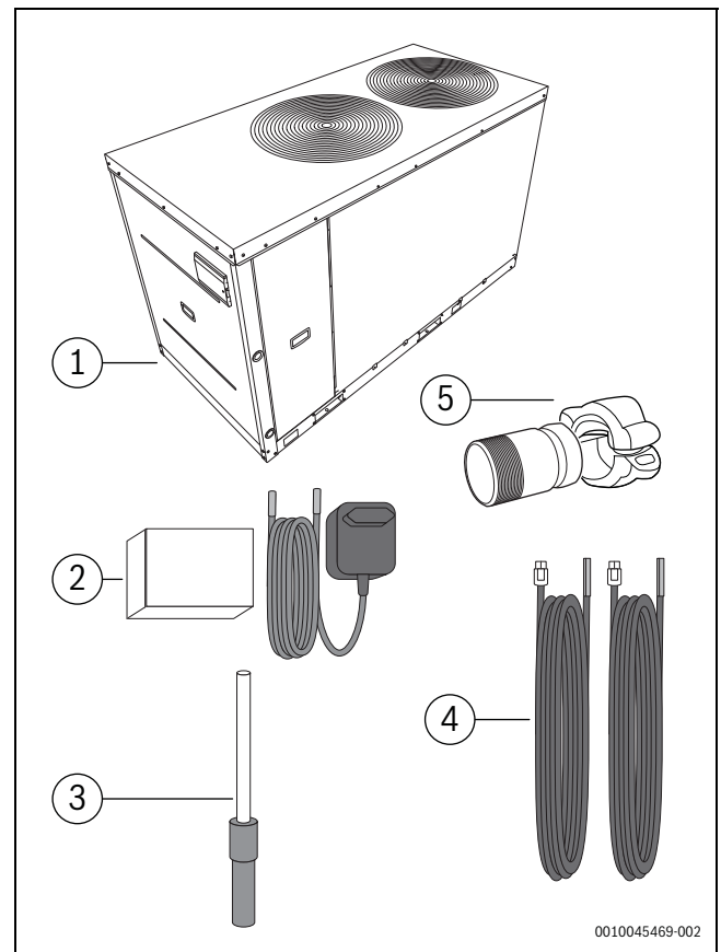
Rys. 2 Zakres dostawy – jednostka pompy ciepła
