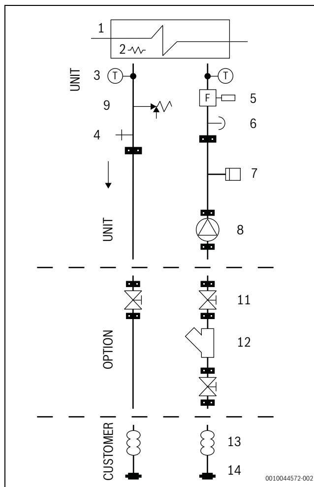
Sl. 24 Jedinica i pumpa
