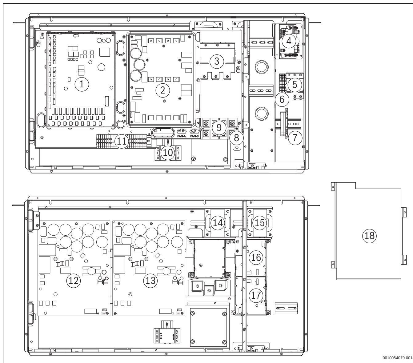
39. ábra AWP31 – AWP59
