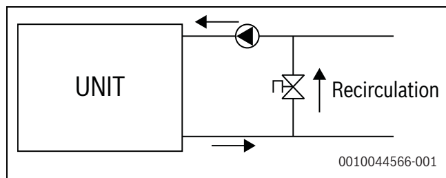
Rys. 20 Układ hydrauliczny: przepływność < maksymalny przepływ
