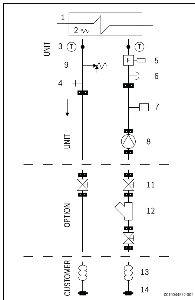
Rys. 24 Jednostka i pompa
