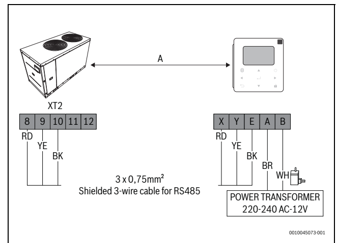
Afb. 37 Maximale afstand 300 m. Separate voeding - voedingsspanning geleverd met de eenheid.
