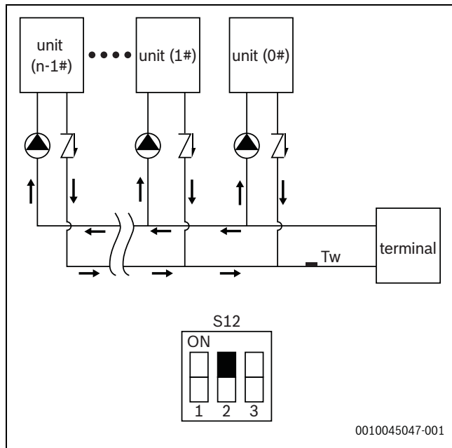
73. ábra Több vízszivattyús
