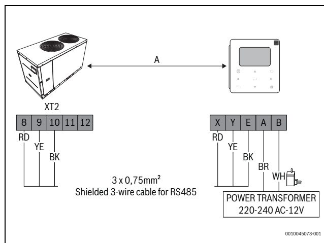
37. ábra A maximális távolság 300 m. Különálló tápegység – a tápellátást az egység biztosítja.
