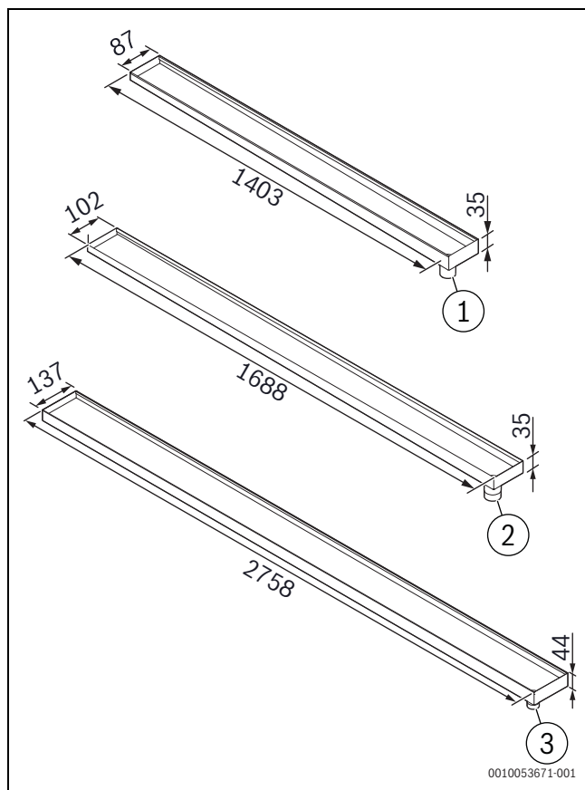
Rys. 13 Rama zbiornika na skropliny 1-4
