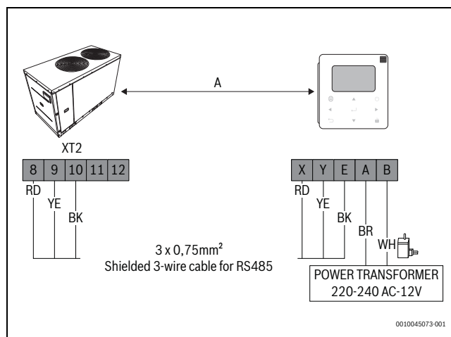
Rys. 37 Maksymalna odległość wynosi 300 m. Oddzielne zasilanie – zasilanie zapewnione z jednostką.
