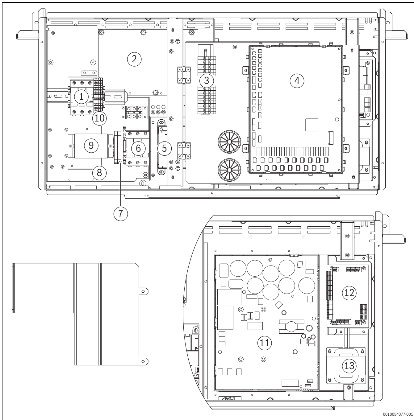
38. ábra AWP16 – AWP24
