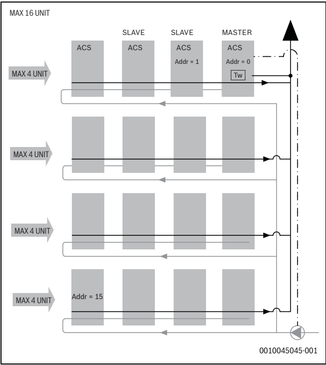
Afb. 71 Systeemschema met omgekeerde retouraansluiting
