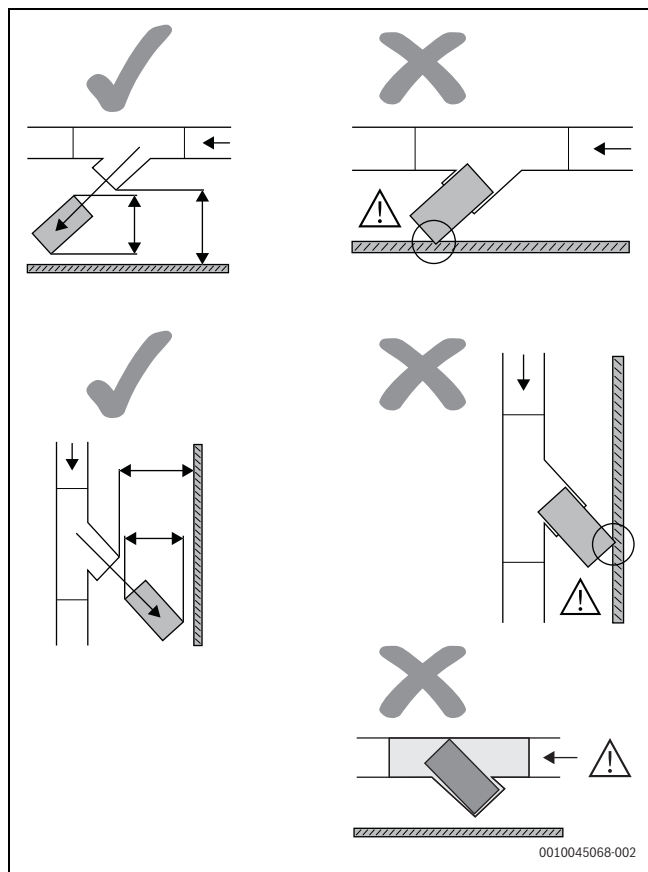
19. ábra Szűrő: szerelési útmutató
