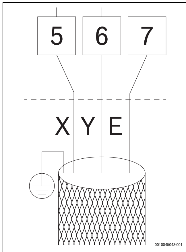
70. ábra Moduláris egység kommunikációs busza
