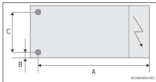
Sl. 15 Priključak posude za odvod kondenzata
