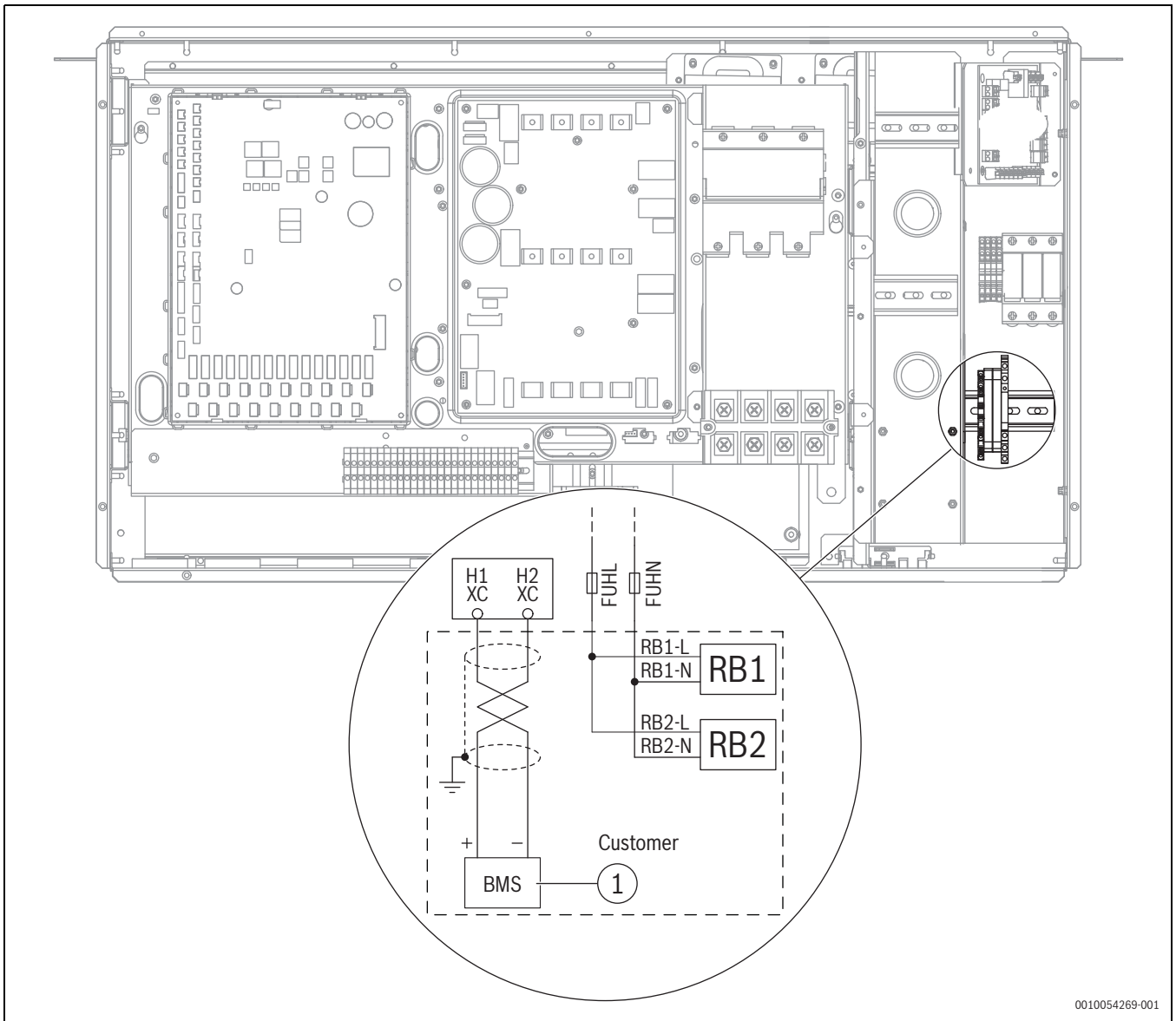
33. ábra AWP31 – AWP89 (új rendszer áttekintés)
