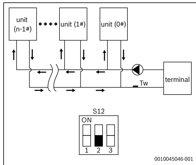
72. ábra Egy szivattyús
