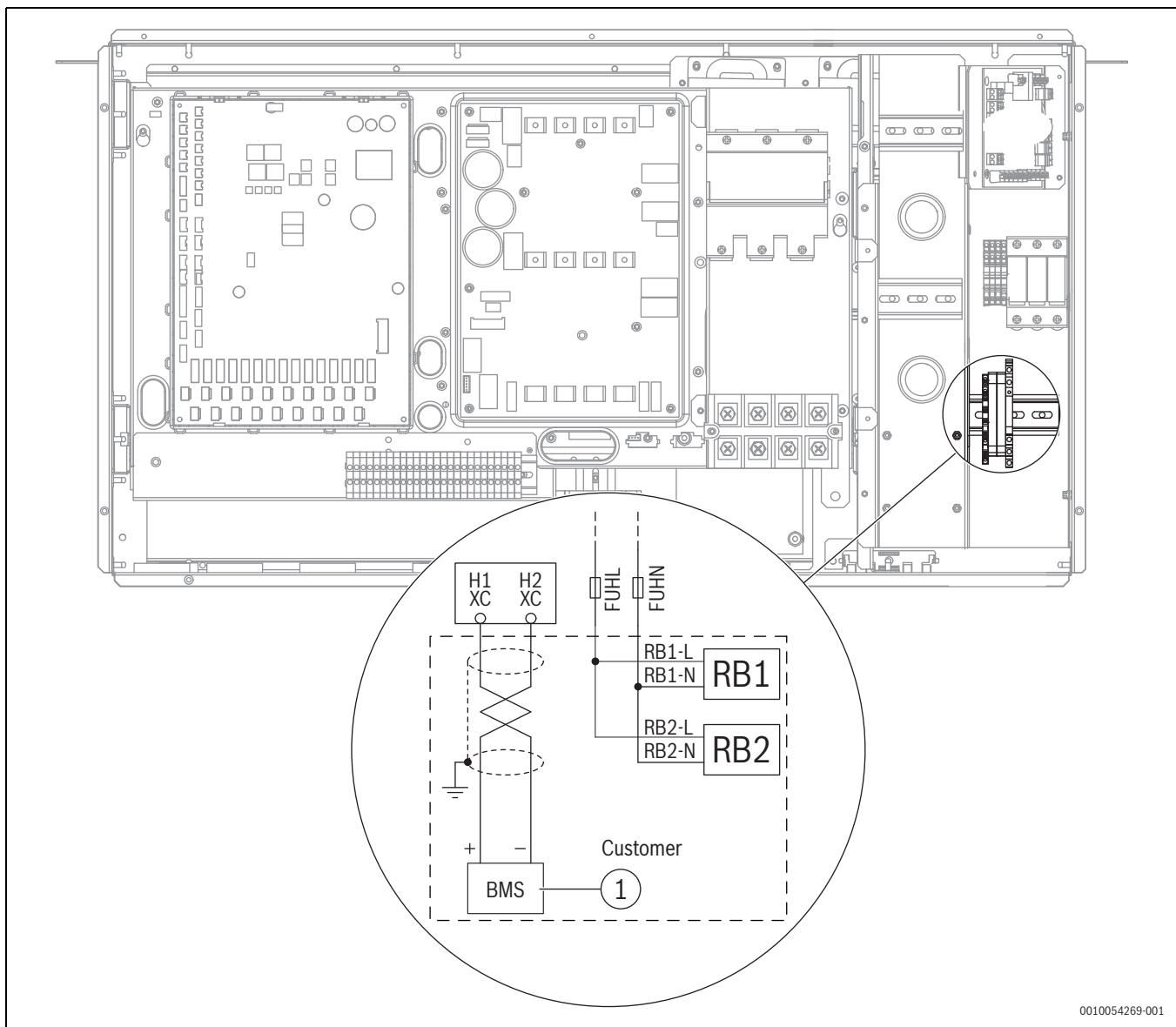
Afb. 33 AWP31 – AWP89 (detail nieuwe installatie)
