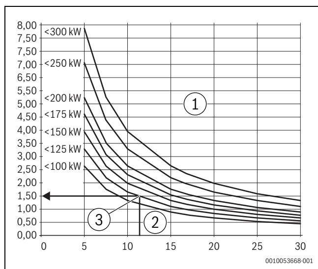
17. ábra A töltő- és pótvíz mennyiségére vonatkozó követelmények 100-300 kW hőtermelők esetén
