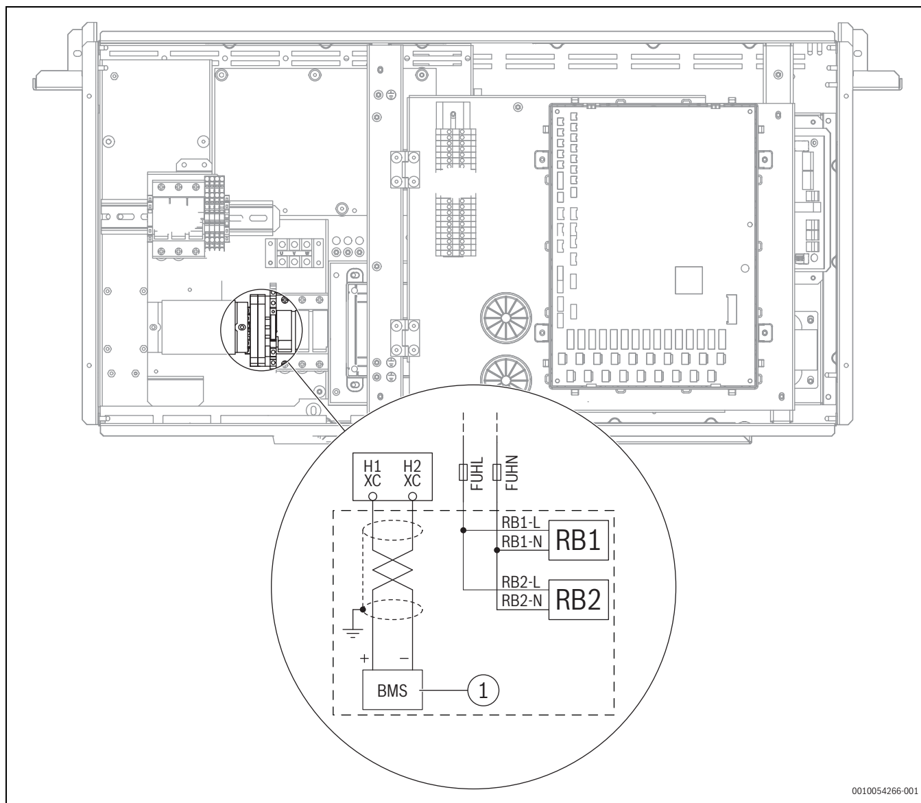
Rys. 30 AWP16 – AWP24 (szczegółowy widok nowej instalacji)
