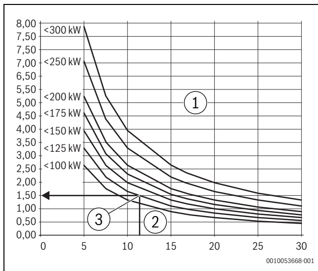
Afb. 17 Voorwaarden voor het vul- en bijvulwatervolume van warmtepompen met een vermogen van 100-300 kW
