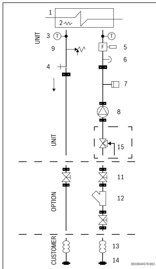
Sl. 26 Jedinica, pumpa, spremnik za vodu i troputni ventil za toplu vodu
