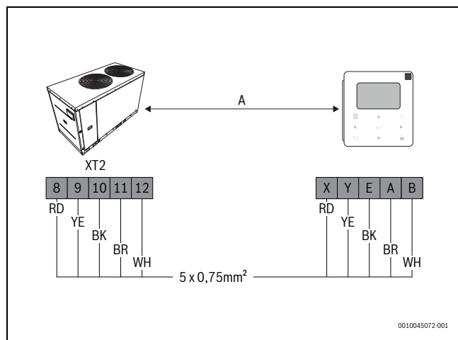
Rys. 36 Maksymalna odległość wynosi 40 m. Zasilanie dostarczane przez jednostkę.
