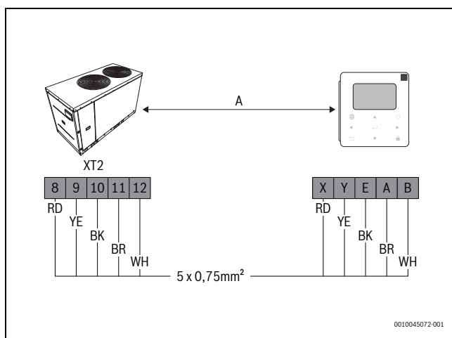
Afb. 36 Maximale afstand 40 m. Voedingsspanning geleverd door de eenheid.
