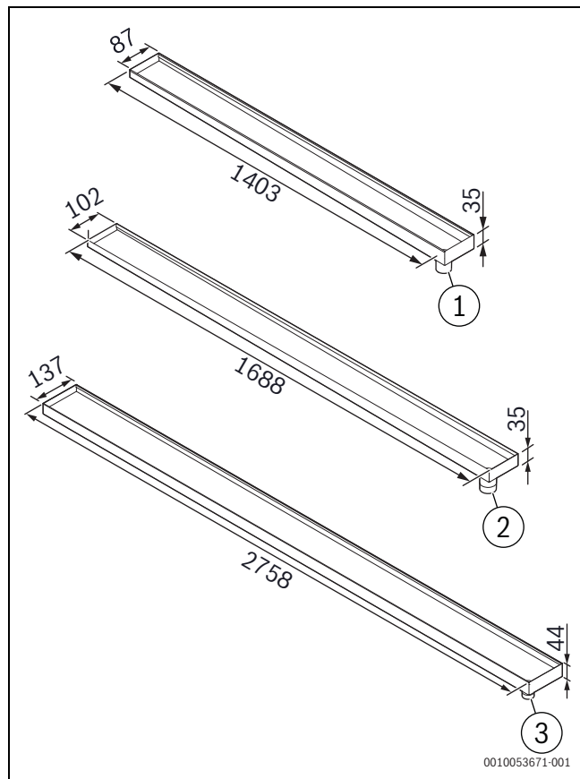
Sl. 13 Odvodna posuda kućišta 1-4
