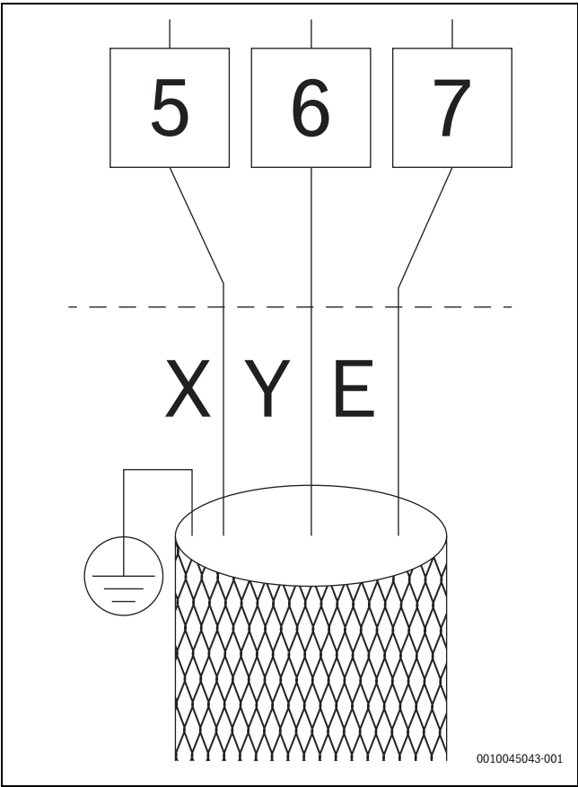
Afb. 70 Communicatiebus modulaire eenheid
