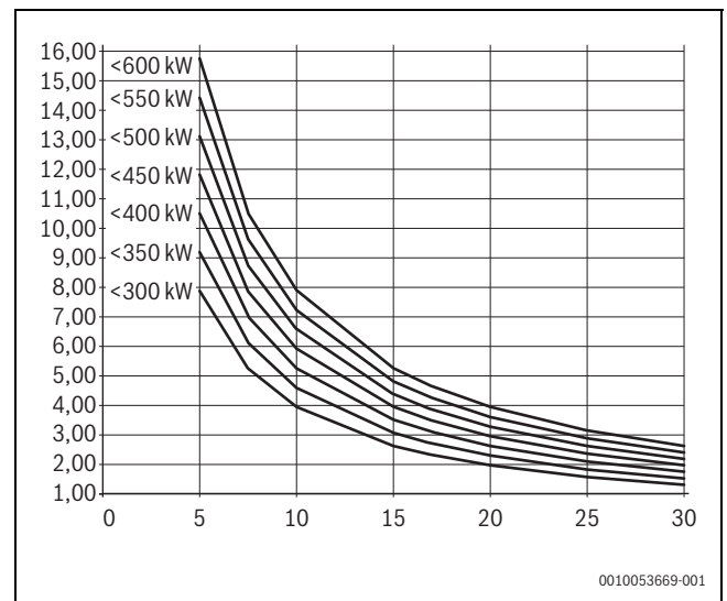
Afb. 18 Voorwaarden voor het vul- en bijvulwatervolume van warmtepompen met een vermogen van 300-600 kW
