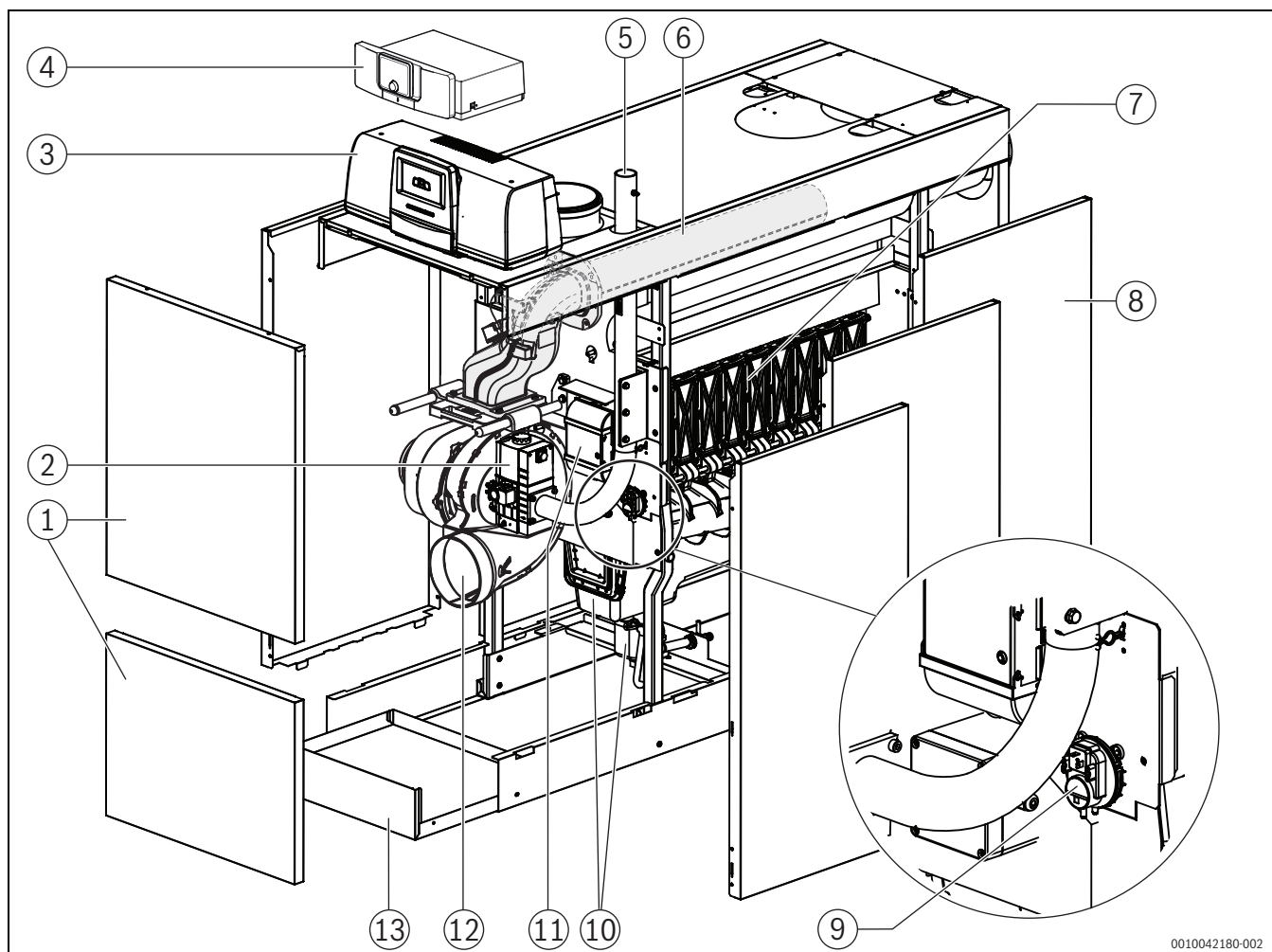
Afb. 1 Condens 7000 FP, 350...620 kW-hoofdcomponenten (getoond: rechtse uitvoering; inspectiedeksel en aanvoer en retour zijn rechts opgesteld)
