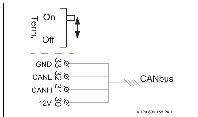
Afb. 30 CAN-BUS-afsluiting
