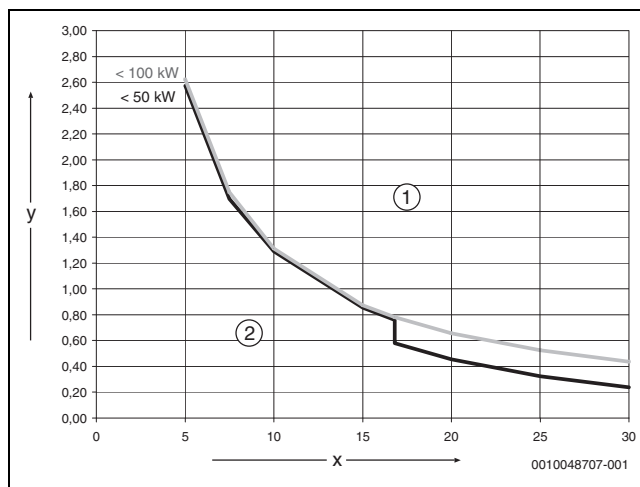
Afb. 6 Warmtebronnen < 50 kW-100 kW
