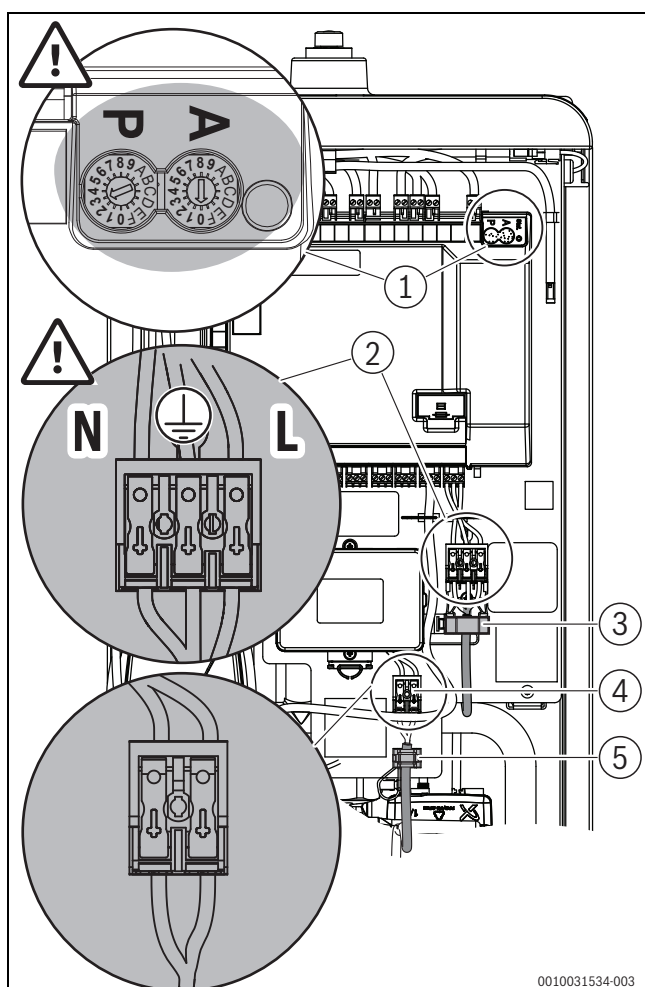
Afb. 29 Uitvoeren netaansluiting en stuurleiding bijverwarming aansluiten
