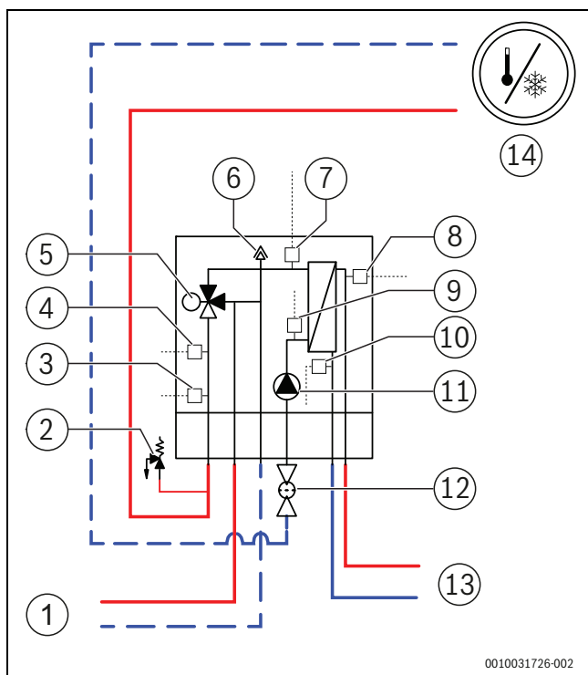
Afb. 43 Hydraulisch schema van de binnenunit
