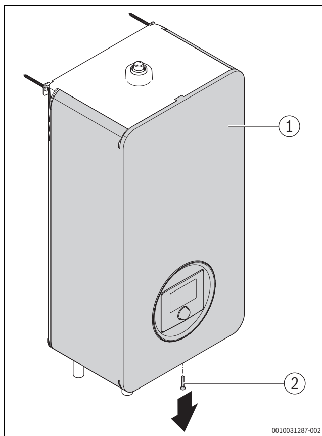
Afb. 11 Afdekkap ontgrendelen
