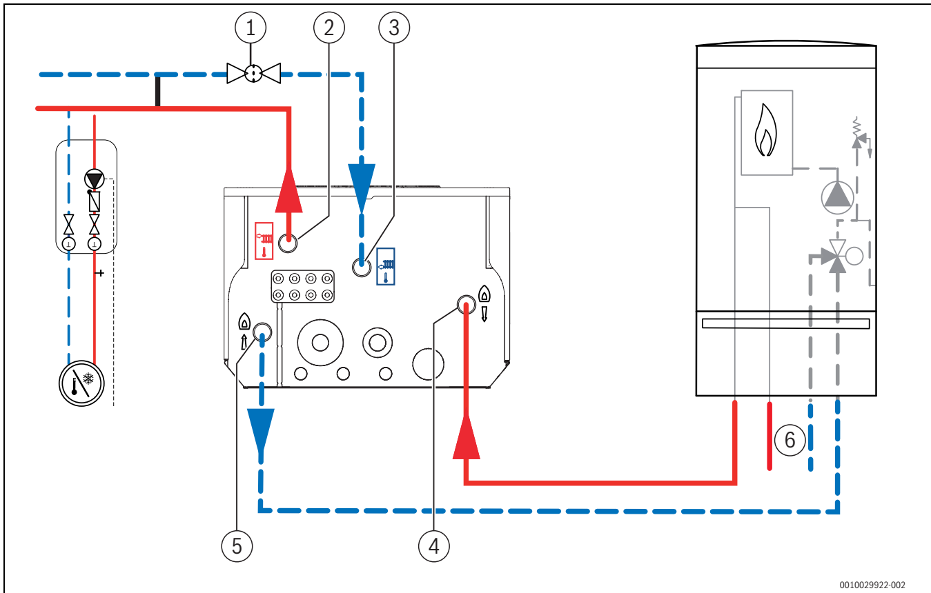
Afb. 22 Aansluiting van de binnenunit op de cv-installatie en de bijverwarming (voorbeeldweergave met bypass en extra cv-pomp)
