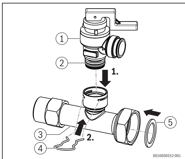
Afb. 7 Montage overstortventiel
