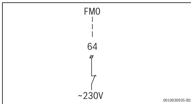
Afb. 32 Aansluiting voor externe bijverwarming met 230 V-alarmuit-gang
