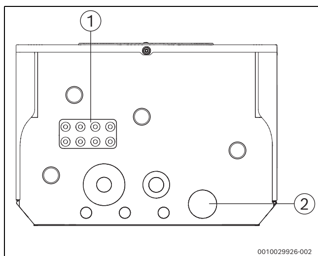
Afb. 28 kabeldoorvoeren
