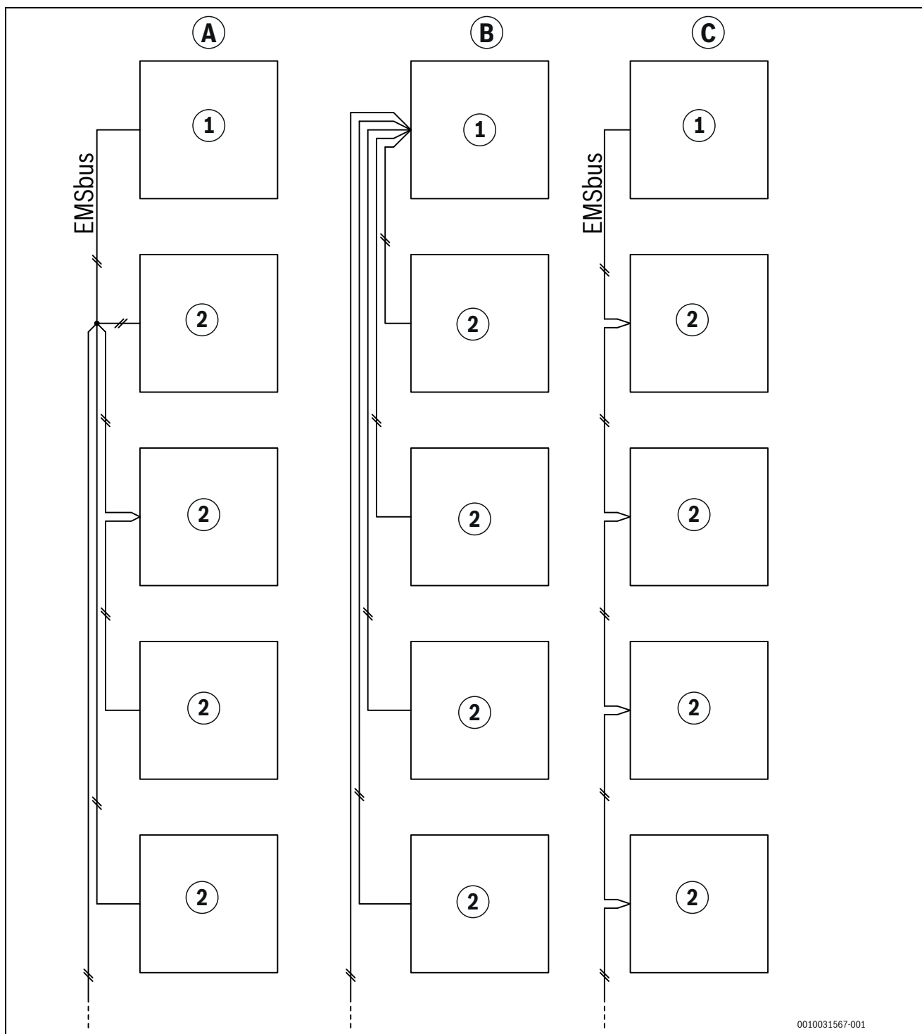
Afb. 35 Aansluitalternatieven voor EMS-bus
