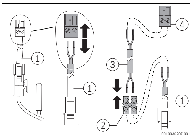
Afb. 37 Aanvoertemperatuursensorkabel verlengen
