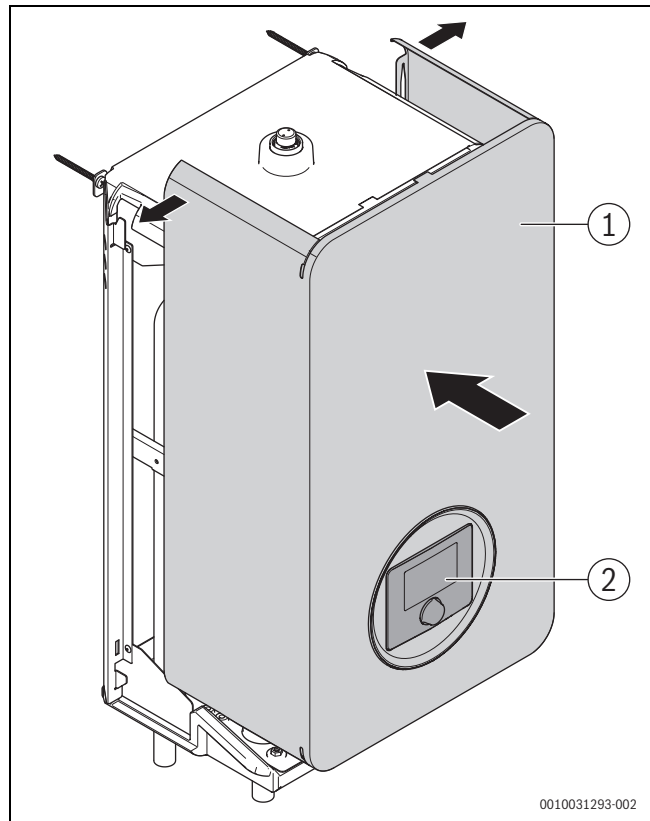
Afb. 16 Afdekkap monteren
