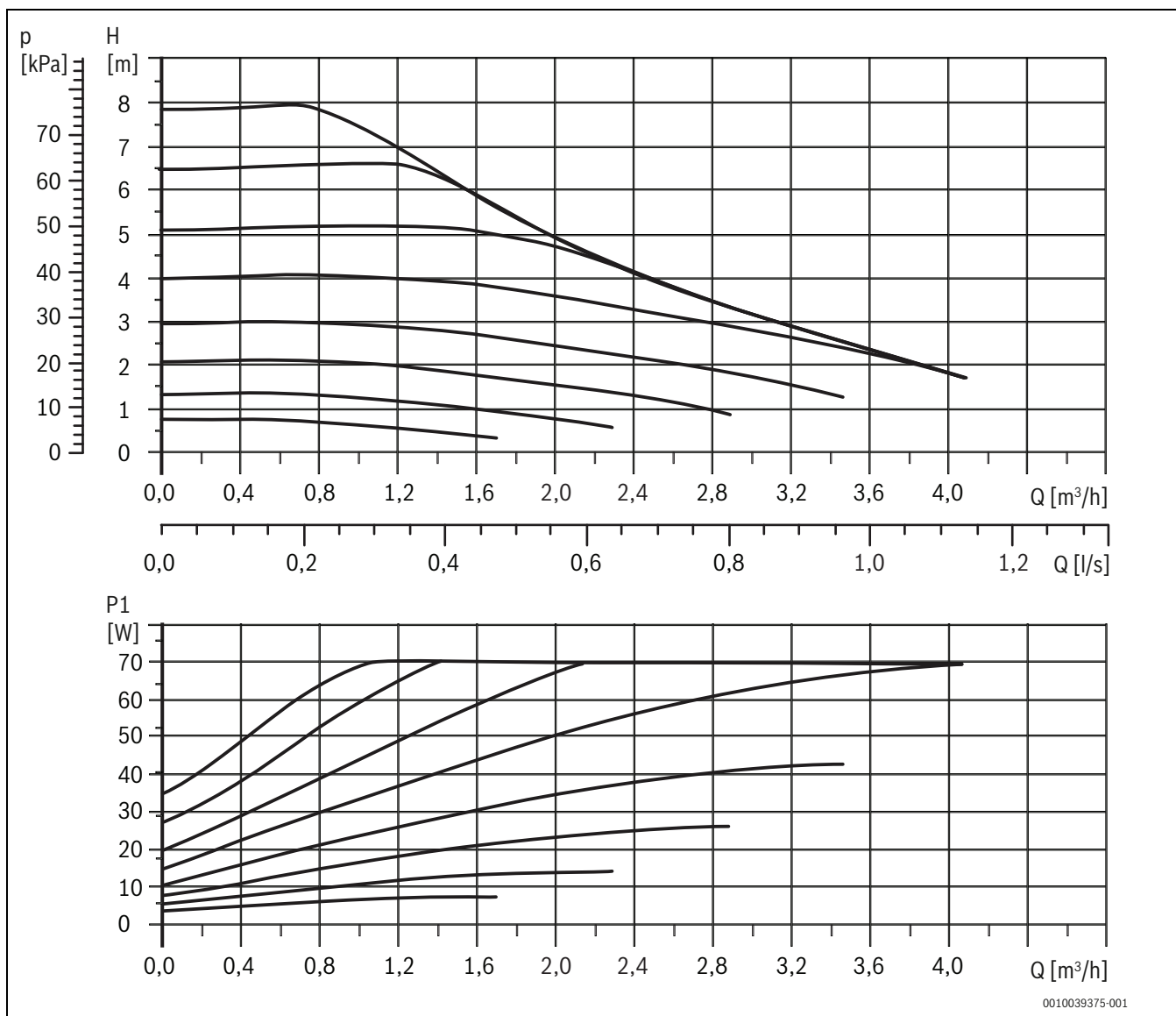
Afb. 21 Opvoercharacteristieken
