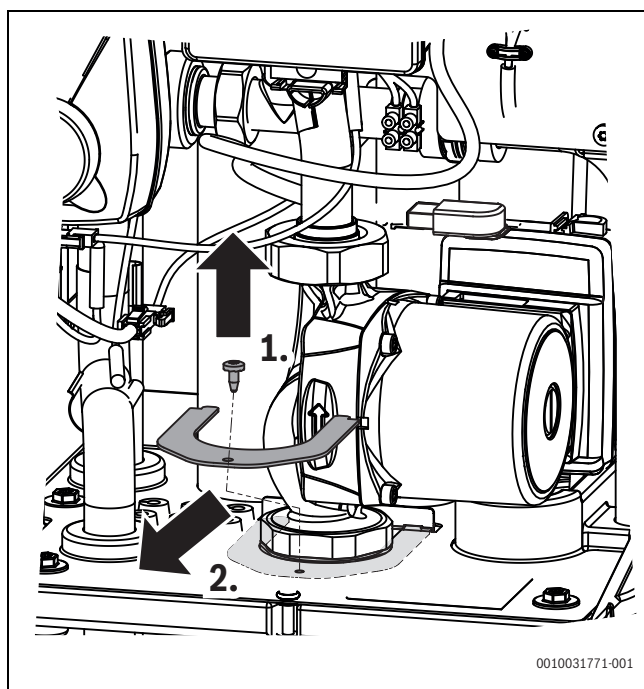
Afb. 41 Borgplaat verwijderen
