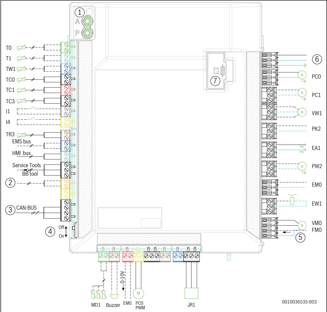
Afb. 48 Aansluitschema installatiemodule
