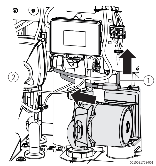
Afb. 40 Stekker aftrekken
