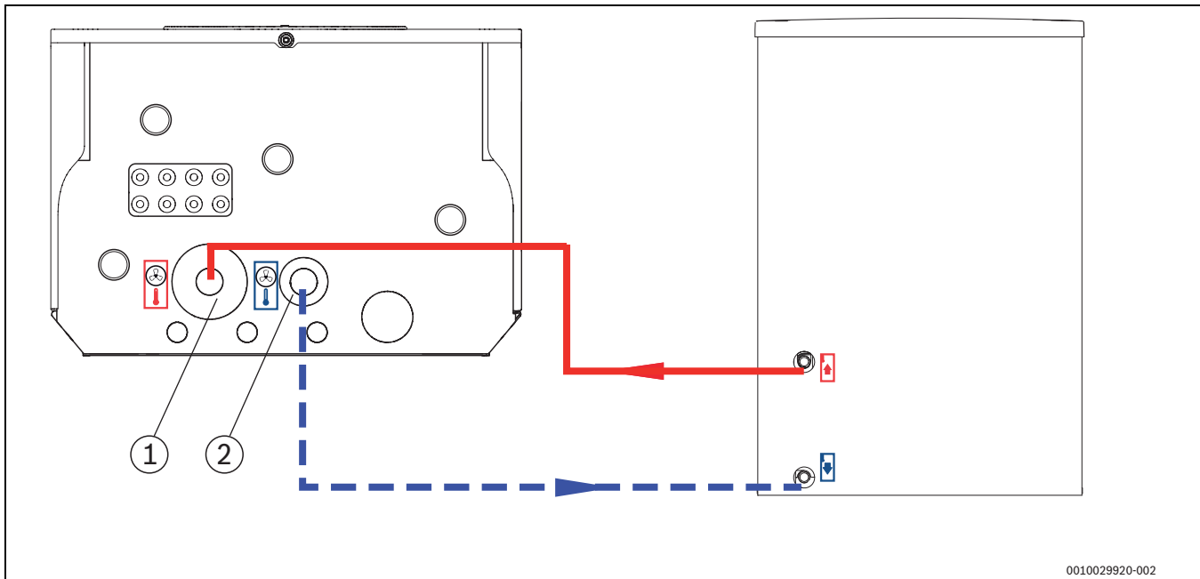
Afb. 20 Aansluiting van de binnenunit aan de buitenunit (principe weergave)
