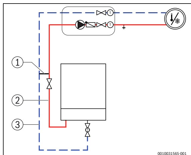
Afb. 8 Binnenunit met cv-circuit en bypass
