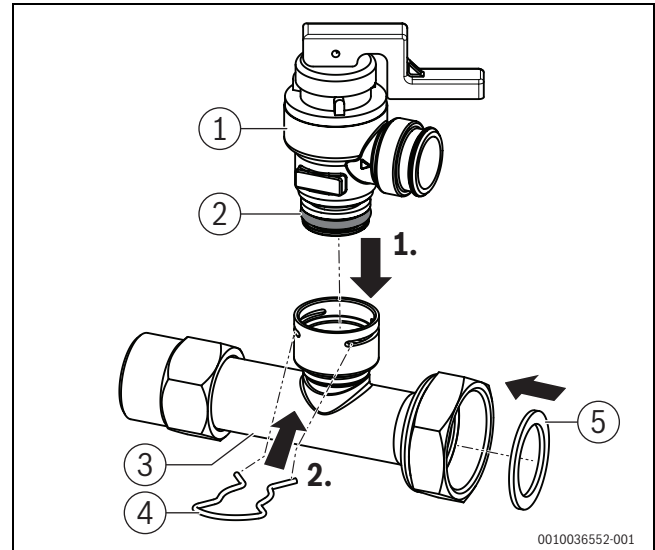
Afb. 6 Montage overstortventiel
