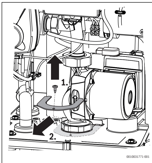
Afb. 38 Borgplaat verwijderen
