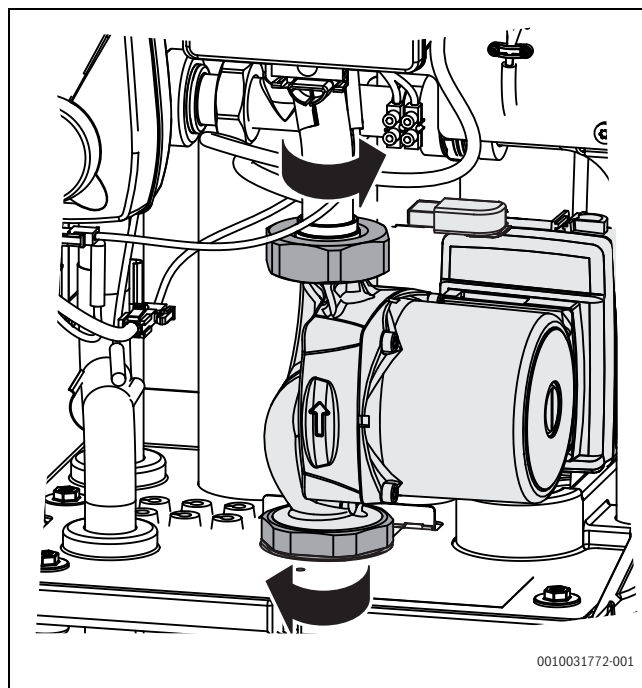
Afb. 39 Wartelmoeren losdraaien
