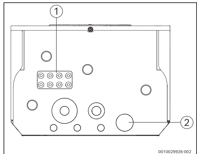
Afb. 25 kabeldoorvoeren
