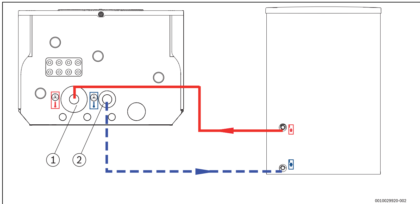
Afb. 19 Aansluiting van de binnenunit aan de buitenunit (principe weergave)
