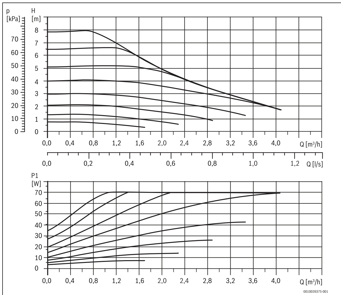
Afb. 20 Opvoercharacteristieken
