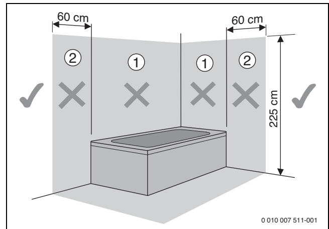
Afb. 24 Veiligheidszones
