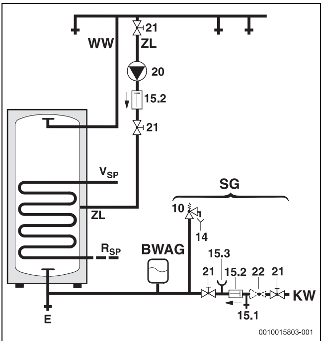
Рис. 1 Схема подключения контура ГВС
