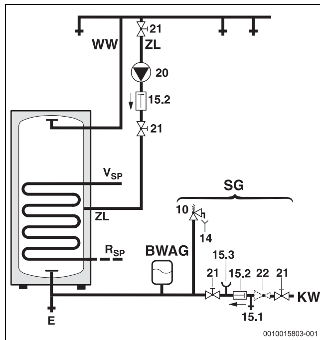
Fig. 1 Esquema de ligação para água sanitária
