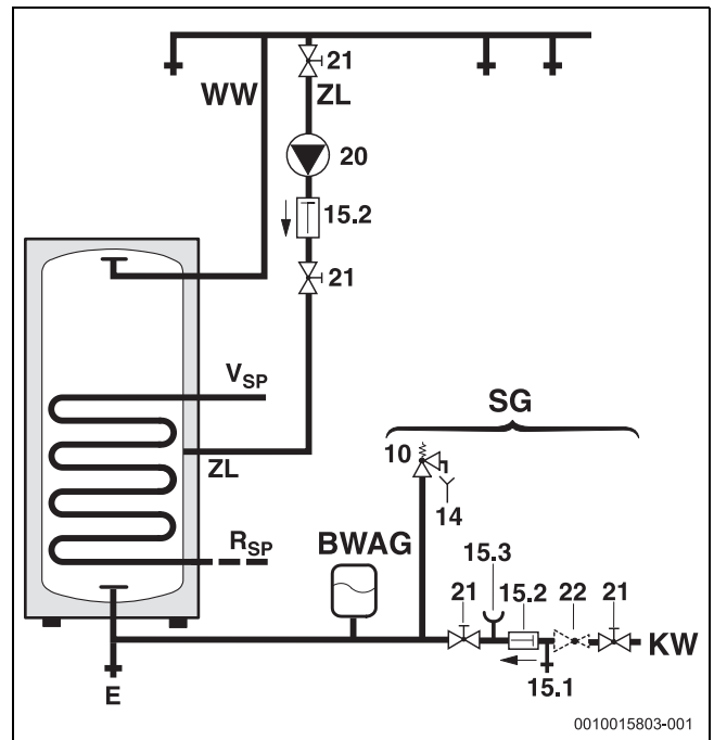
Fig. 1 Aansluitschema drinkwaterzijde
