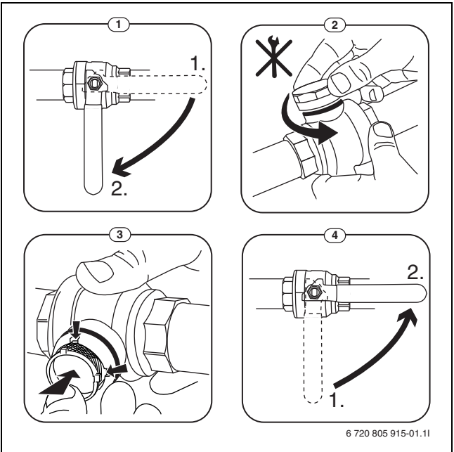
Afb. 8 Filterreiniging
