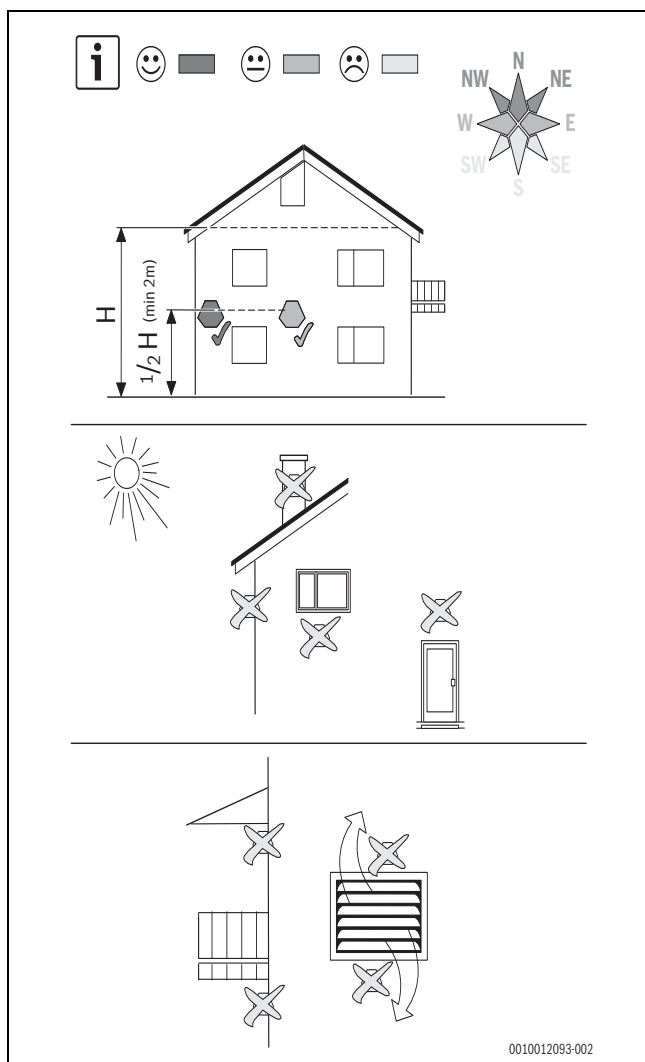
Afb. 19 Positie van de buitentemperatuursensor
