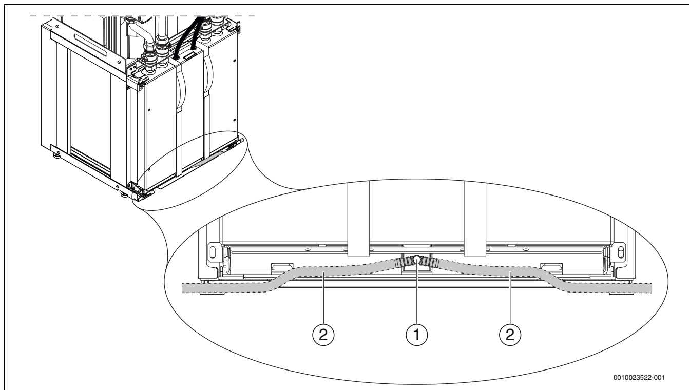
Afb. 14 De aftapslang aansluiten
