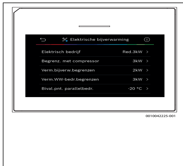
Afb. 37 Instellingen voor elektrische bijverwarming
