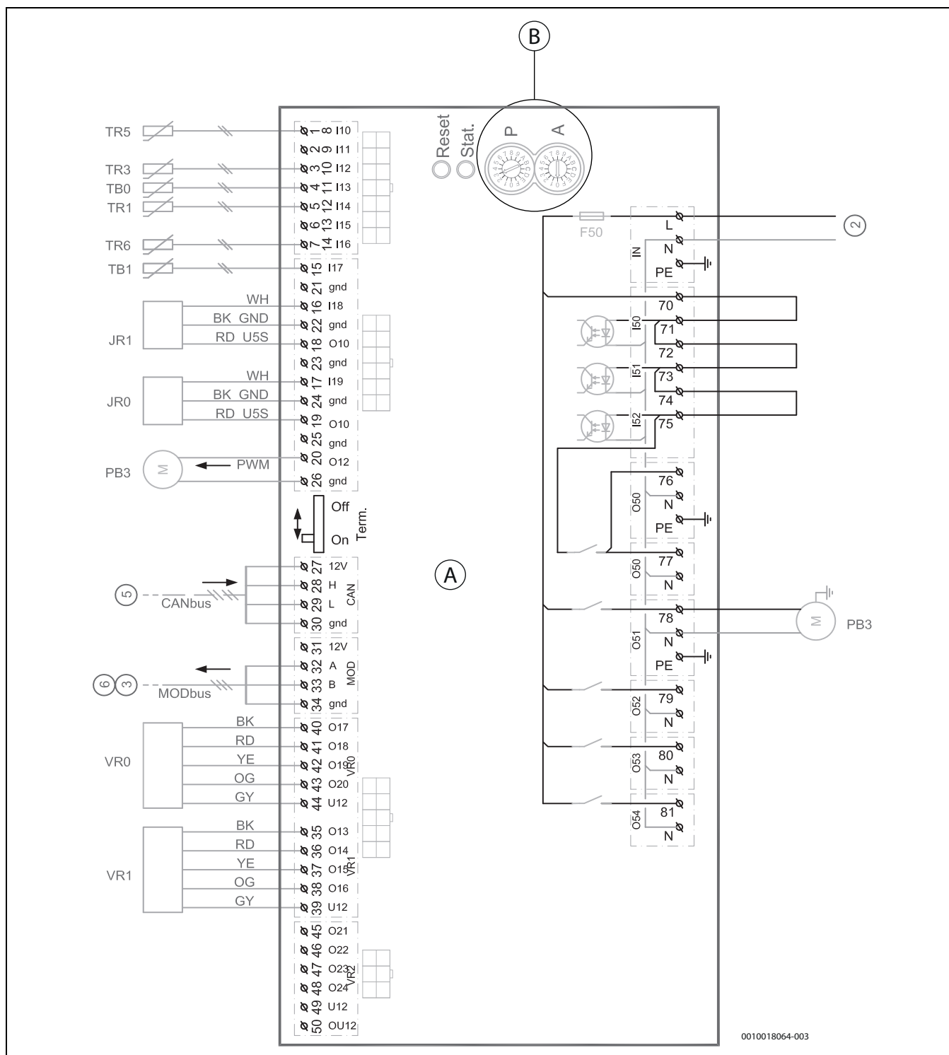
Afb. 52 Schakelschema I/O-module
