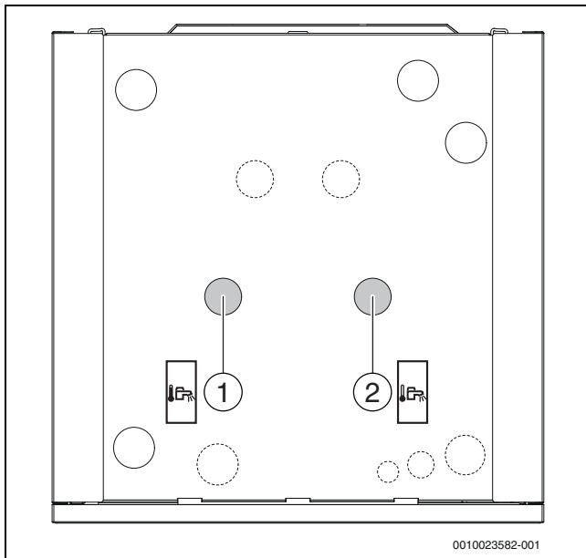
Afb. 17 Wateraansluitingen op de warmtepomp
