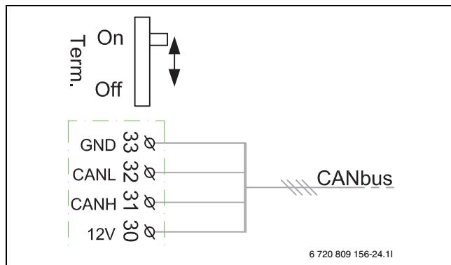
Afb. 18 Afsluiting CAN-BUS
