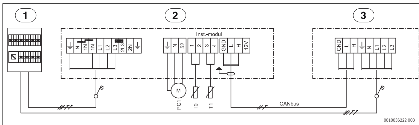
Afb. 39 Elektrisch schema 9 kW 400 V 3 N~, alternatieve schakeling
