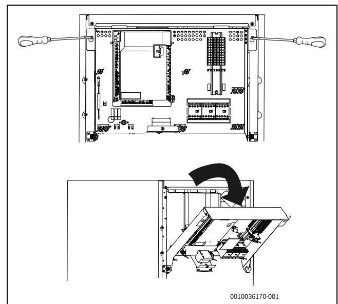
Afb. 19 Kantelen van de aansluitdoos
