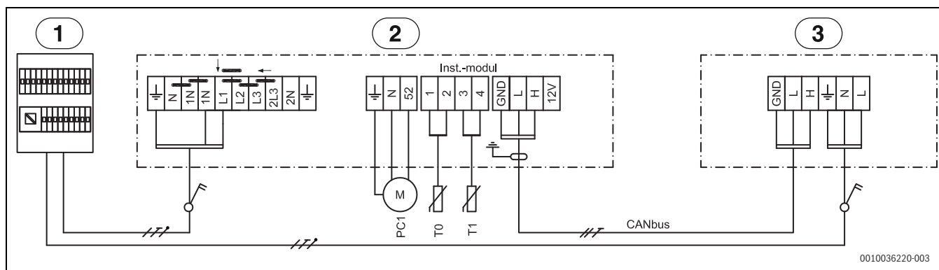
Afb. 37 Elektrisch schema 9 kW 230 V~
