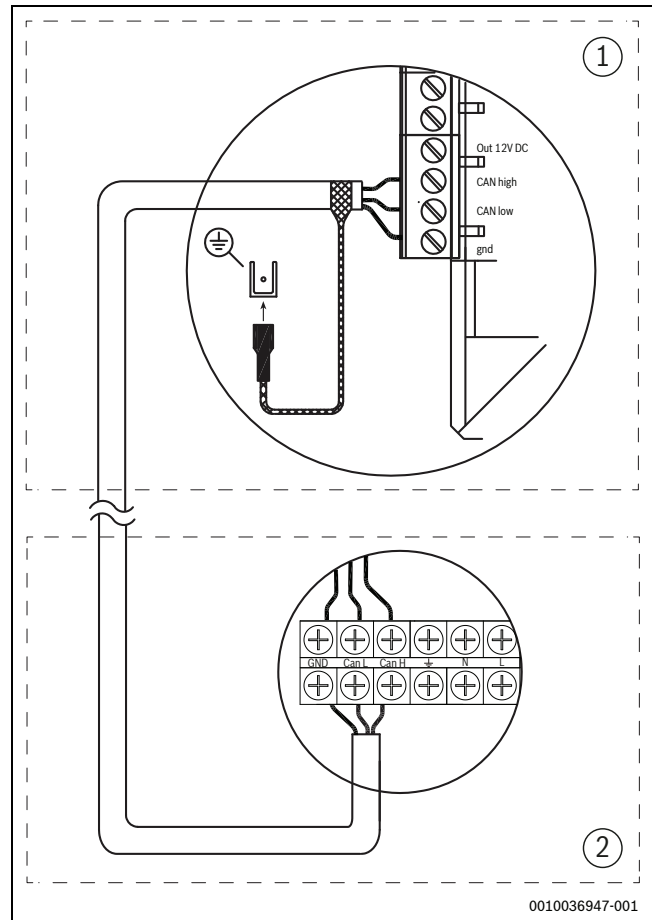
Afb. 13 CAN-BUS-aansluiting
