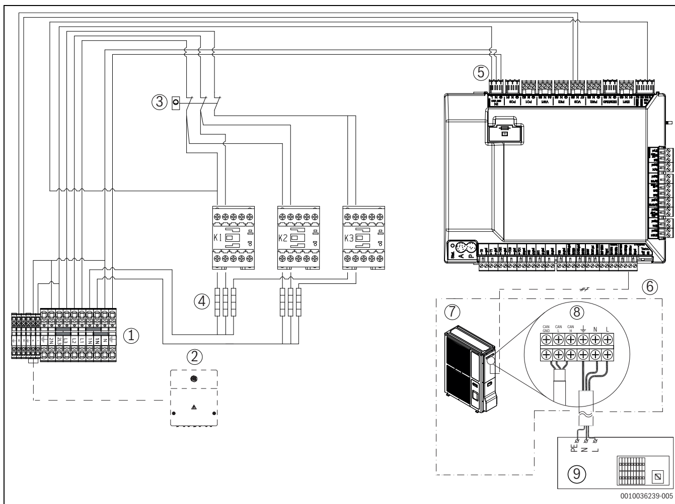
Afb. 40 400 V 3N~ binnenunit met 230 V~ buitenunit
