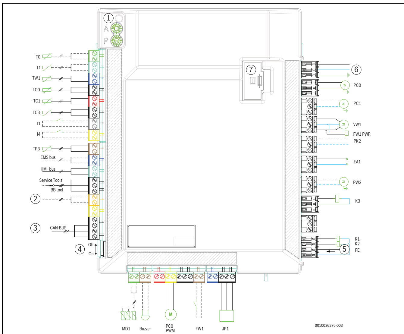
Afb. 35 Installatiemodule van de binnenunit
