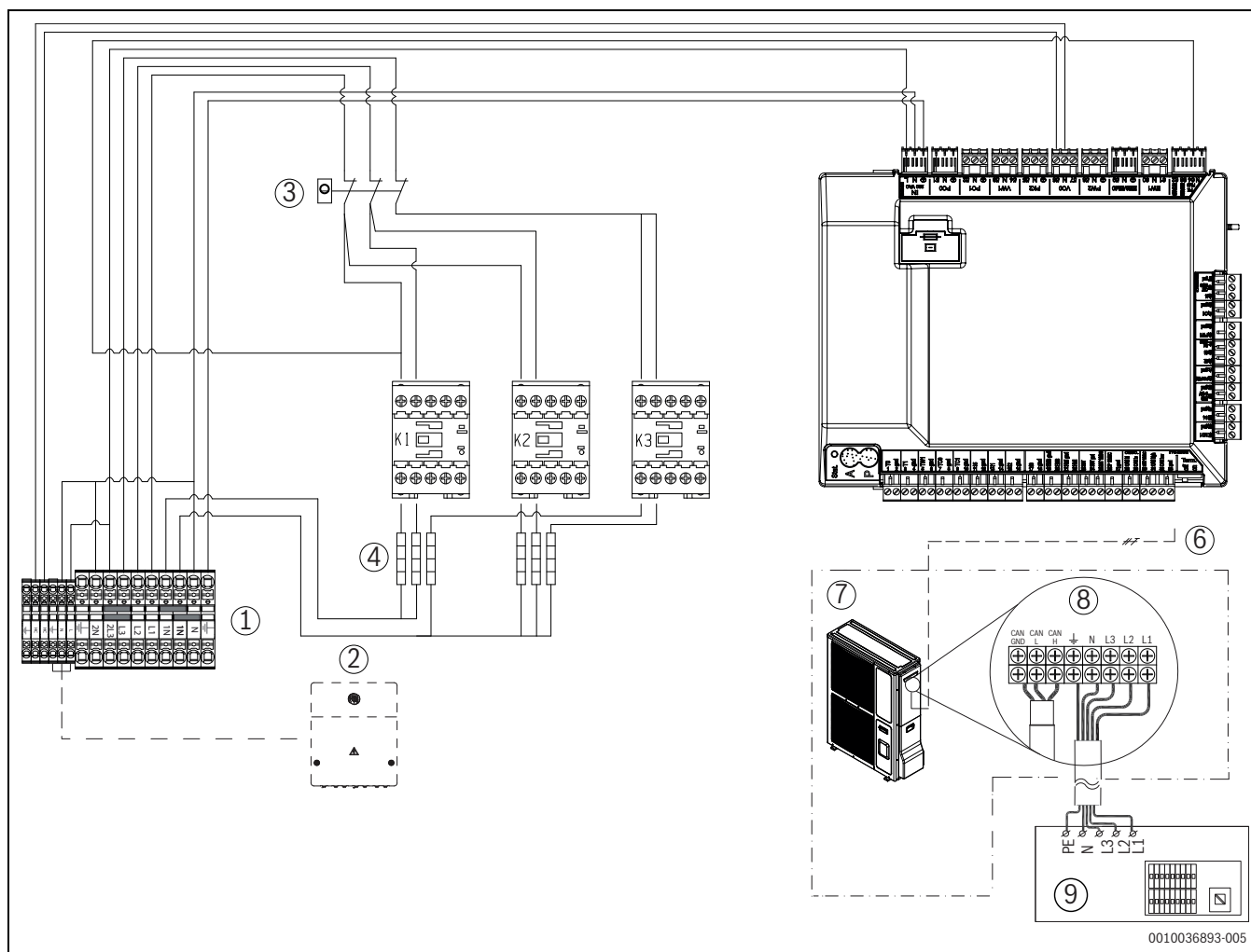
Afb. 41 400 V 3 N~ binnenunit met 400 V 3 N~ buitenunit
