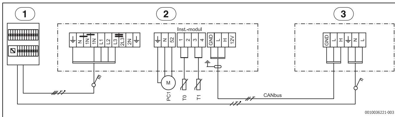
Afb. 38 Elektrisch schema 9 kW 3 N~
