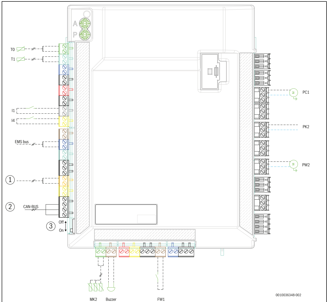
Afb. 12 Installatiemodule van de binnenunit
