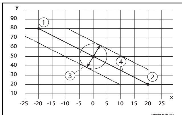
Afb. 4 Weersafhankelijk geregelde stooklijn
