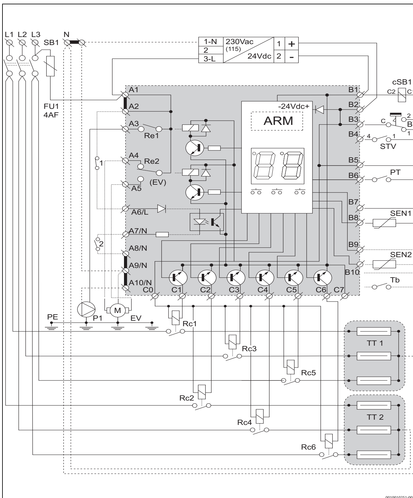
Afb. 21 Bedieningsschema van het cv-toestel Tronic Heat 3500 (15-24 kW), 3x 400/230 V AC
