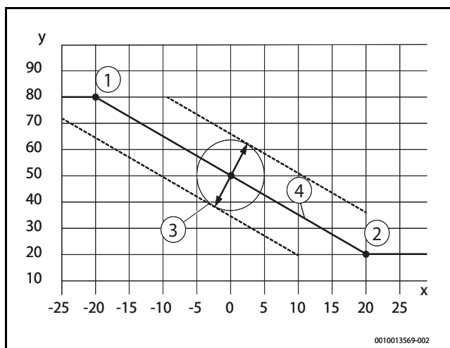
Afb. 35 Weersafhankelijk geregelde stooklijn
