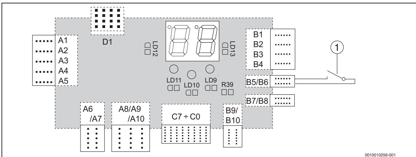
Afb. 23 Aansluiting kamerthermostaat
