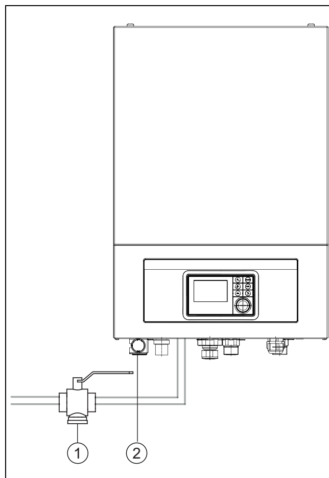
Afb. 6 Binnenunit IDU Monoblock B
