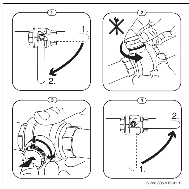
Afb. 7 Filterreiniging
