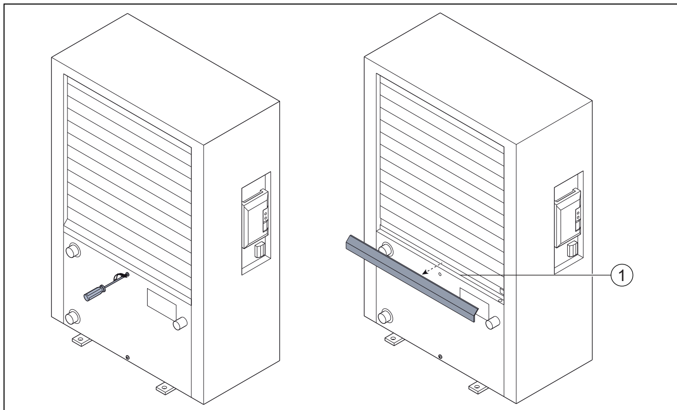
Afb. 8 De condensbak van de buitenunit
