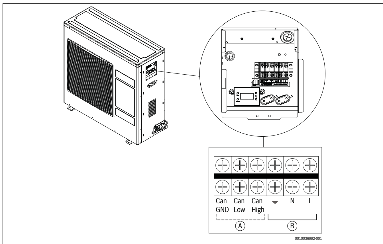
Afb. 19 Kabelaansluitingen
