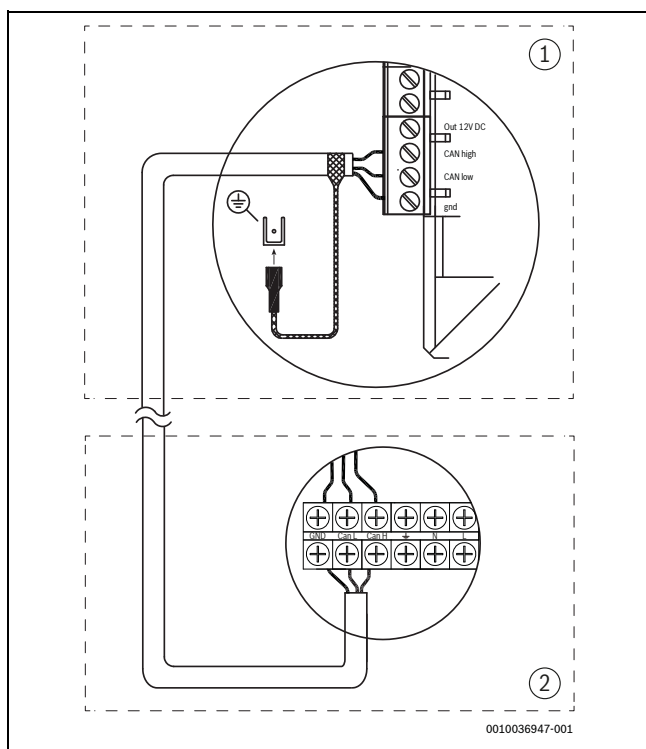
Afb. 20 CAN-BUS-aansluiting
