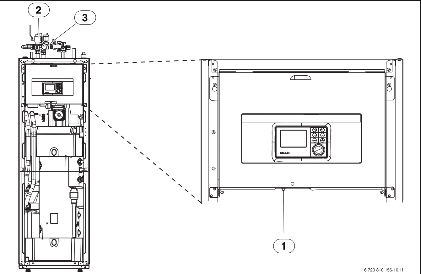
Afb. 5 Binnenunit IDU Split T / TS
