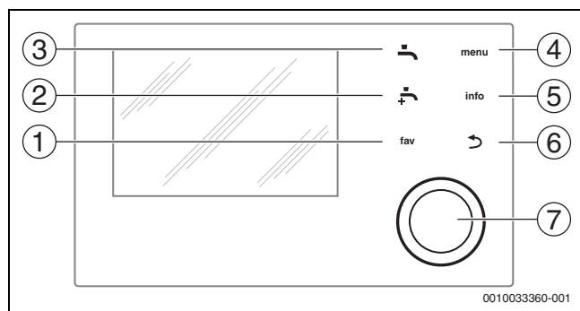
Afb. 3 Bedieningselementen
