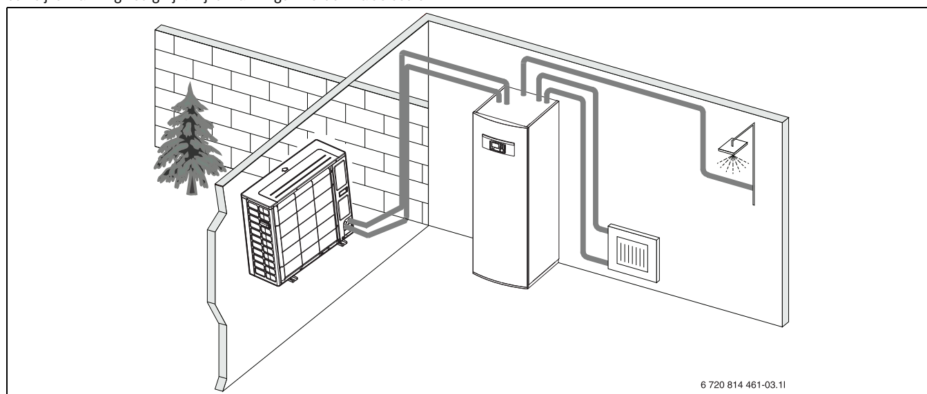
Afb. 2 Warmtepomp buitenunit, binnenunit IDU SplitT/TS met geïntegreerde boiler en elektrische bijverwarming
