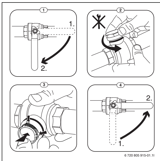
Afb. 7 Filterreiniging
