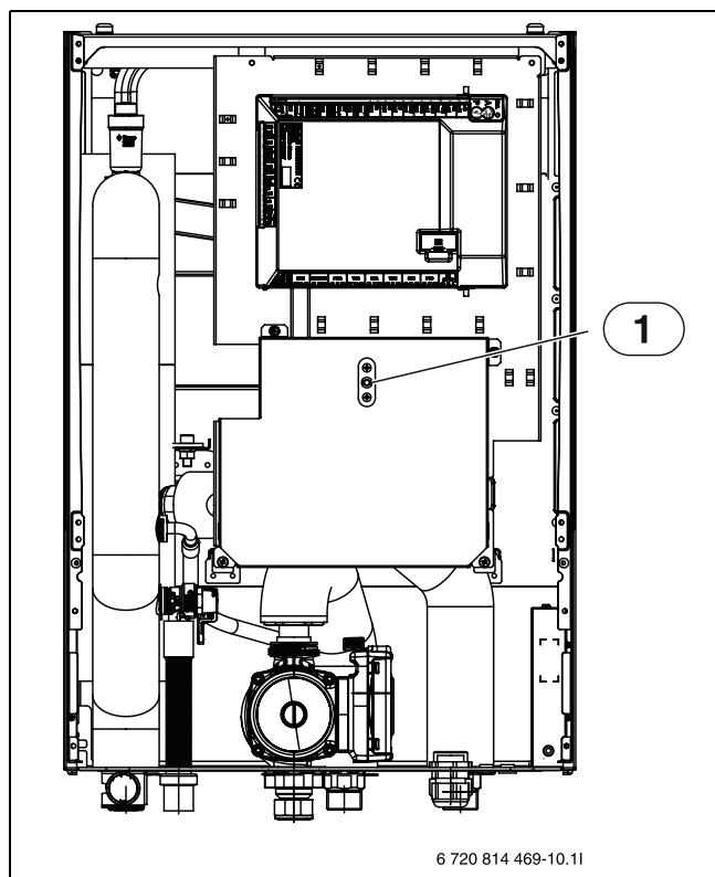
Afb. 6 Binnenunit IDU Split E
