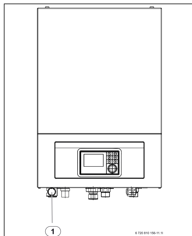
Afb. 5 Binnenunit IDU Split E
