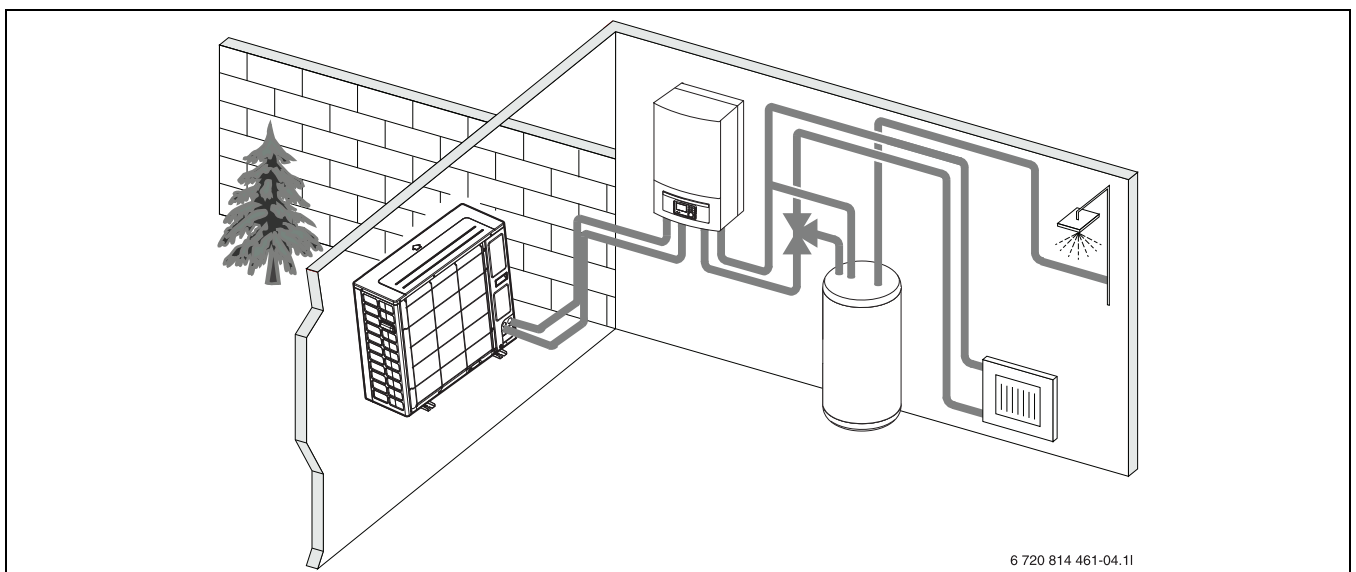
Afb. 2 Warmtepomp buitenunit, binnenunit IDU Split E met elektrische bijverwarming, externe boiler
