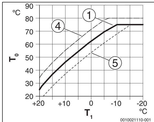
Afb. 5 Instelling van de stooklijn voor radiator Parallelverschuiving via Offset ruimtetemperatuur of gewenste kamertemperatuur
