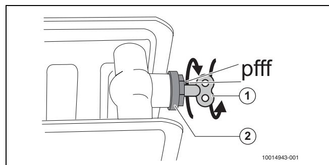
Afb. 9 Ontluchten radiator
