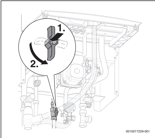
Afb. 3 Gaskraan
