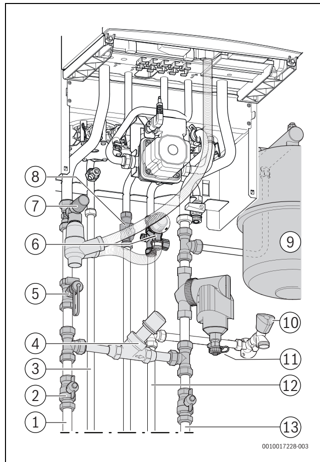
Afb. 2 Overzicht aansluitingen
