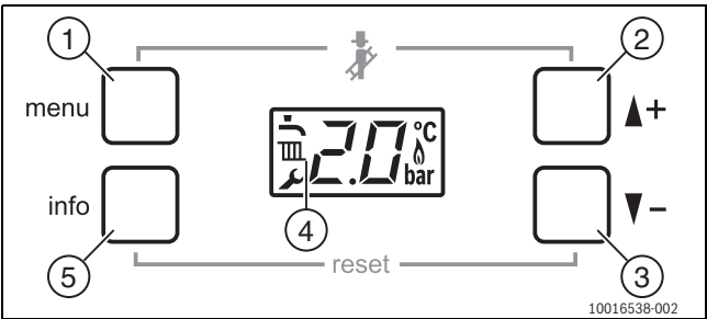
Afb. 6 Bedieningspaneel
