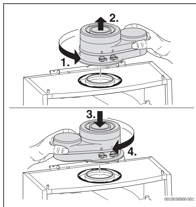
Afb. 6 Omdraaien rookgasafvoeradapter
