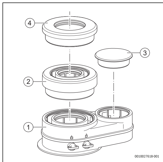
Afb. 5 Opbouw rookgasafvoeradapter
