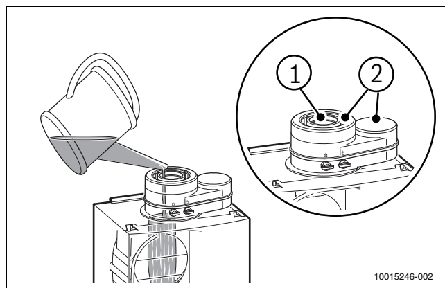
Afb. 22 Vullen toestelsifon
