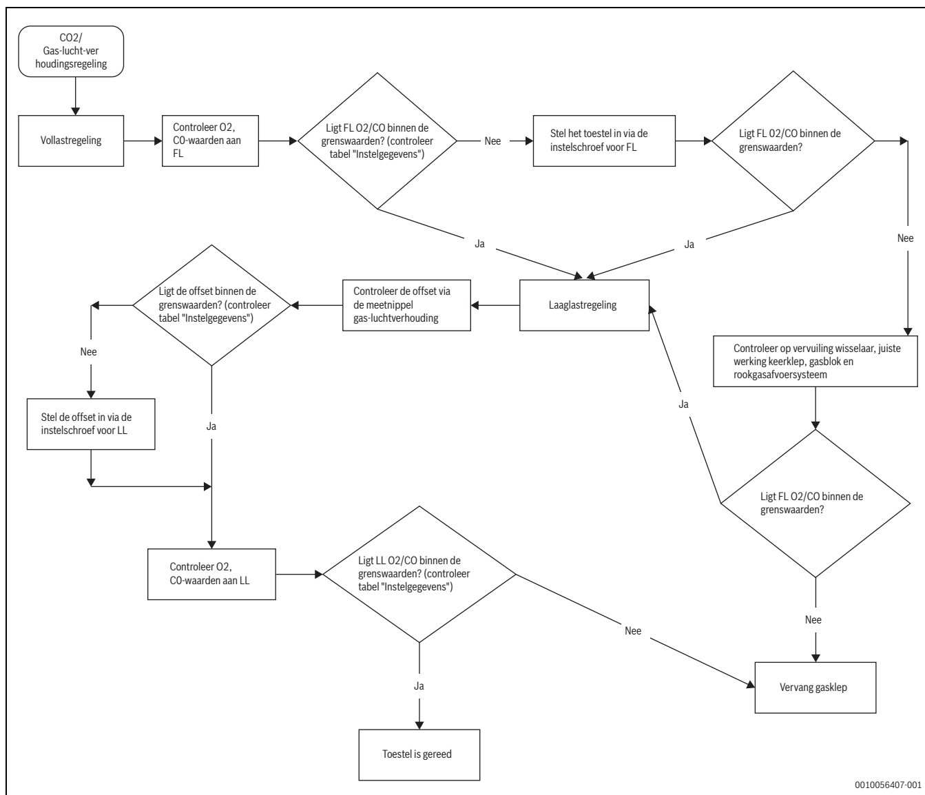
Afb. 34 Flowchart instelinstructies
