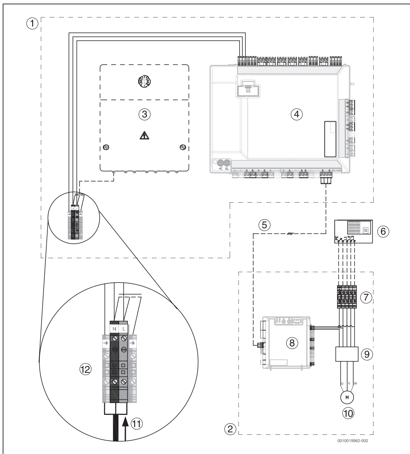
Afb. 33 Driefasige warmtepomp en binnenunit met externe bijverwarming
