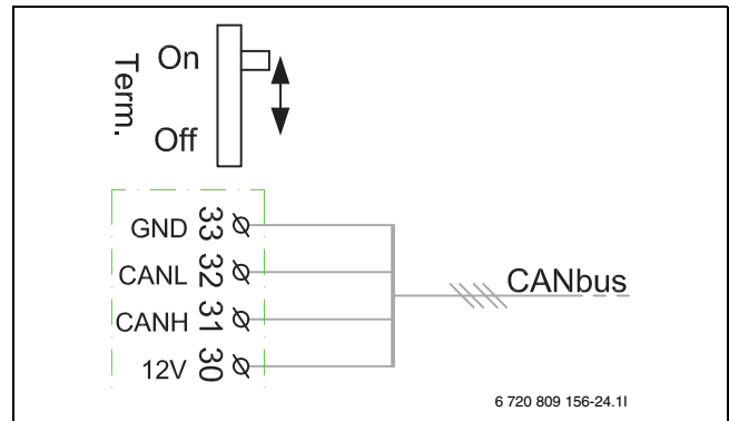
Afb. 9 CAN-BUS-afsluiting
