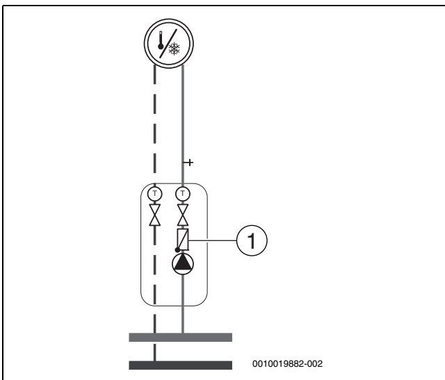
Afb. 29 Cv-groep
