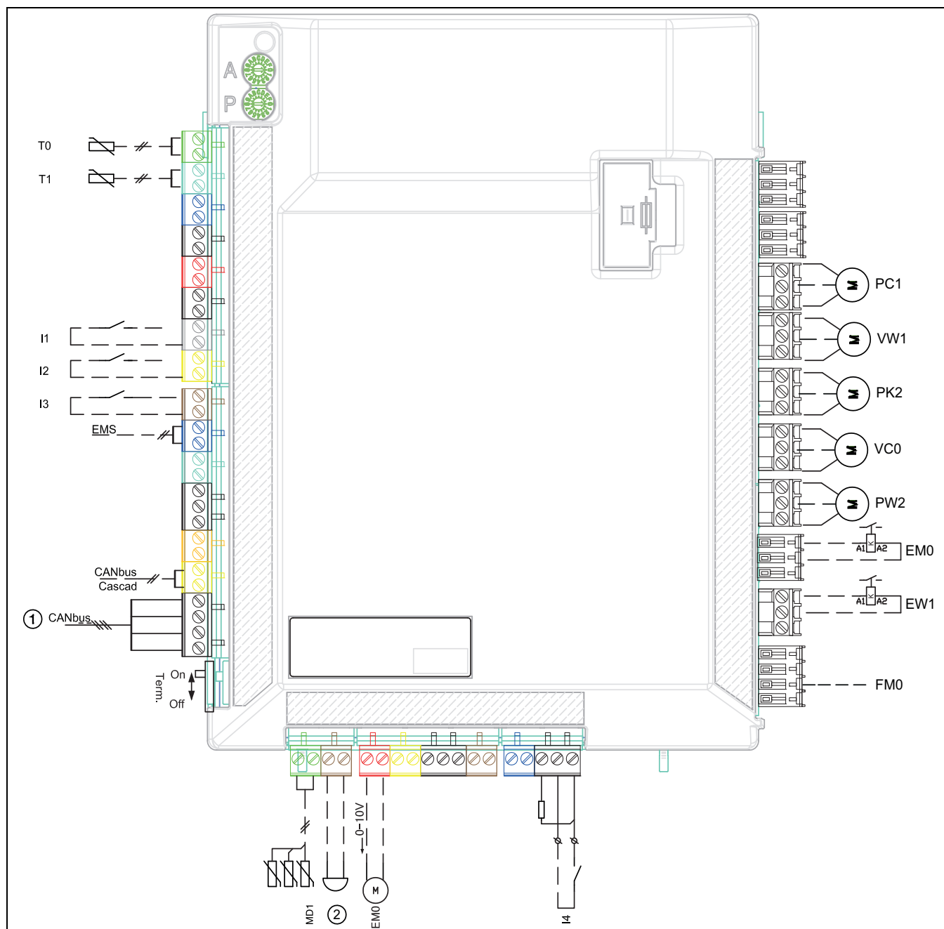
Afb. 12 Aansluitingen installatiemodule
