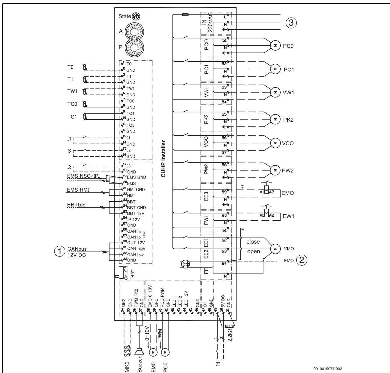
Afb. 34 Elektrische schema installatiemodule voor binnenunit met mengers voor externe bijverwarming
