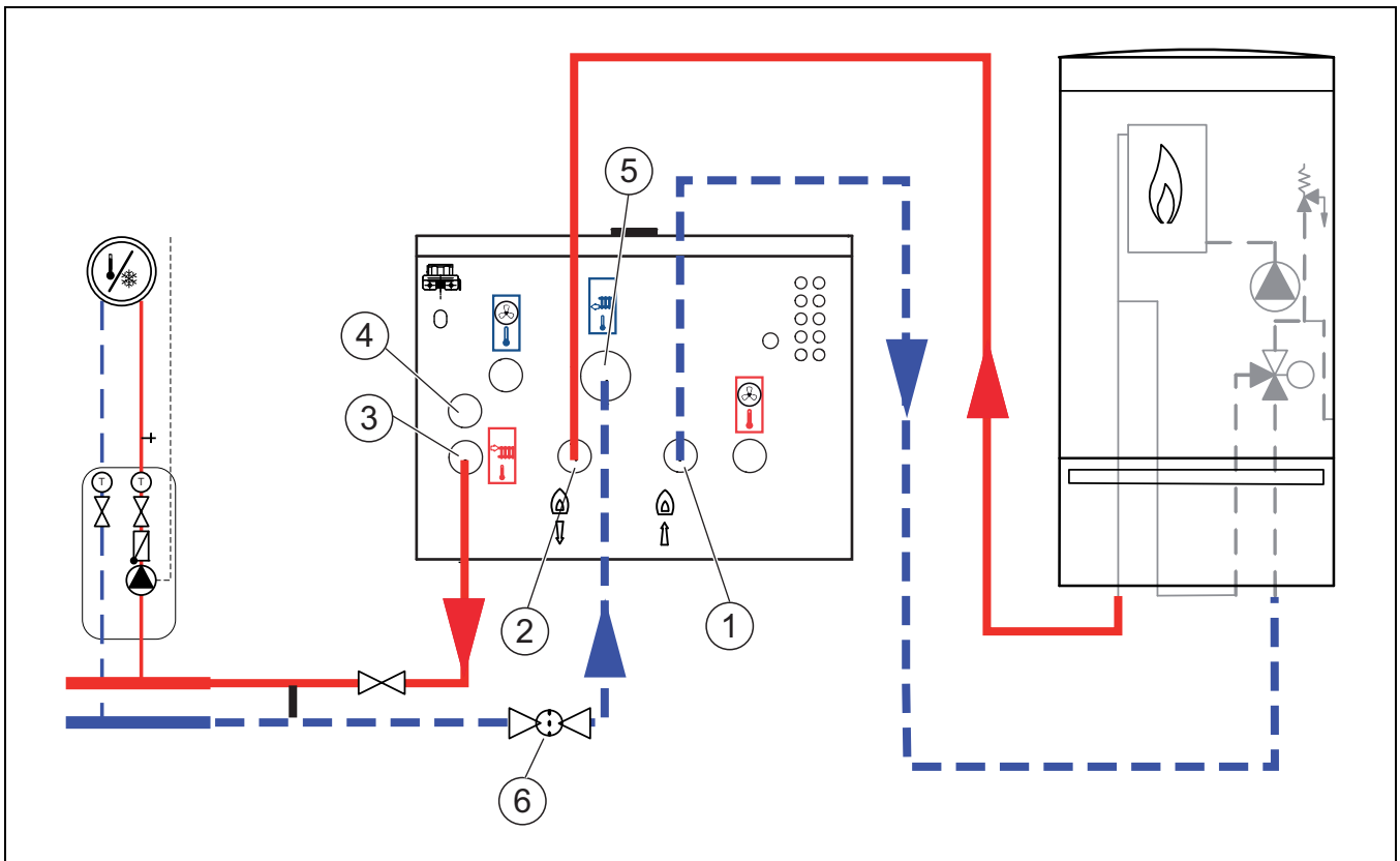
Afb. 7 Aansluiting van de binnenunit met mengers voor externe bijverwarming op de cv-installatie en de bijverwarming
