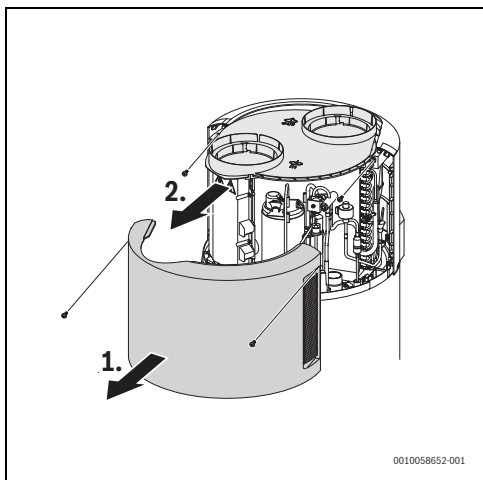
Afb. 24 Verwijder het bovenmantel
