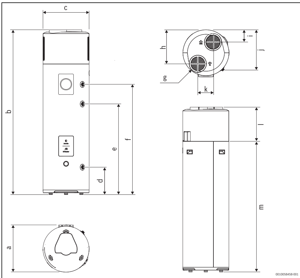
Bild 3 Geräteabmessungen
