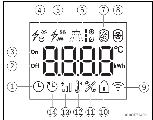
Fig. 19 Interface utilisateur - symboles à l'écran
