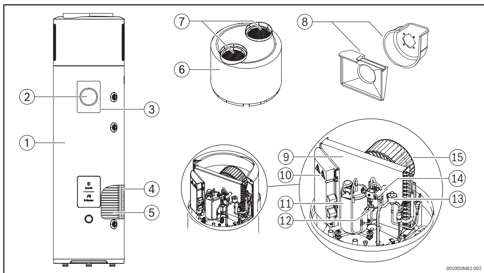
Afb. 4 Productoverzicht
