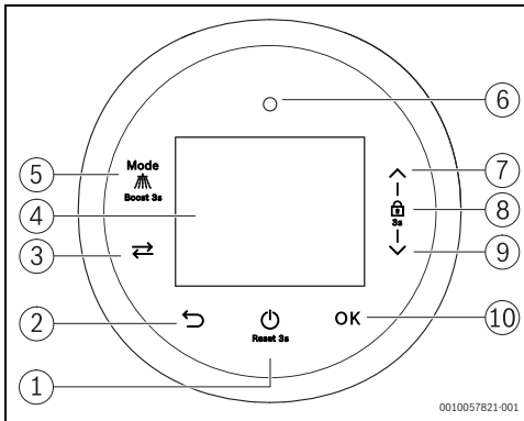
Bild 18 Bedienfeld
