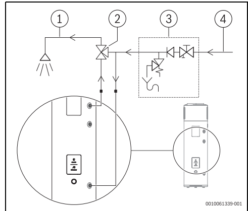
Afb. 14 Watertoevoeraansluitingen
