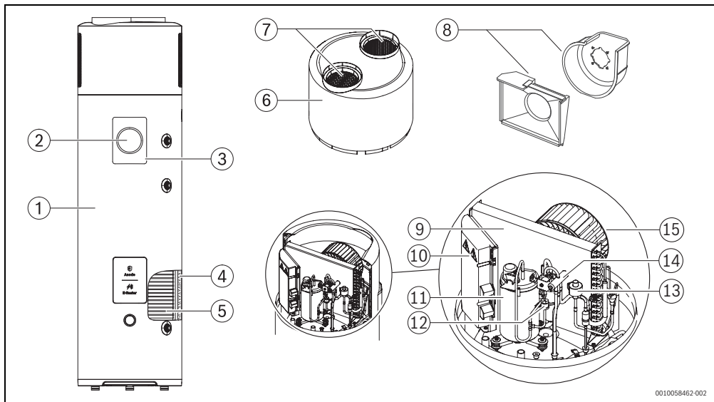
Bild 4 Produktübersicht
