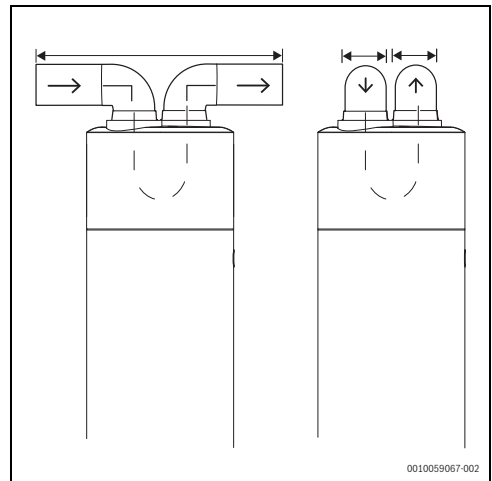
Afb. 11 Tweede speciale ventilatieschacht
