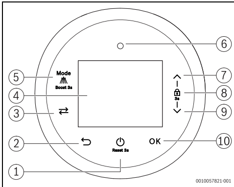
Afb. 18 Bedieningspaneel
