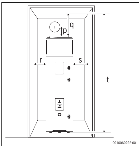
Fig. 9 Espacements minimaux
