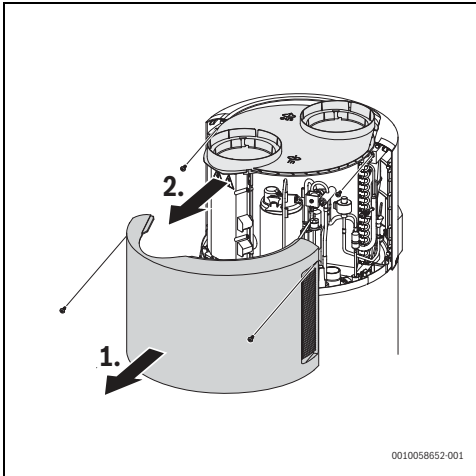
Afb. 24 Verwijder de bovenste afdekking
