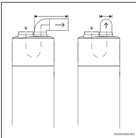
Fig. 10 Conduit d'air dédié
