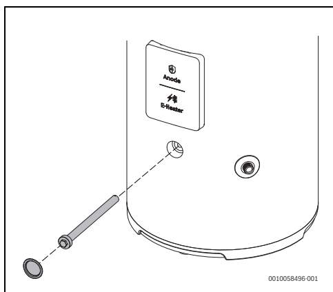
Fig. 25 Retirer l'anode en magnésium
