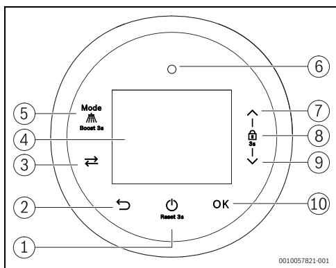
Afb. 18 Bedieningspaneel
