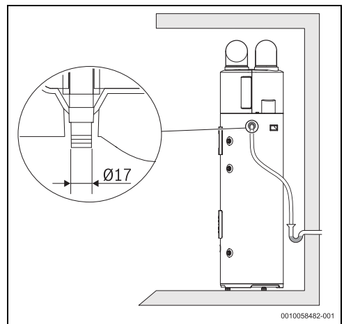
Afb. 15 Aansluiting van de condensafvoer
