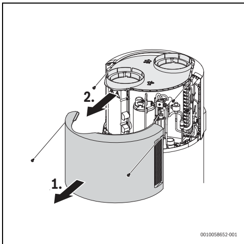
Bild 24 Obere Abdeckung demontieren
