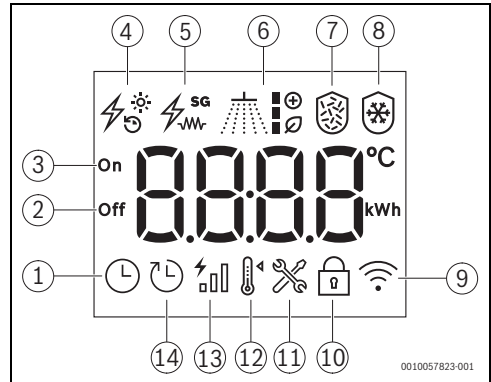
Afb. 19 Gebruikersinterface - symbolen op het display
