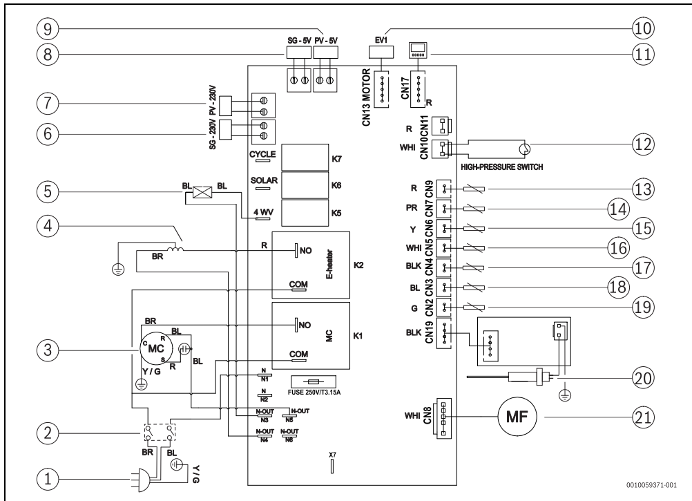
Bild 27 Schaltplan
