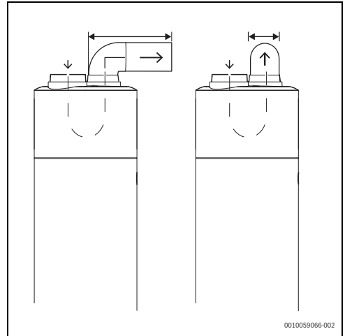
Afb. 10 Speciaal luchtkanaal
