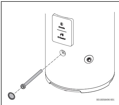
Afb. 25 Demonteren van de magnesiumanode
