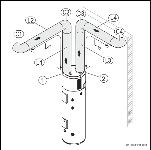
Afb. 13 Installatievoorbeeld
