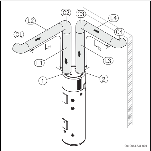
Bild 12 Installationsbeispiel
