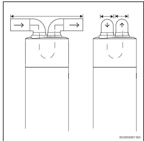
Bild 11 Zweite Luftleitung
