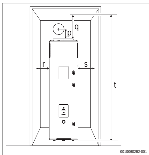
Afb. 9 Minimale afstanden
