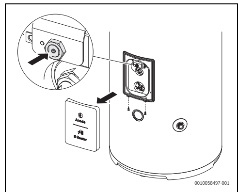
Bild 26 Sicherheitsthermostat zurücksetzen
