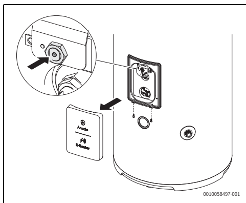
Fig. 26 Réinitialisation du thermostat de sécurité
