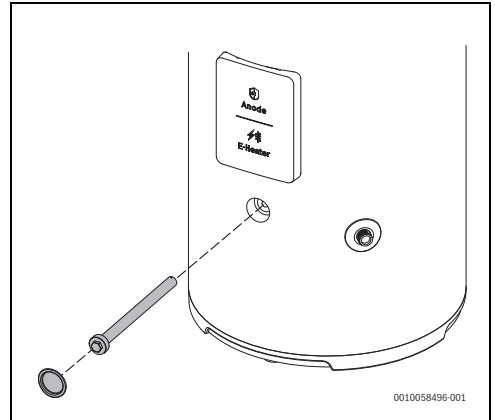
Afb. 25 Verwijderen van de magnesiumanode
