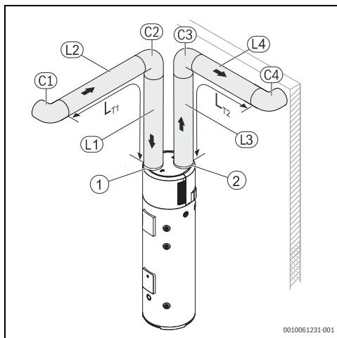
Afb. 12 Installatievoorbeeld
