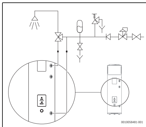
Afb. 14 Watertoevoeraansluitingen
