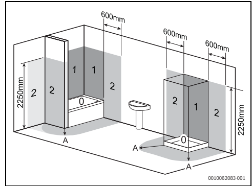
Afb. 8 Aanbevolen minimumafstanden (mm)
