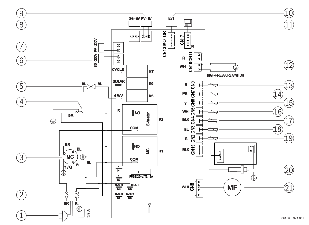
Fig. 27 Schéma électrique
