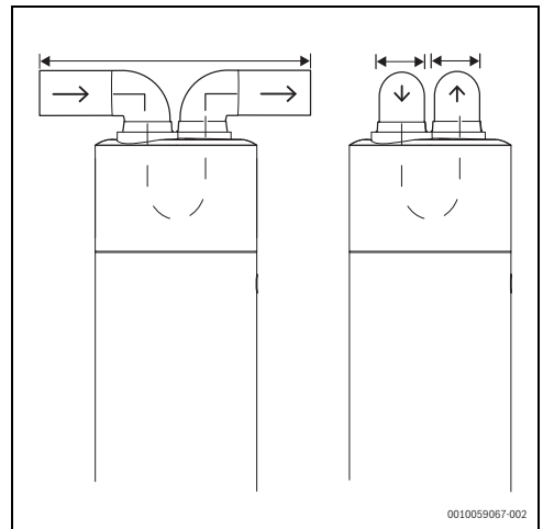
Afb. 11 Tweede speciale ventilatieschacht
