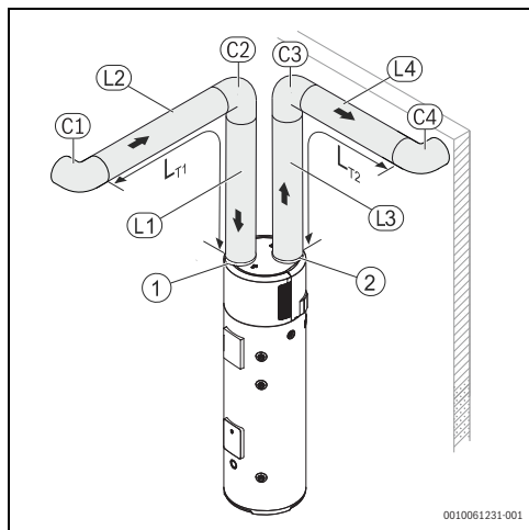
Fig. 12 Exemple d'installation
