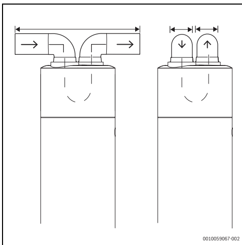
Fig. 11 Deuxième puits d'aérage dédié
