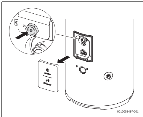
Afb. 26 Resetten van de maximaalthermostaat
