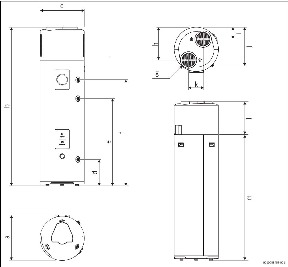
Afb. 3 Toestelafmetingen
