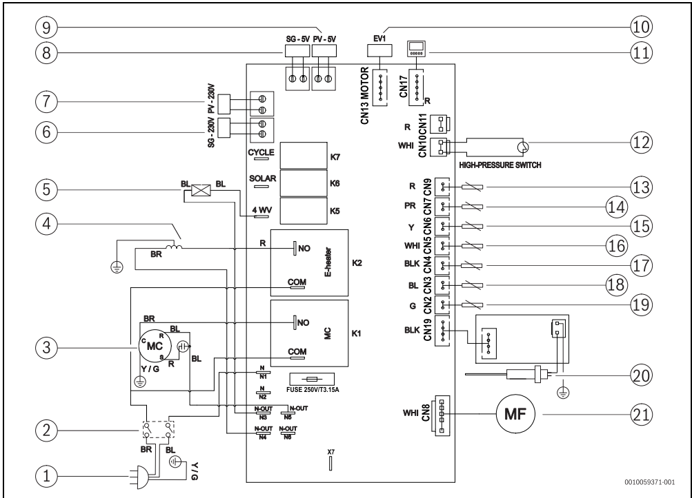
Afb. 27 Elektrisch schema
