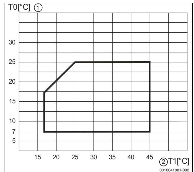
Afb. 6 Warmtepomp in koelmodus
