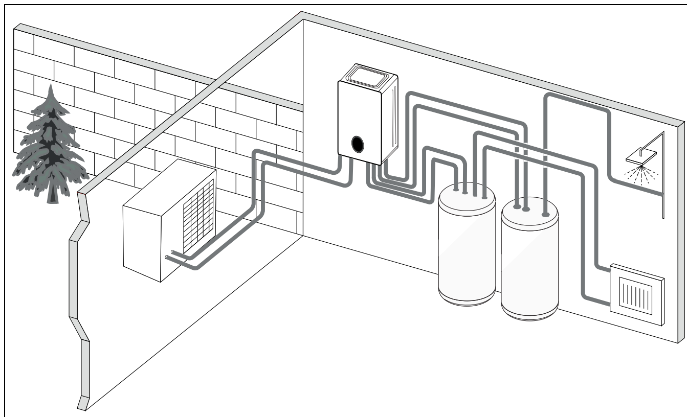
Afb. 8 Warmtepomp AW OR, binnenunit Compress 5800i 12 E met verwarmingstaaf en externe boiler
