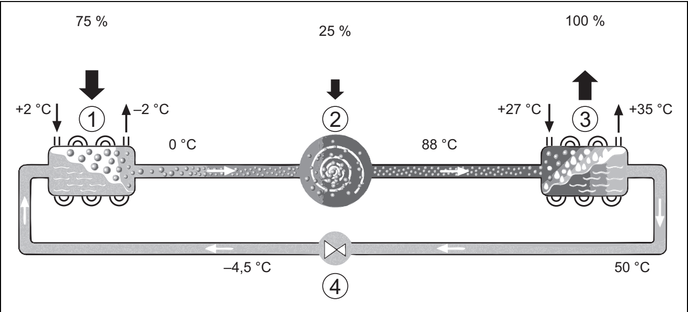
Afb. 7 Werkingssprincipe van het koelmiddelcircuit in de warmtepomp
