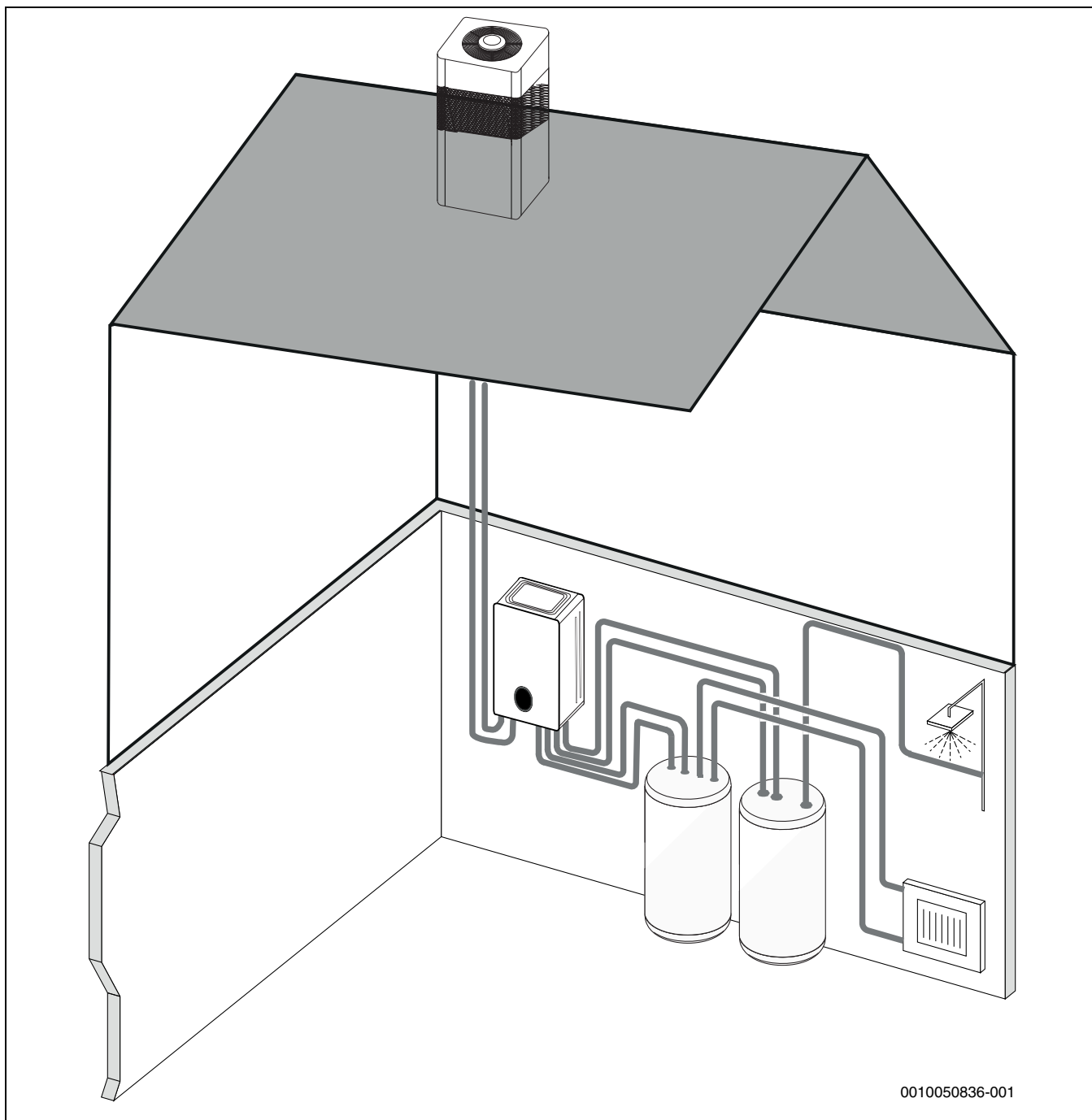
Afb. 9 Warmtepomp AWR, binneneenheid Compress 5800i 12 E met verwarmingsstaaf en externe boiler
