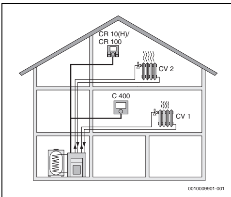
Afb. 2 CR 10 (H) / CR 100 als afstandsbediening voor de tweede cv-groep (HK 2) en C 400/C 800 als regelaar voor de eerste cv-groep (HK 1)
