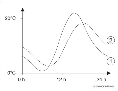
Afb. 15 Voorbeeld voor de gedempte buitentemperatuur
