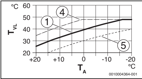
Afb. 17 Instelling van de stooklijn voor vloerverwarming Parallelle verschuiving via Offset ruimtetemperatuur of gewenste kamertemperatuur
