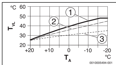
Afb. 16 Instelling van de stooklijn voor vloerverwarming Stijging via dimensioneringstemperatuur T_{AL} en minimale buitentemperatuur T_{A,min}
