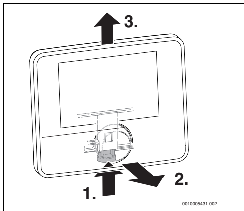
Afb. 9 Bedieningsunit afnemen
