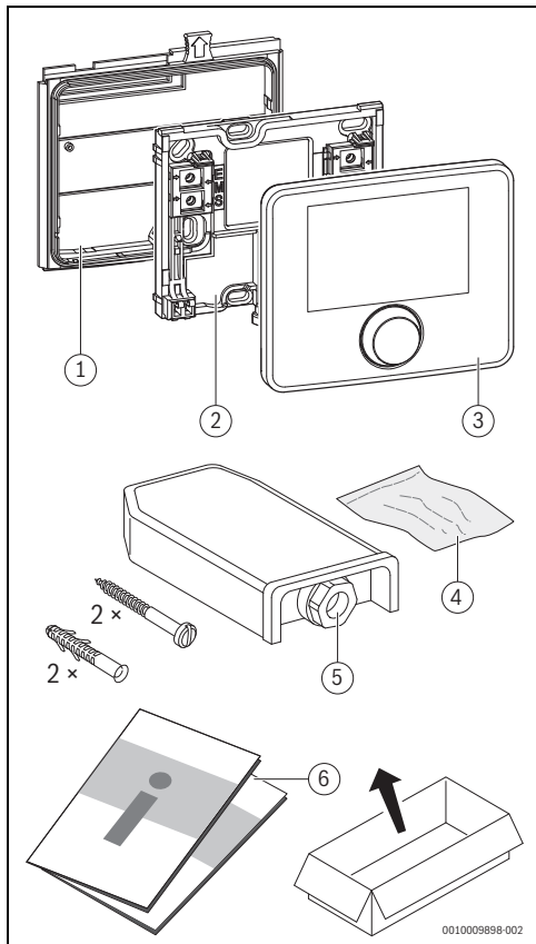
Afb. 3 Leveringsomvang
