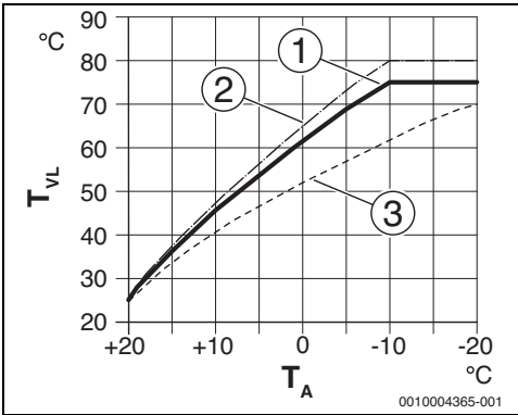
Afb. 18 Instelling van de stooklijn voor radiator Stijging via dimensioneringstemperatuur T_{AL} en minimale buitentemperatuur T_{A,\min}
