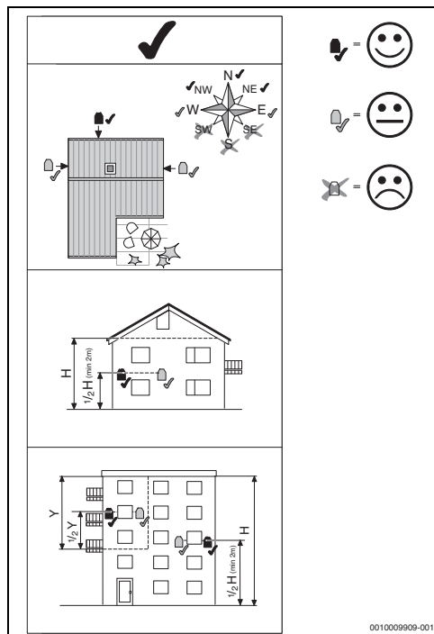
Afb. 13 Geschikte installatieplaats van de buitentemperatuursensor
